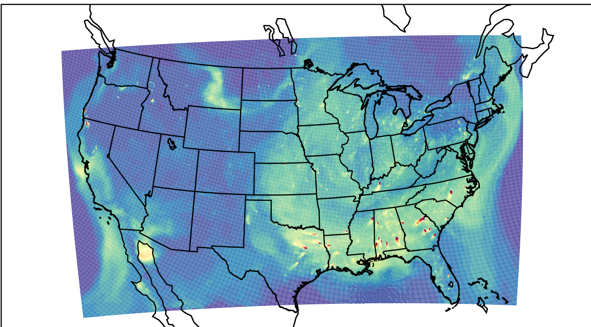
WRF 2023-09-14_23:00:00
