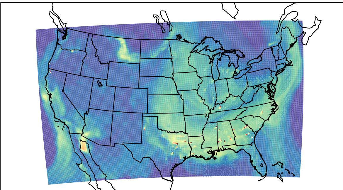
WRF 2023-09-14_20:00:00
