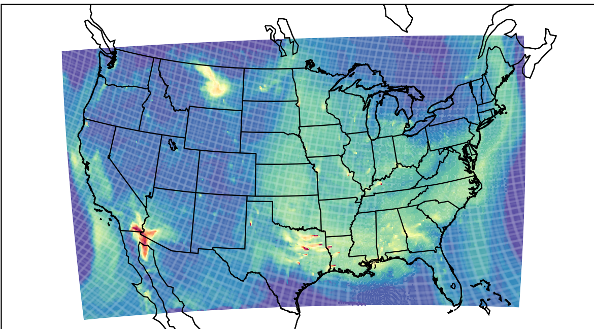
WRF 2023-09-14_16:00:00
