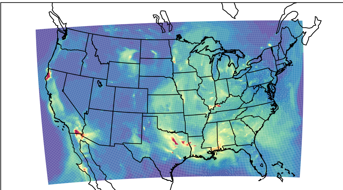
WRF 2023-09-15_10:00:00
