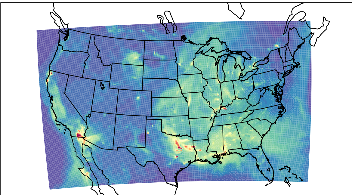
WRF 2023-09-15_13:00:00
