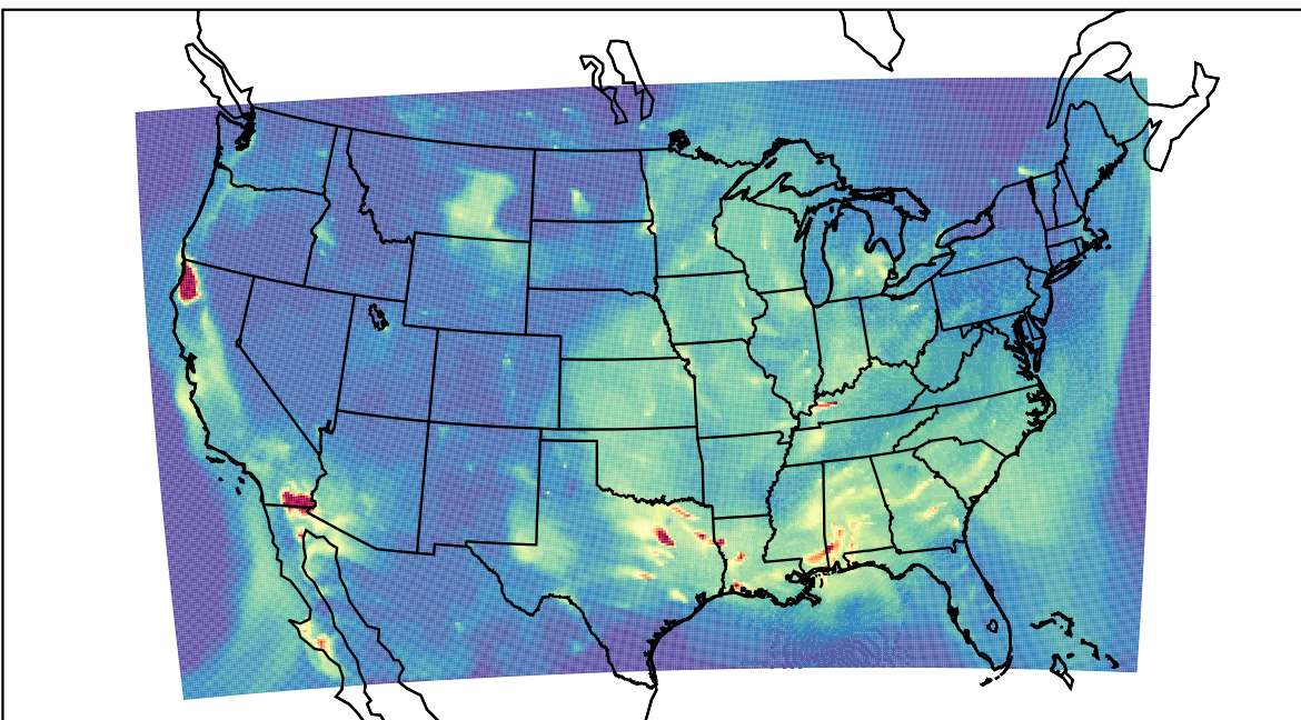
WRF 2023-09-15_06:00:00
