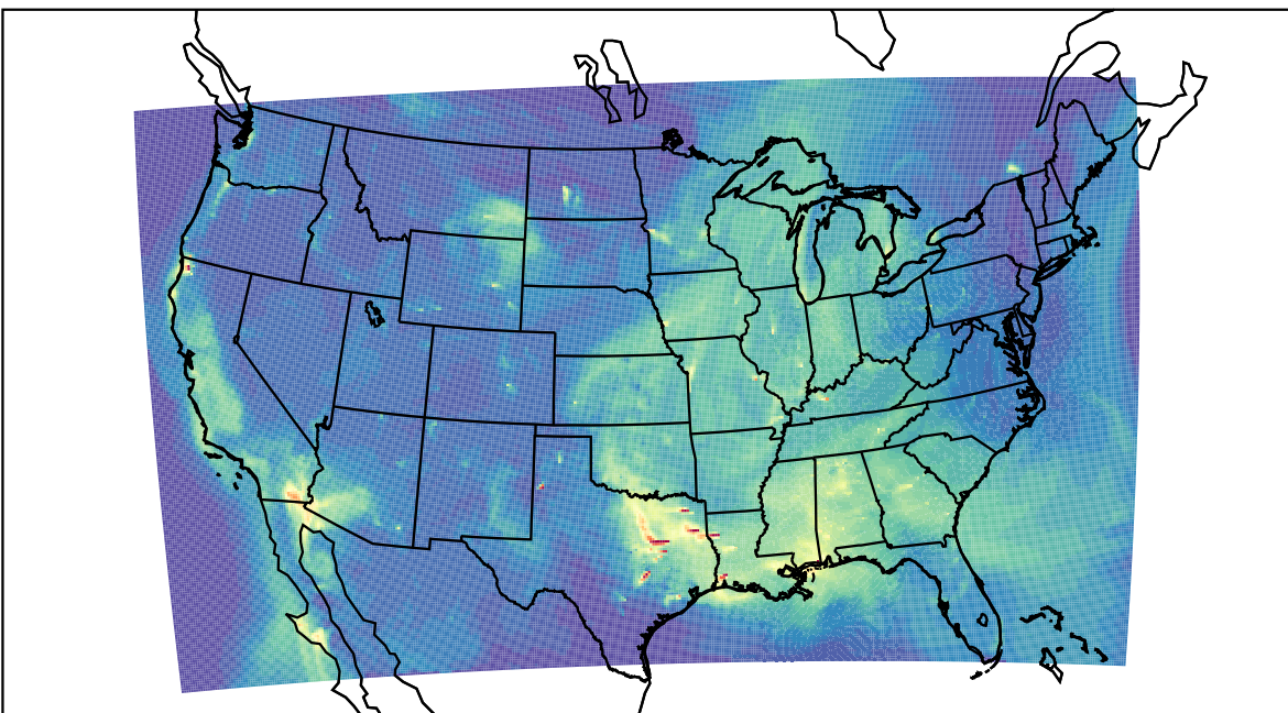
WRF 2023-09-15_16:00:00
