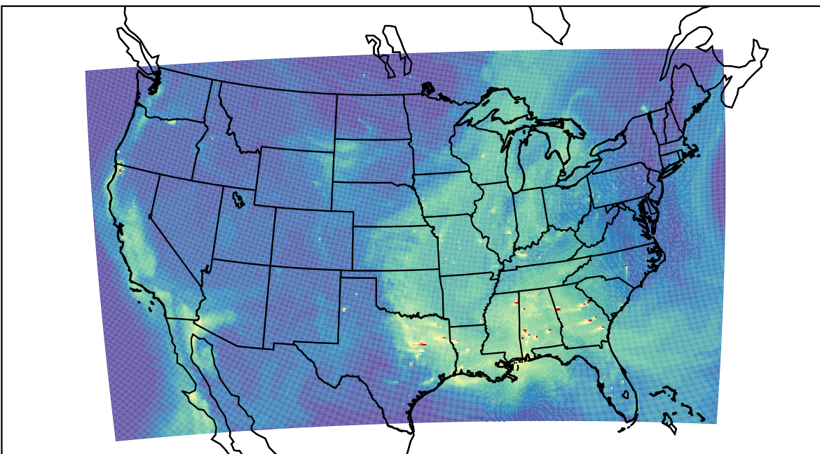
WRF 2023-09-15_20:00:00
