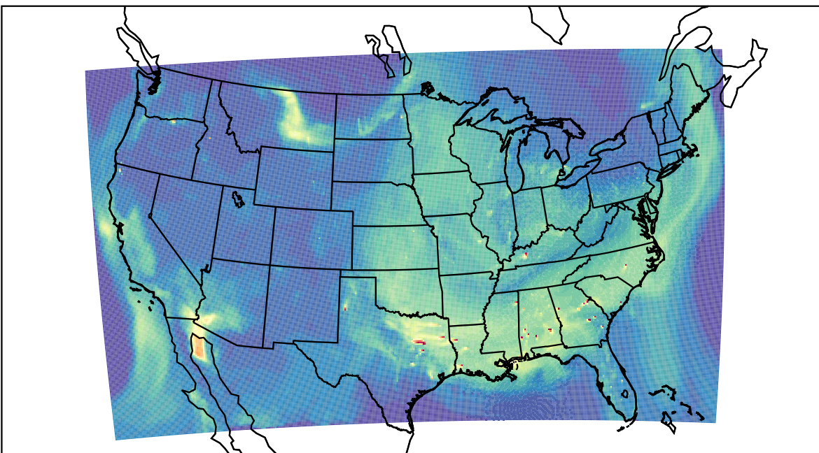
WRF 2023-09-14_19:00:00
