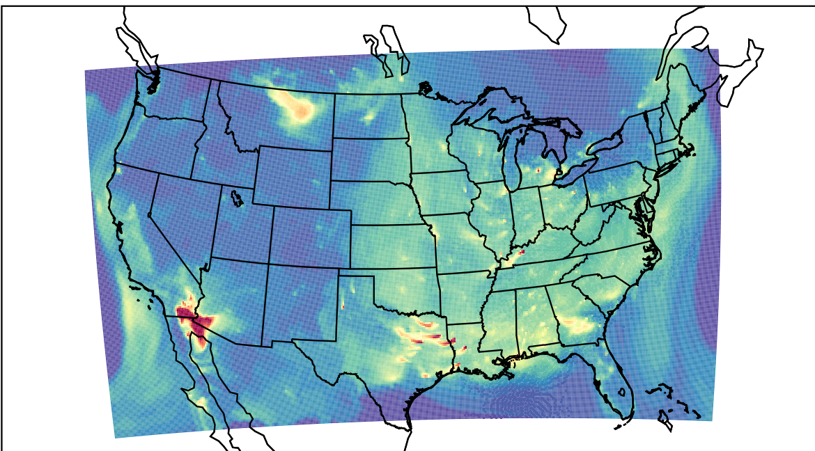
WRF 2023-09-14_13:00:00
