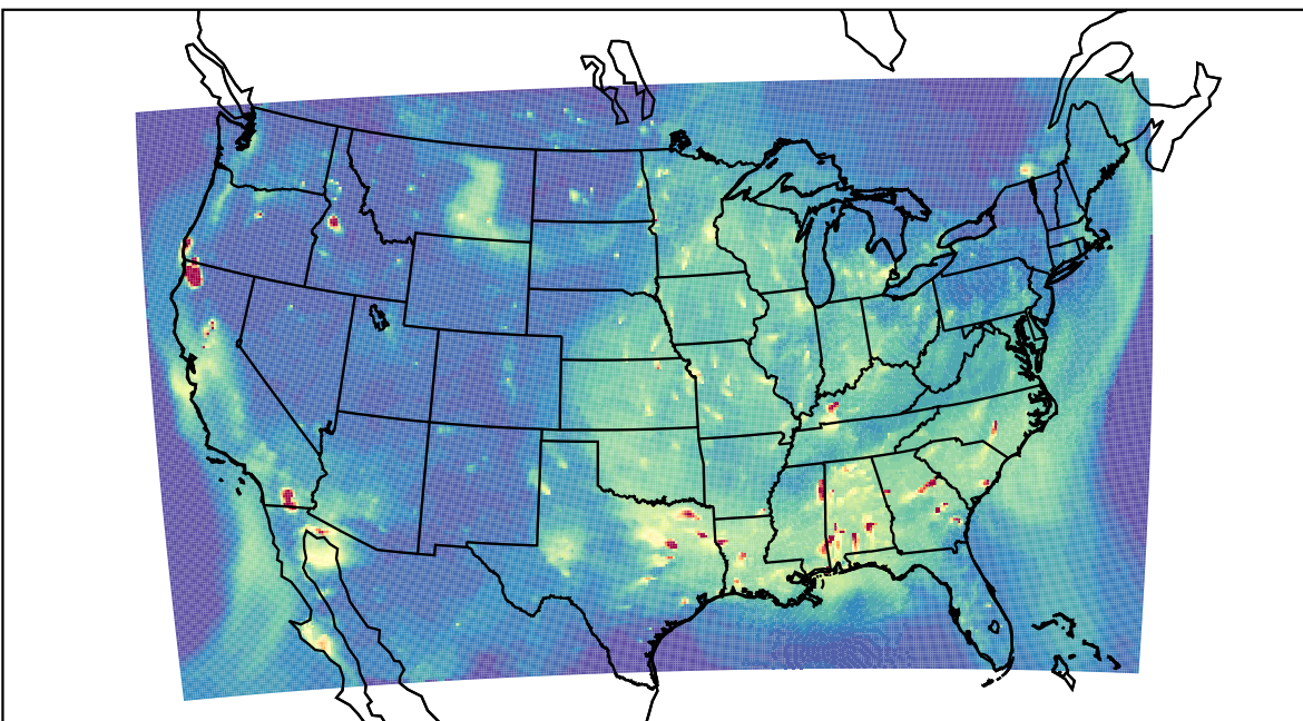
WRF 2023-09-15_02:00:00
