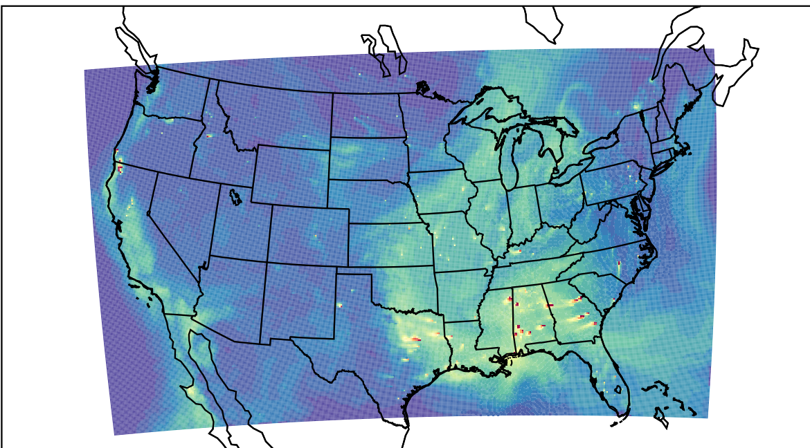
WRF 2023-09-15_22:00:00
