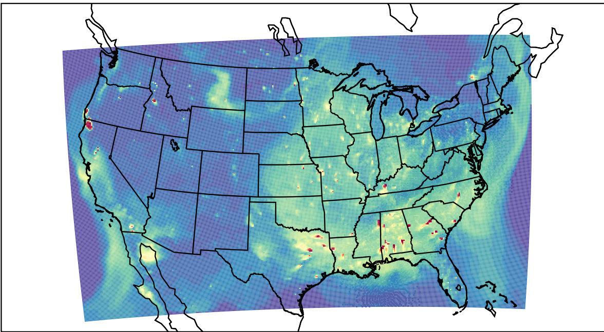
WRF 2023-09-15_01:00:00
