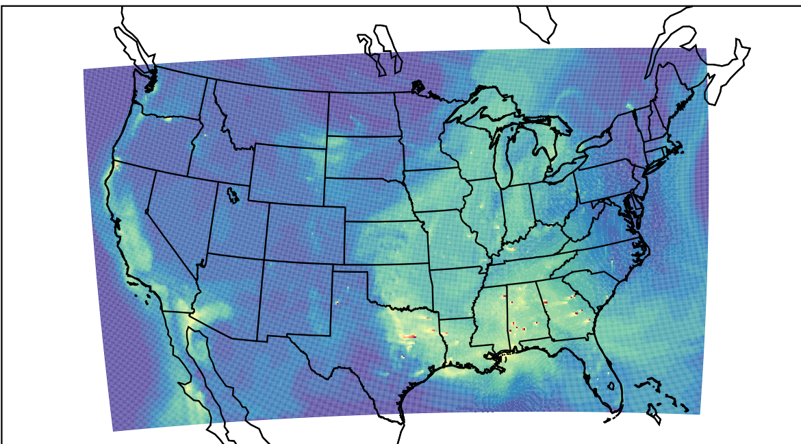
WRF 2023-09-15_19:00:00
