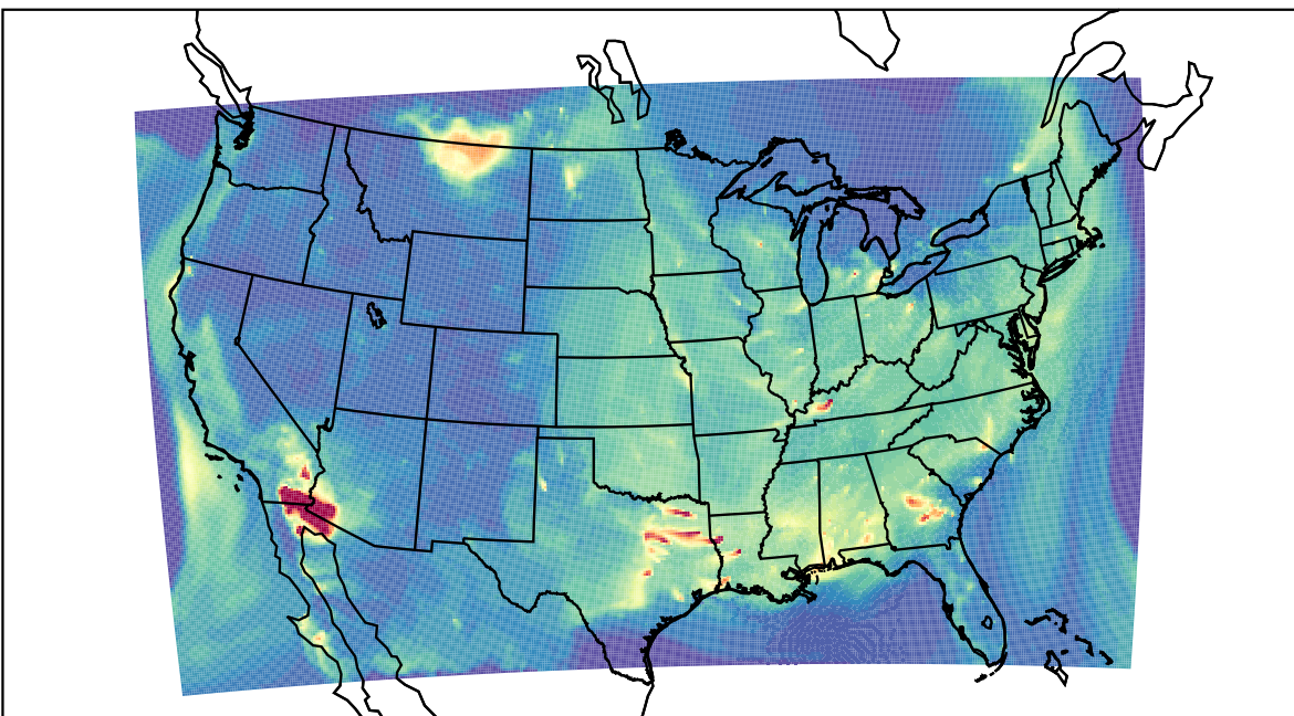
WRF 2023-09-14_09:00:00
