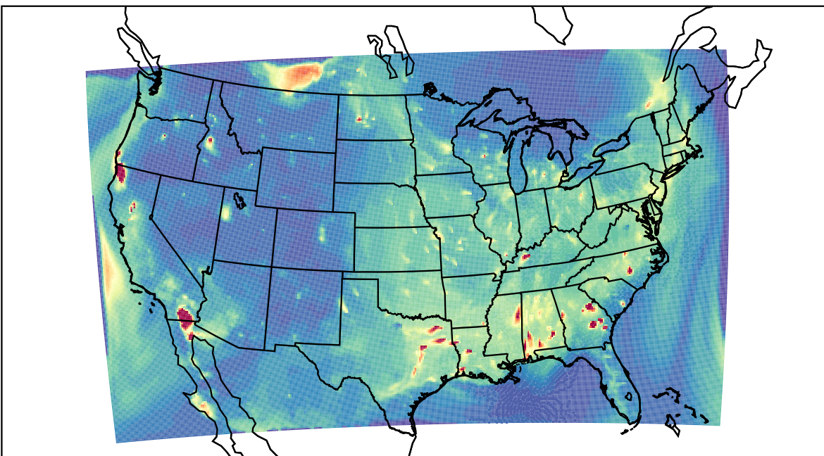
WRF 2023-09-14_03:00:00
