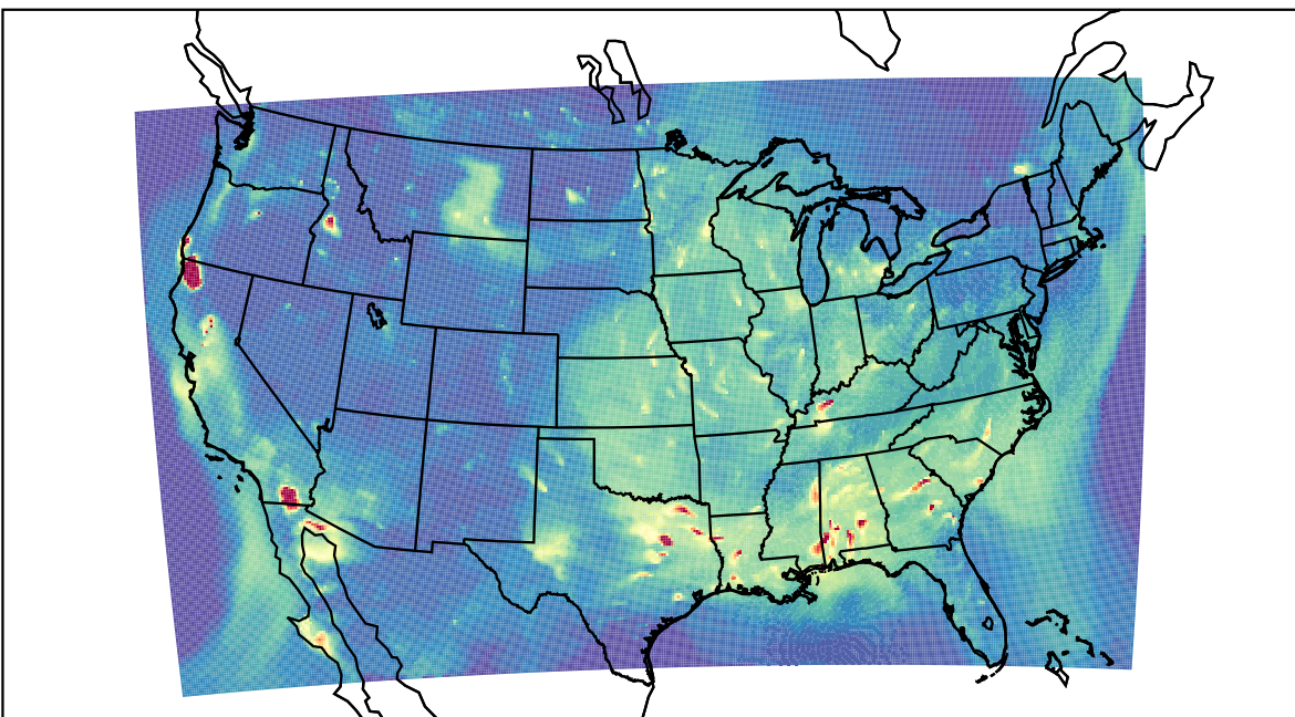
WRF 2023-09-15_03:00:00
