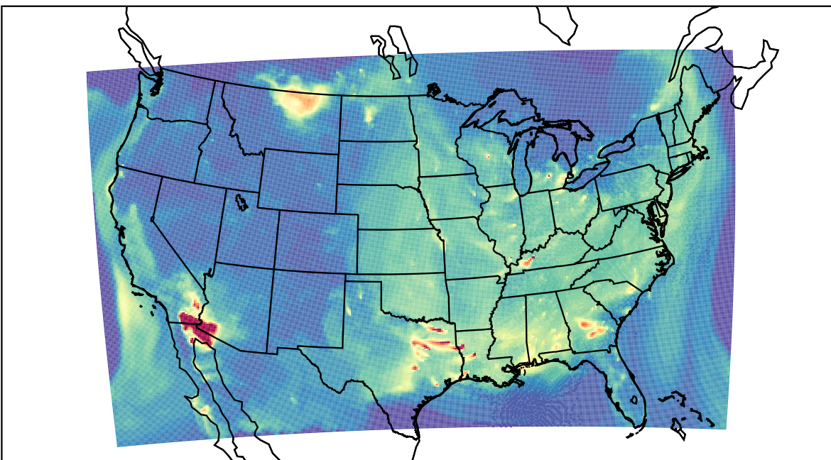
WRF 2023-09-14_10:00:00
