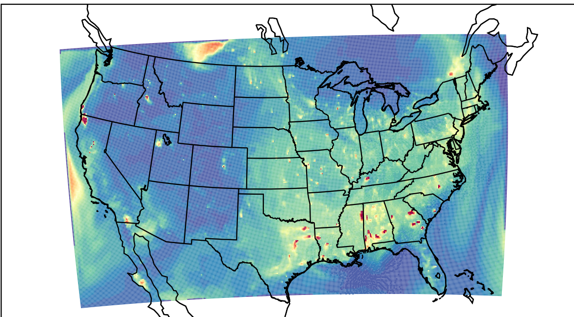
WRF 2023-09-14_01:00:00
