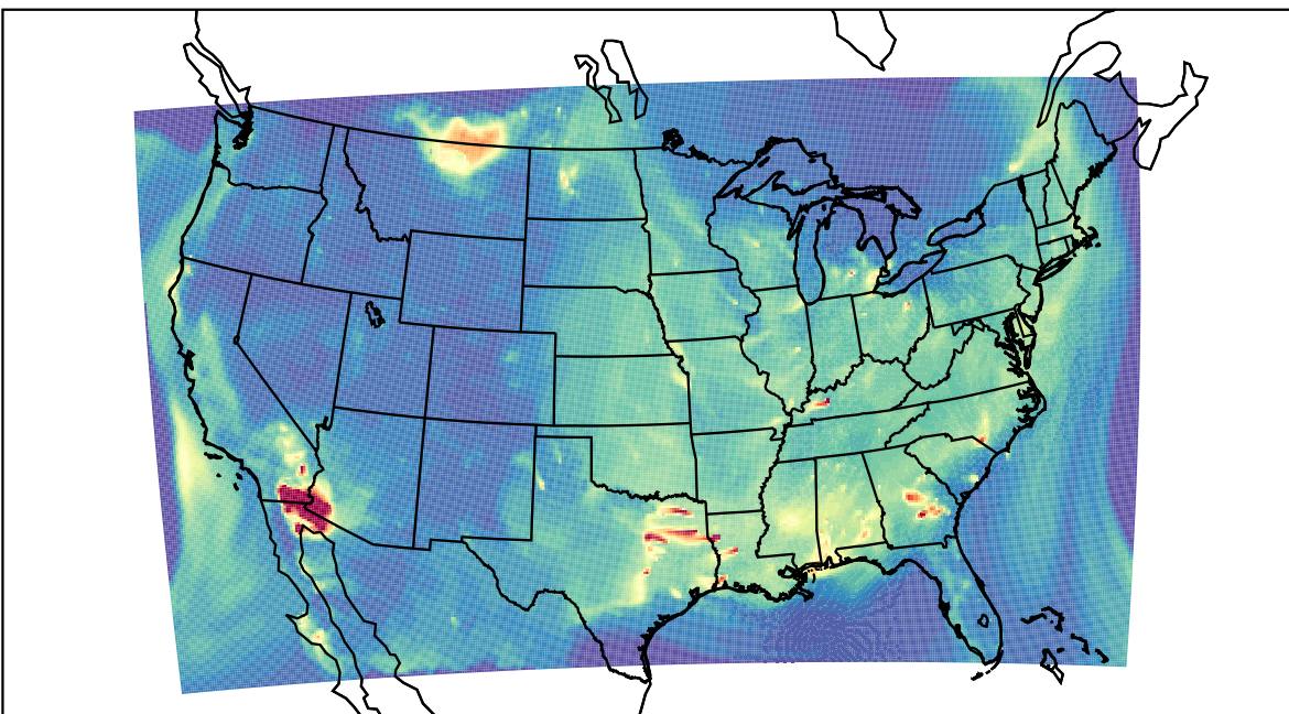
WRF 2023-09-14_08:00:00
