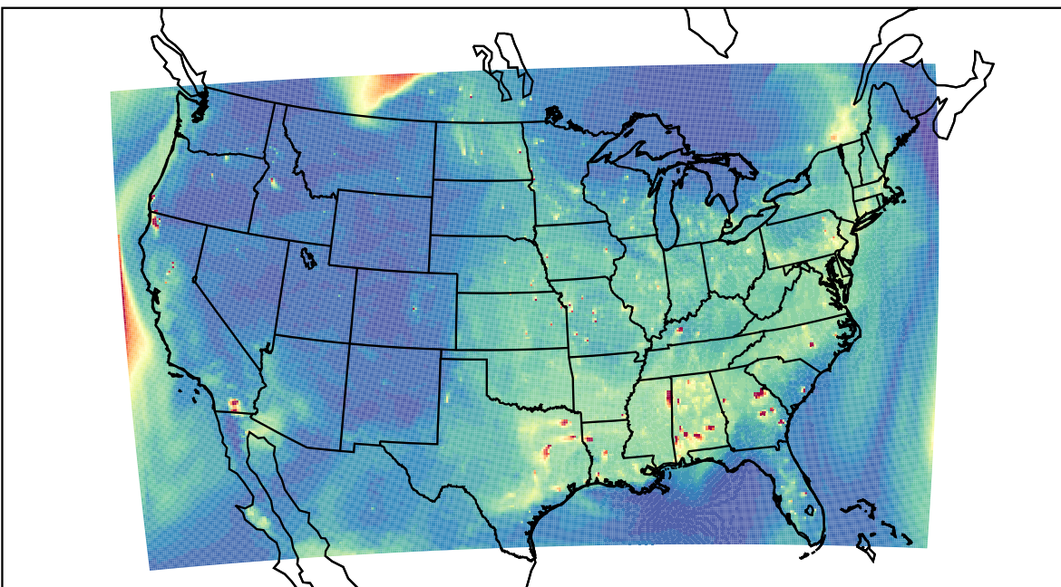
WRF 2023-09-14_00:00:00
