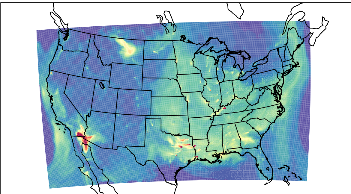
WRF 2023-09-14_15:00:00
