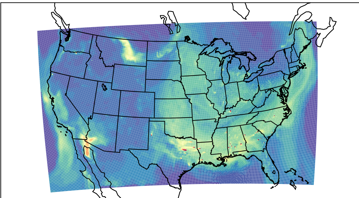
WRF 2023-09-14_18:00:00
