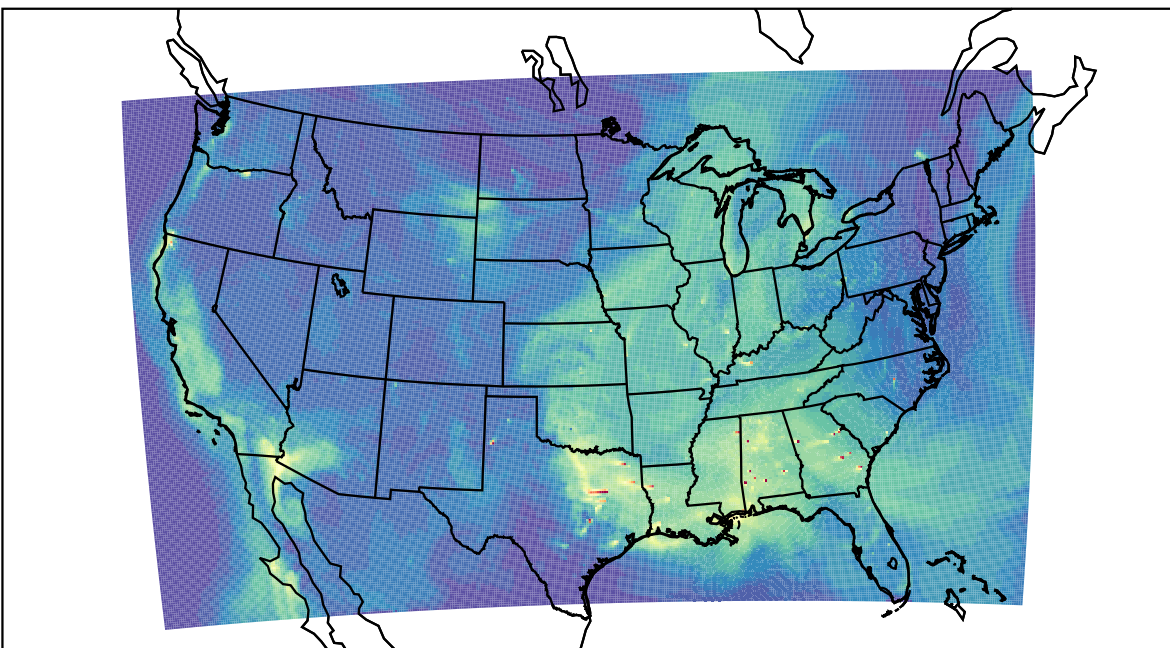
WRF 2023-09-15_18:00:00
