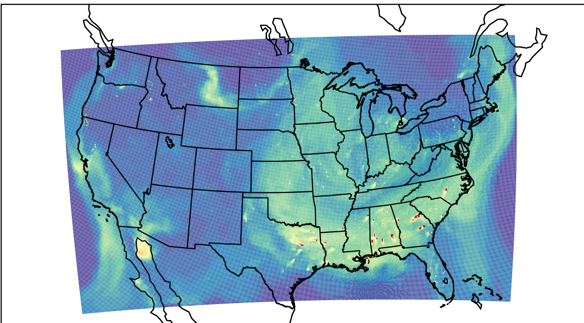
WRF 2023-09-14_22:00:00
