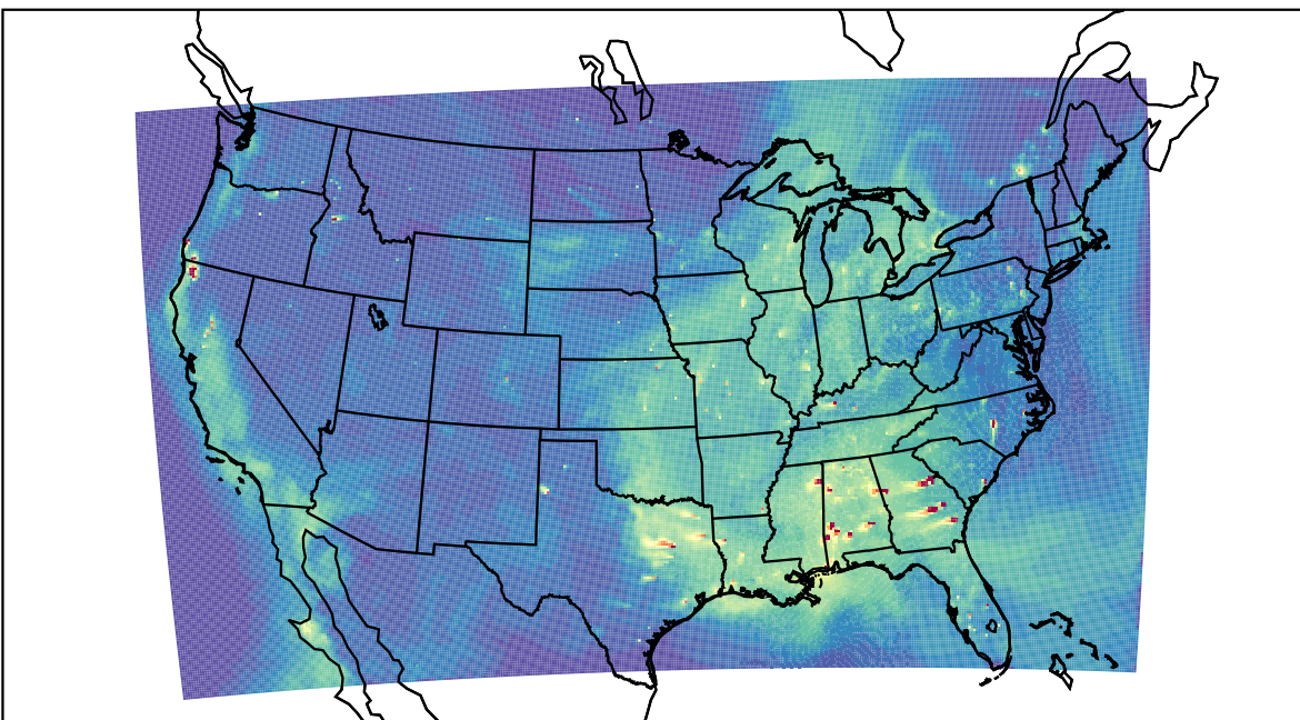
WRF 2023-09-15_23:00:00
