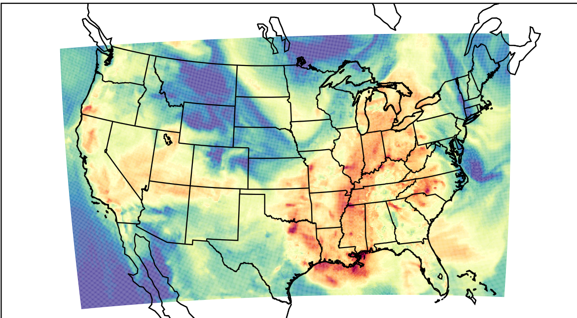
WRF (2023-09-16_20:00:00)
