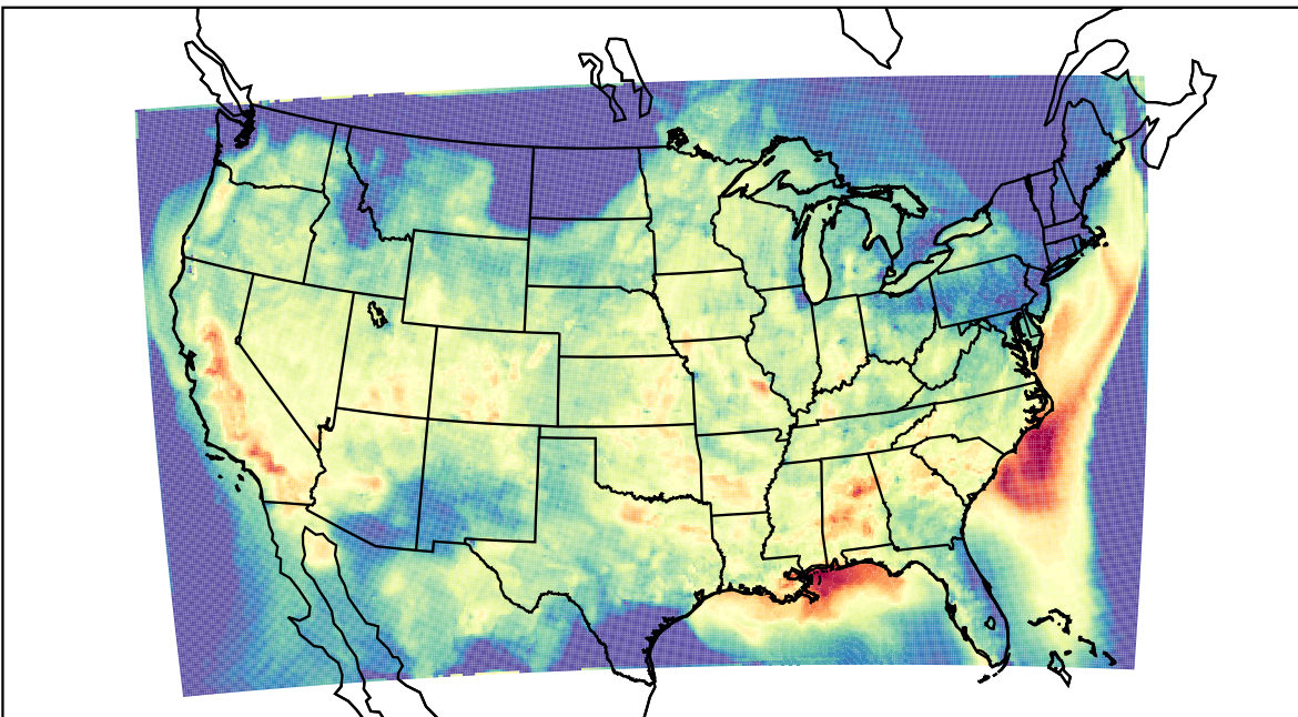
WRF (2023-09-15_01:00:00)
