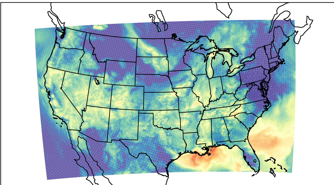
WRF (2023-09-16_10:00:00)
