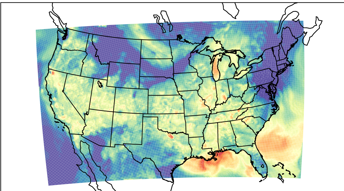
WRF (2023-09-16_04:00:00)
