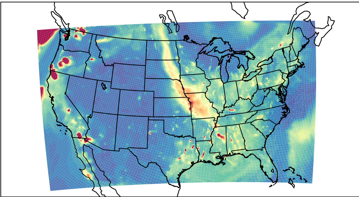
WRF 2023-09-18_03:00:00
