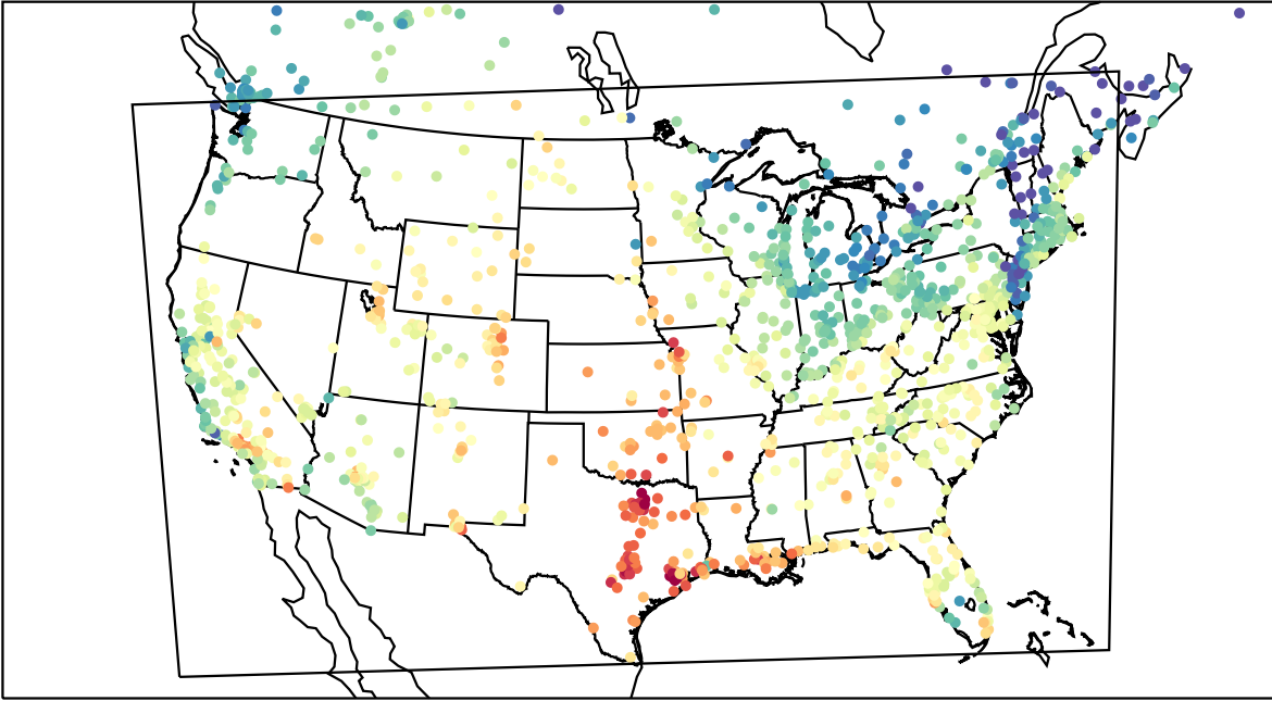
AirNOW (2023-09-18_20:00:00)
