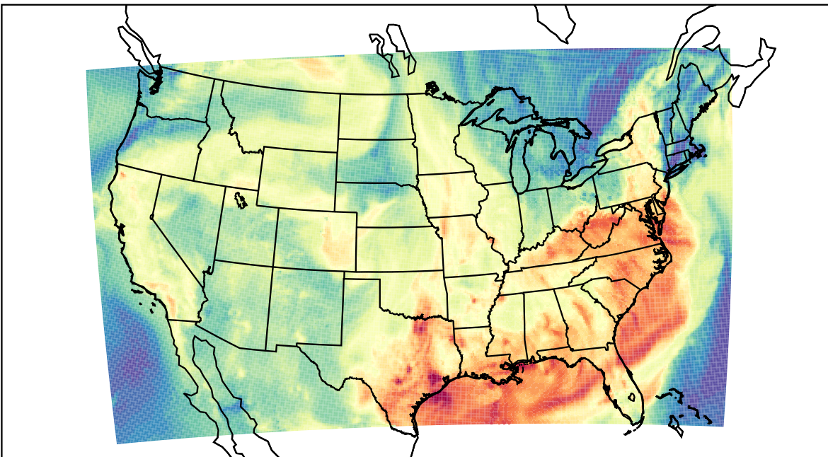
WRF (2023-09-18_20:00:00)
