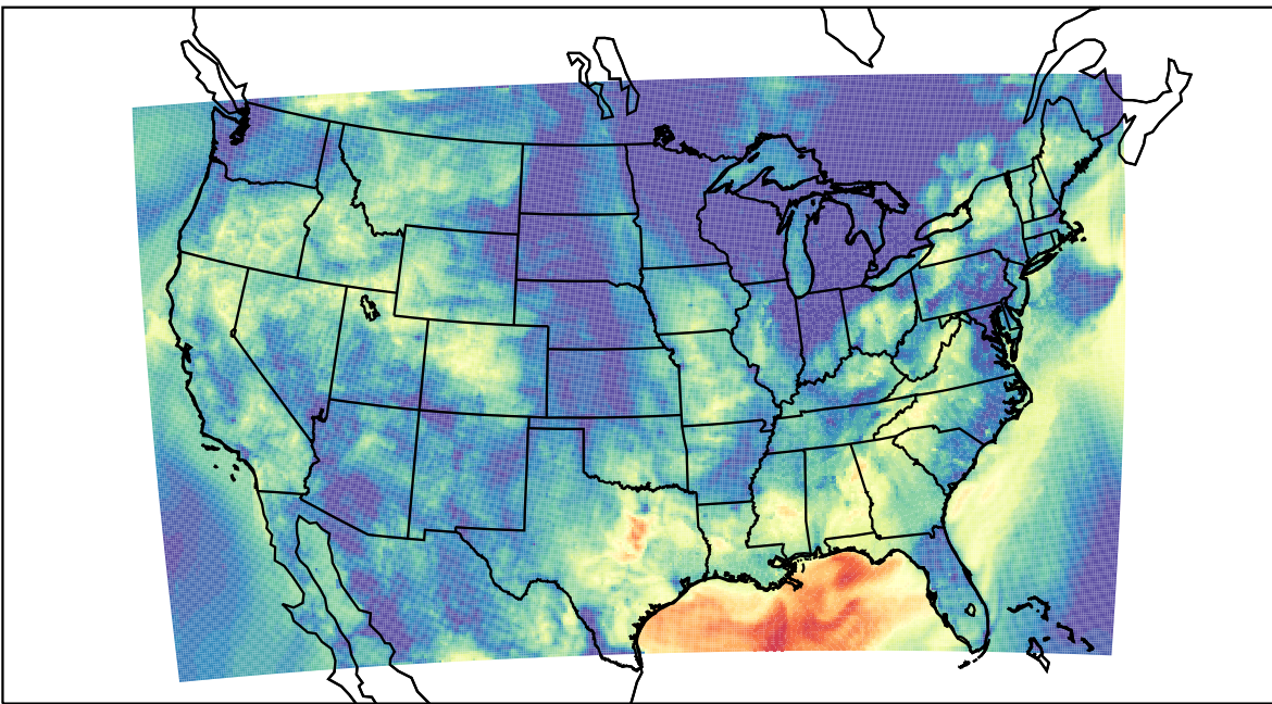
WRF (2023-09-18_11:00:00)
