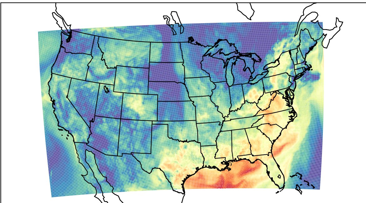
WRF (2023-09-18_15:00:00)
