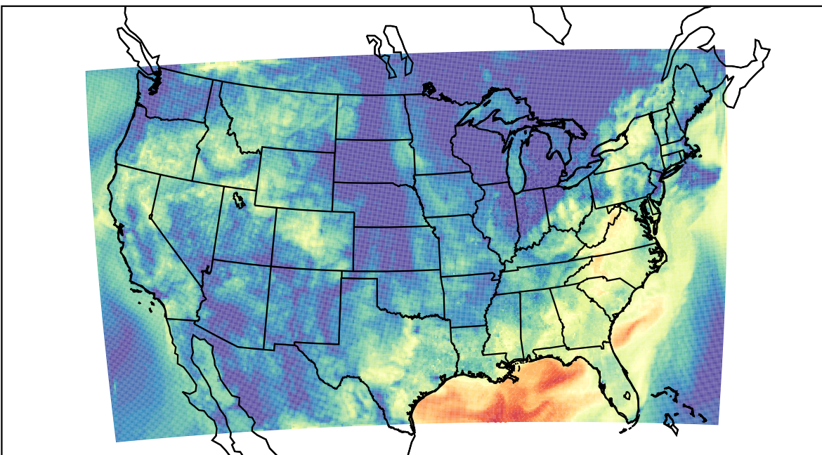
WRF (2023-09-18_14:00:00)
