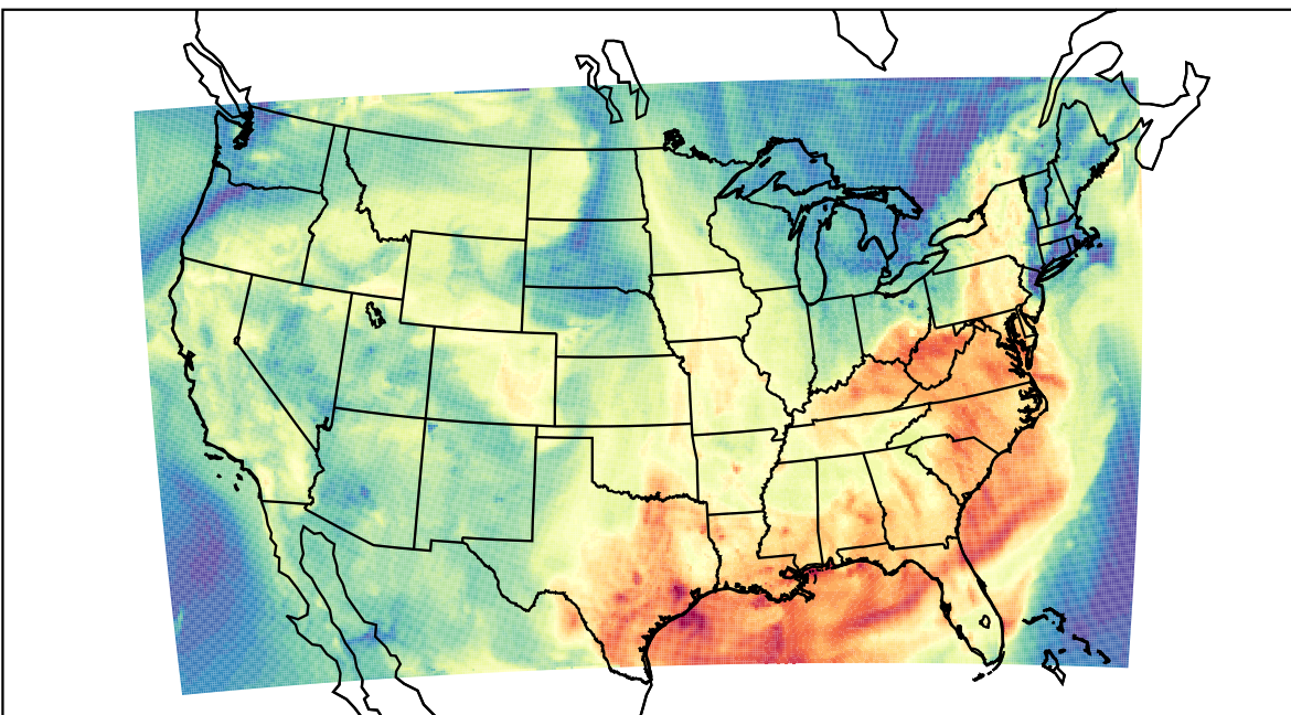
WRF (2023-09-18_18:00:00)
