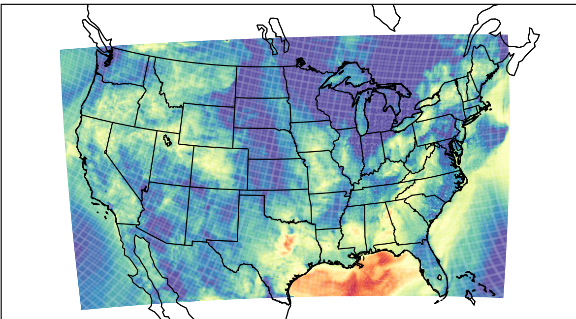
WRF (2023-09-18_10:00:00)
