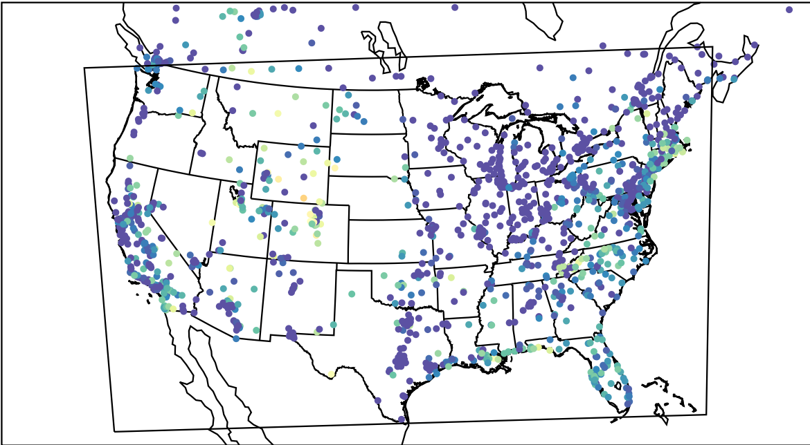
AirNOW (2023-09-18_13:00:00)
