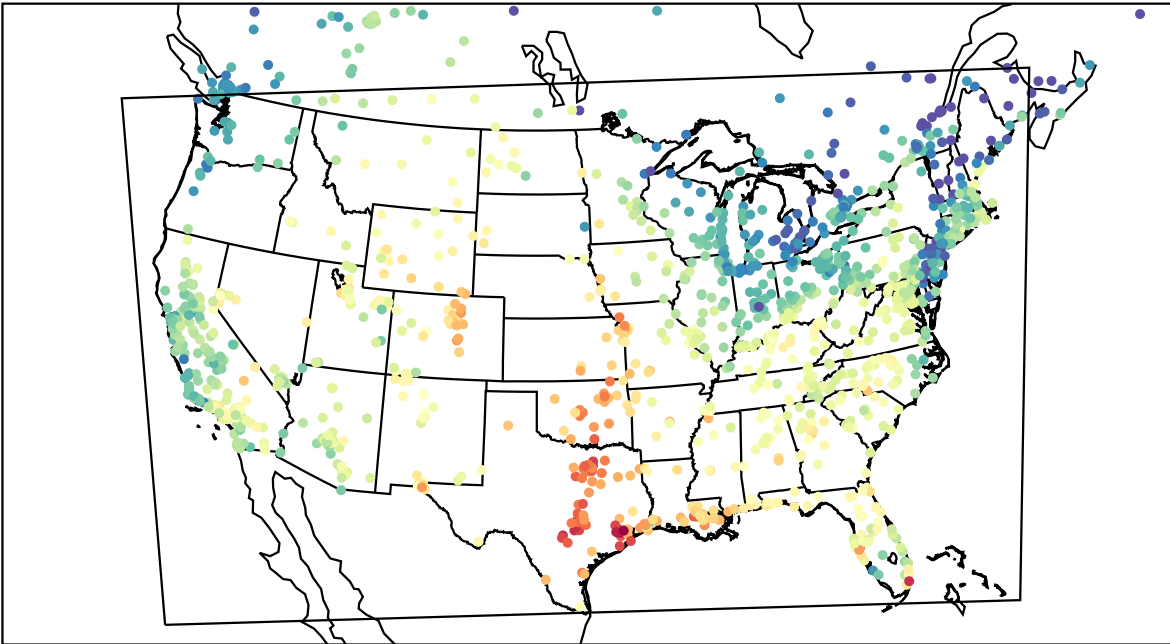
AirNOW (2023-09-18_18:00:00)
