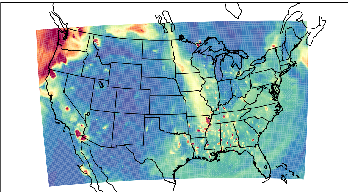
WRF 2023-09-19_03:00:00
