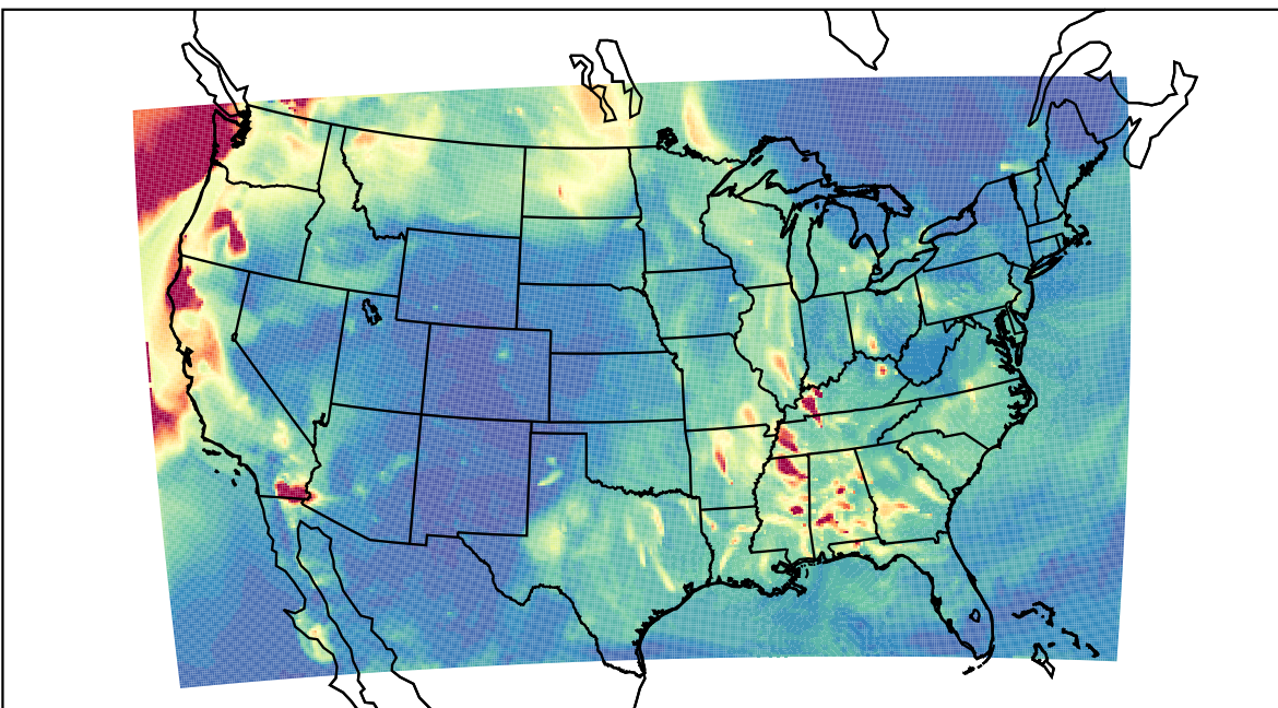
WRF 2023-09-20_06:00:00
