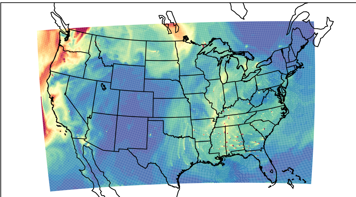
WRF 2023-09-20_20:00:00
