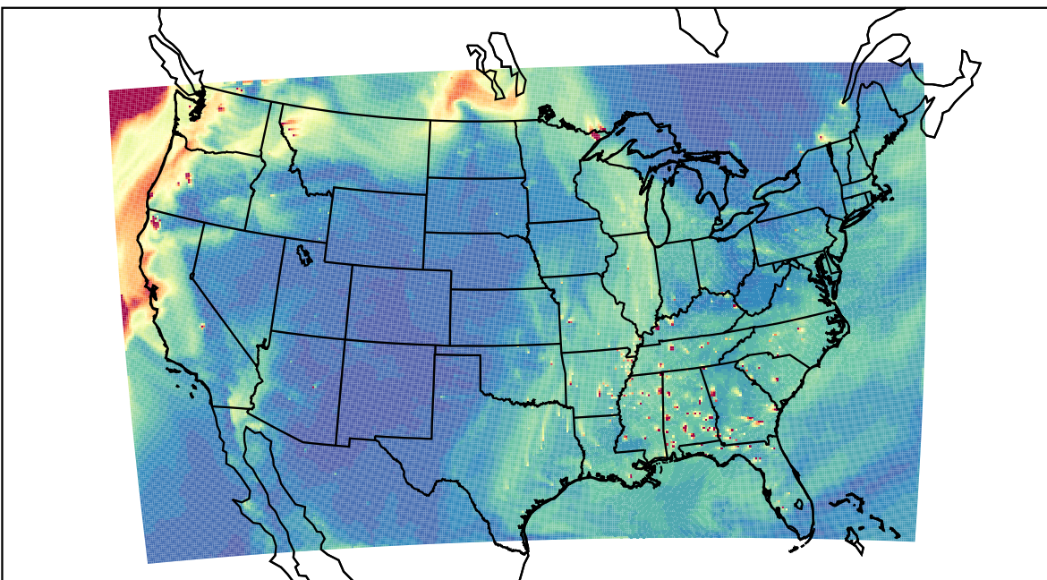
WRF 2023-09-19_22:00:00
