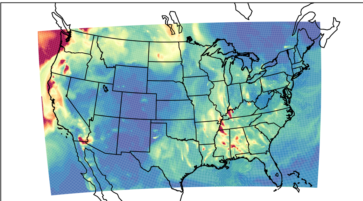
WRF 2023-09-20_08:00:00
