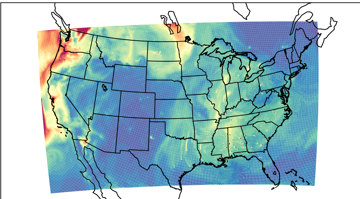
WRF 2023-09-20_18:00:00
