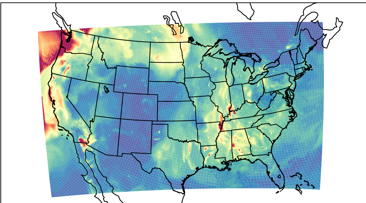
WRF 2023-09-20_11:00:00
