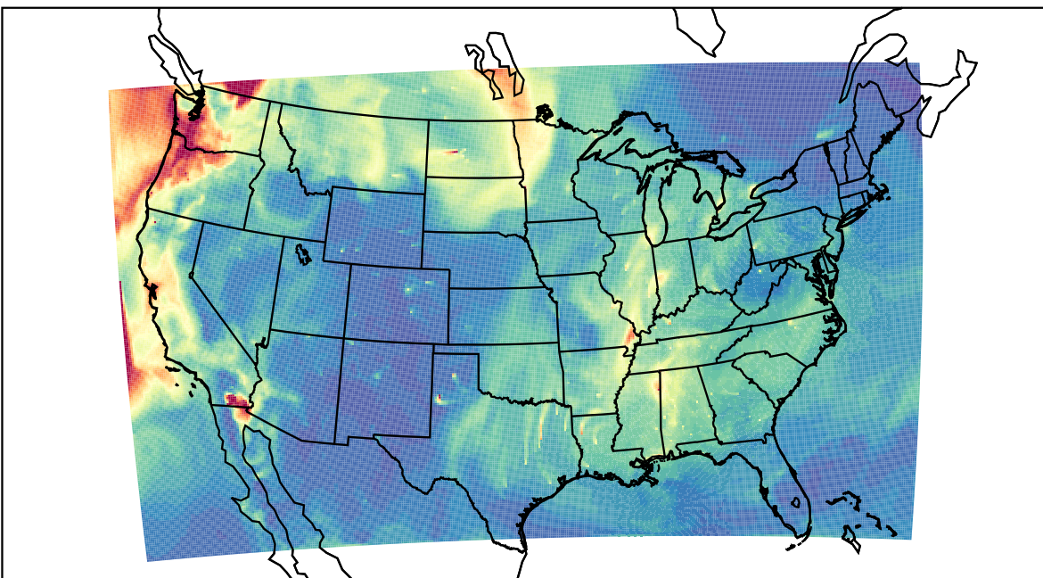
WRF 2023-09-20_16:00:00
