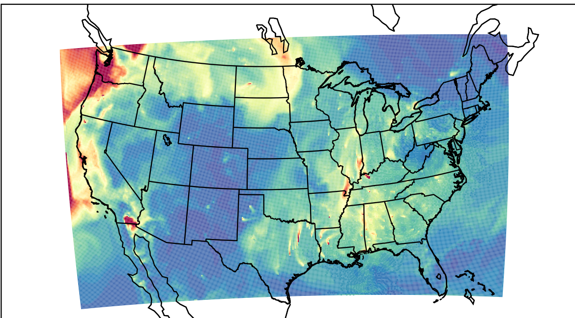
WRF 2023-09-20_14:00:00
