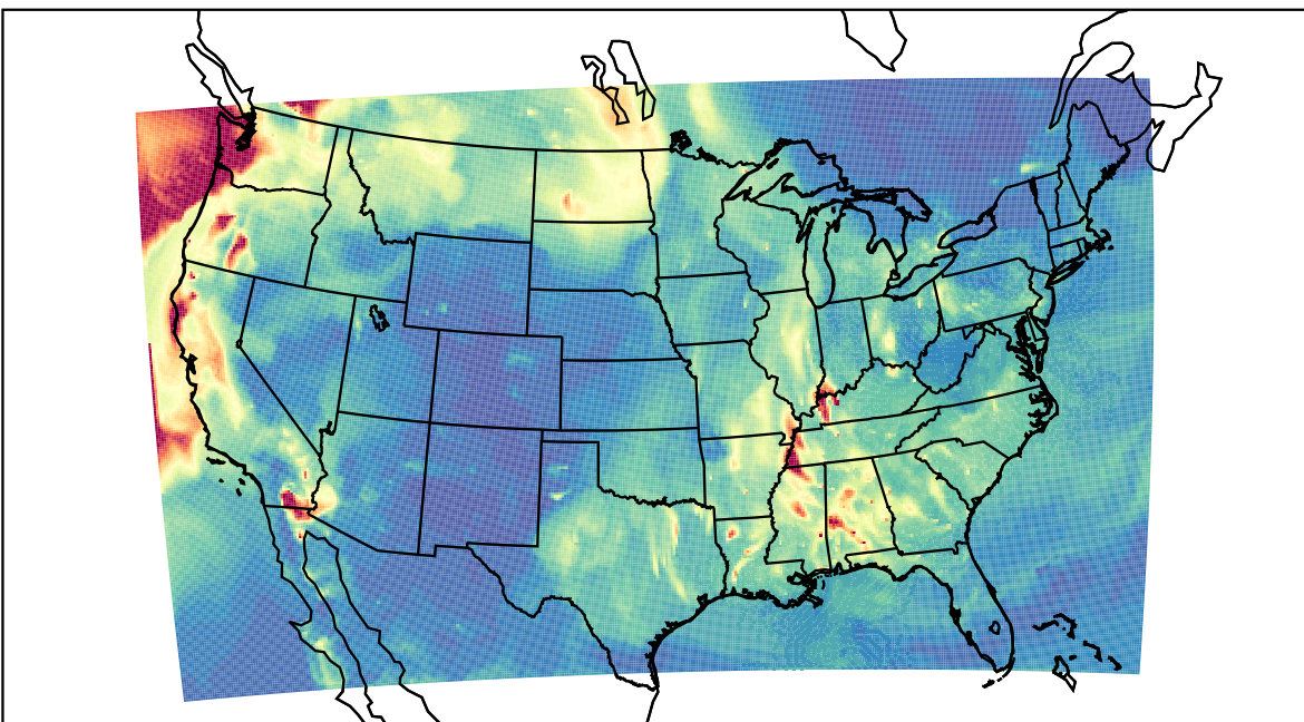
WRF 2023-09-20_09:00:00
