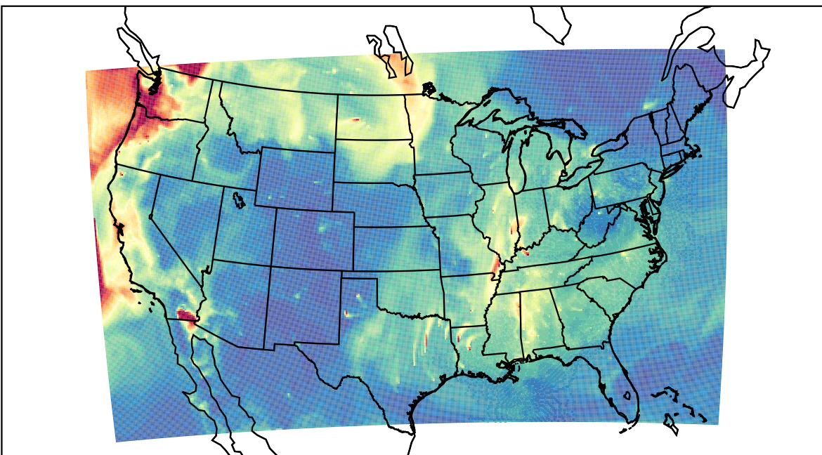
WRF 2023-09-20_15:00:00
