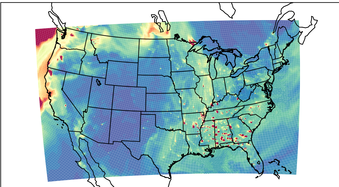
WRF 2023-09-20_00:00:00
