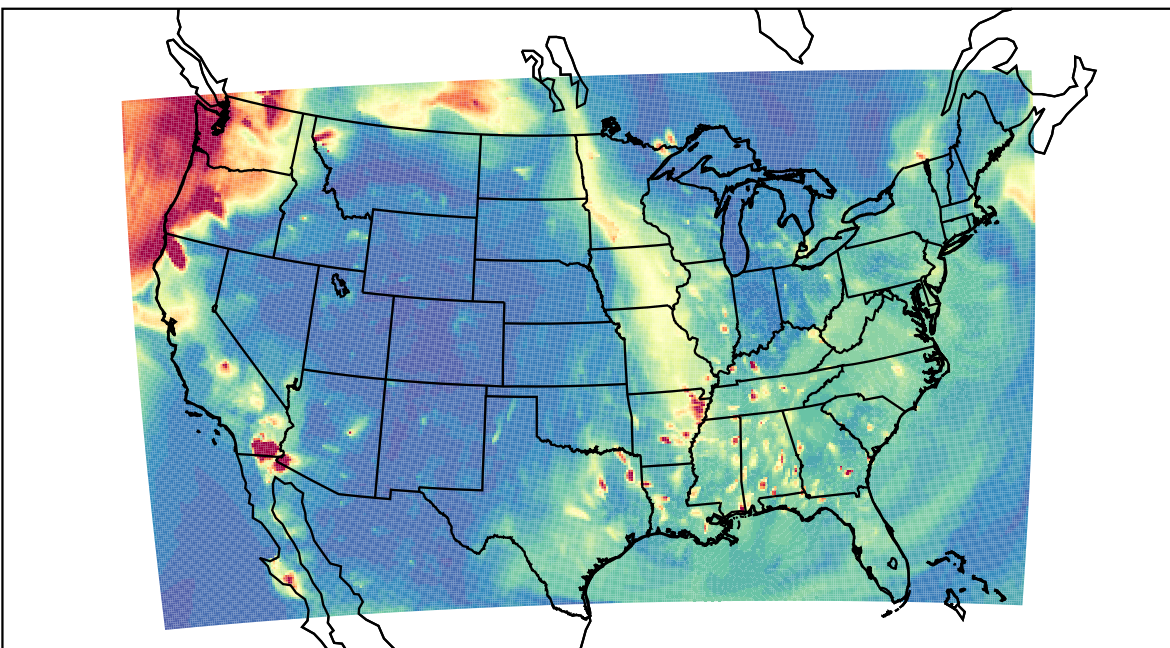
WRF 2023-09-19_04:00:00
