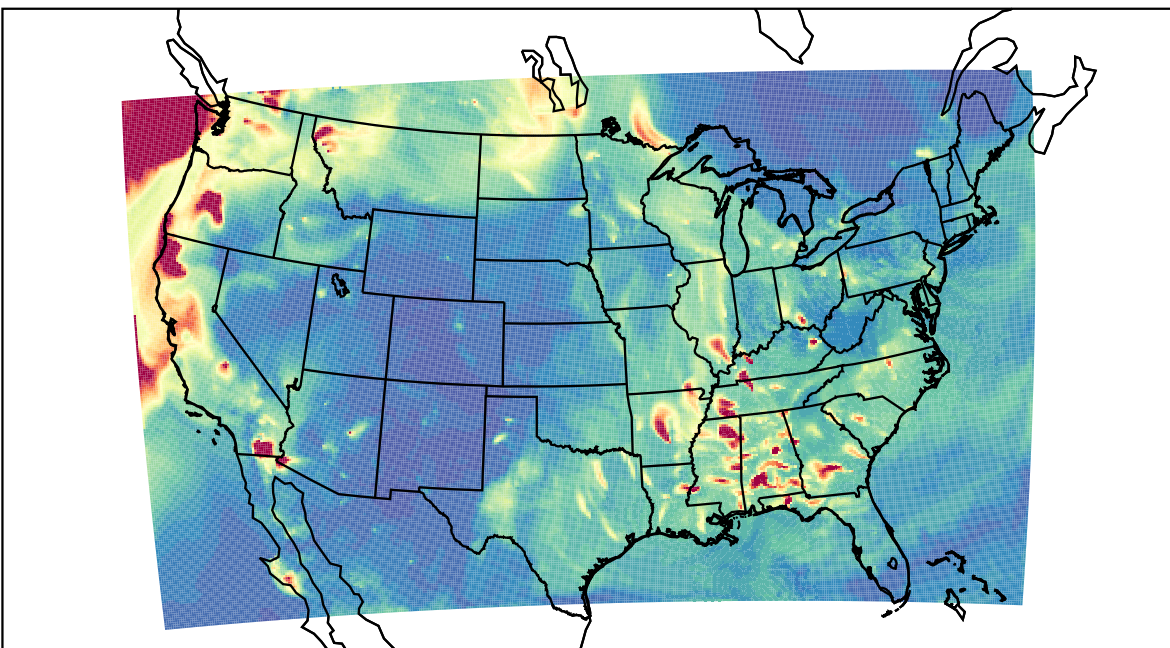
WRF 2023-09-20_04:00:00
