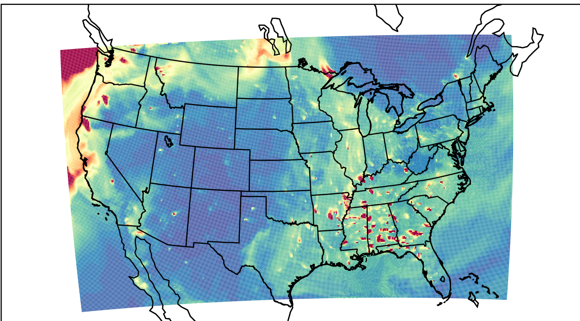
WRF 2023-09-20_01:00:00
