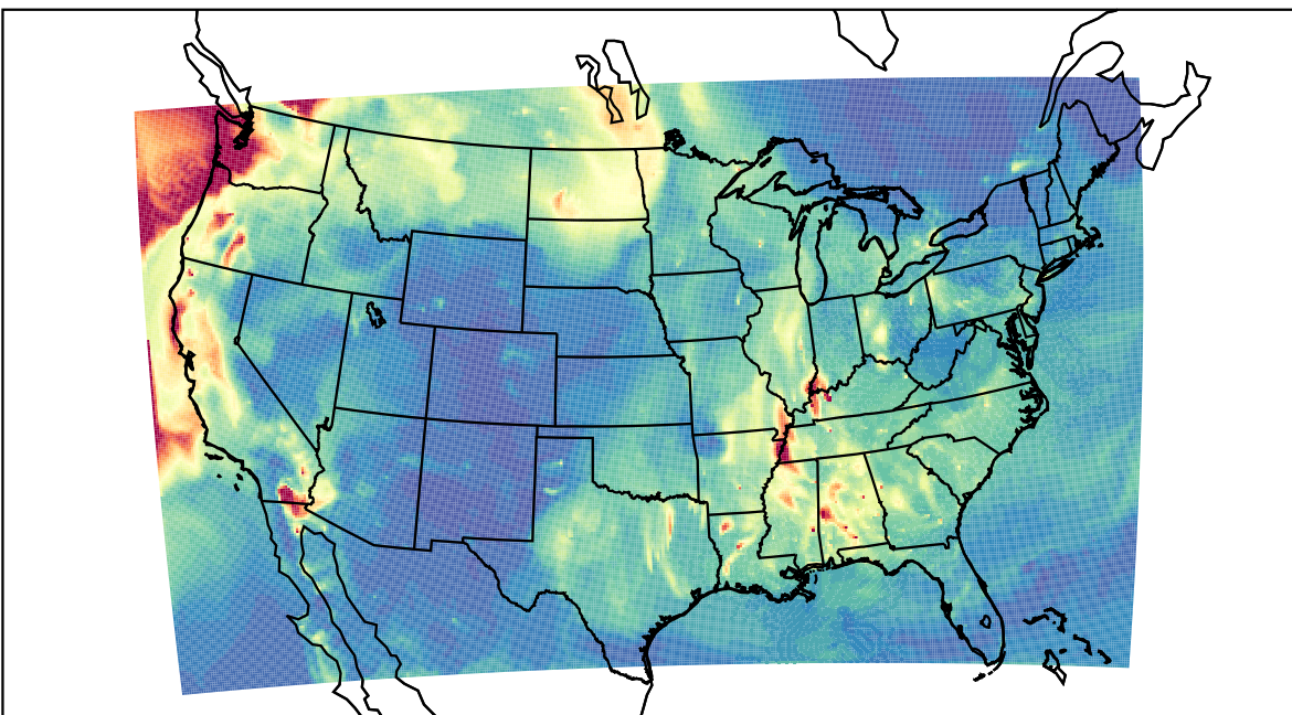
WRF 2023-09-20_10:00:00
