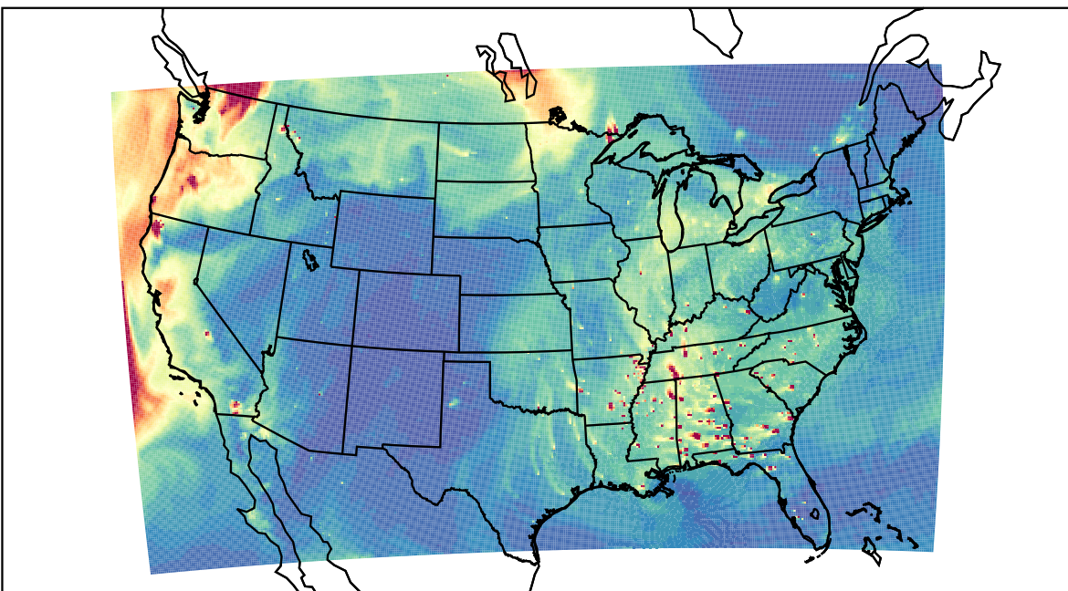
WRF 2023-09-20_23:00:00
