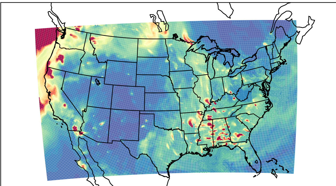
WRF 2023-09-20_03:00:00
