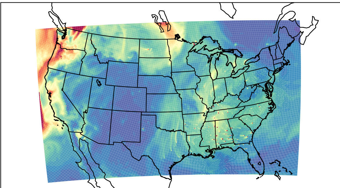
WRF 2023-09-20_19:00:00
