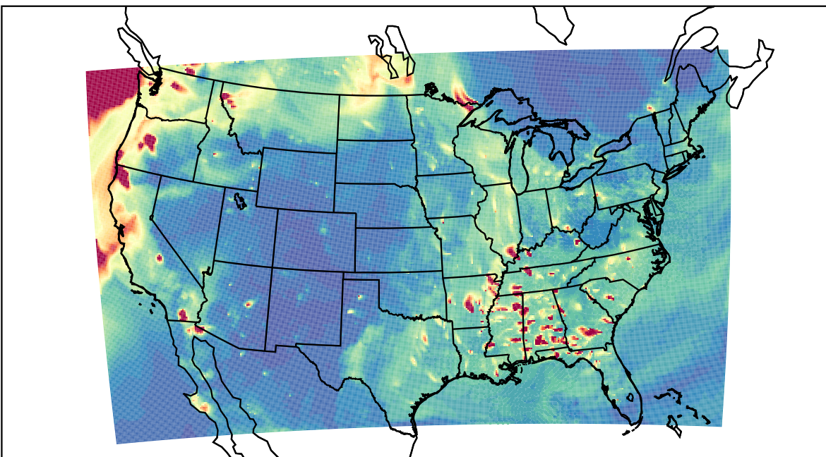
WRF 2023-09-20_02:00:00
