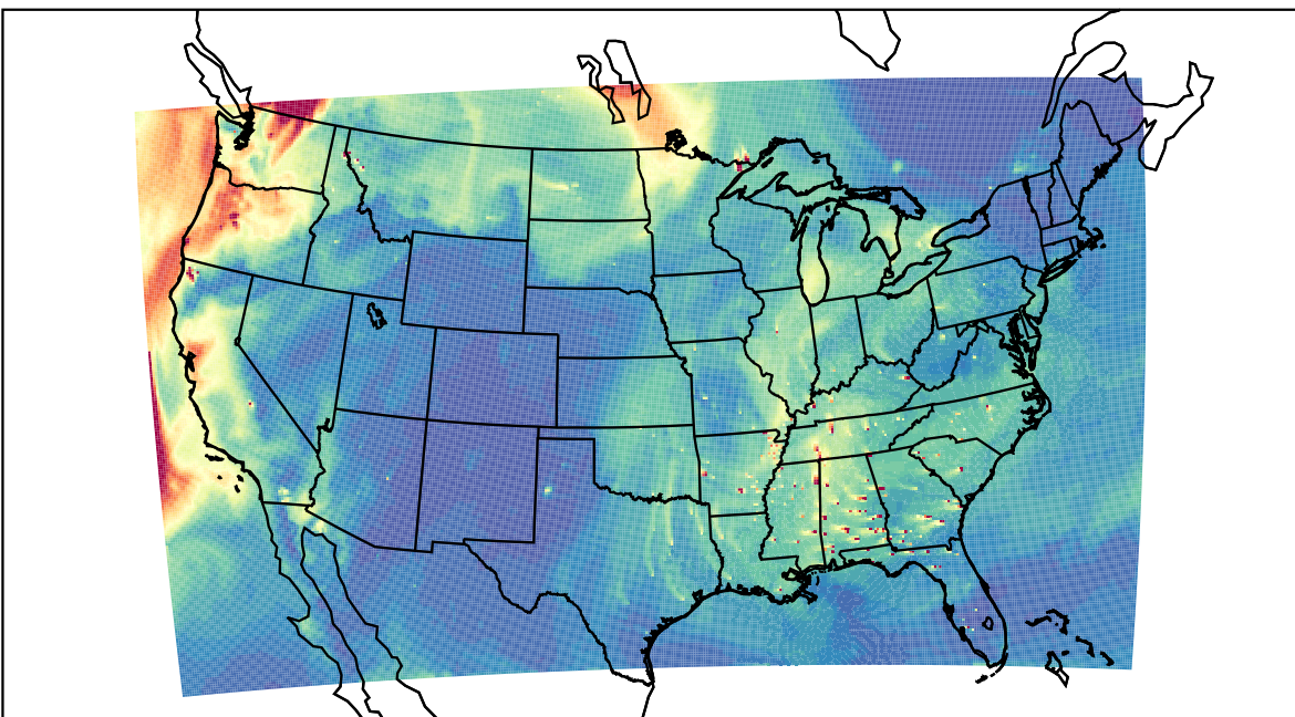
WRF 2023-09-20_21:00:00
