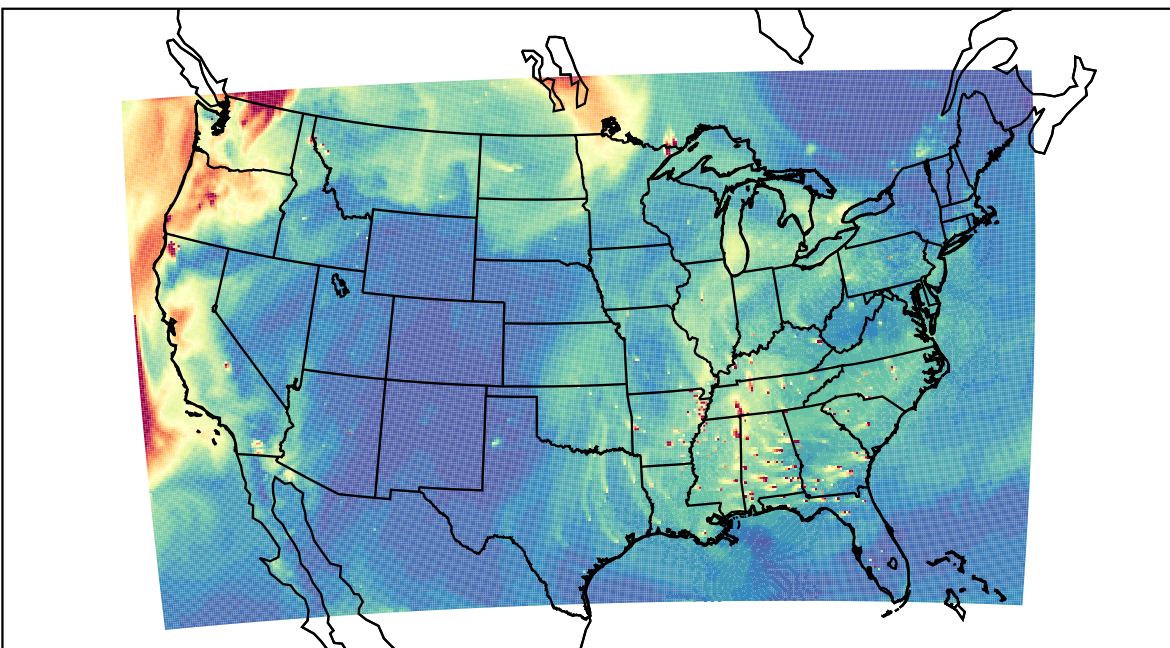
WRF 2023-09-20_22:00:00
