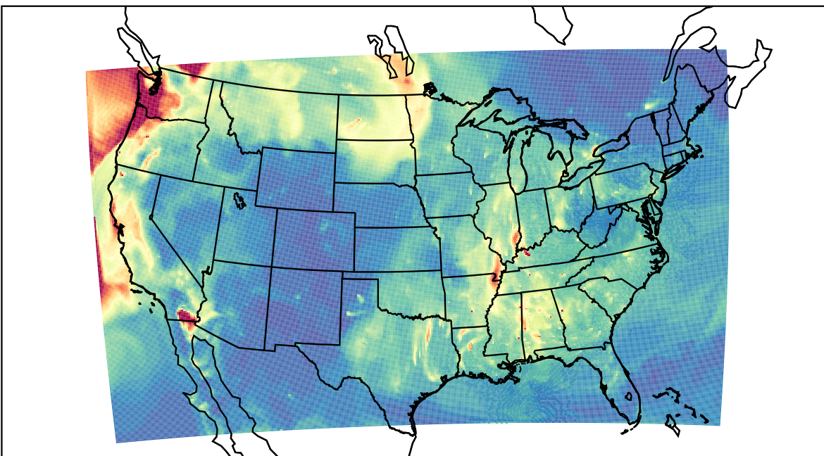
WRF 2023-09-20_13:00:00
