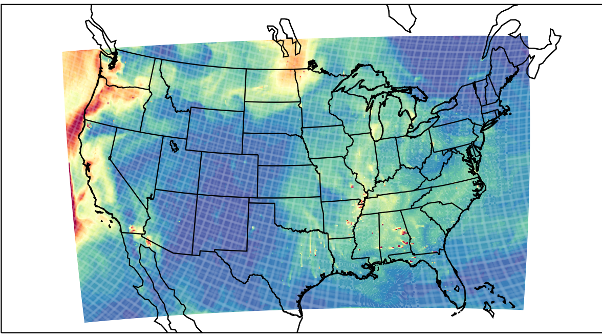
WRF 2023-09-20_20:00:00
