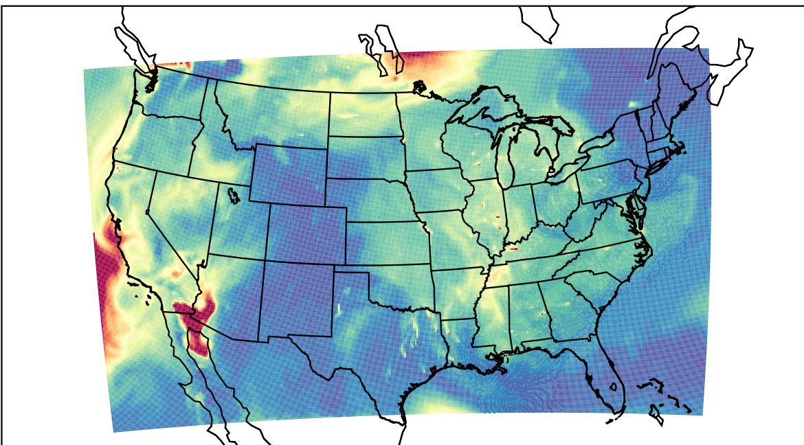
WRF 2023-09-21_16:00:00
