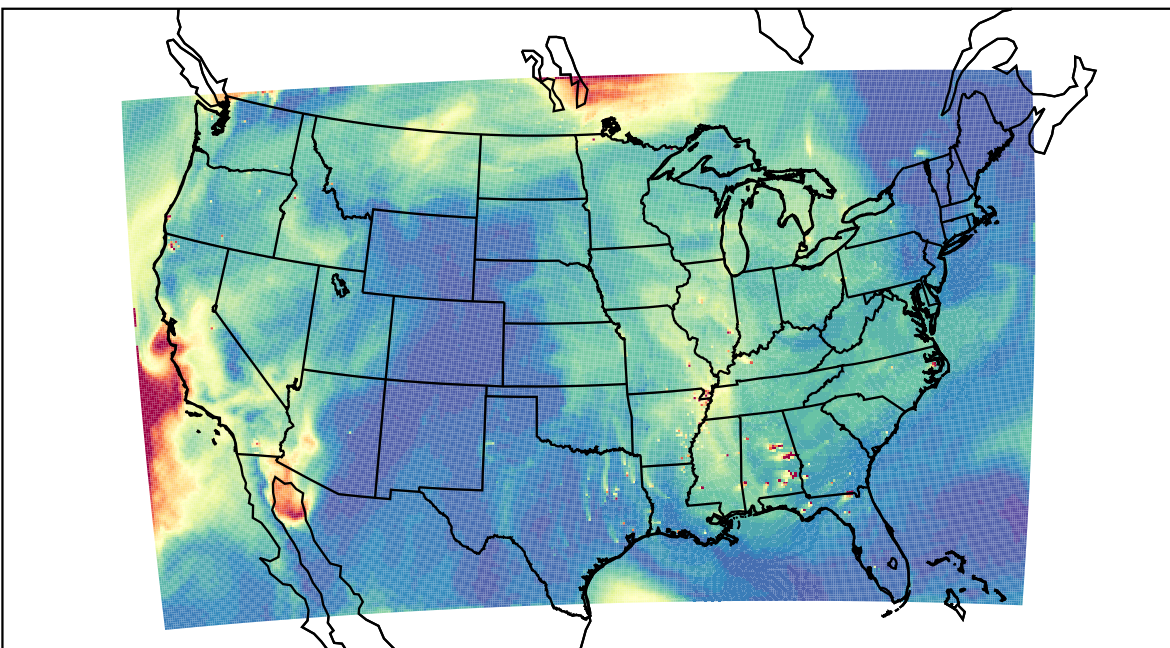
WRF 2023-09-21_20:00:00
