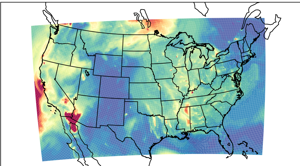
WRF 2023-09-21_12:00:00
