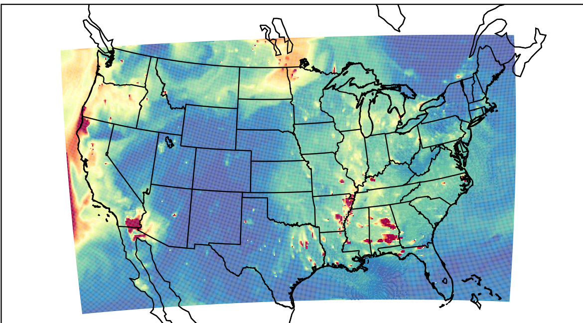
WRF 2023-09-21_01:00:00
