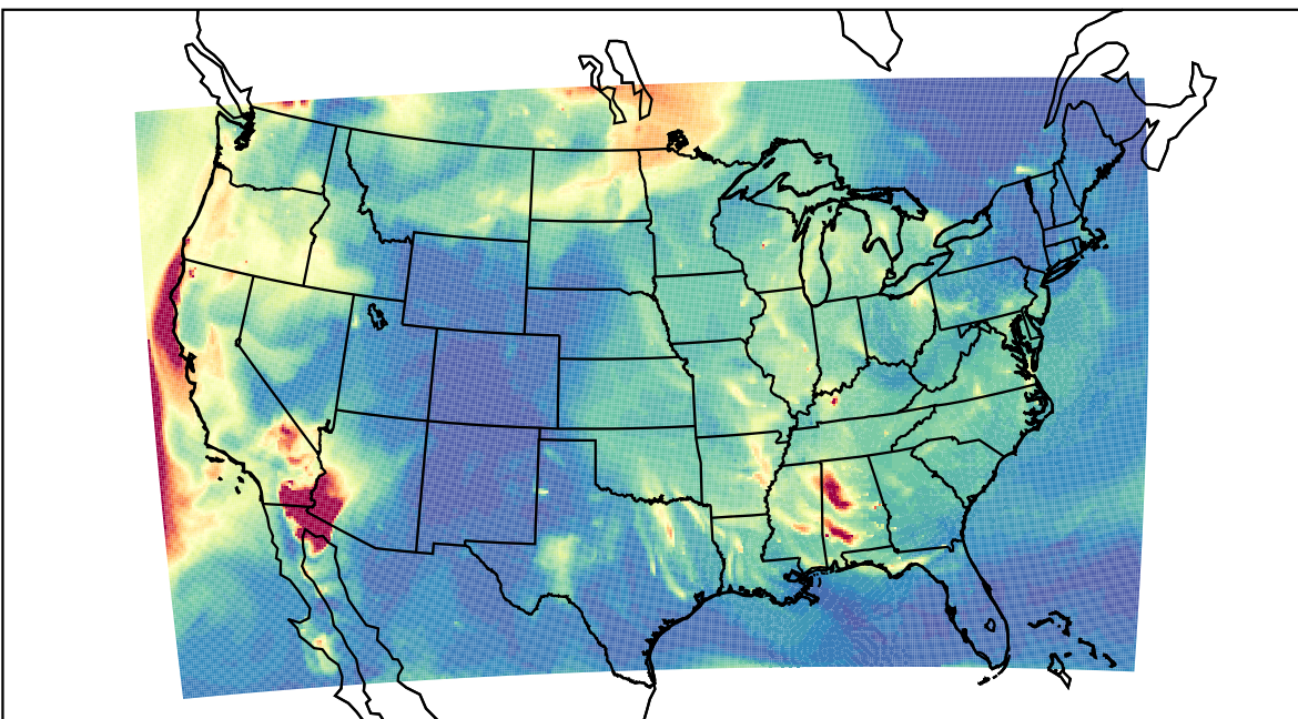
WRF 2023-09-21_07:00:00
