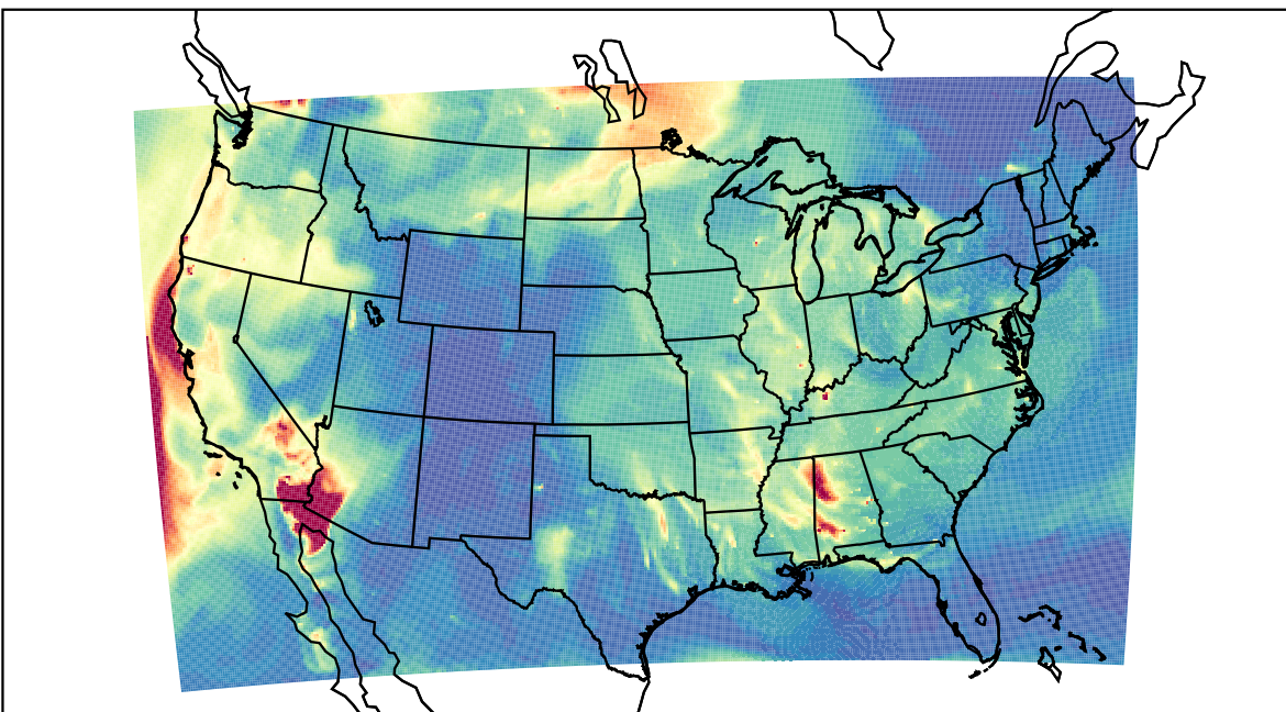
WRF 2023-09-21_08:00:00
