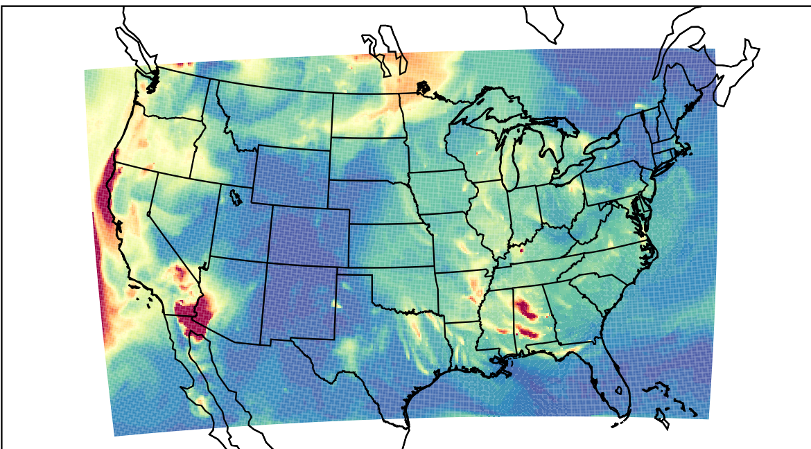
WRF 2023-09-21_06:00:00
