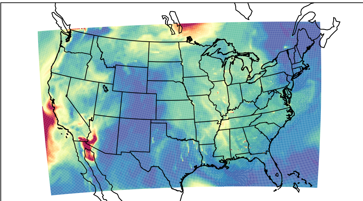
WRF 2023-09-21_17:00:00
