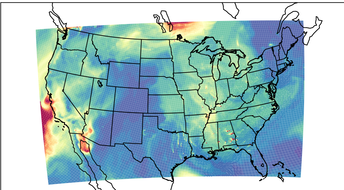
WRF 2023-09-21_19:00:00
