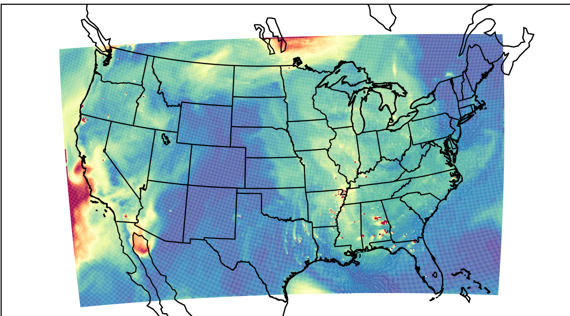
WRF 2023-09-21_21:00:00
