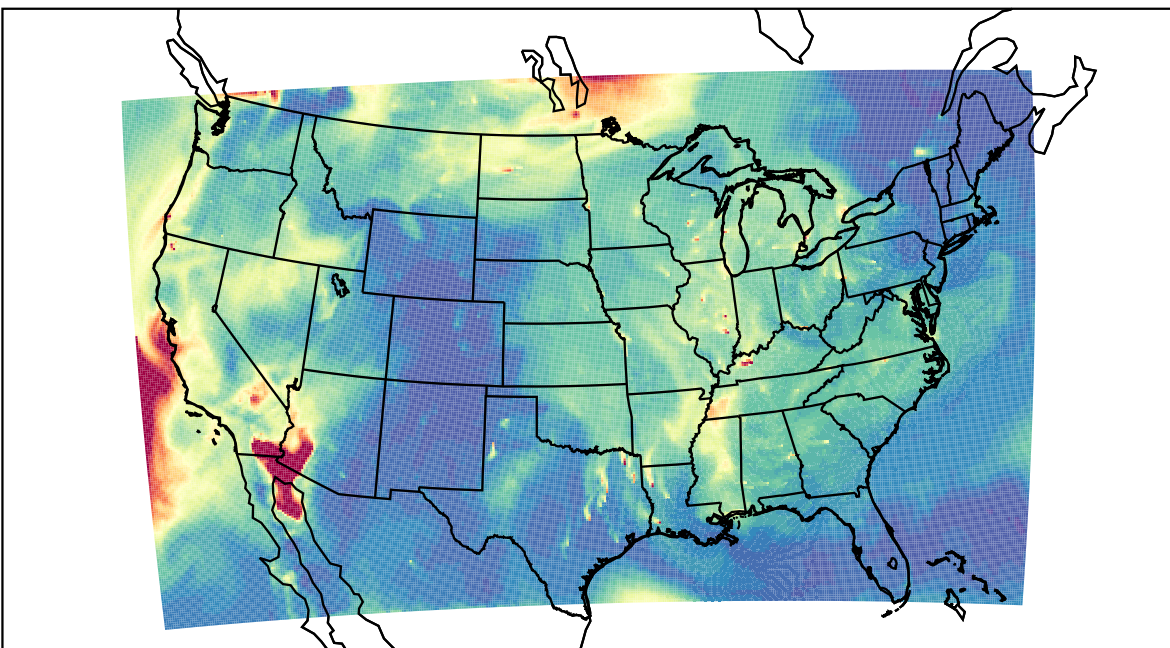
WRF 2023-09-21_15:00:00
