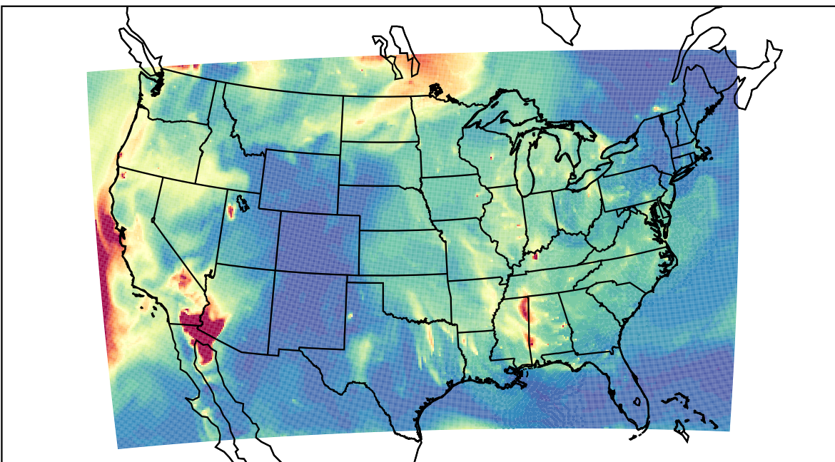
WRF 2023-09-21_10:00:00
