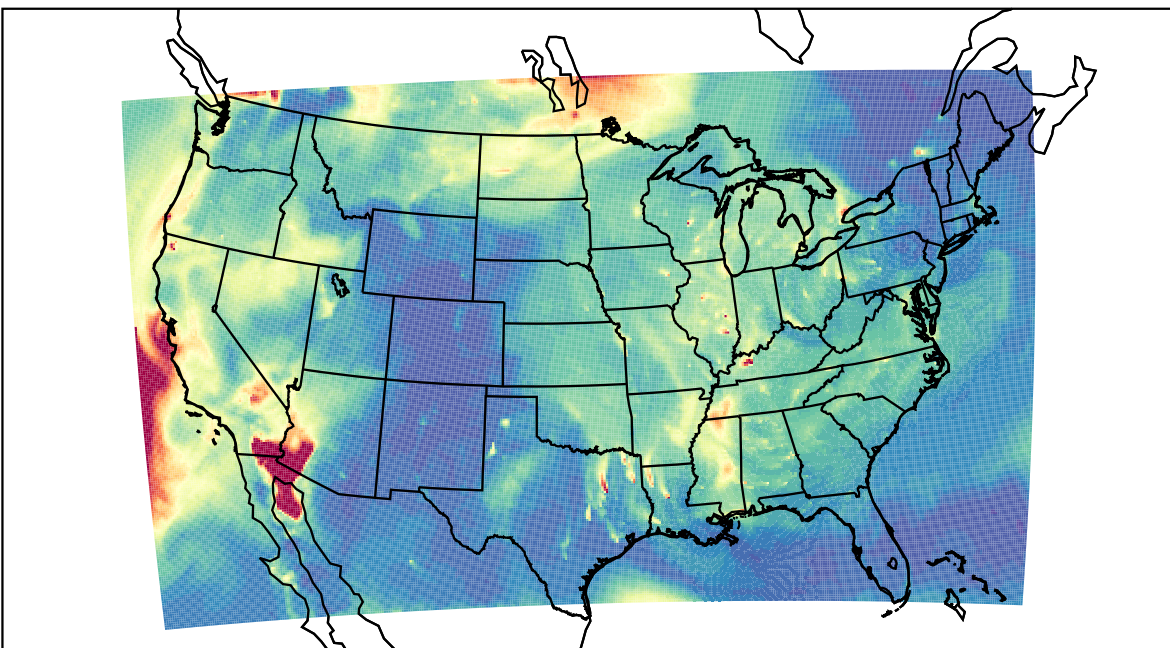
WRF 2023-09-21_14:00:00
