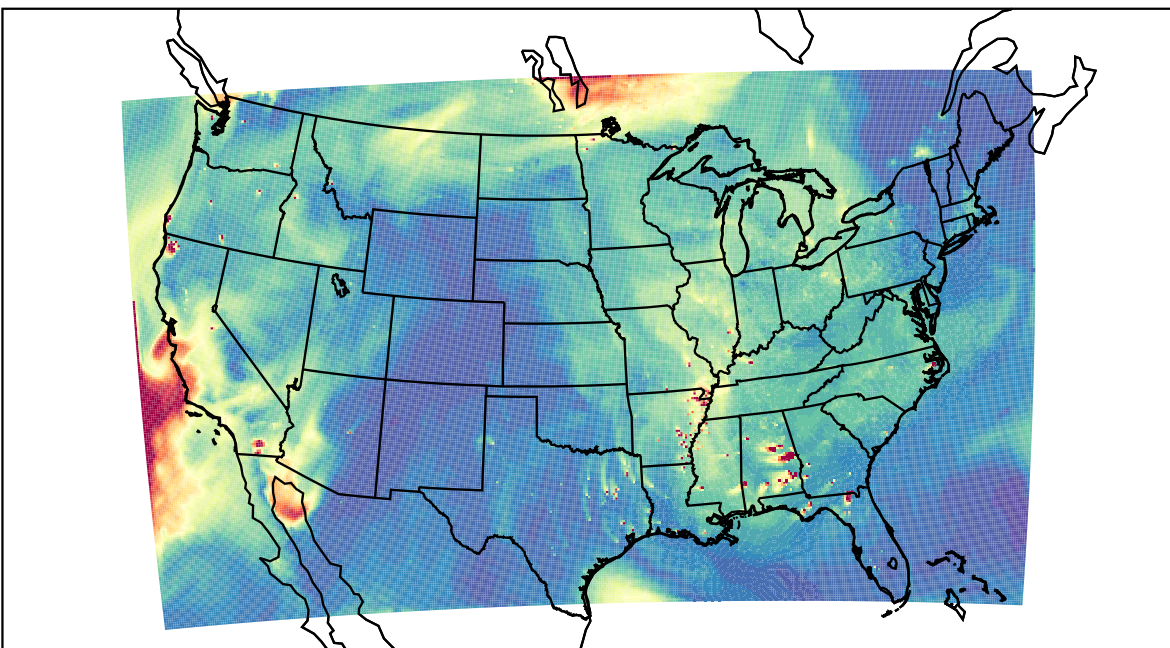
WRF 2023-09-21_22:00:00
