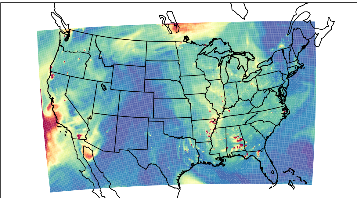
WRF 2023-09-21_23:00:00
