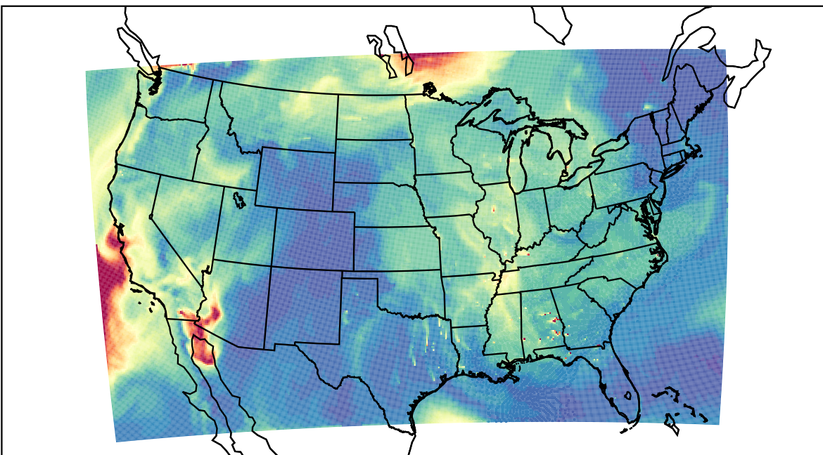
WRF 2023-09-21_18:00:00
