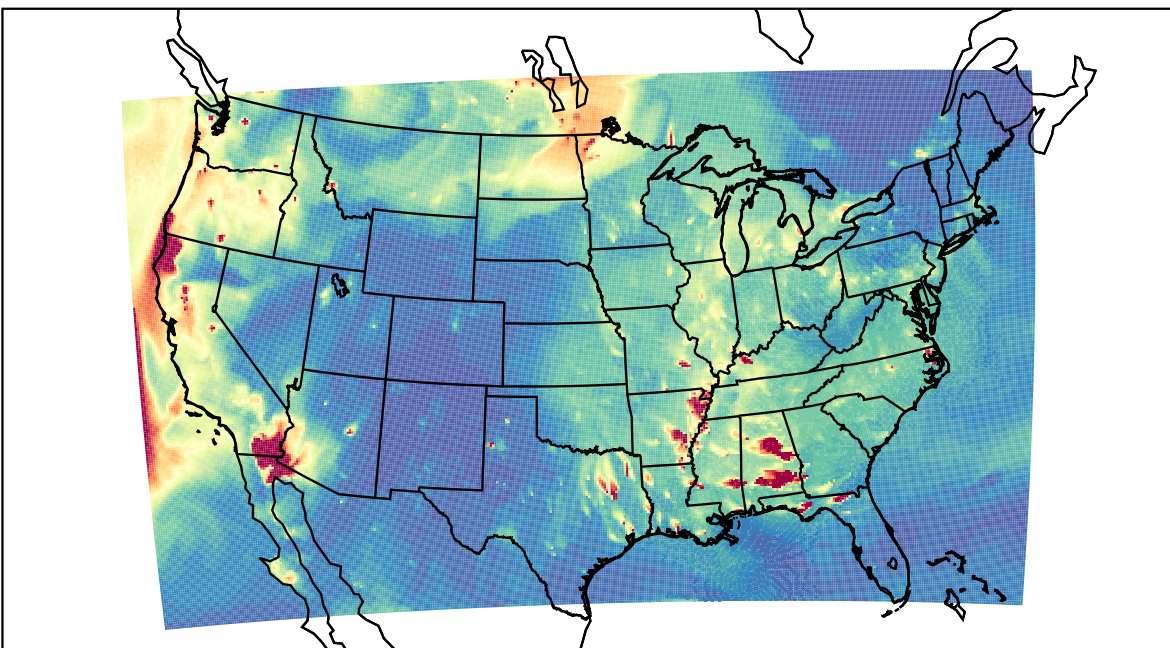
WRF 2023-09-21_02:00:00
