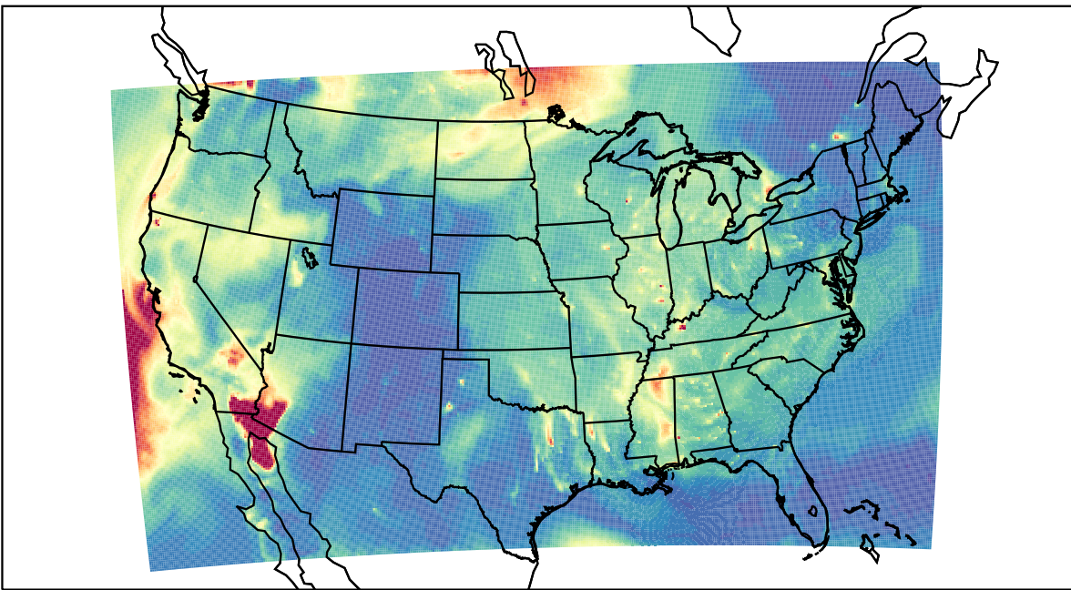
WRF 2023-09-21_13:00:00
