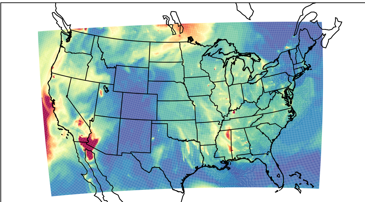
WRF 2023-09-21_11:00:00
