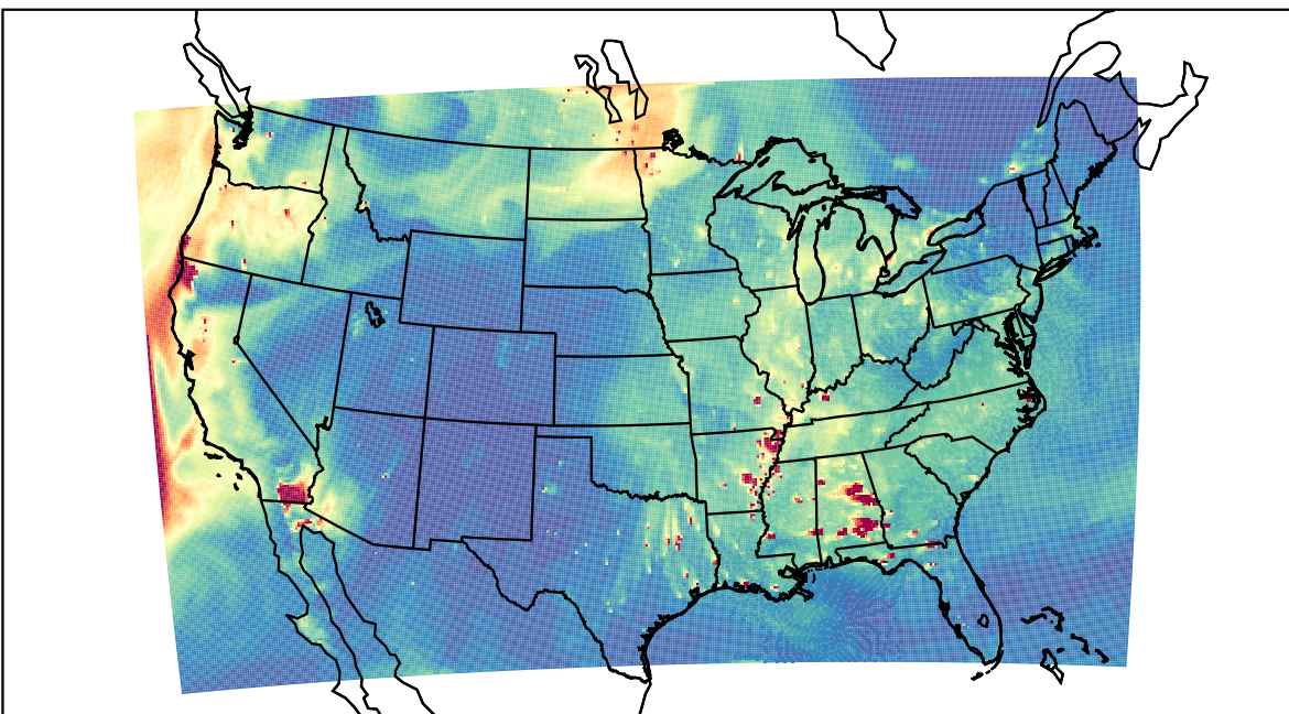
WRF 2023-09-21_00:00:00
