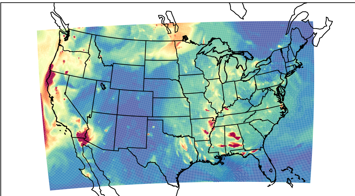
WRF 2023-09-21_03:00:00
