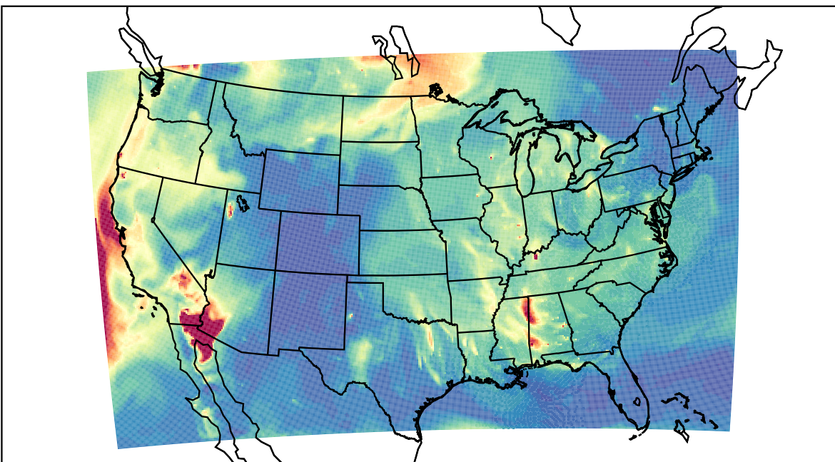
WRF 2023-09-21_09:00:00
