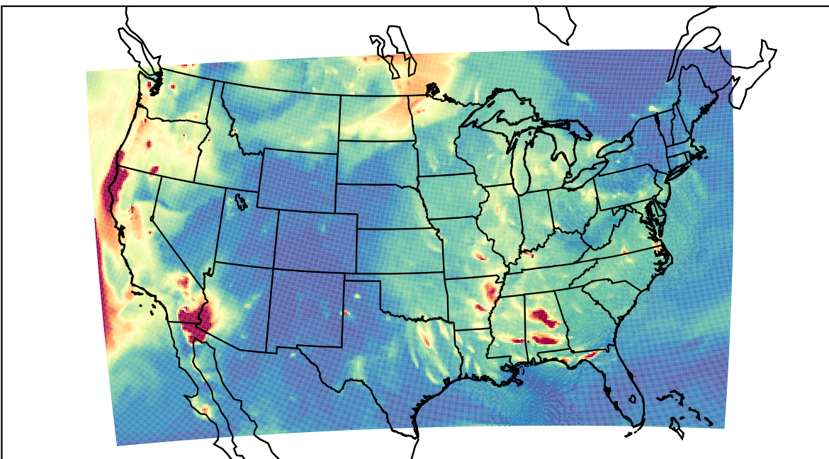
WRF 2023-09-21_04:00:00
