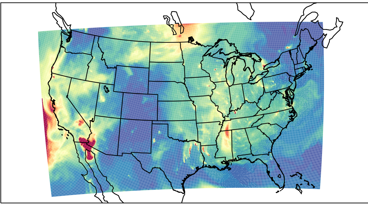
WRF 2023-09-21_14:00:00
