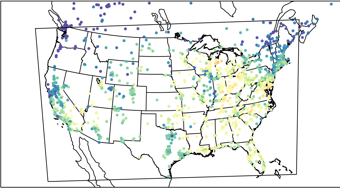
AirNOW (2023-09-21_16:00:00)
