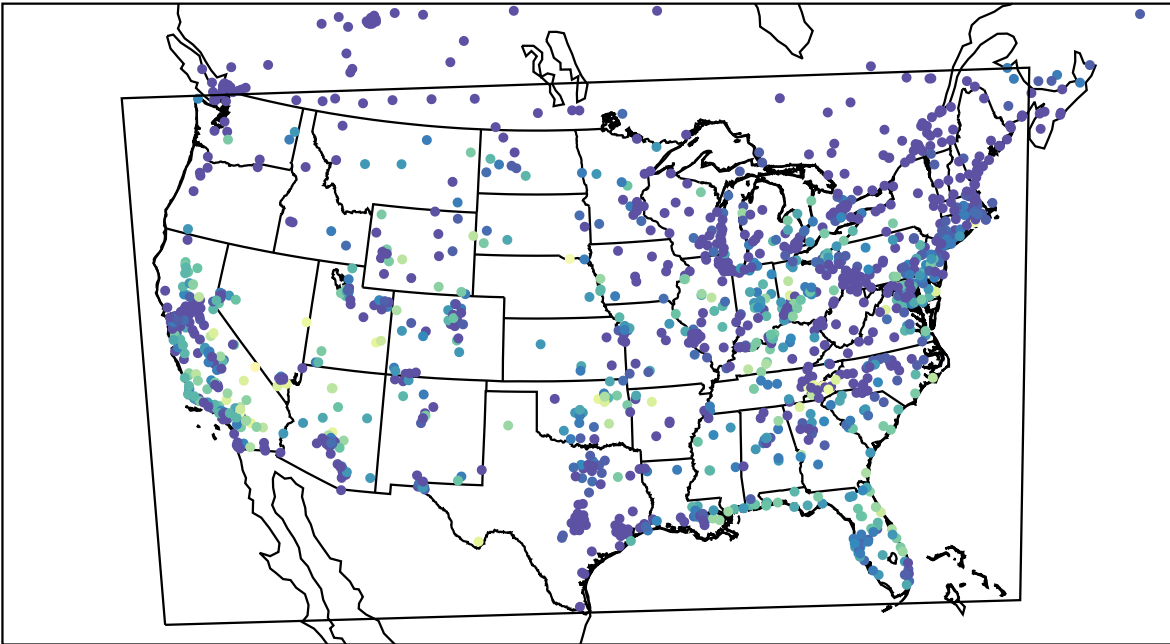
AirNOW (2023-09-21_13:00:00)
