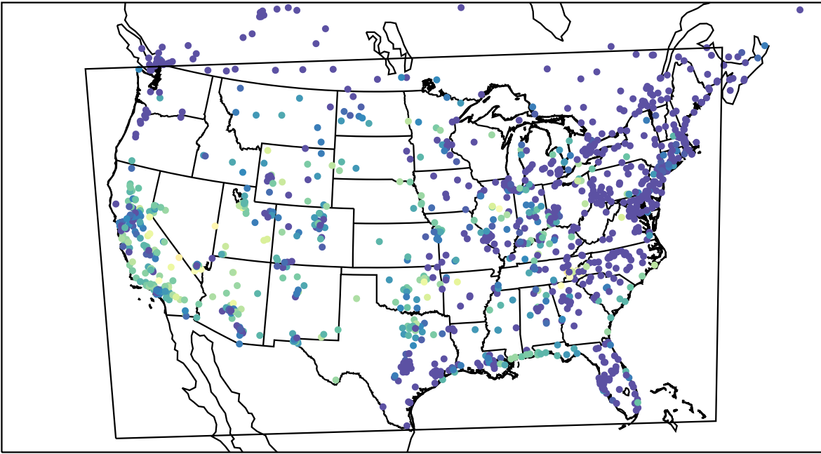
AirNOW (2023-09-21_10:00:00)
