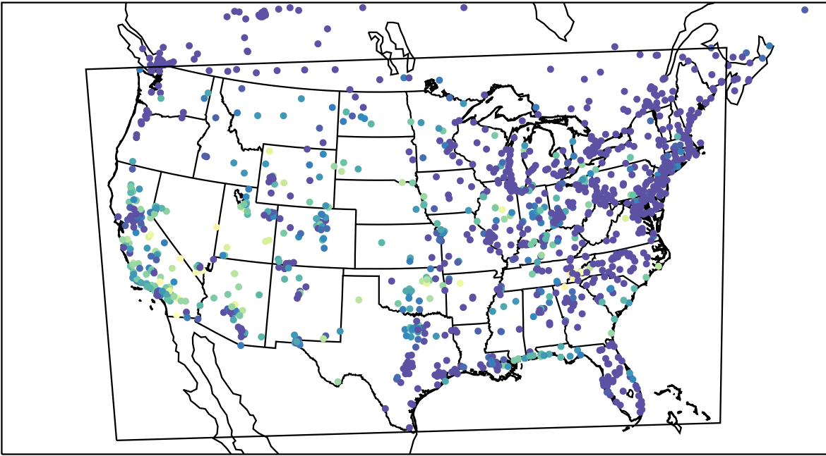
AirNOW (2023-09-21_11:00:00)
