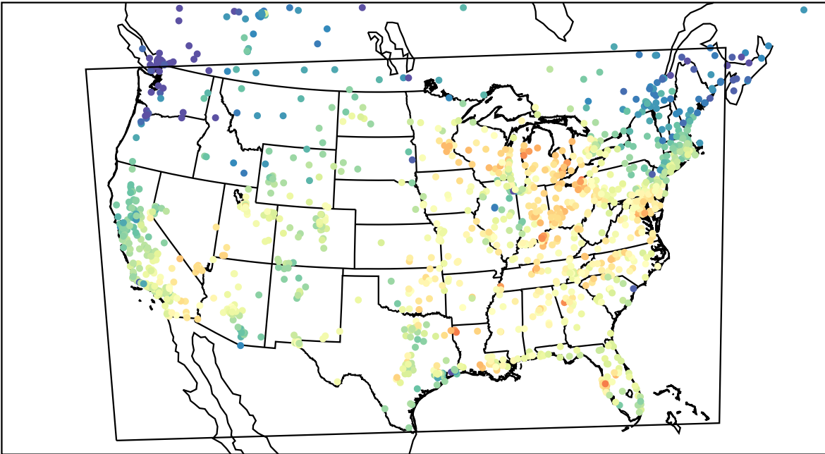
AirNOW (2023-09-21_18:00:00)
