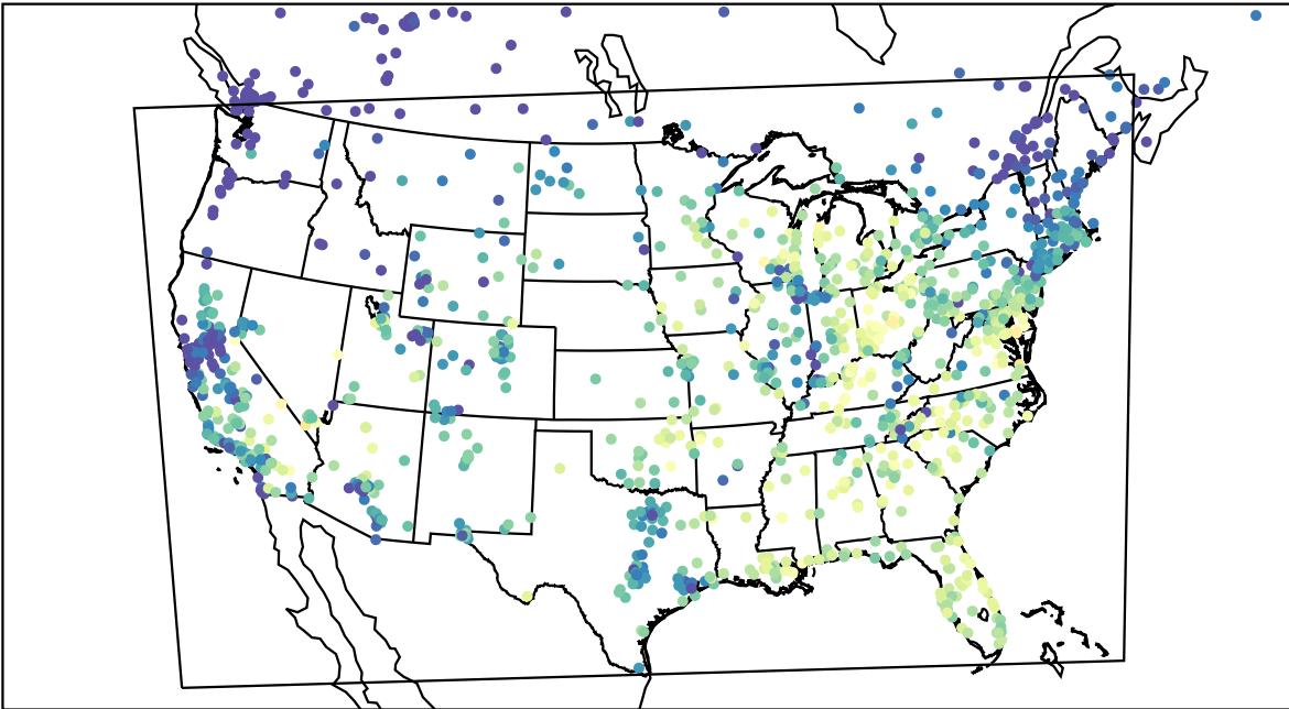
AirNOW (2023-09-21_15:00:00)
