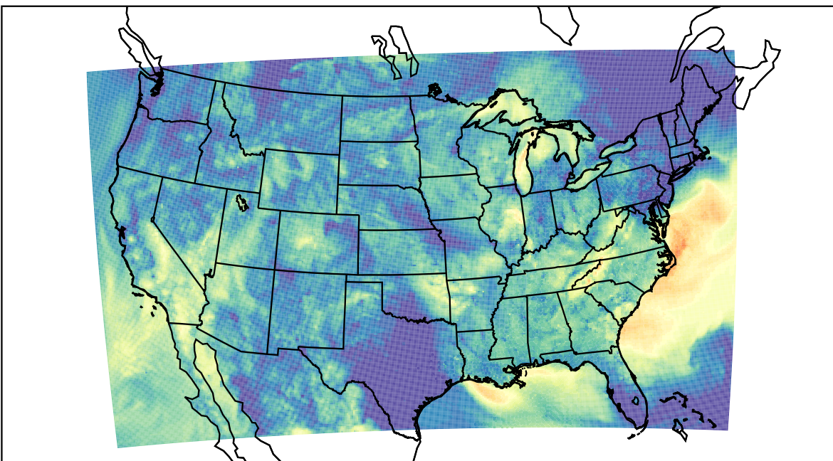
WRF (2023-09-21_13:00:00)
