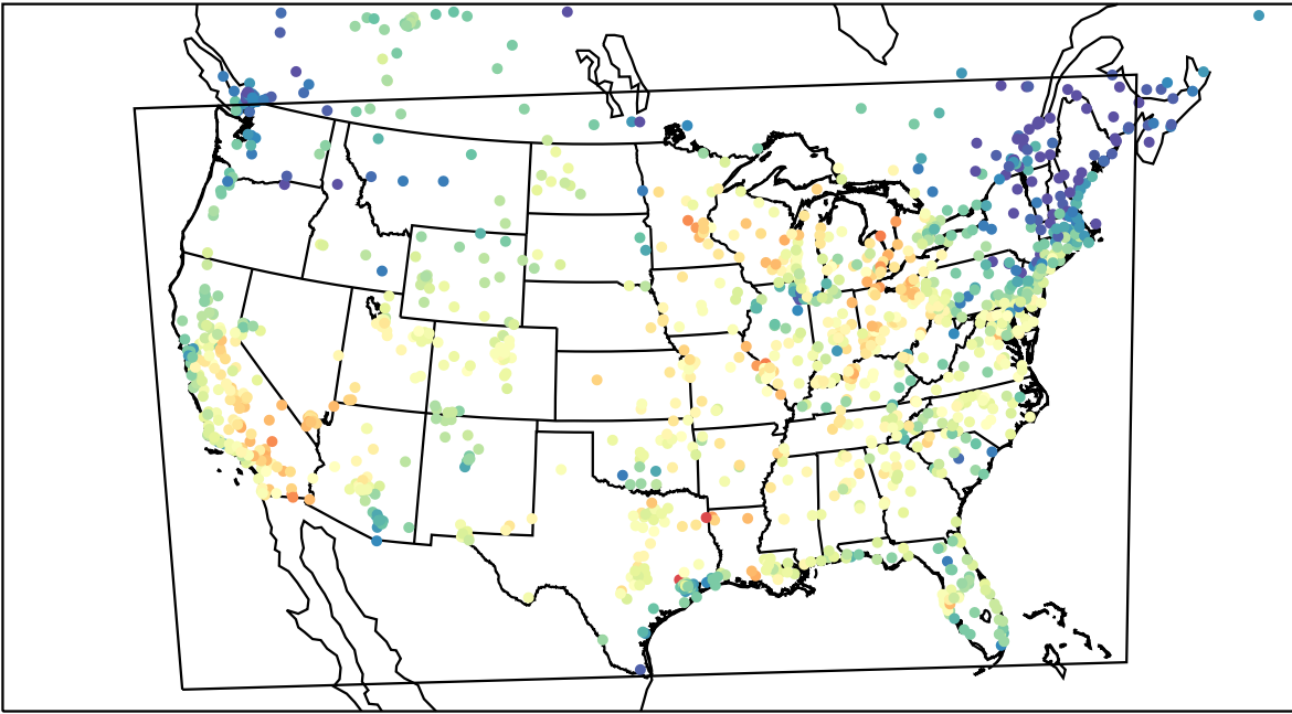
AirNOW (2023-09-21_22:00:00)
