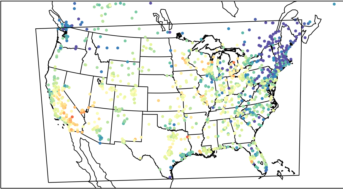
AirNOW (2023-09-21_23:00:00)
