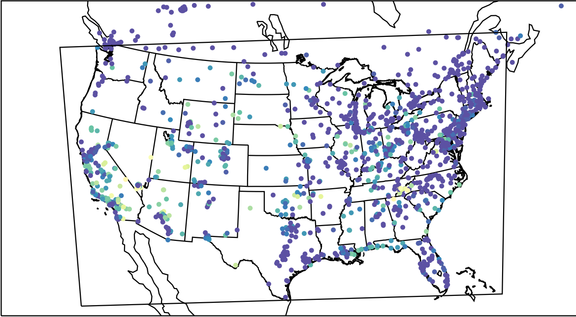
AirNOW (2023-09-21_12:00:00)
