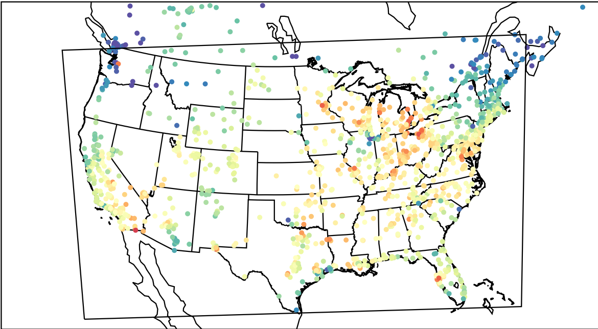
AirNOW (2023-09-21_20:00:00)
