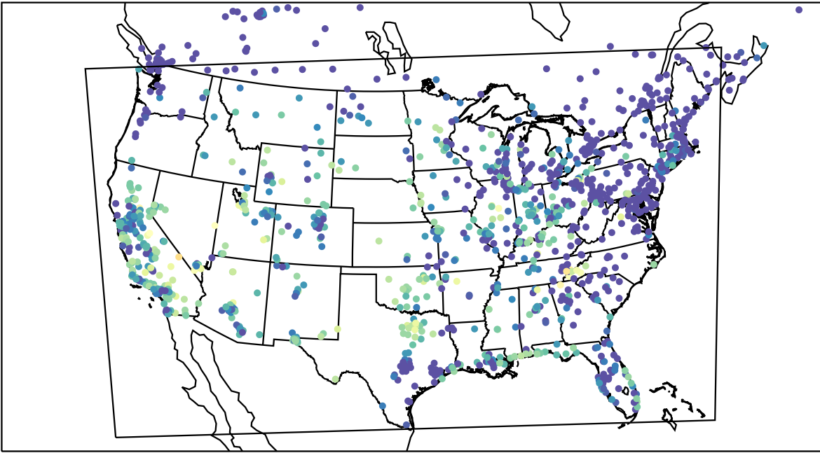
AirNOW (2023-09-21_08:00:00)
