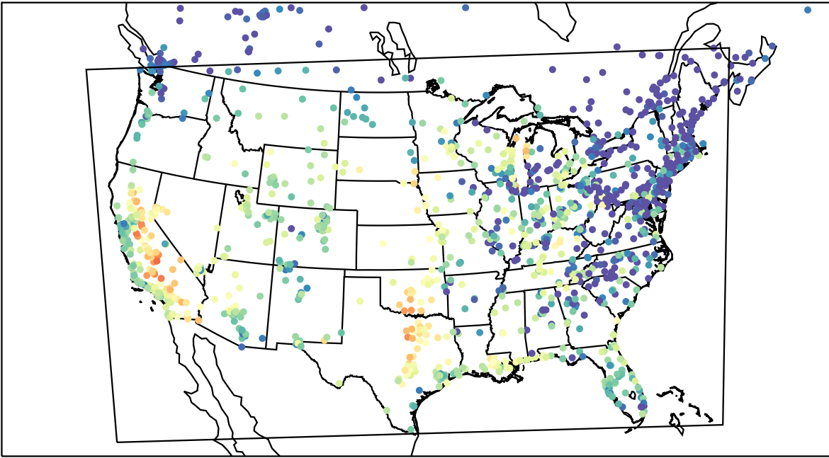
AirNOW (2023-09-21_01:00:00)
