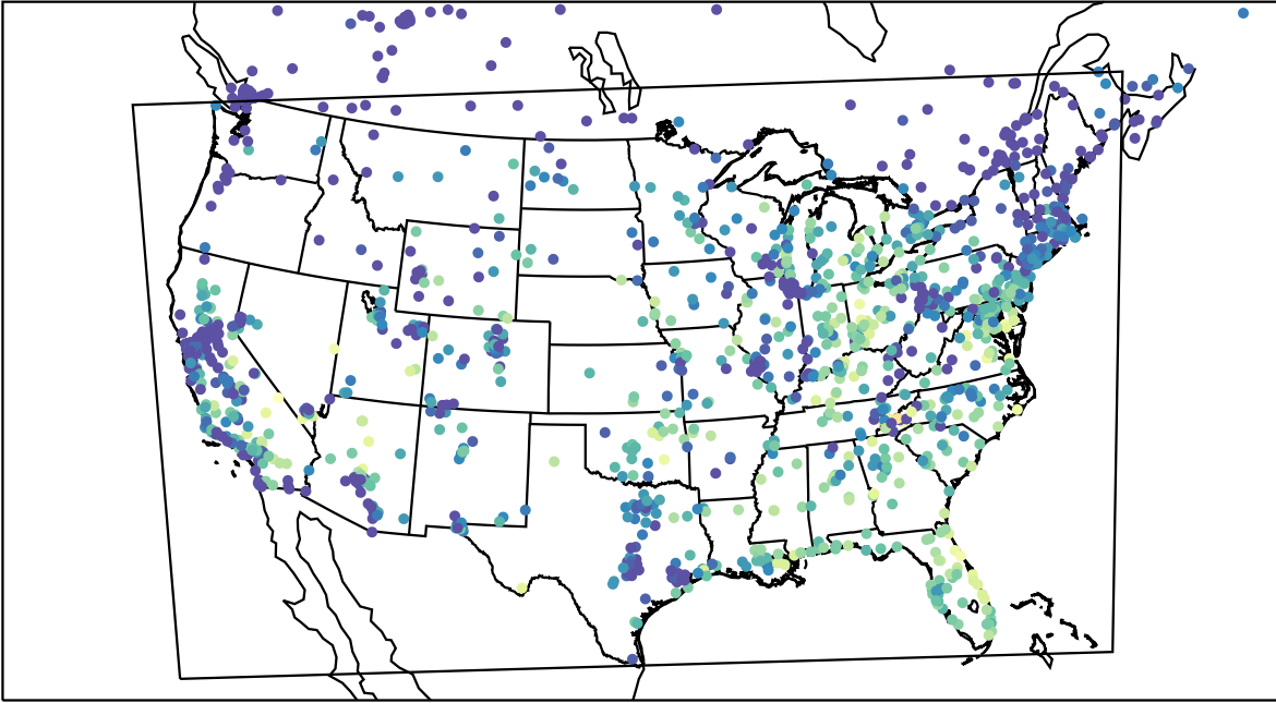
AirNOW (2023-09-21_14:00:00)
