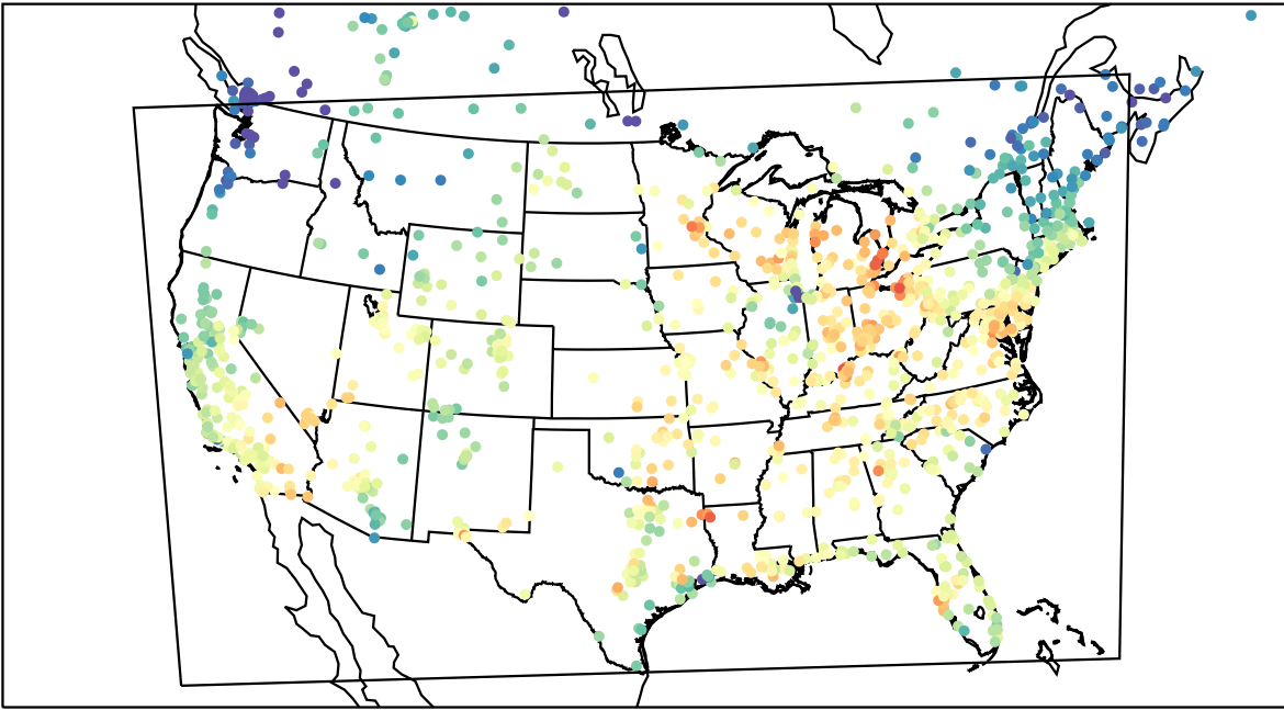
AirNOW (2023-09-21_19:00:00)
