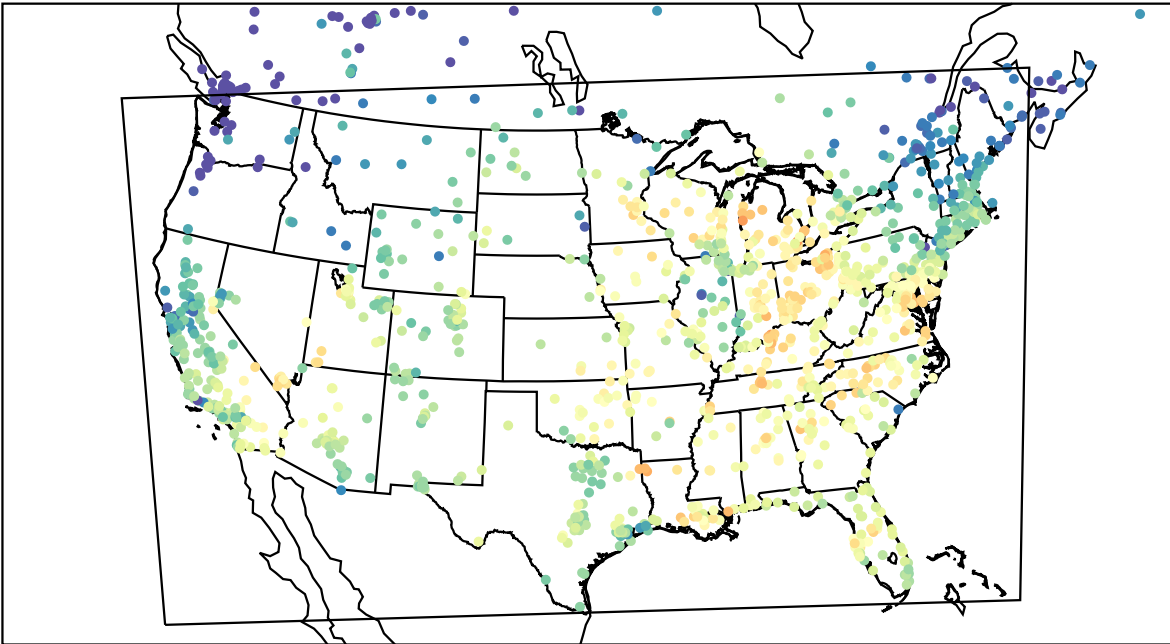
AirNOW (2023-09-21_17:00:00)
