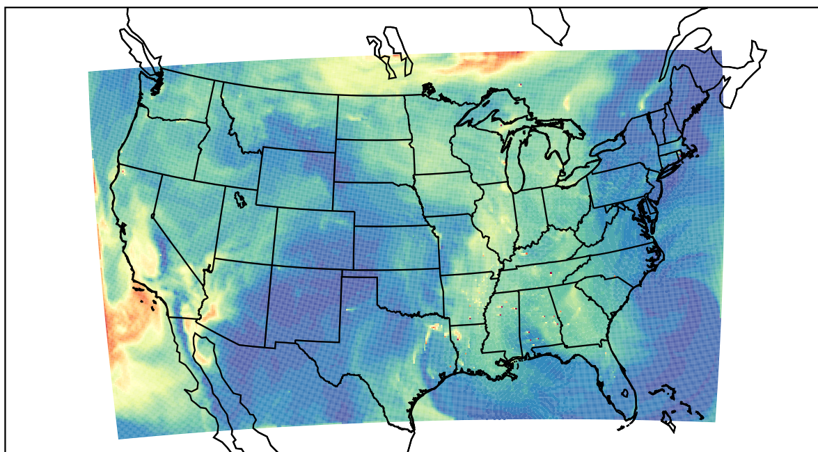
WRF 2023-09-22_18:00:00
