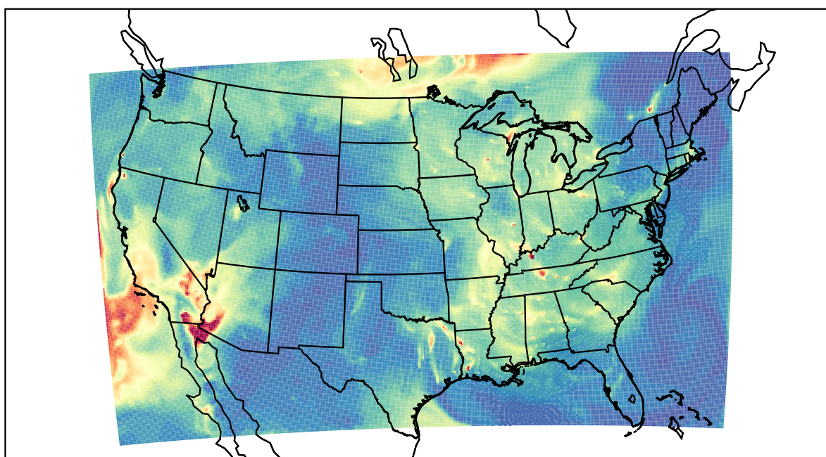
WRF 2023-09-22_10:00:00
