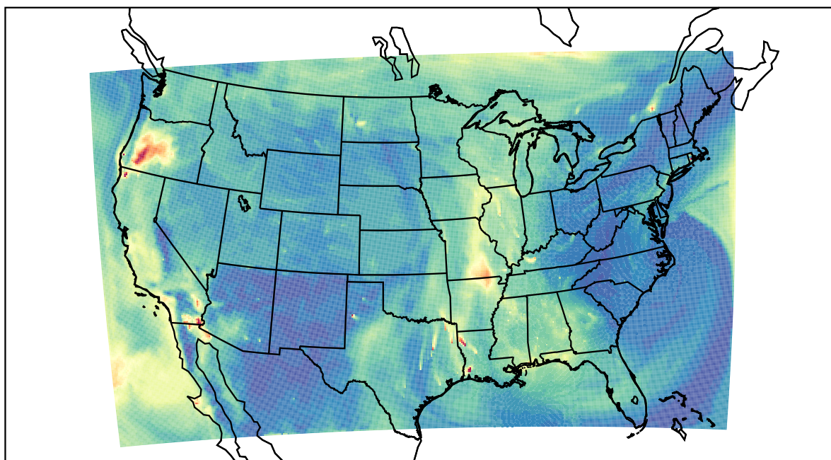
WRF 2023-09-23_16:00:00
