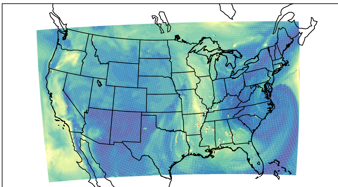
WRF 2023-09-23_20:00:00
