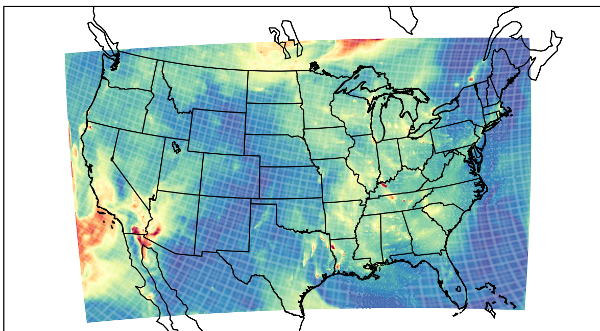
WRF 2023-09-22_13:00:00
