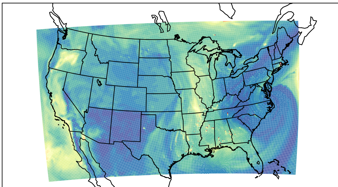
WRF 2023-09-23_19:00:00
