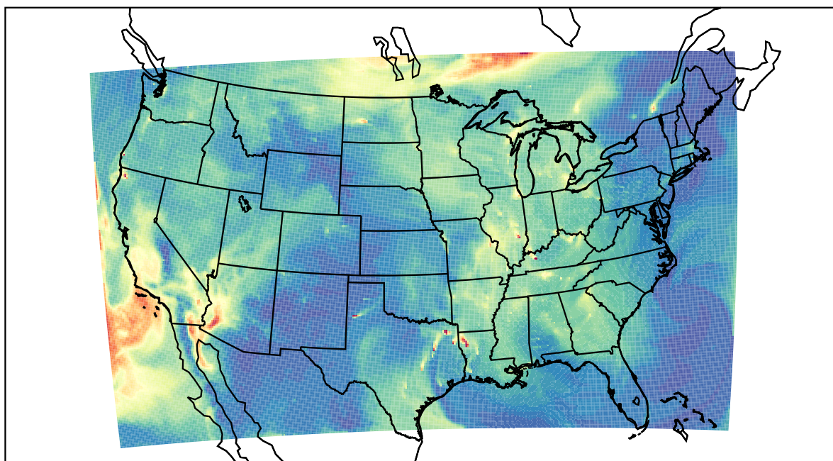
WRF 2023-09-22_16:00:00
