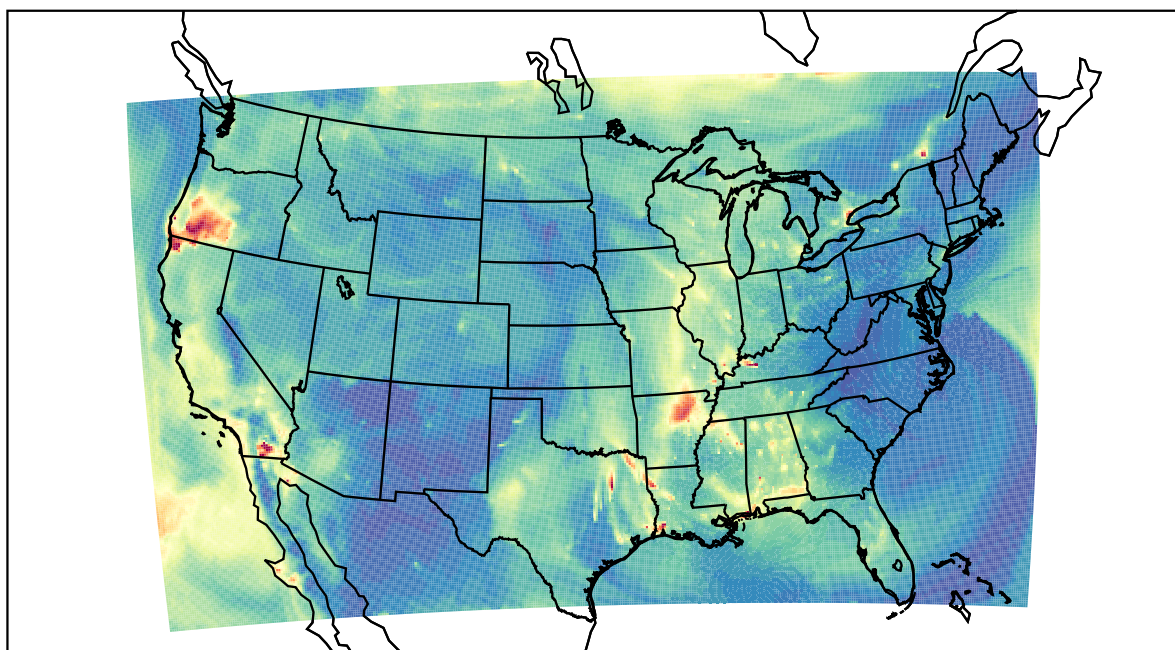
WRF 2023-09-23_13:00:00
