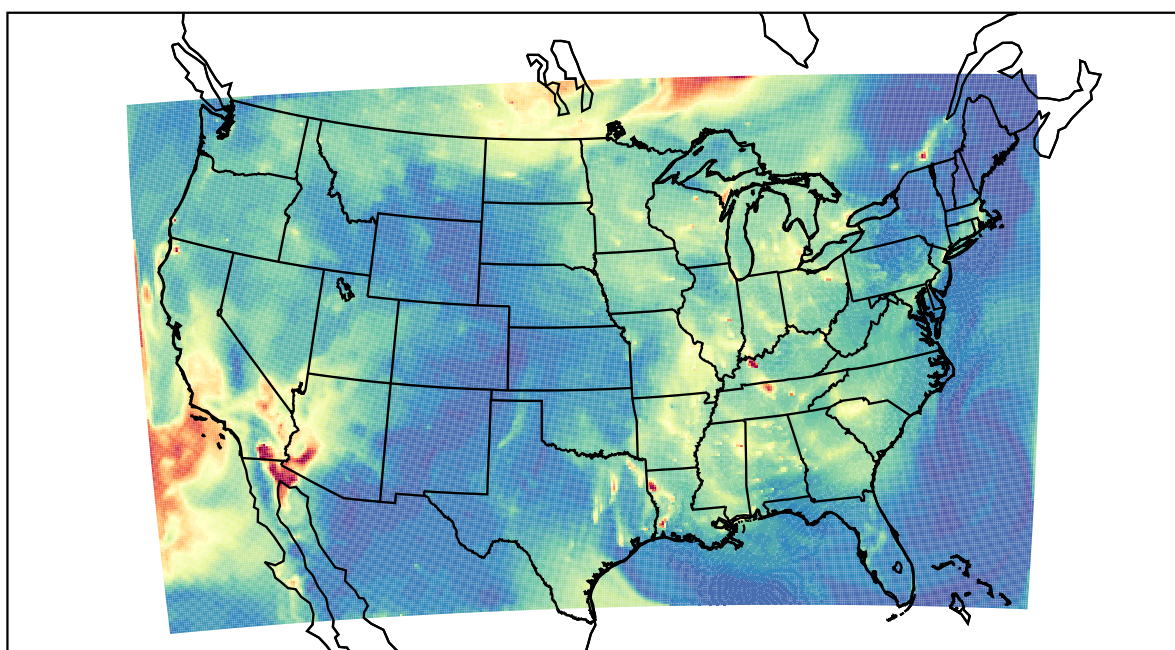
WRF 2023-09-22_12:00:00
