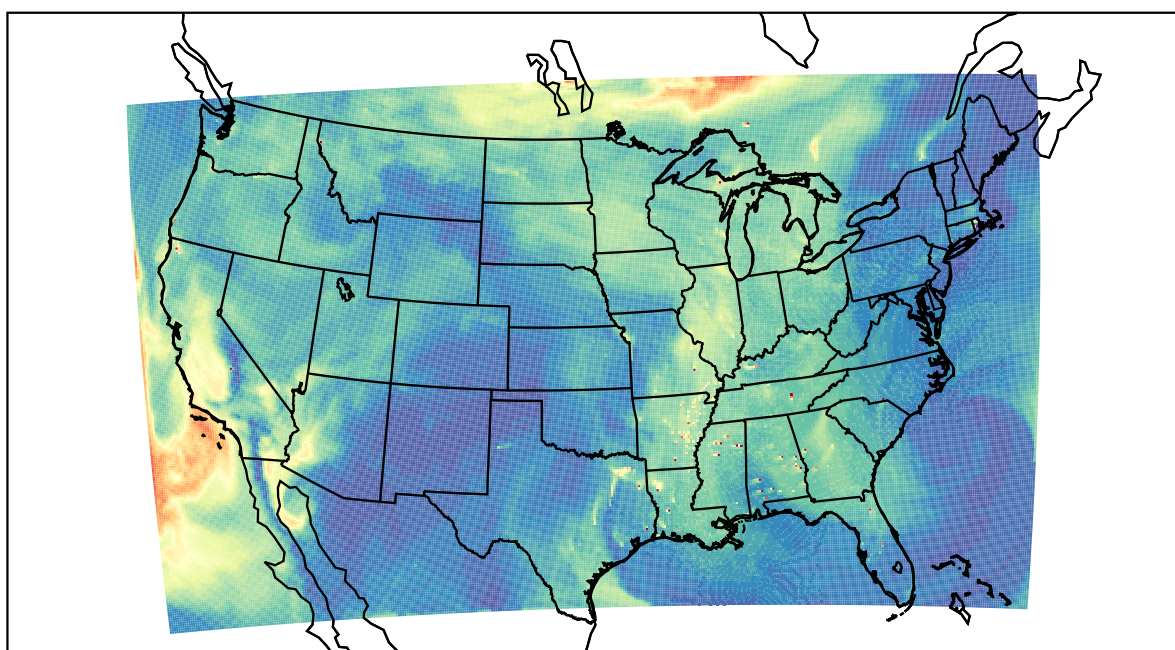
WRF 2023-09-22_19:00:00
