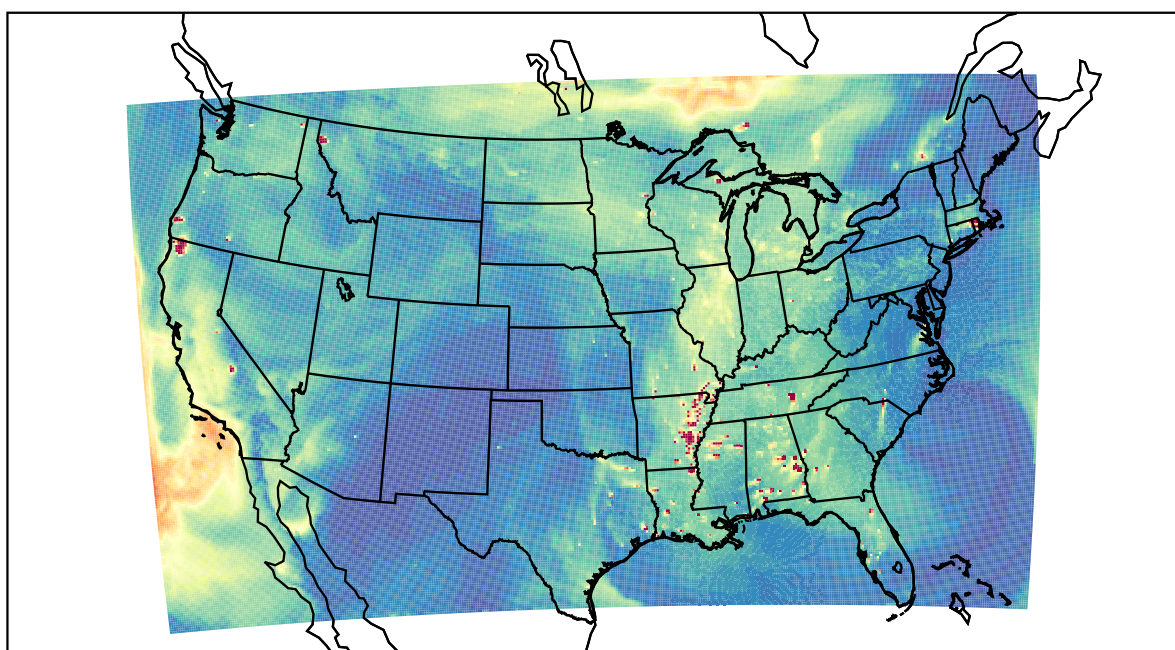
WRF 2023-09-22_23:00:00
