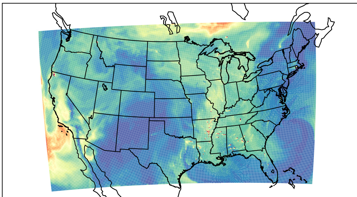
WRF 2023-09-22_20:00:00
