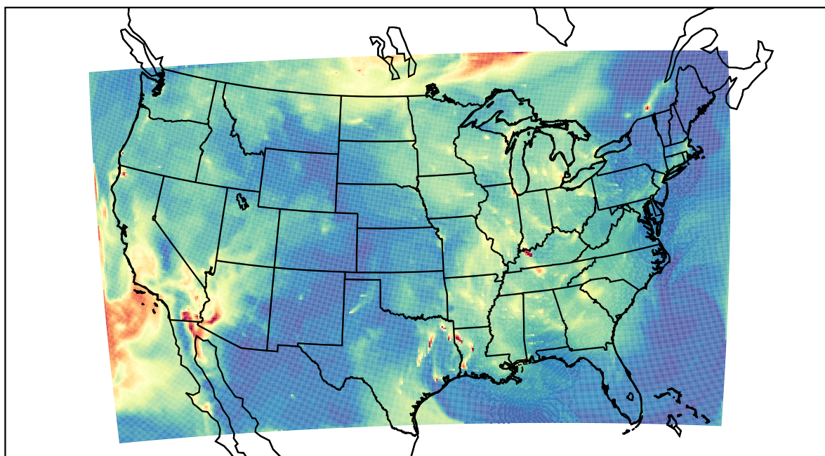
WRF 2023-09-22_14:00:00
