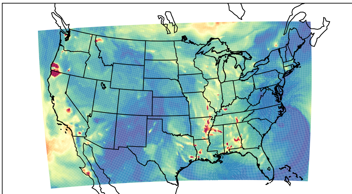
WRF 2023-09-23_04:00:00
