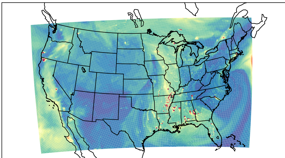
WRF 2023-09-23_23:00:00
