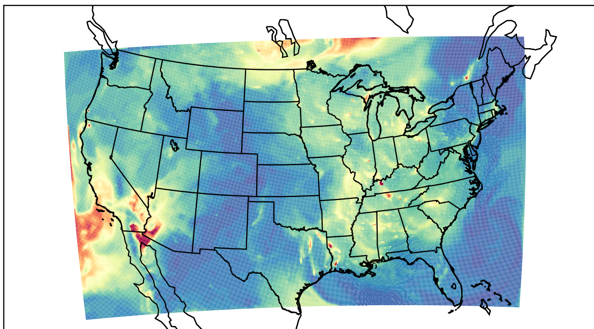
WRF 2023-09-22_11:00:00
