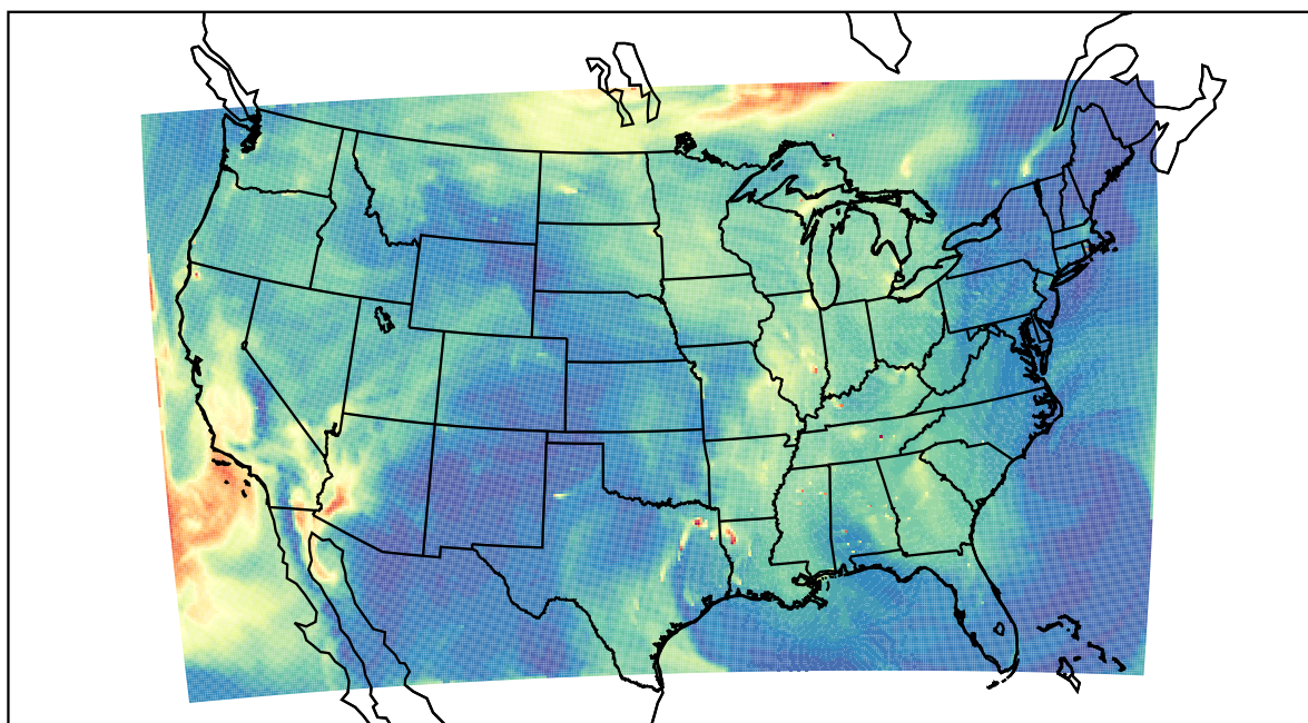
WRF 2023-09-22_17:00:00
