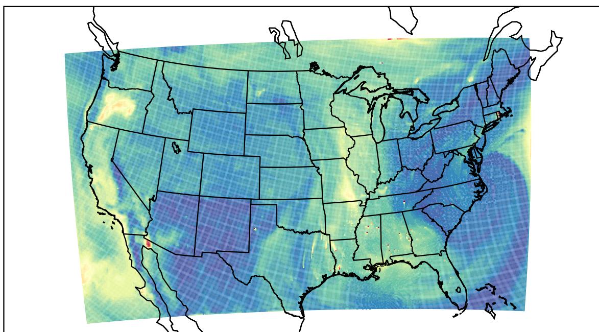
WRF 2023-09-23_18:00:00
