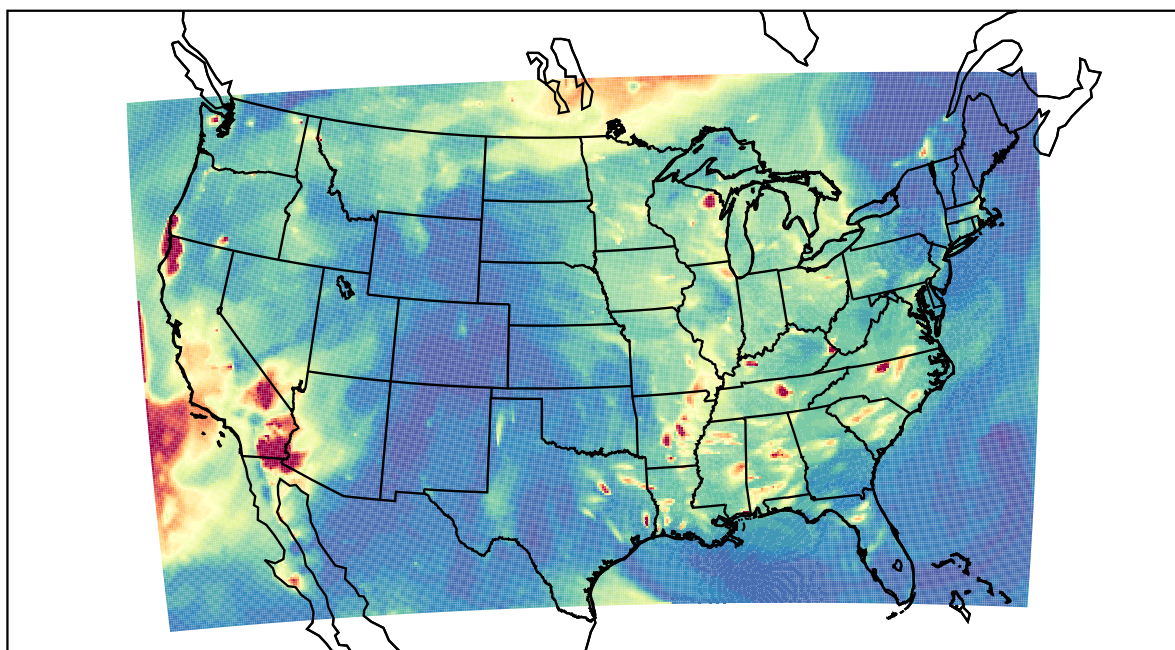
WRF 2023-09-22_04:00:00
