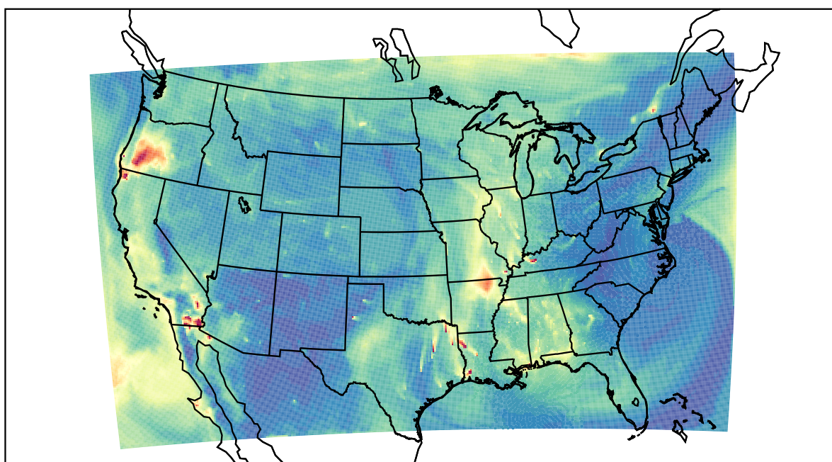
WRF 2023-09-23_15:00:00
