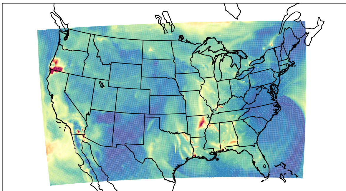
WRF 2023-09-23_10:00:00
