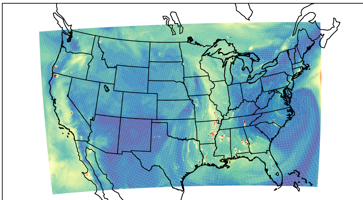
WRF 2023-09-23_22:00:00
