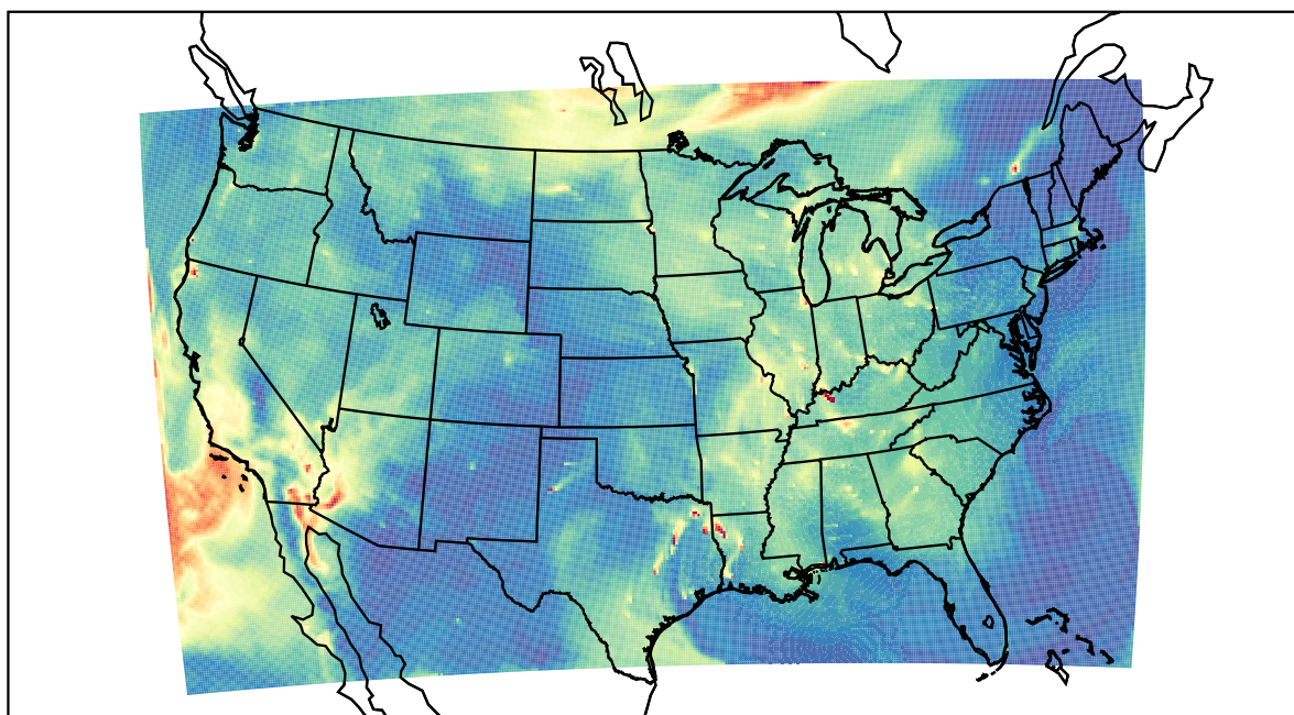
WRF 2023-09-22_15:00:00
