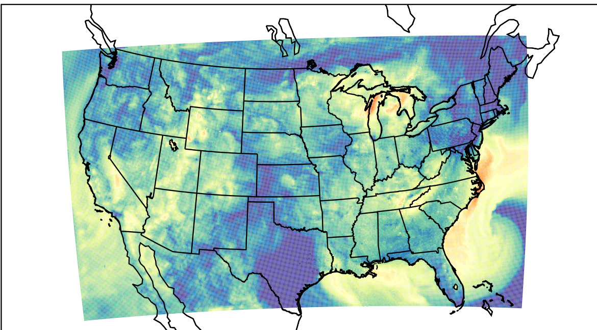
WRF (2023-09-22_10:00:00)
