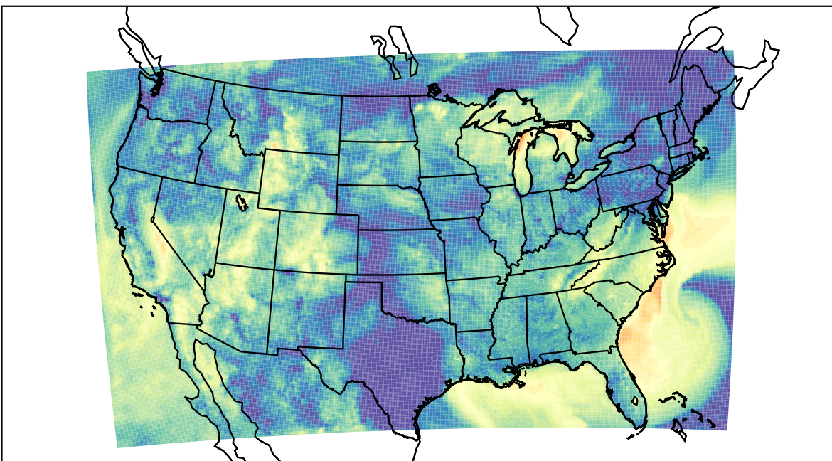
WRF (2023-09-22_13:00:00)
