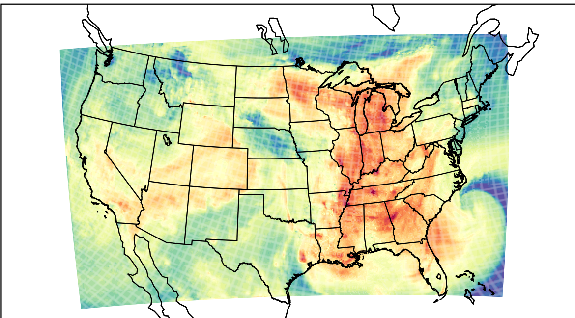
WRF (2023-09-22_20:00:00)
