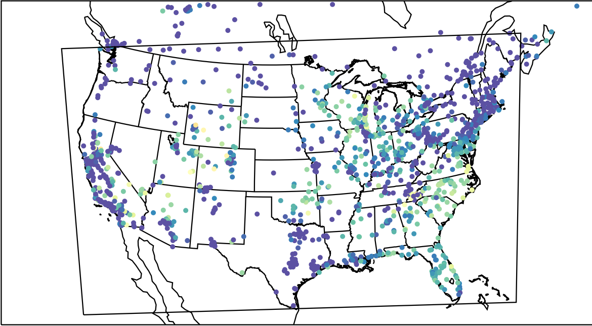
AirNOW (2023-09-22_13:00:00)
