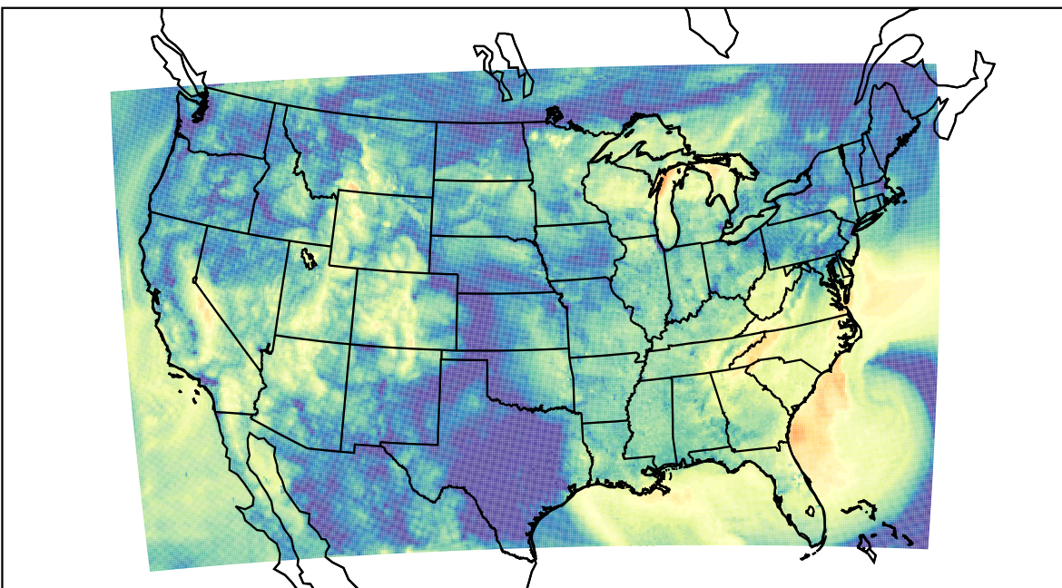
WRF (2023-09-22_14:00:00)
