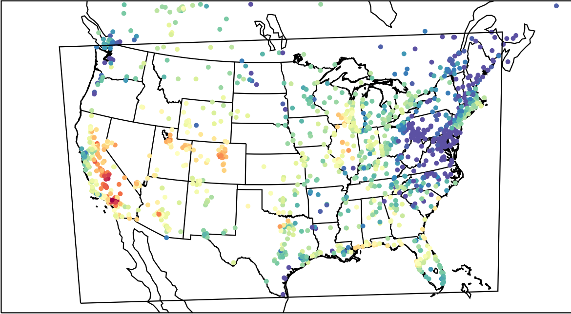
AirNOW (2023-09-24_23:00:00)
