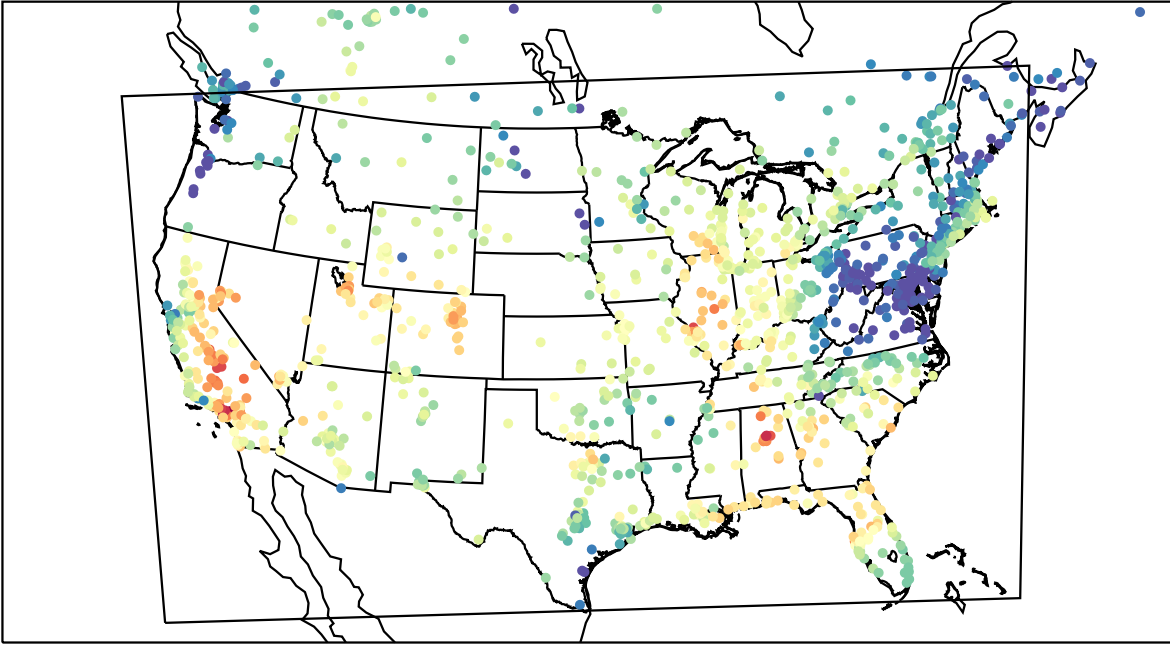
AirNOW (2023-09-24_20:00:00)
