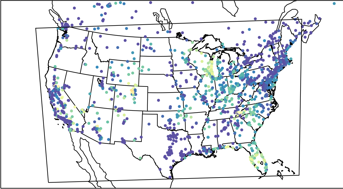
AirNOW (2023-09-23_13:00:00)
