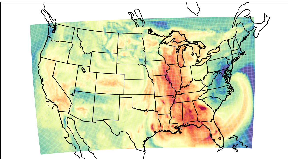
WRF (2023-09-23_20:00:00)
