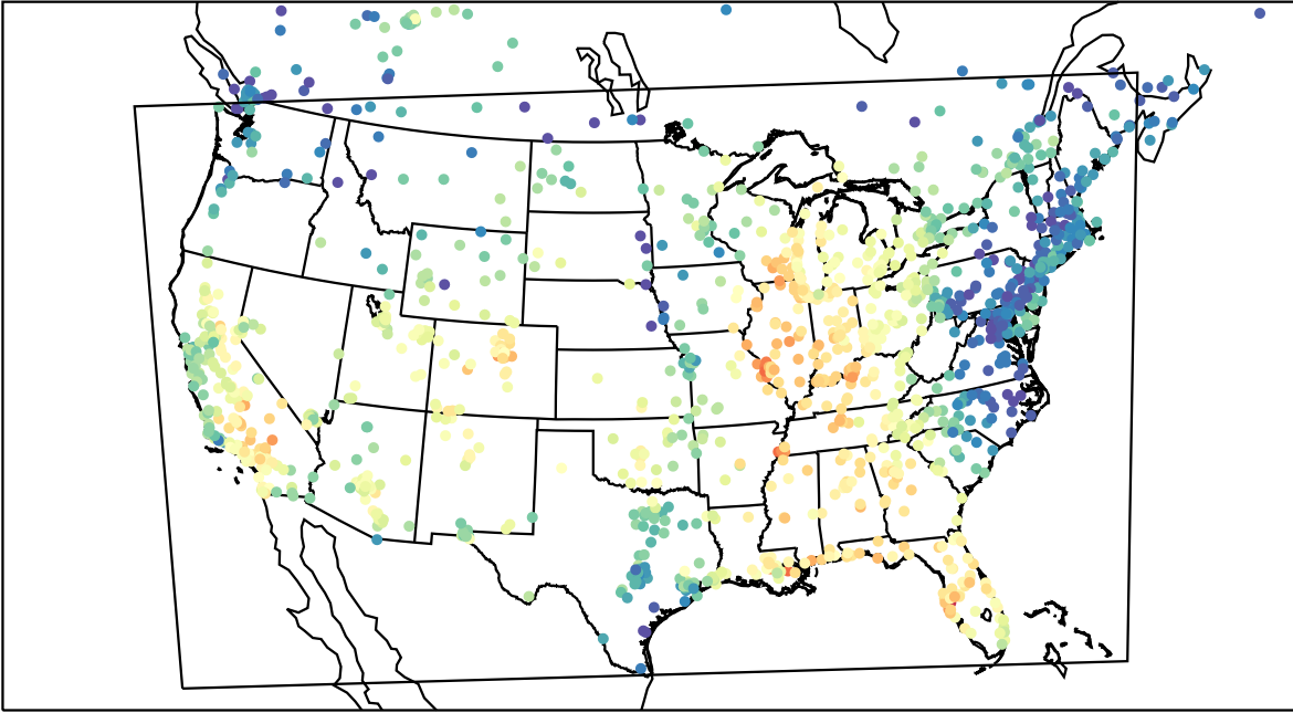
AirNOW (2023-09-23_18:00:00)
