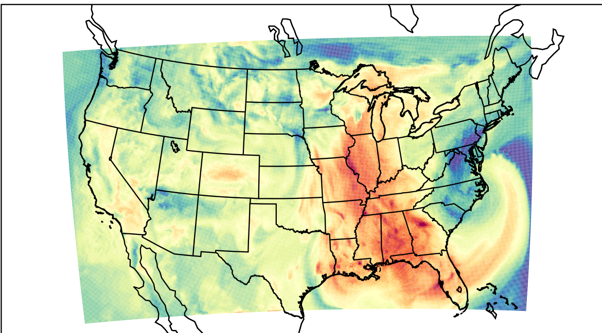
WRF (2023-09-23_18:00:00)
