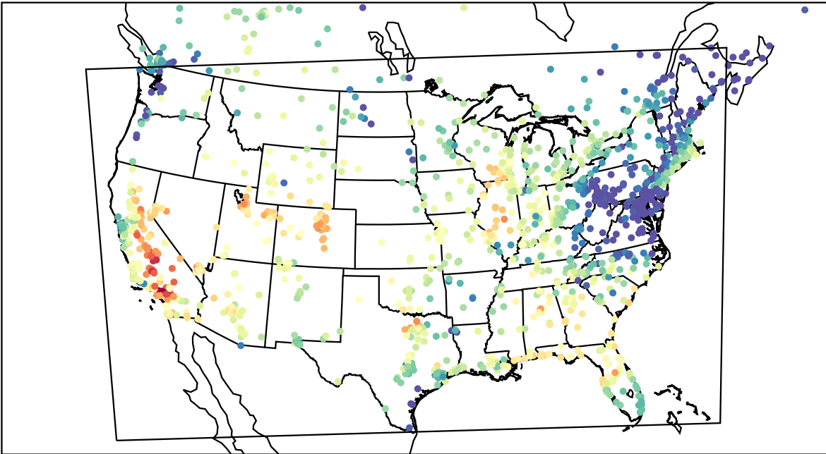
AirNOW (2023-09-24_22:00:00)
