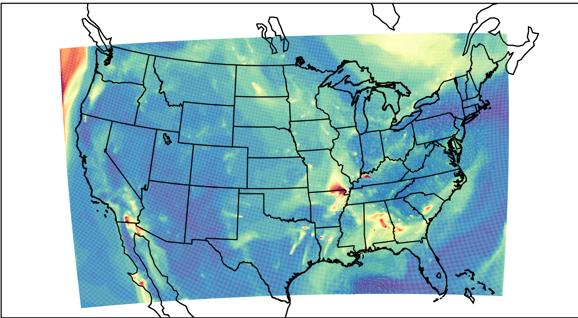
WRF 2023-09-25_10:00:00
