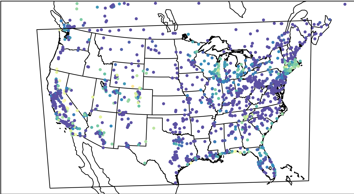
AirNOW (2023-09-25_13:00:00)
