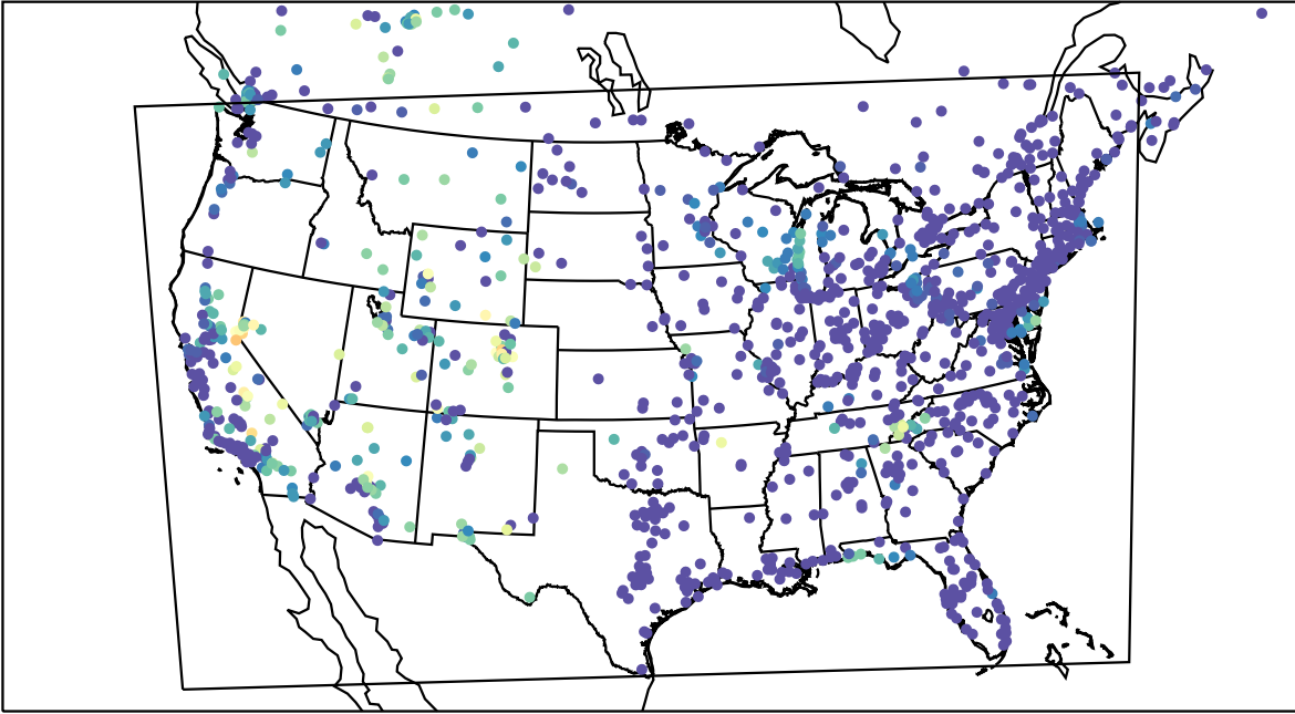
AirNOW (2023-09-26_11:00:00)
