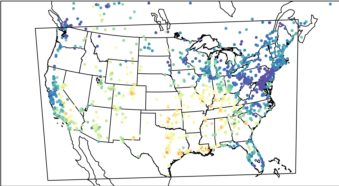
AirNOW (2023-09-26_17:00:00)
