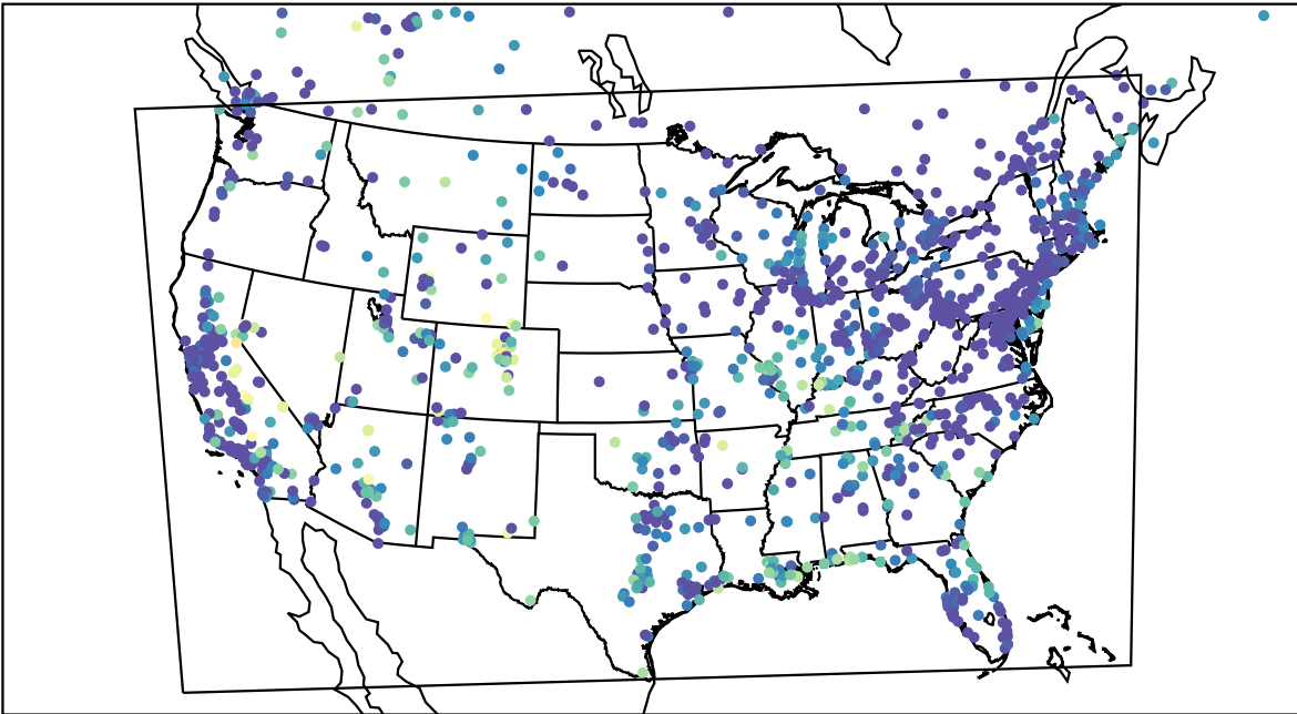
AirNOW (2023-09-26_14:00:00)
