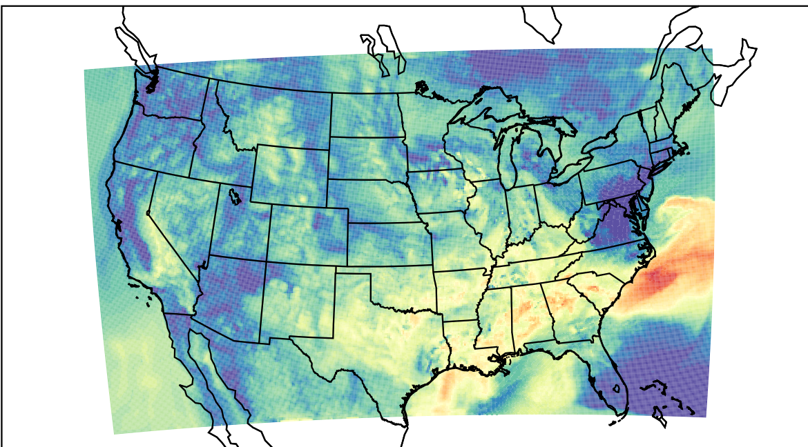
WRF (2023-09-26_15:00:00)
