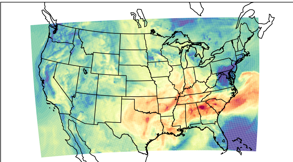
WRF (2023-09-26_17:00:00)
