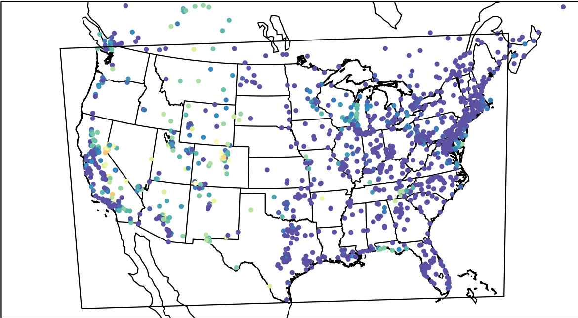
AirNOW (2023-09-26_10:00:00)
