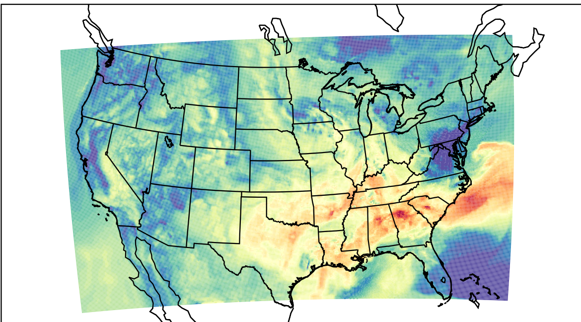
WRF (2023-09-26_16:00:00)
