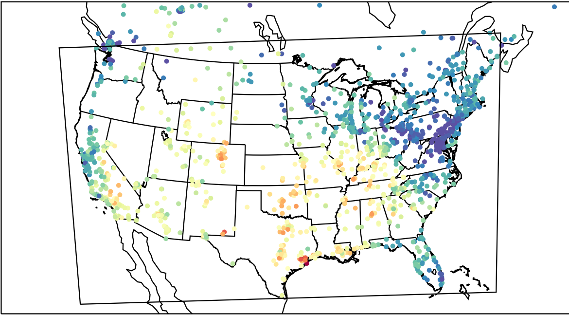
AirNOW (2023-09-26_18:00:00)
