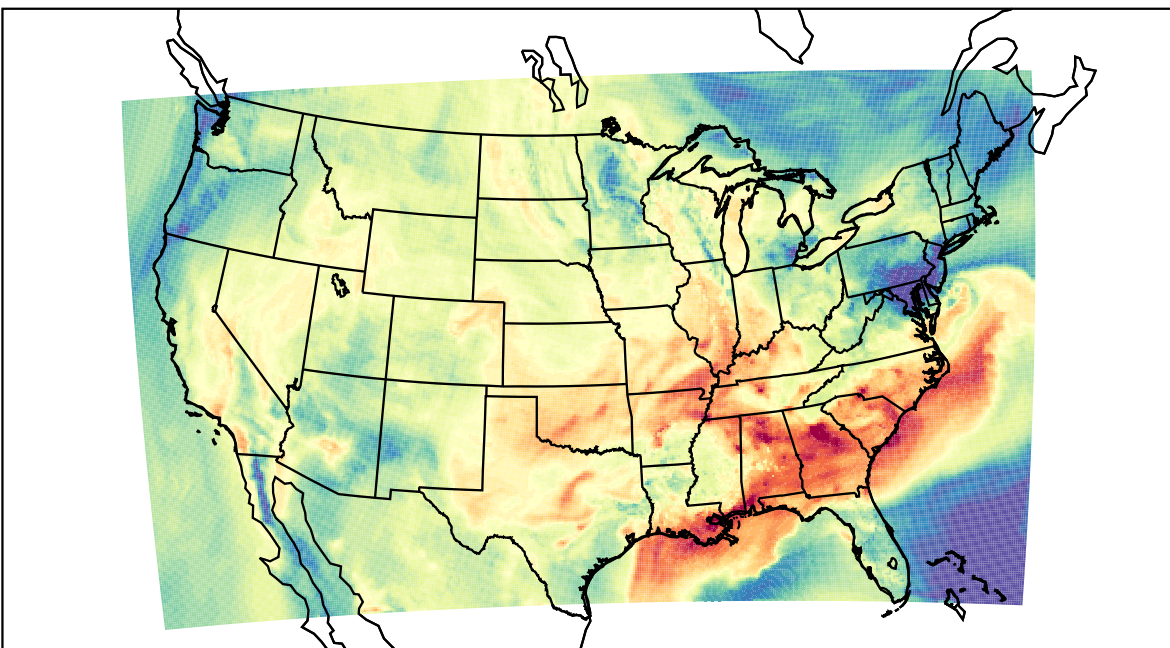
WRF (2023-09-25_20:00:00)
