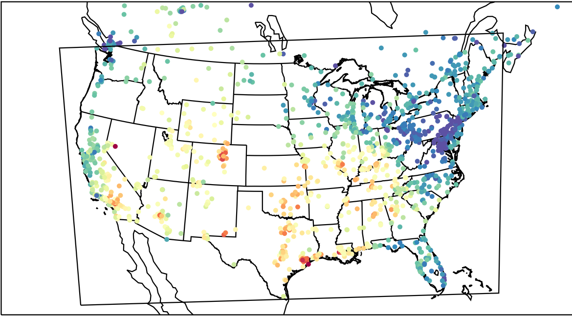
AirNOW (2023-09-26_19:00:00)
