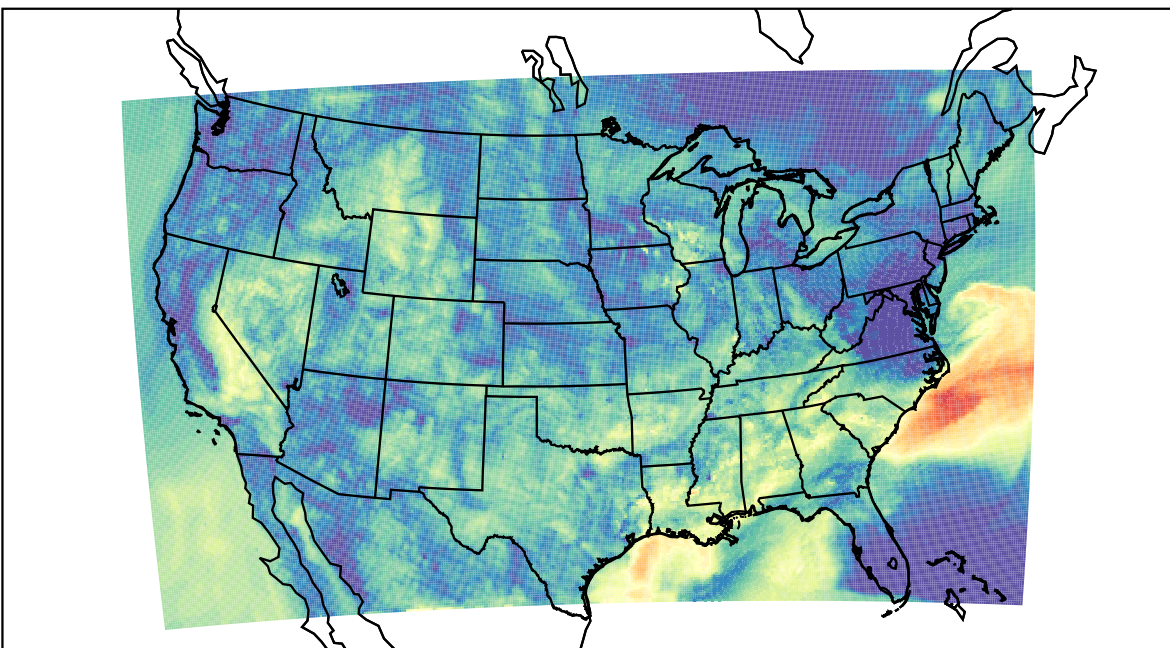
WRF (2023-09-26_14:00:00)
