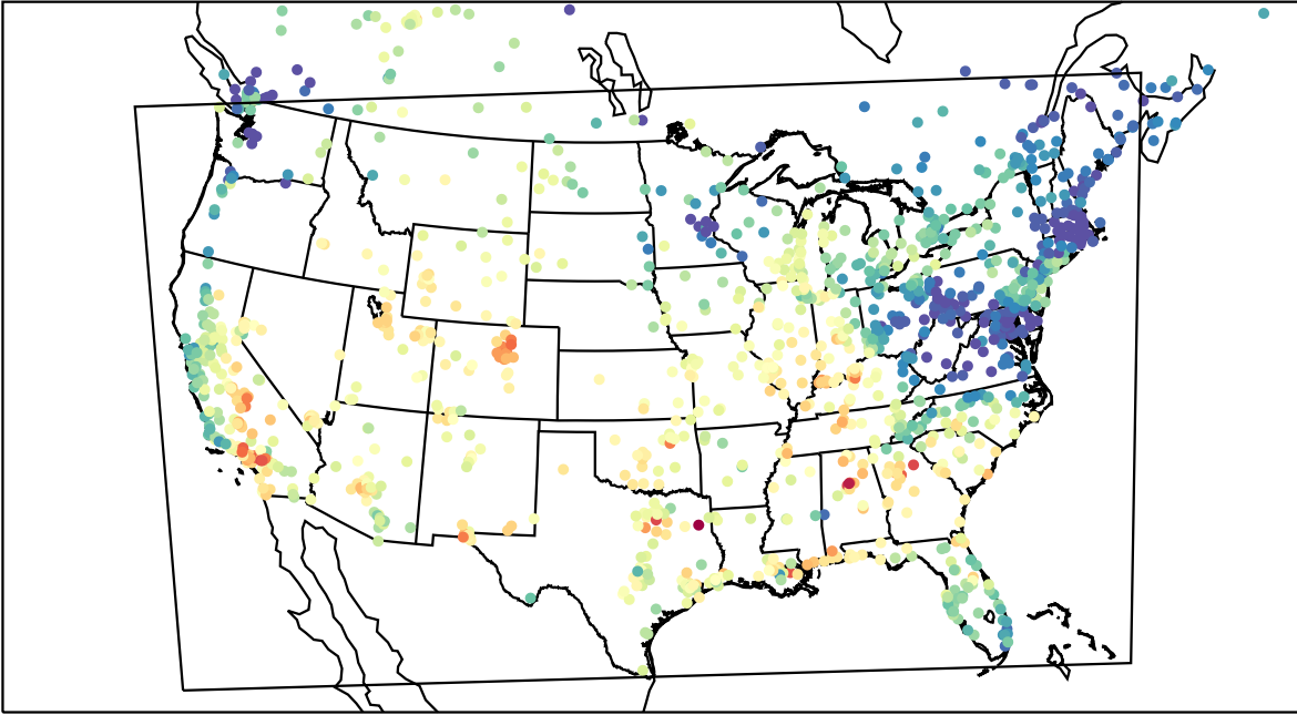
AirNOW (2023-09-25_20:00:00)
