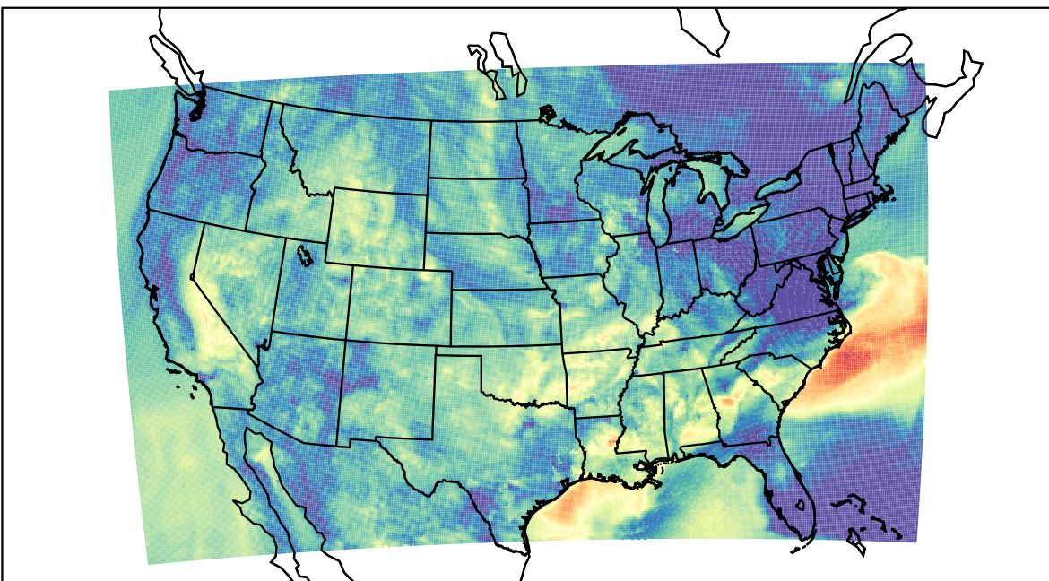
WRF (2023-09-26_10:00:00)
