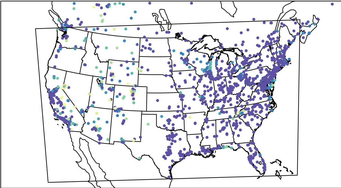
AirNOW (2023-09-26_12:00:00)
