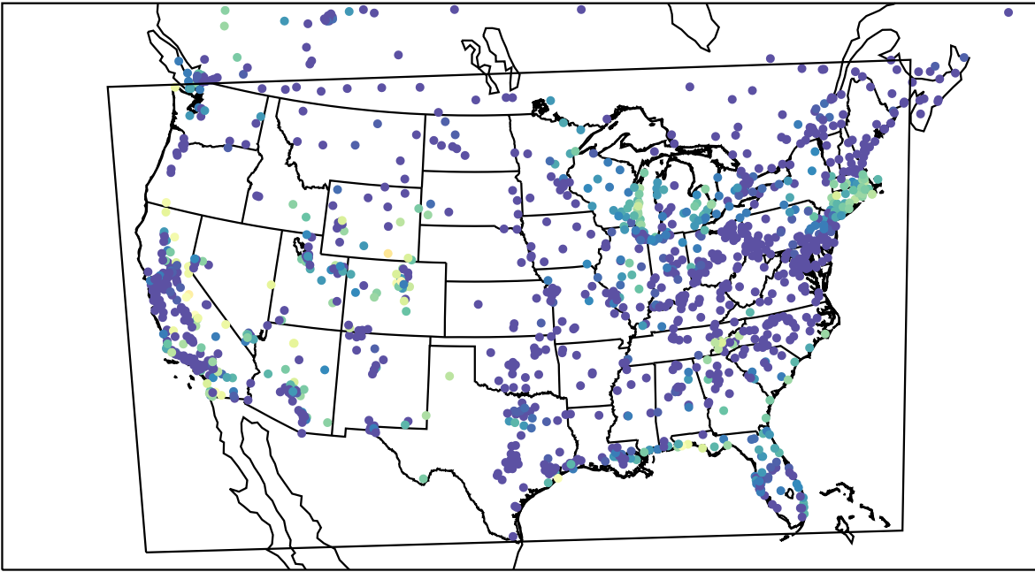
AirNOW (2023-09-25_13:00:00)
