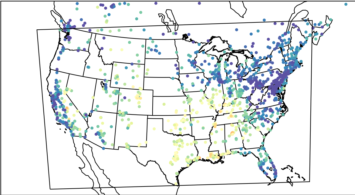
AirNOW (2023-09-26_16:00:00)
