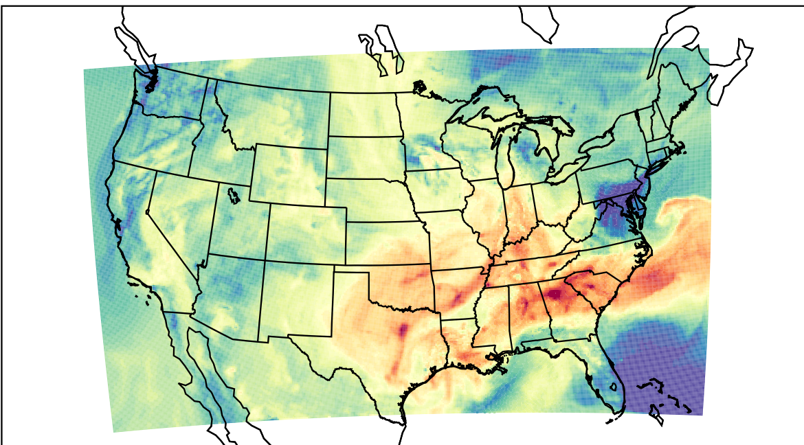
WRF (2023-09-26_18:00:00)
