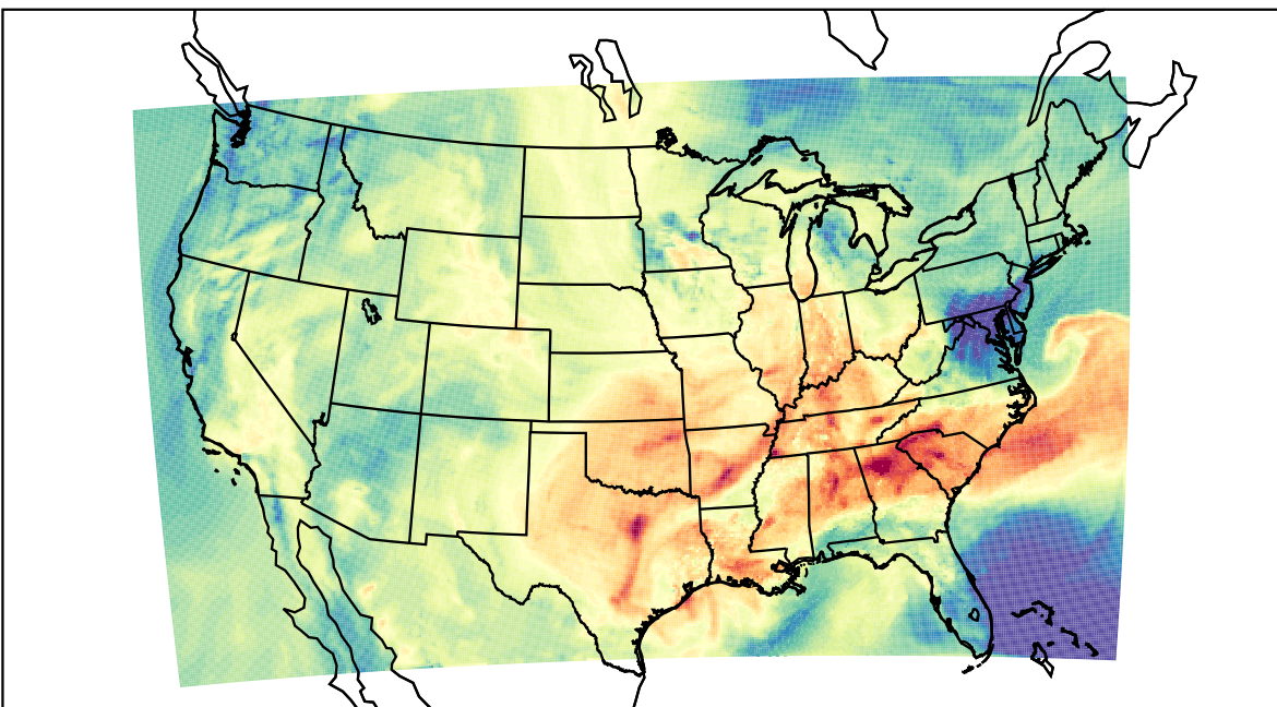
WRF (2023-09-26_19:00:00)
