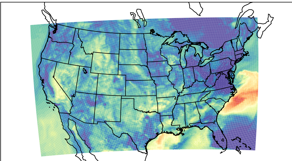
WRF (2023-09-26_13:00:00)
