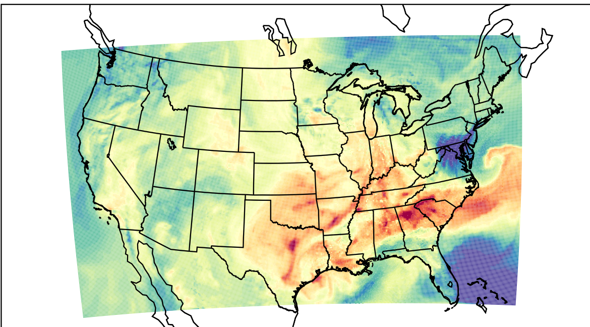
WRF (2023-09-26_20:00:00)
