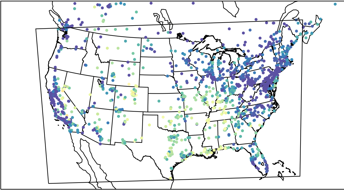
AirNOW (2023-09-26_15:00:00)
