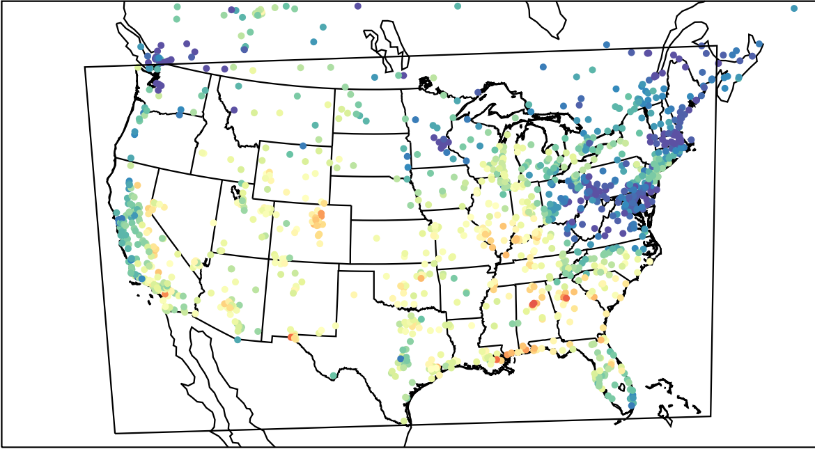
AirNOW (2023-09-25_18:00:00)
