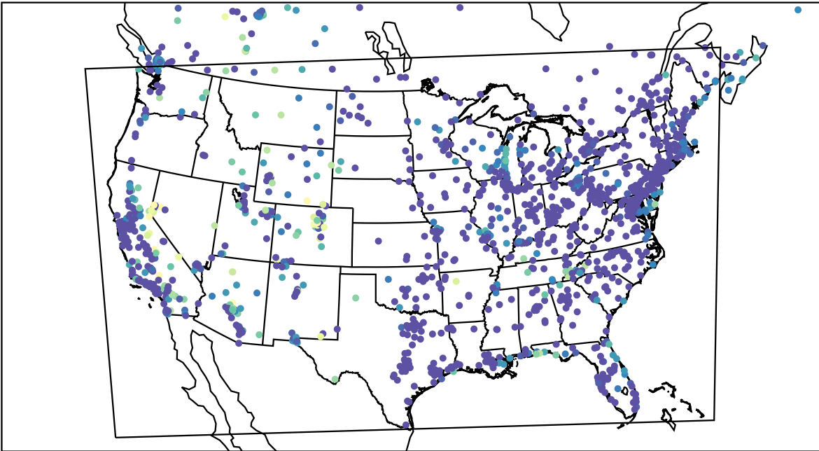
AirNOW (2023-09-26_13:00:00)
