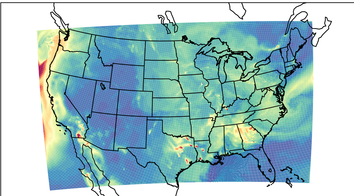
WRF 2023-09-27_08:00:00
