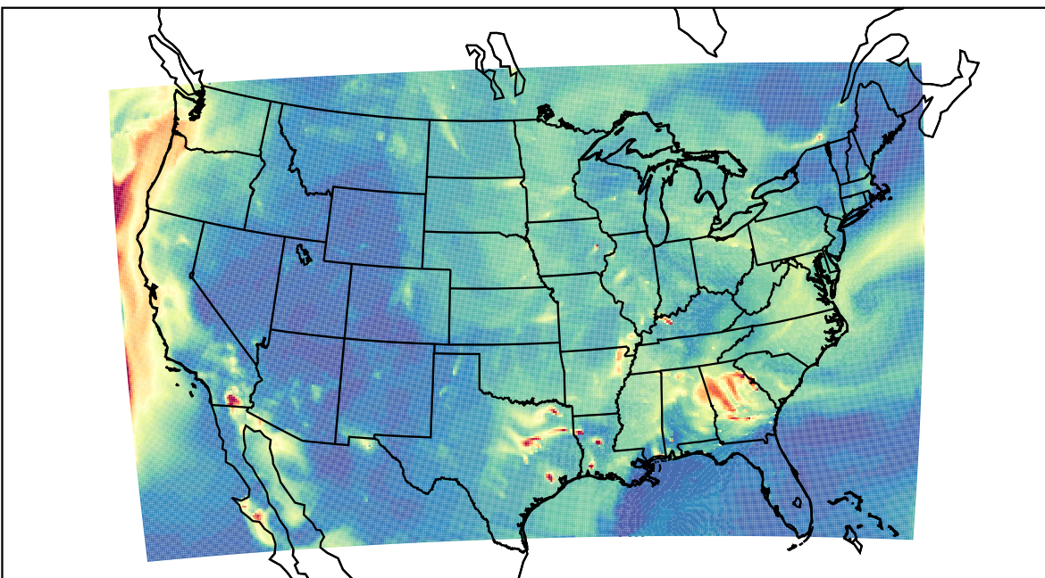
WRF 2023-09-27_06:00:00
