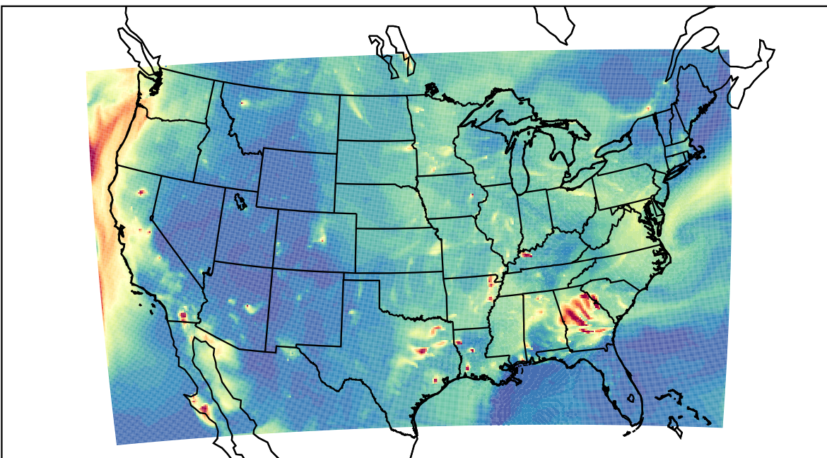
WRF 2023-09-27_04:00:00
