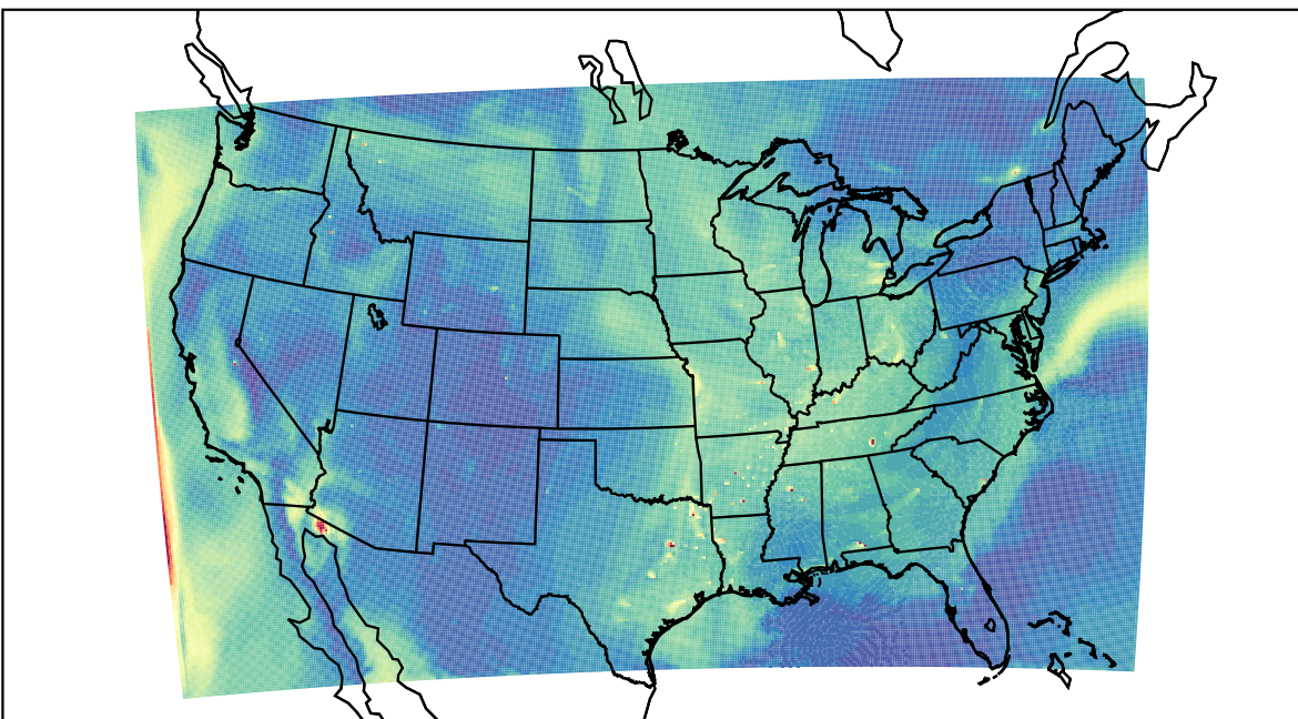
WRF 2023-09-28_19:00:00
