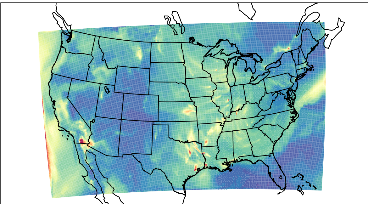
WRF 2023-09-28_08:00:00
