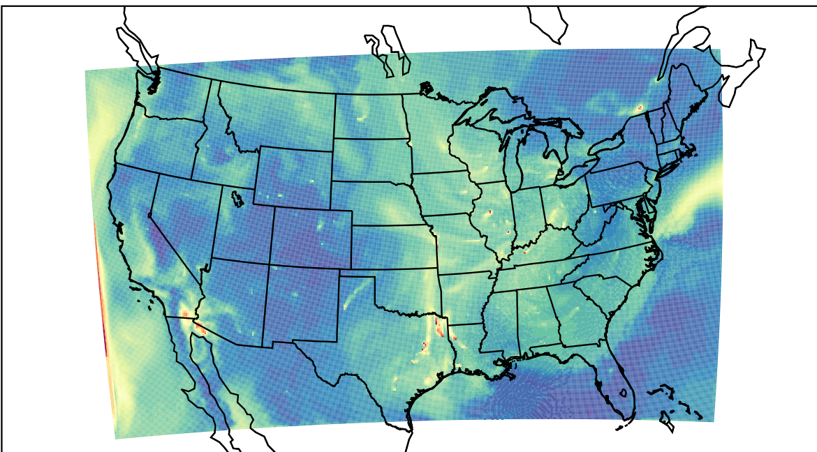
WRF 2023-09-28_16:00:00
