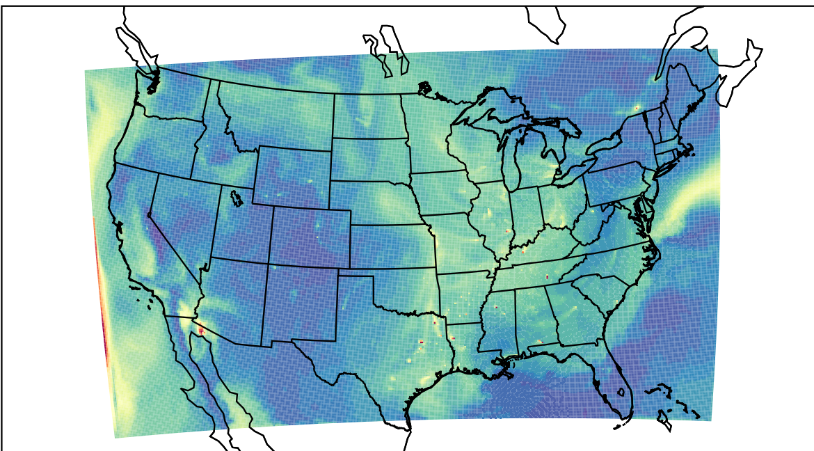
WRF 2023-09-28_18:00:00
