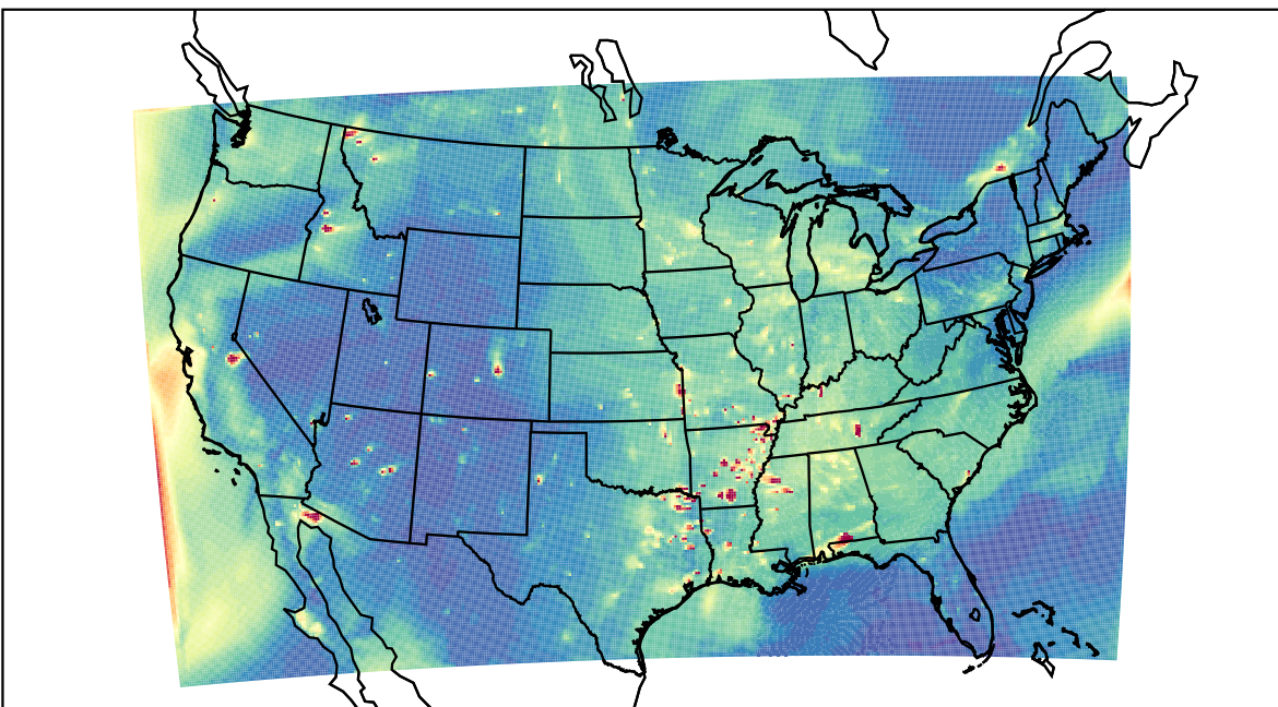
WRF 2023-09-28_01:00:00
