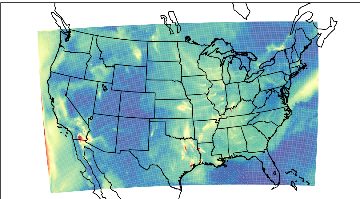
WRF 2023-09-28_09:00:00
