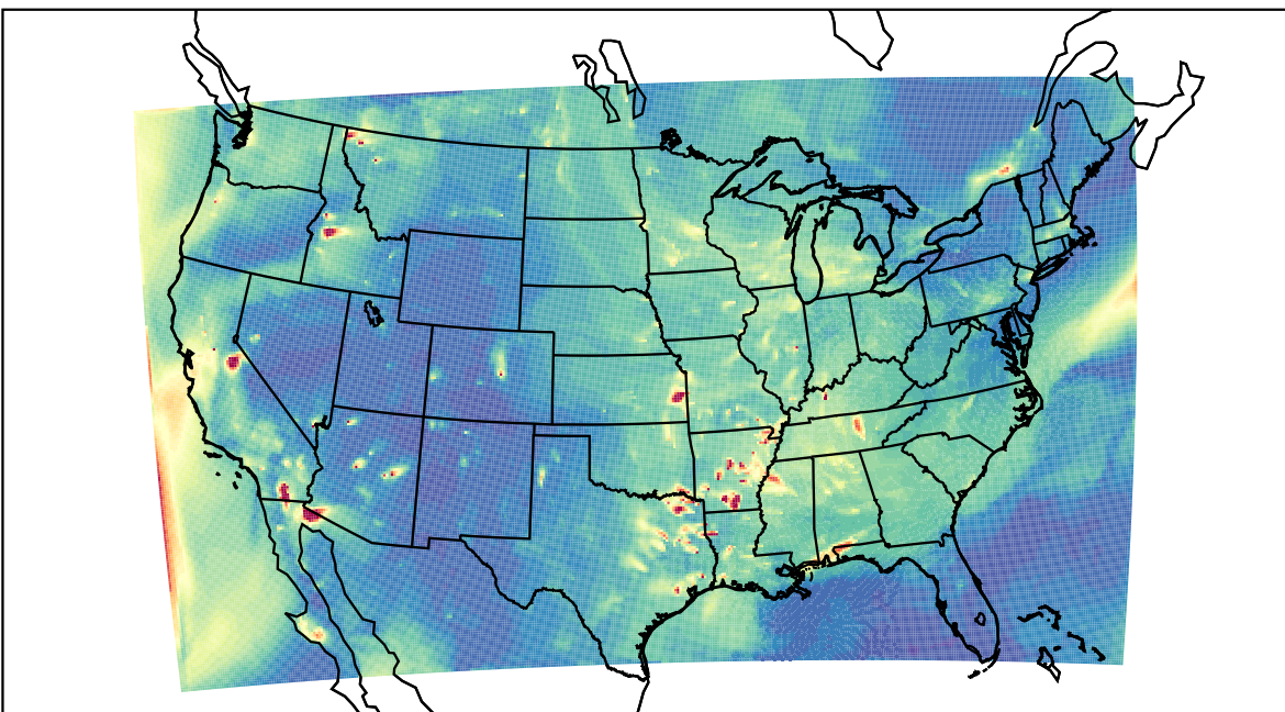
WRF 2023-09-28_03:00:00
