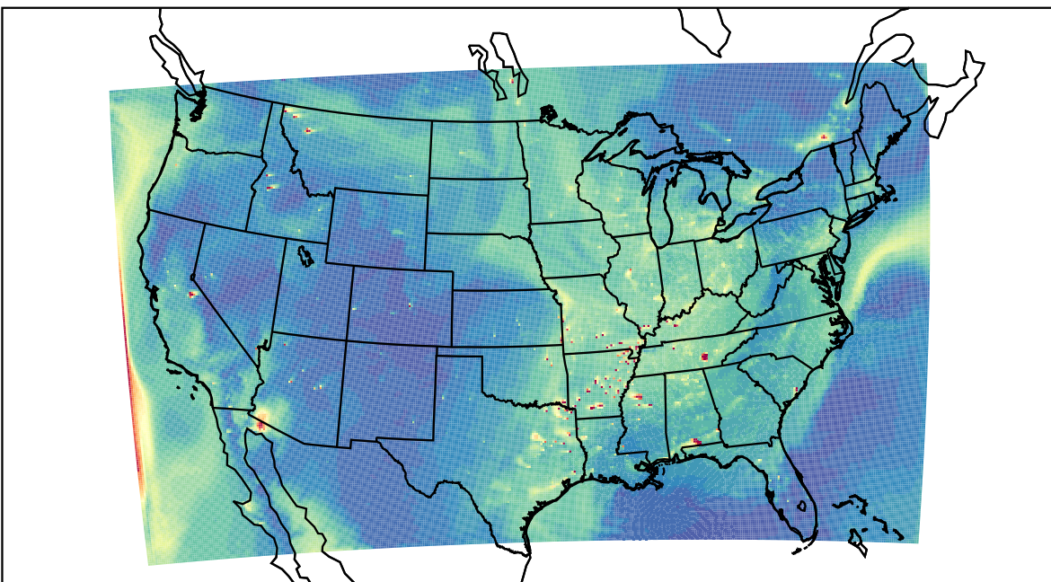
WRF 2023-09-28_23:00:00
