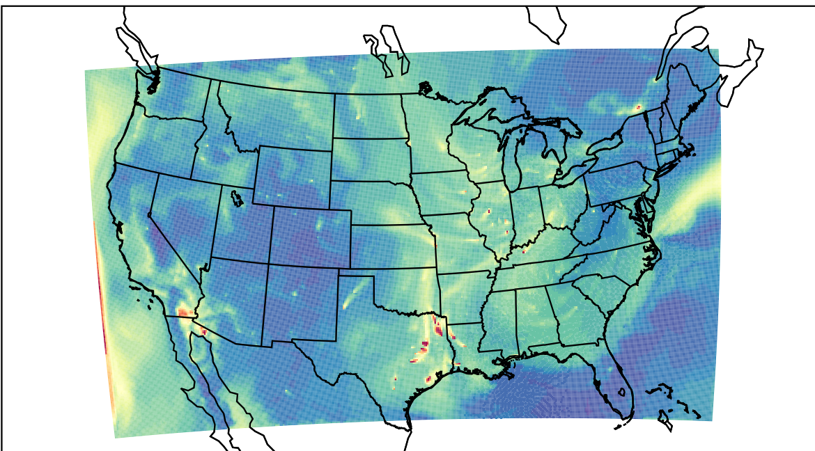
WRF 2023-09-28_15:00:00
