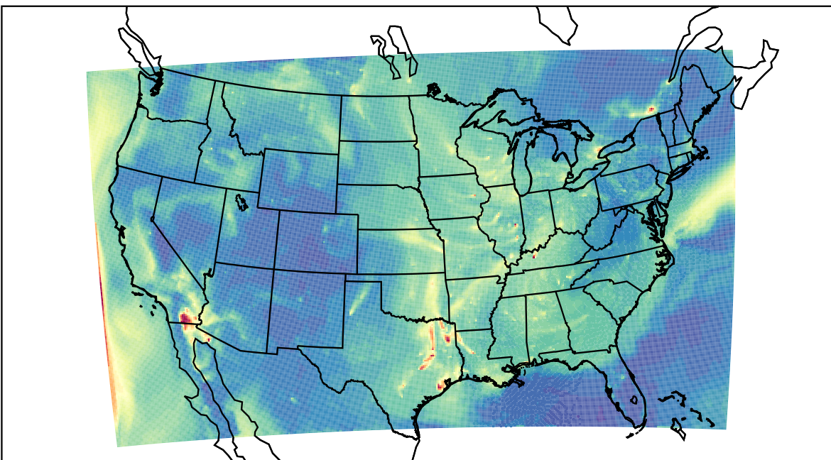
WRF 2023-09-28_13:00:00
