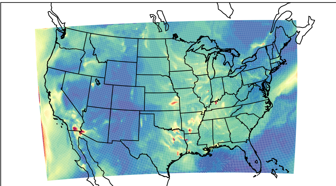
WRF 2023-09-28_06:00:00
