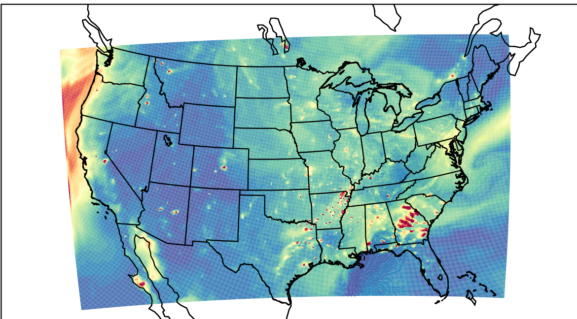
WRF 2023-09-27_01:00:00
