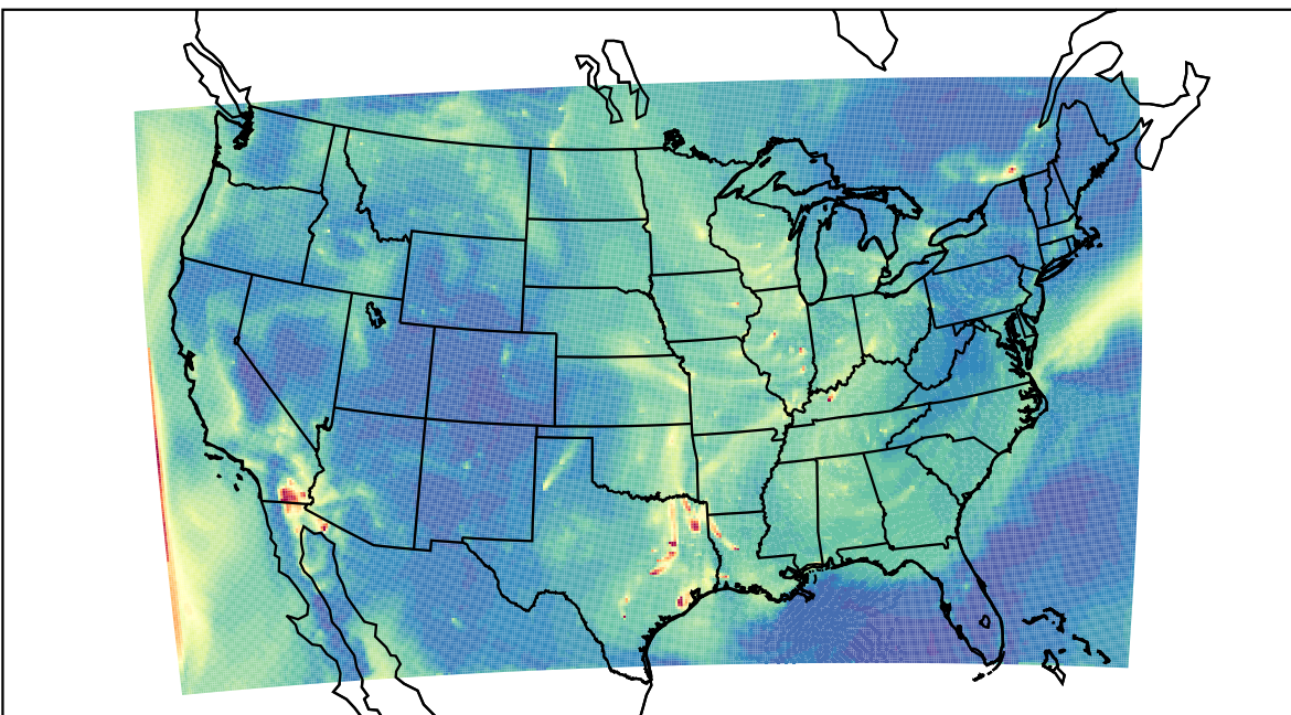
WRF 2023-09-28_14:00:00
