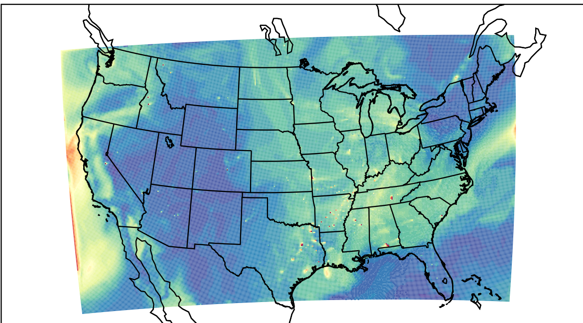
WRF 2023-09-27_20:00:00
