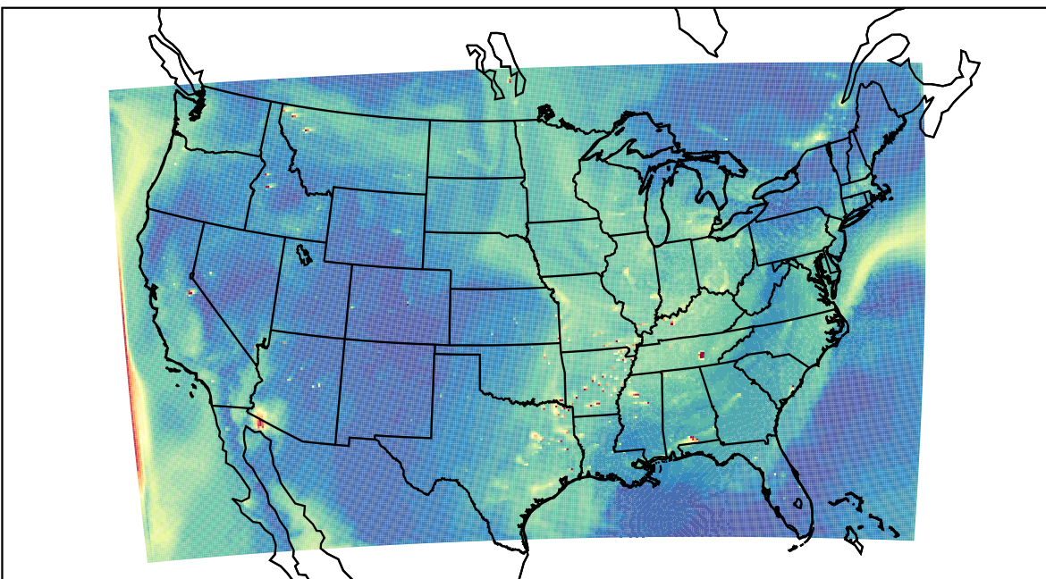
WRF 2023-09-28_22:00:00
