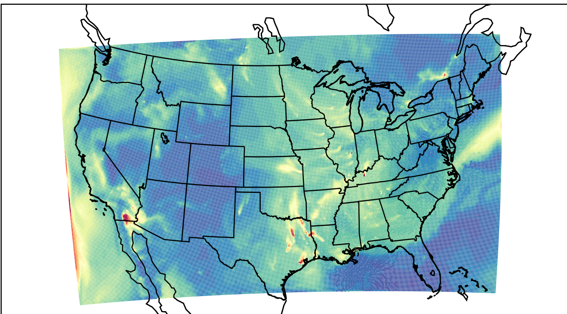
WRF 2023-09-28_10:00:00
