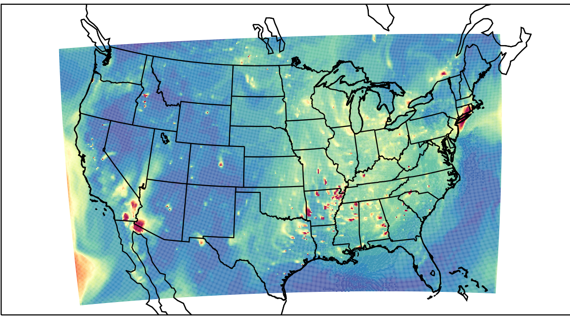
WRF 2023-09-30_01:00:00
