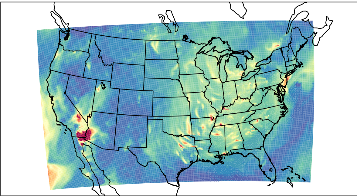
WRF 2023-09-30_06:00:00
