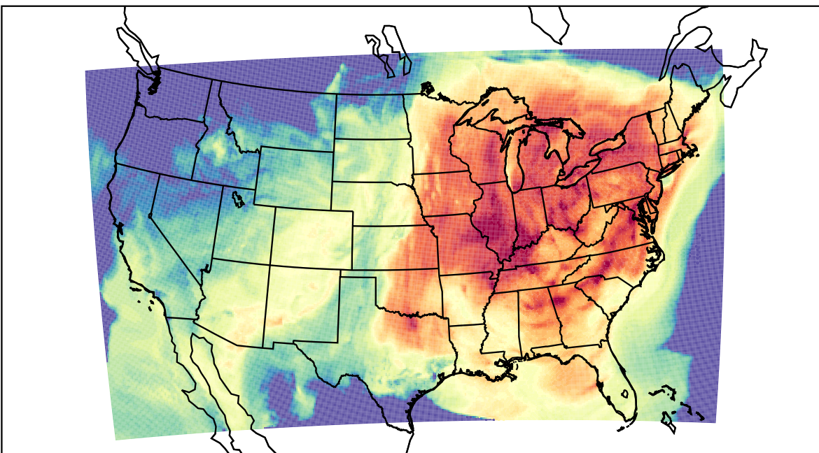
WRF (2023-10-03_18:00:00)
