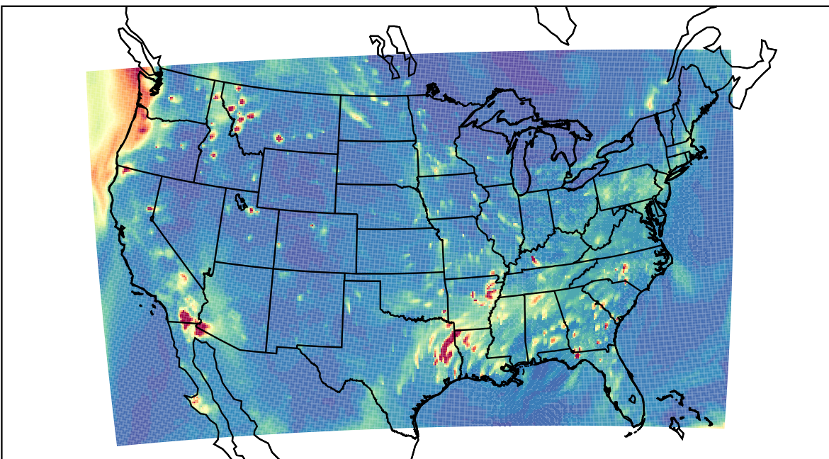
WRF 2023-10-10_03:00:00
