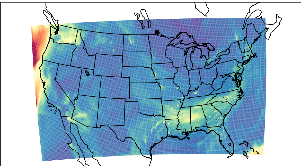
WRF 2023-10-10_18:00:00
