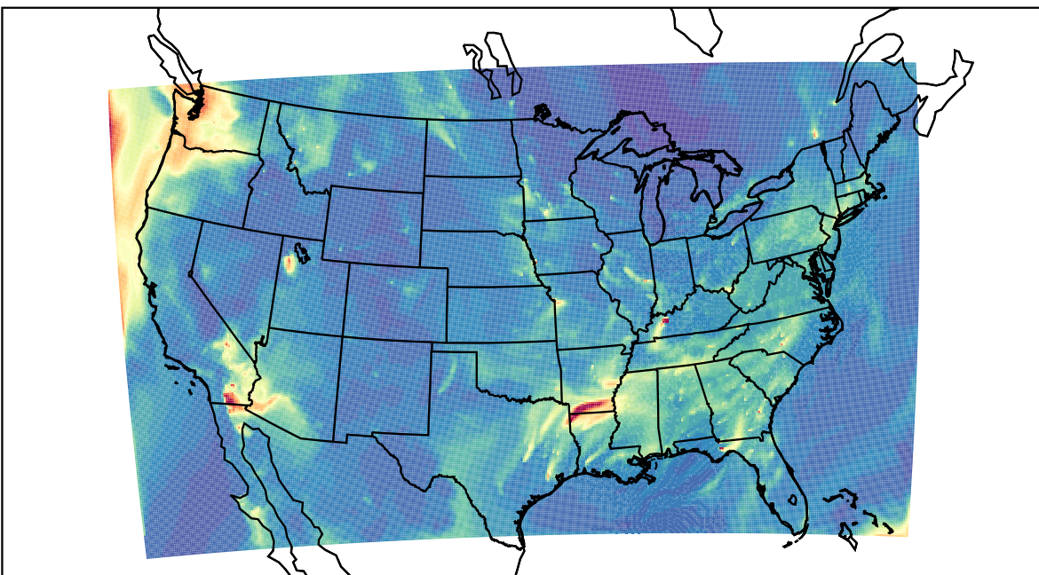
WRF 2023-10-10_10:00:00
