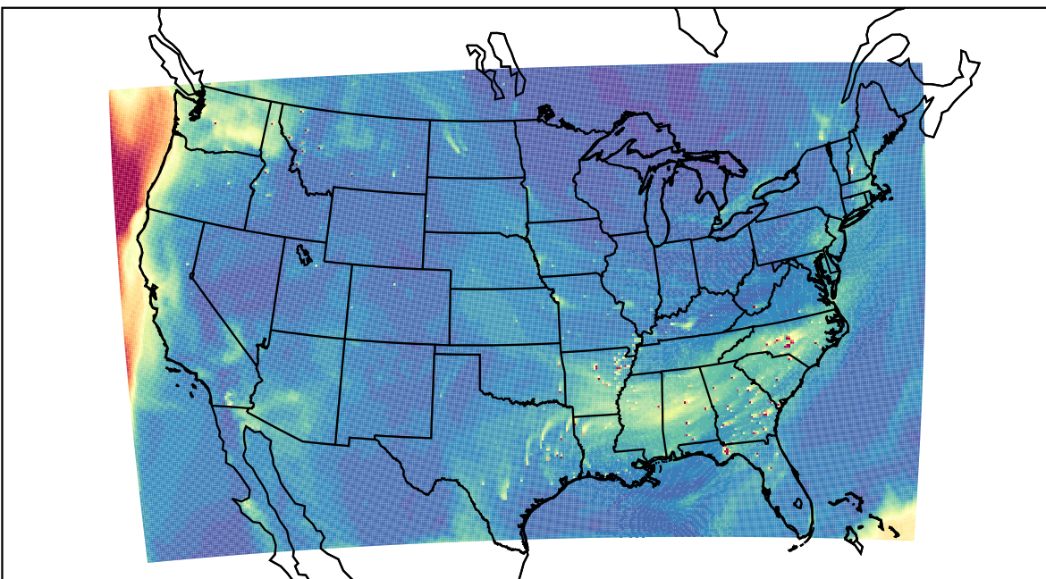
WRF 2023-10-10_20:00:00
