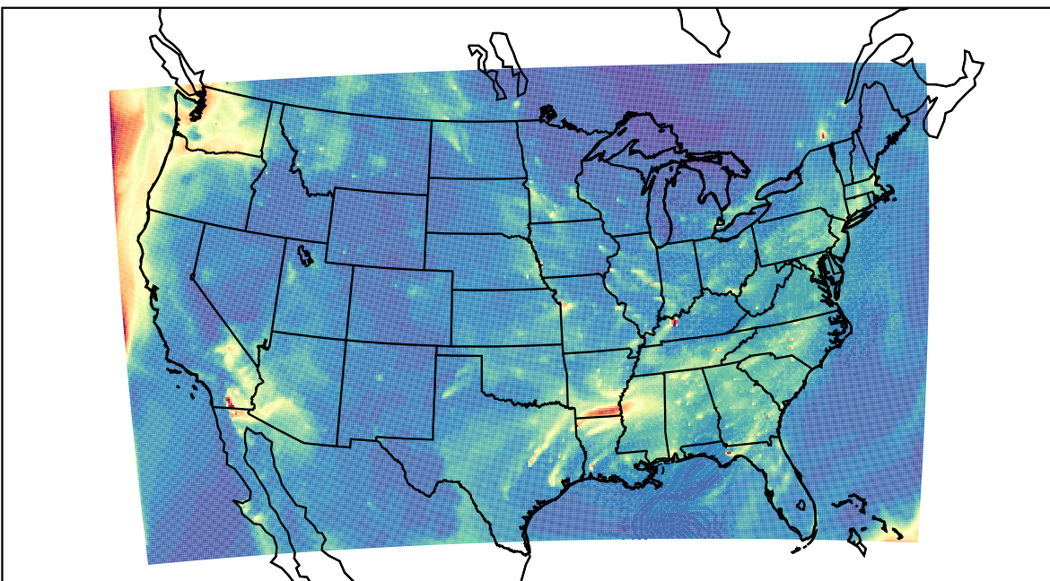
WRF 2023-10-10_13:00:00
