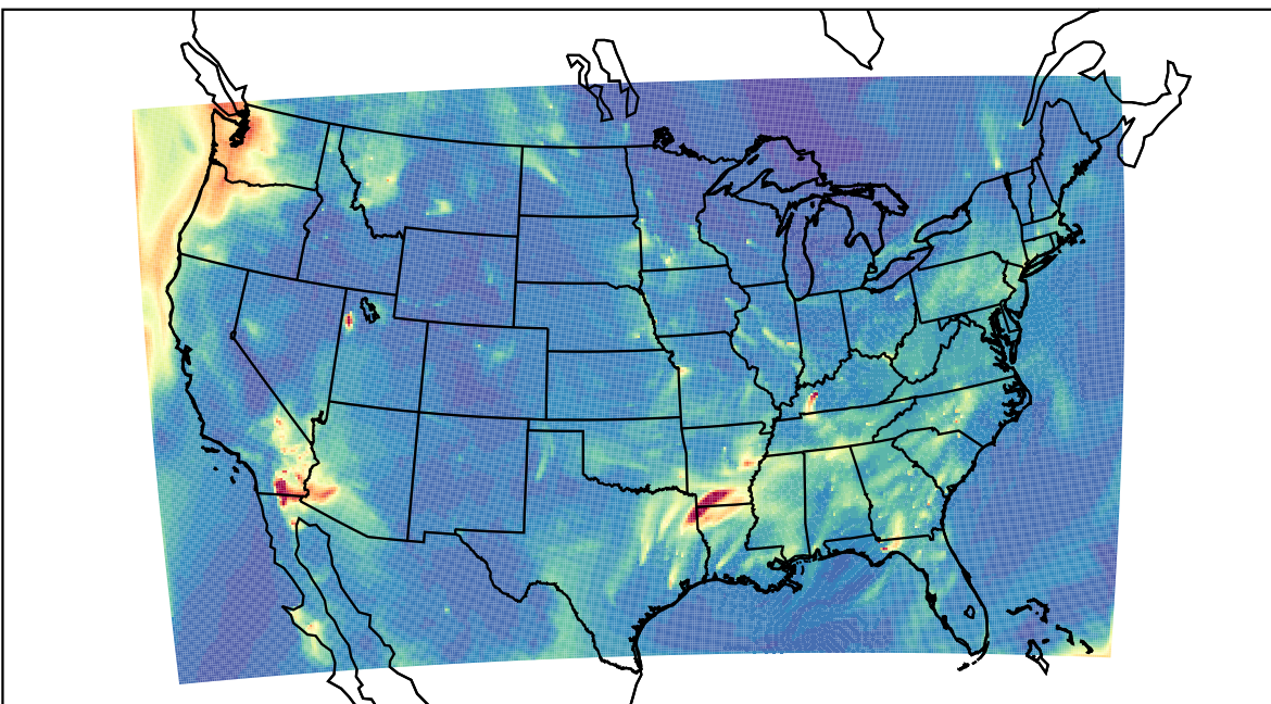
WRF 2023-10-10_08:00:00
