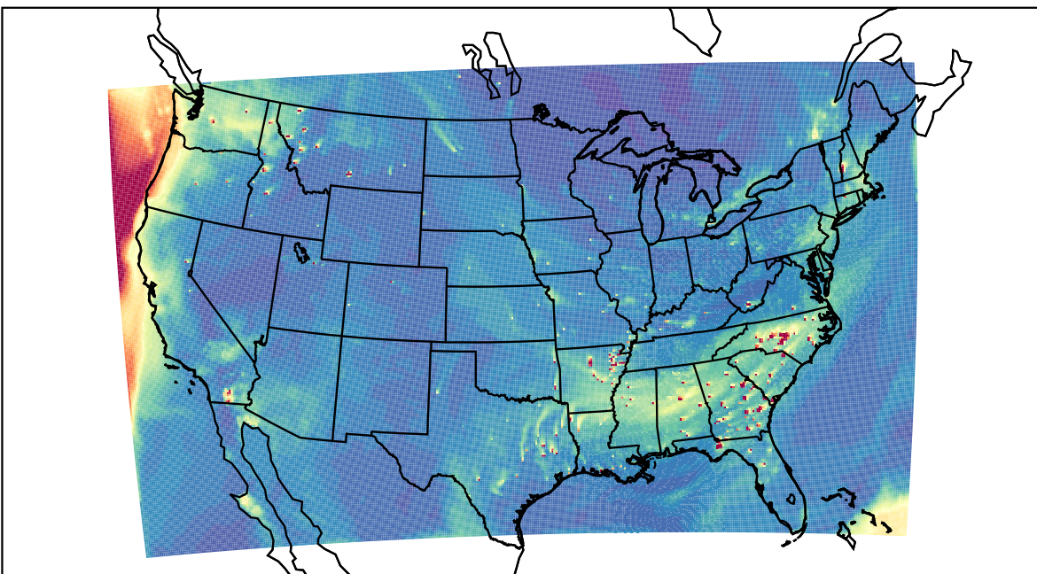
WRF 2023-10-10_22:00:00
