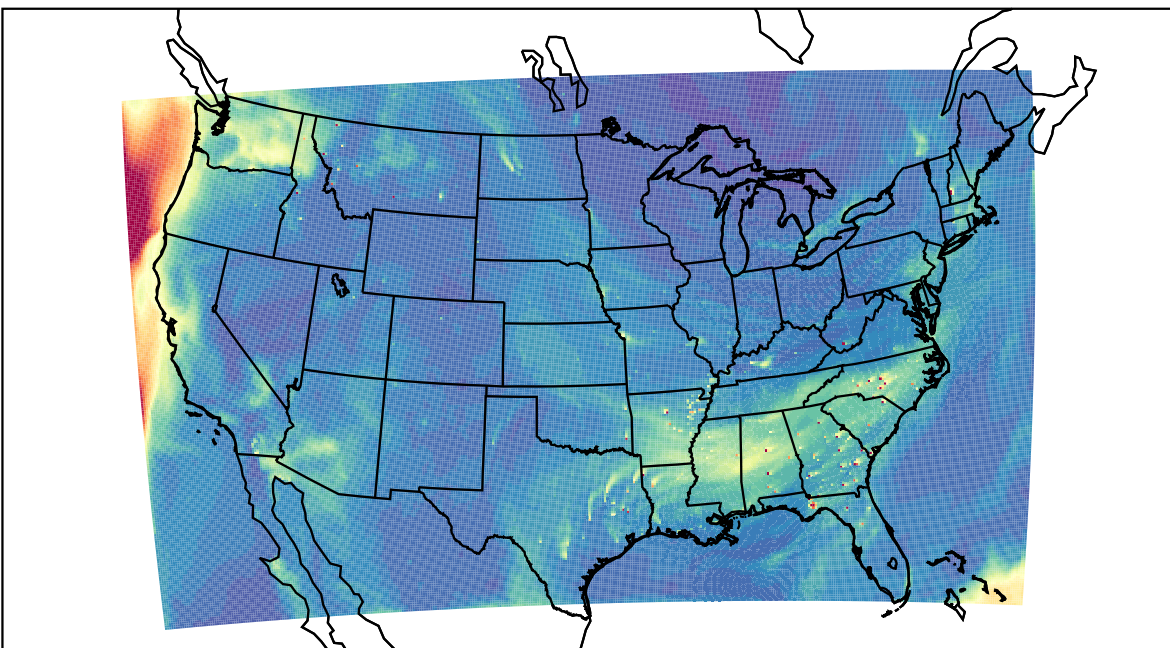
WRF 2023-10-10_19:00:00
