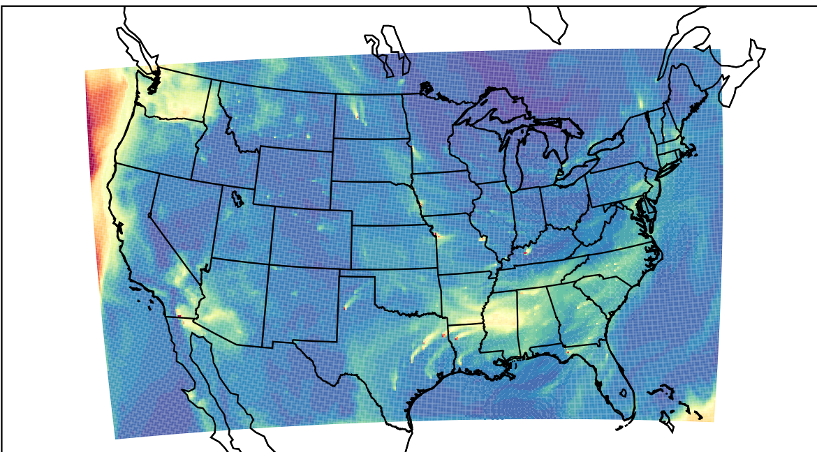
WRF 2023-10-10_16:00:00
