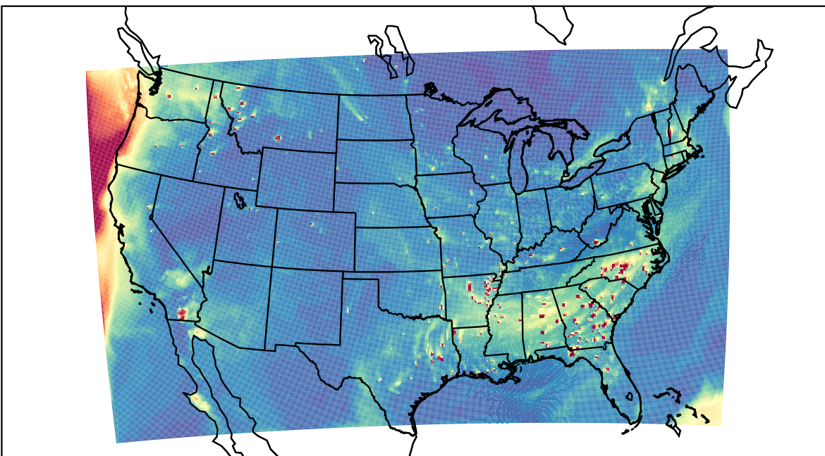
WRF 2023-10-10_23:00:00
