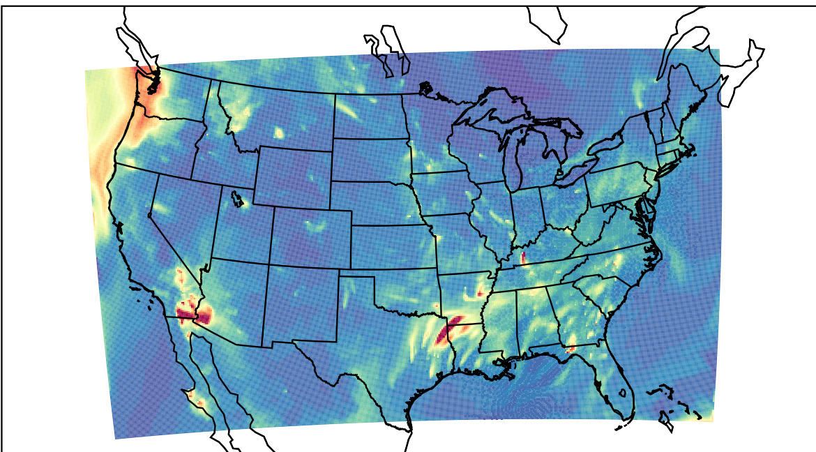
WRF 2023-10-10_06:00:00
