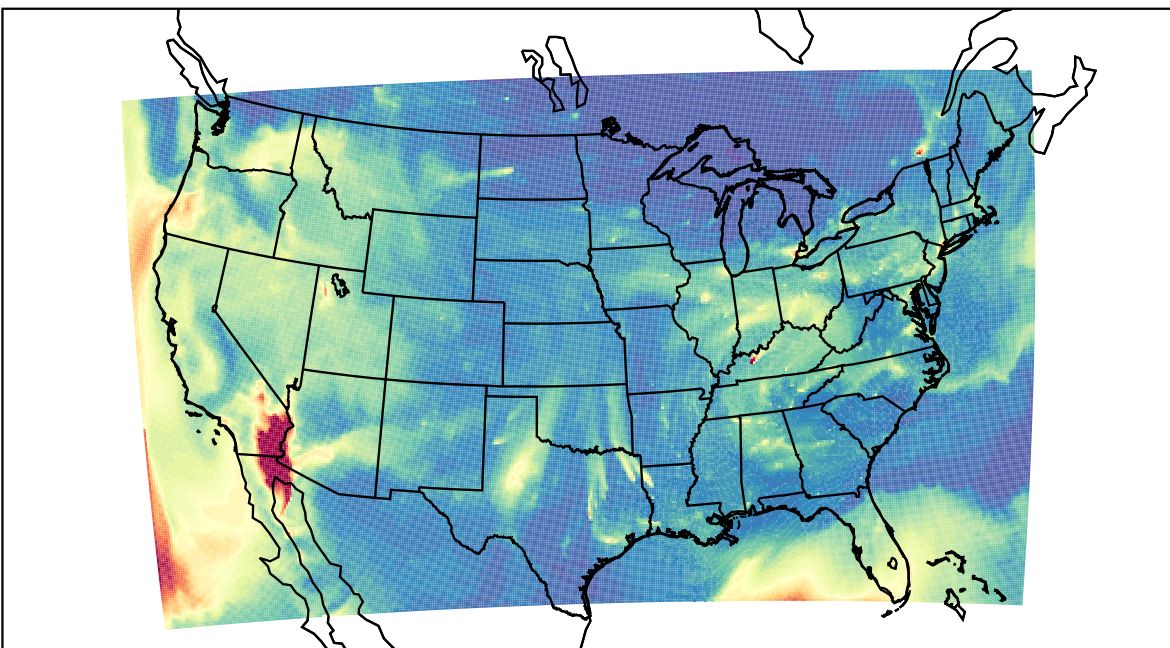
WRF 2023-10-12_13:00:00
