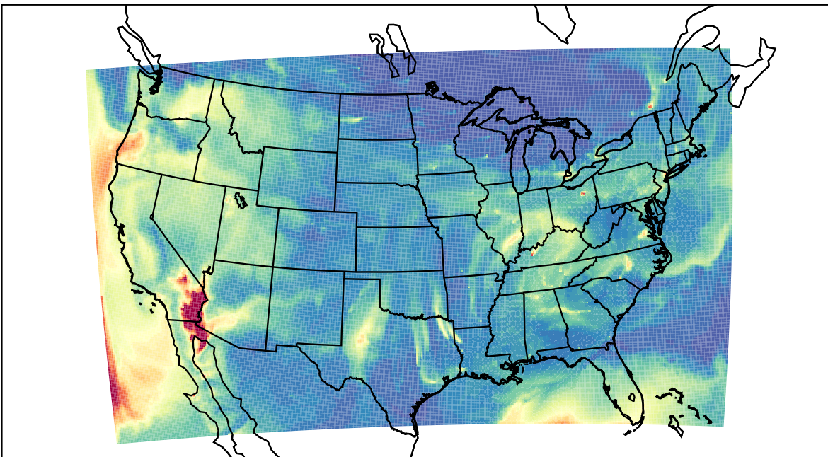
WRF 2023-10-12_10:00:00
