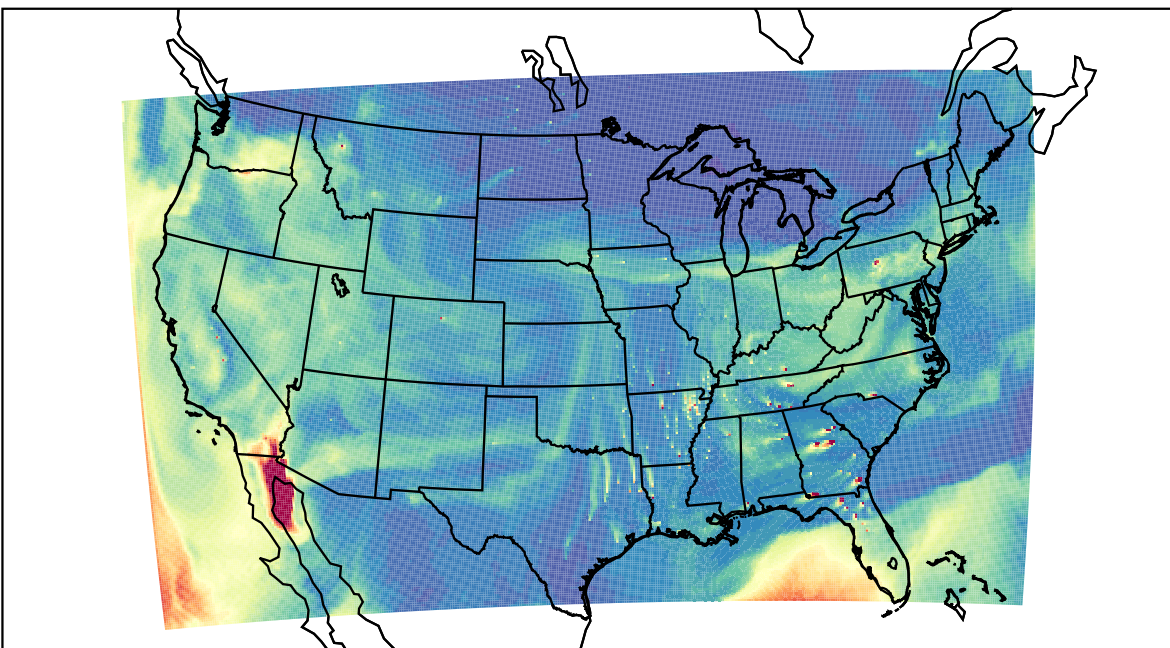
WRF 2023-10-12_20:00:00
