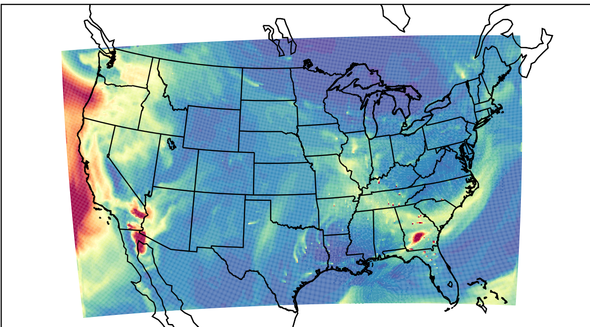
WRF 2023-10-11_18:00:00
