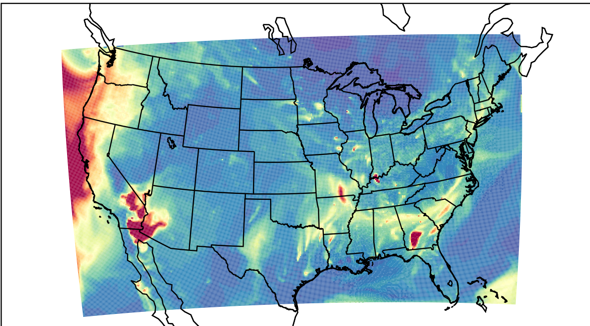
WRF 2023-10-11_10:00:00
