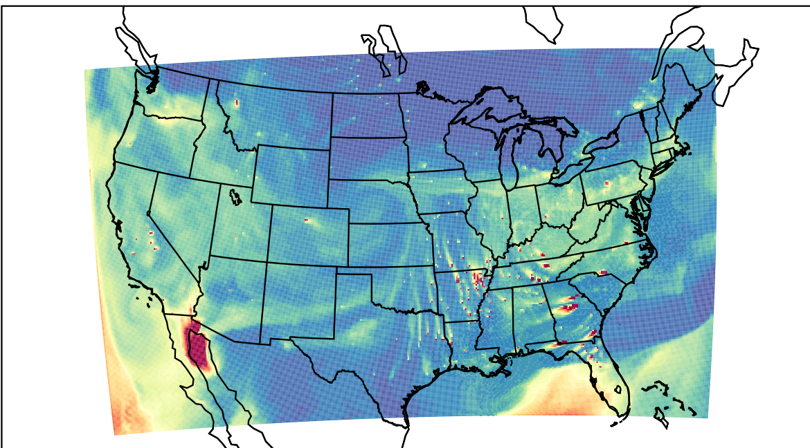
WRF 2023-10-12_23:00:00
