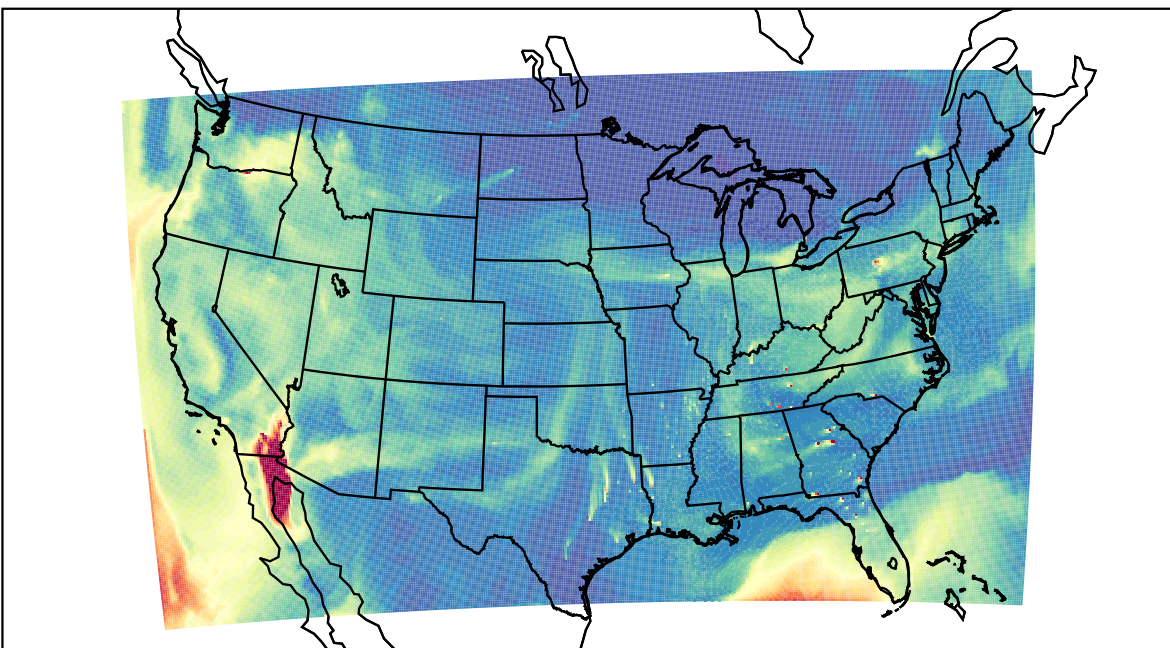
WRF 2023-10-12_18:00:00
