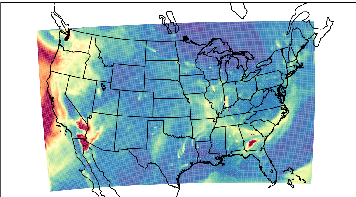
WRF 2023-10-11_16:00:00
