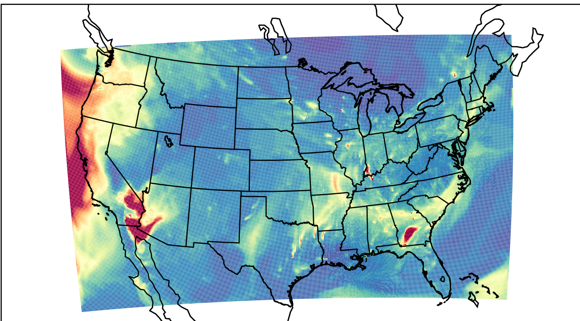
WRF 2023-10-11_13:00:00
