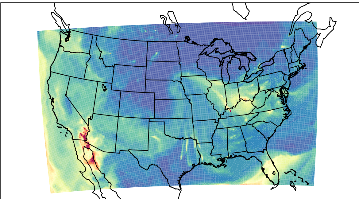
WRF 2023-10-13_10:00:00
