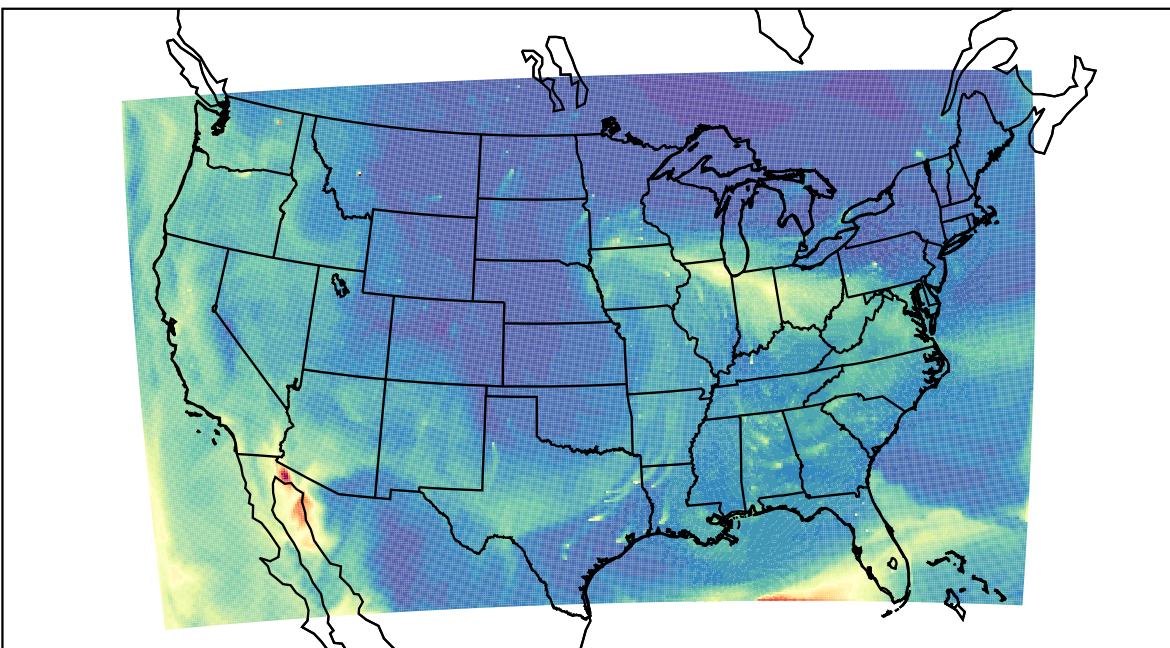
WRF 2023-10-13_20:00:00
