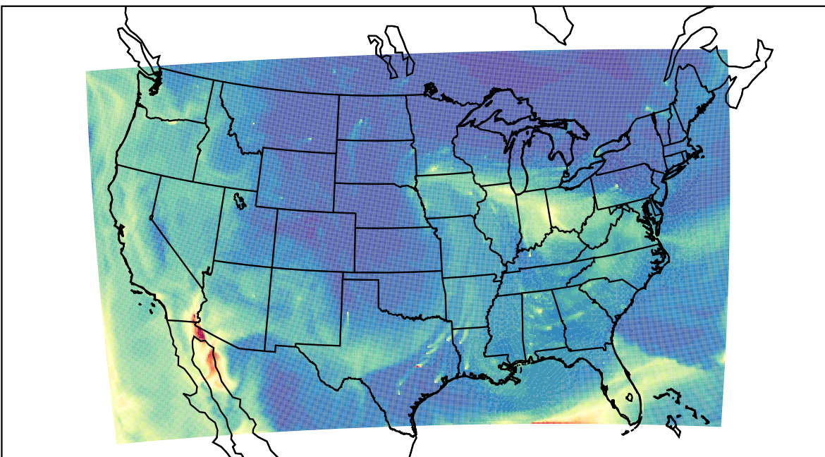
WRF 2023-10-13_18:00:00
