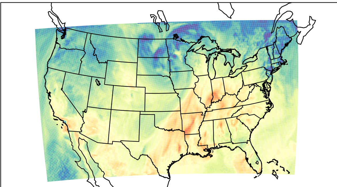
WRF (2023-10-18_20:00:00)
