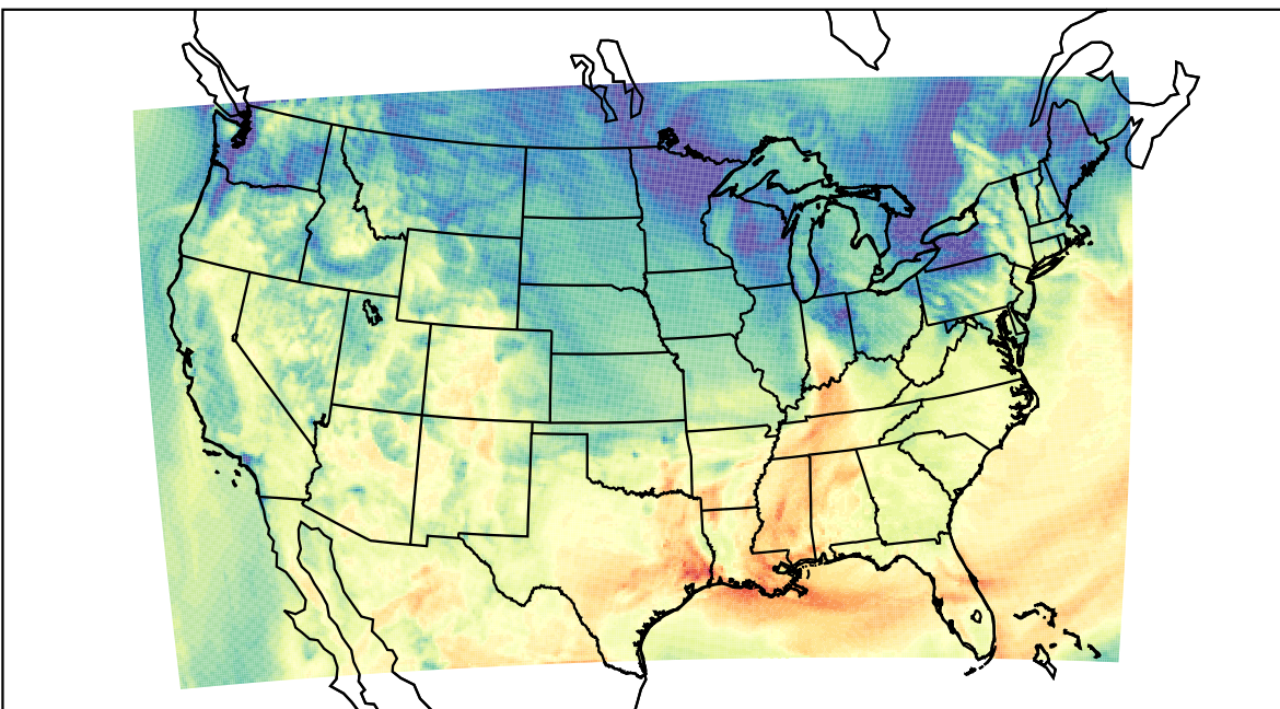
WRF (2023-10-21_18:00:00)
