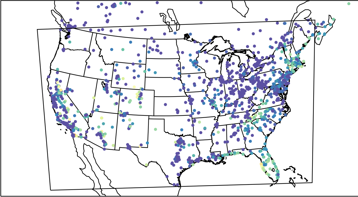
AirNOW (2023-10-21_13:00:00)
