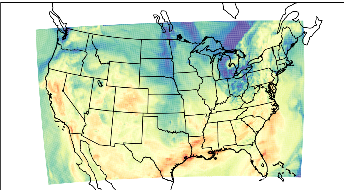
WRF (2023-10-20_20:00:00)
