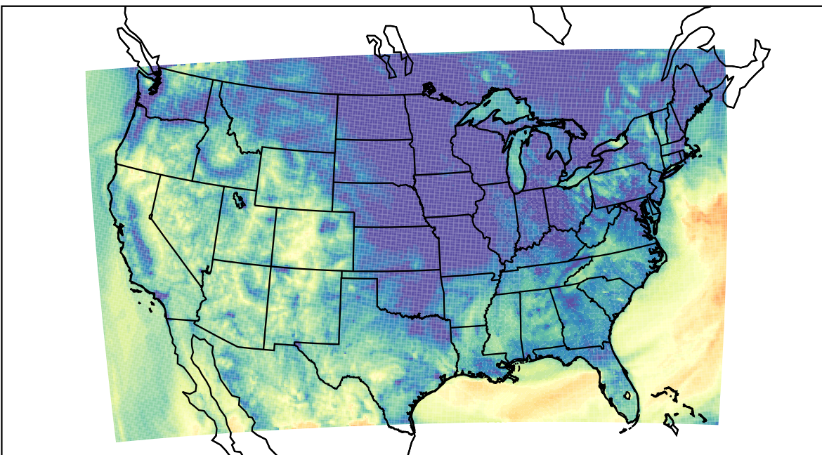
WRF (2023-10-21_13:00:00)
