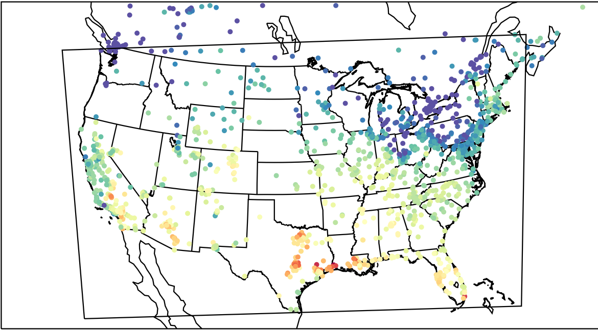
AirNOW (2023-10-21_18:00:00)
