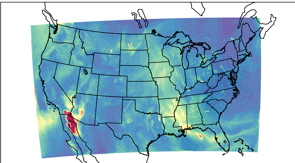
WRF 2023-10-23_18:00:00
