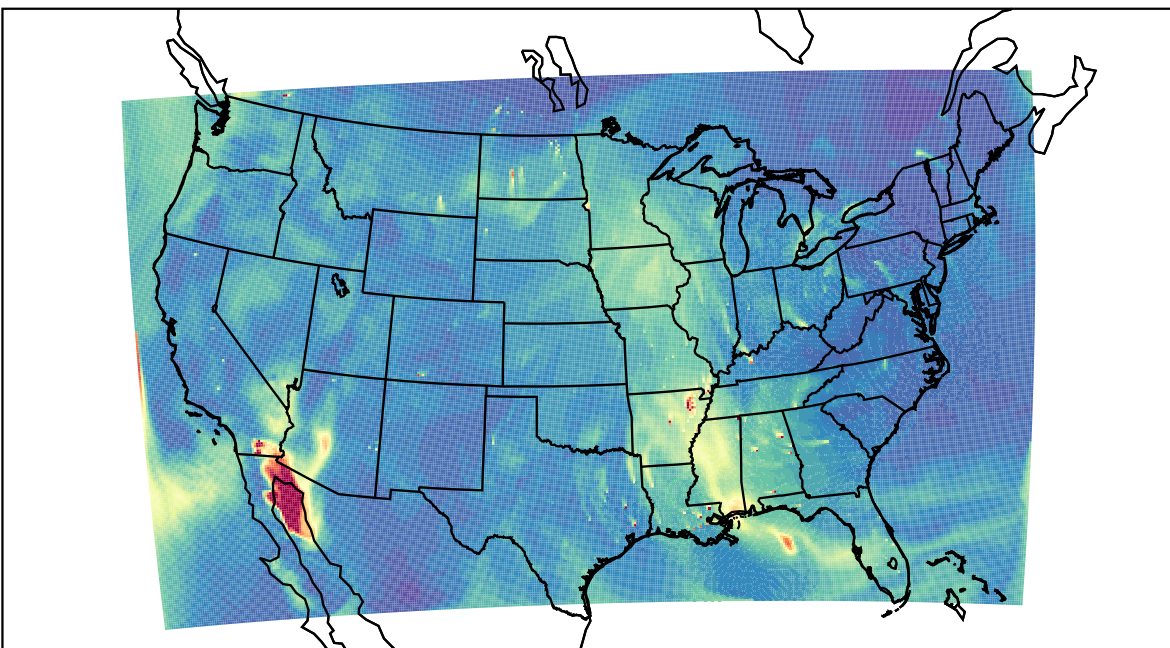
WRF 2023-10-23_20:00:00
