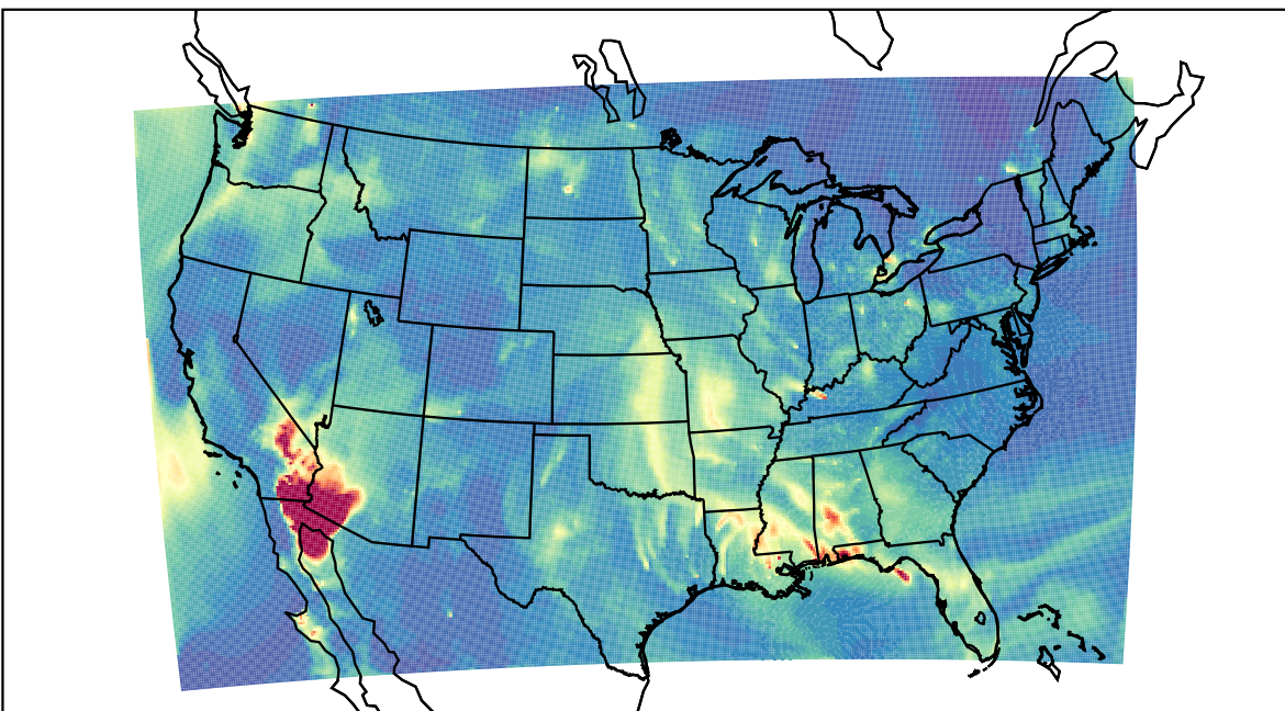
WRF 2023-10-23_10:00:00
