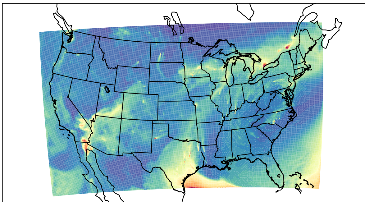
WRF 2023-10-26_16:00:00
