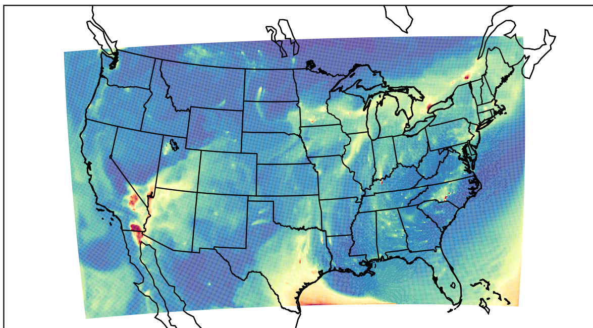
WRF 2023-10-26_13:00:00
