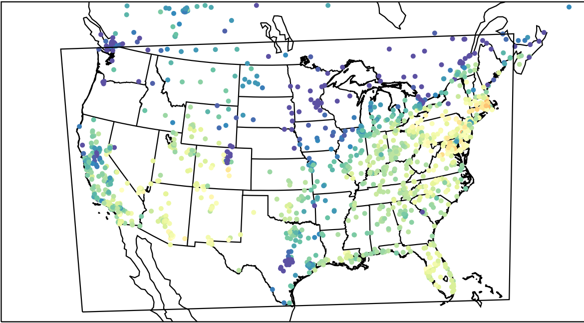
AirNOW (2023-10-26_18:00:00)
