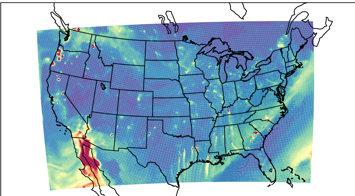
WRF 2023-10-31_01:00:00
