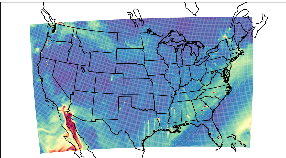
WRF 2023-10-30_22:00:00
