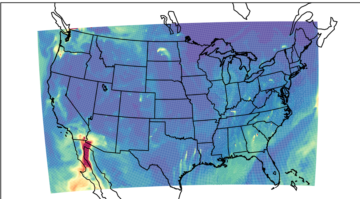
WRF 2023-10-31_18:00:00
