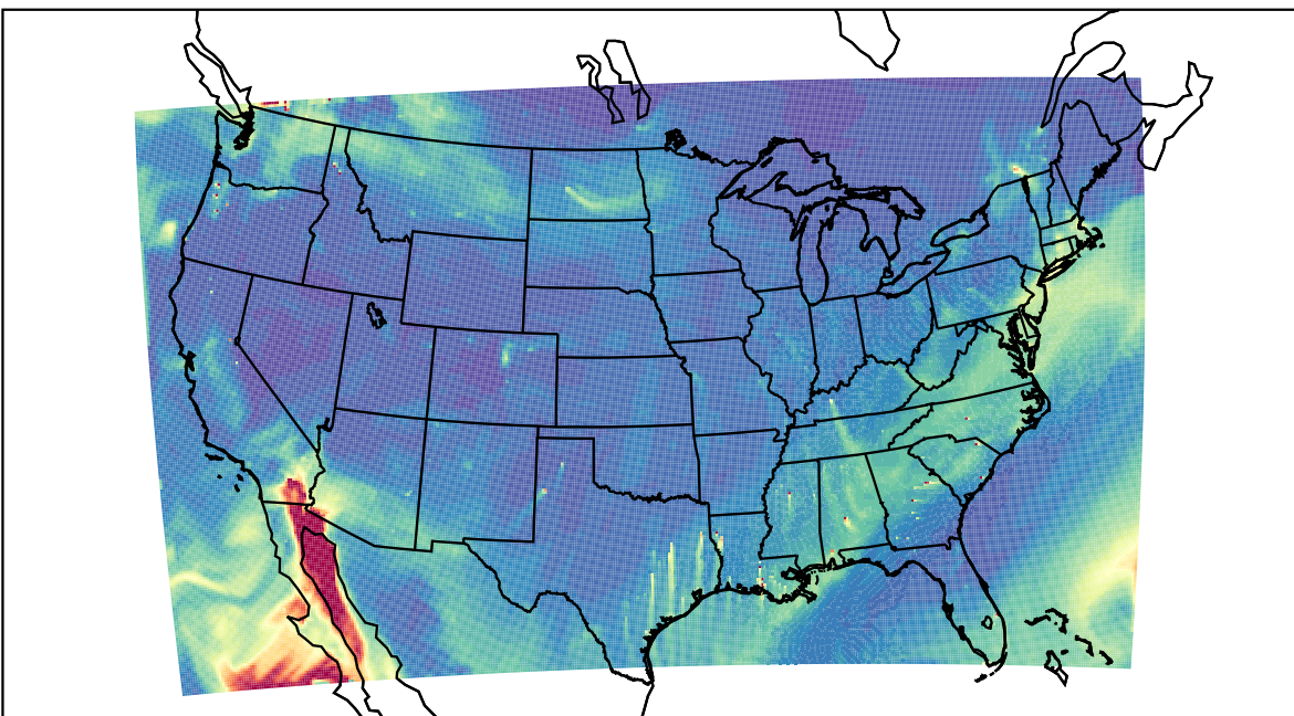
WRF 2023-10-30_20:00:00
