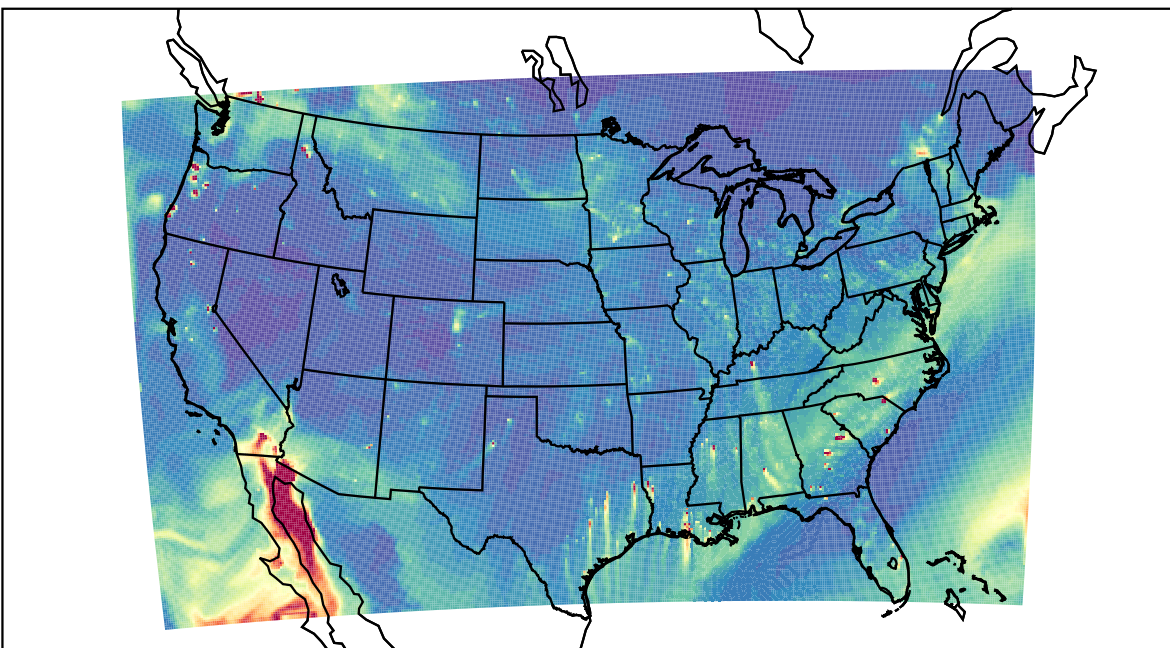
WRF 2023-10-30_23:00:00
