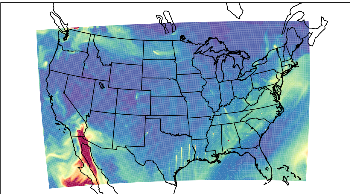
WRF 2023-10-30_18:00:00
