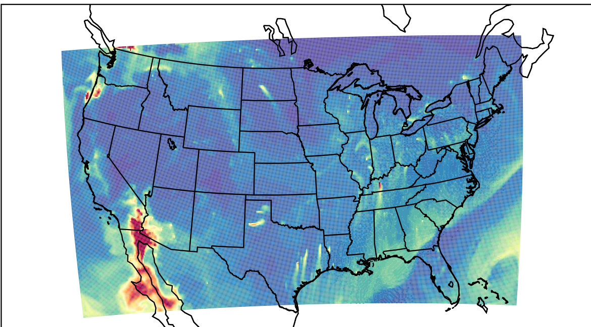
WRF 2023-10-31_10:00:00
