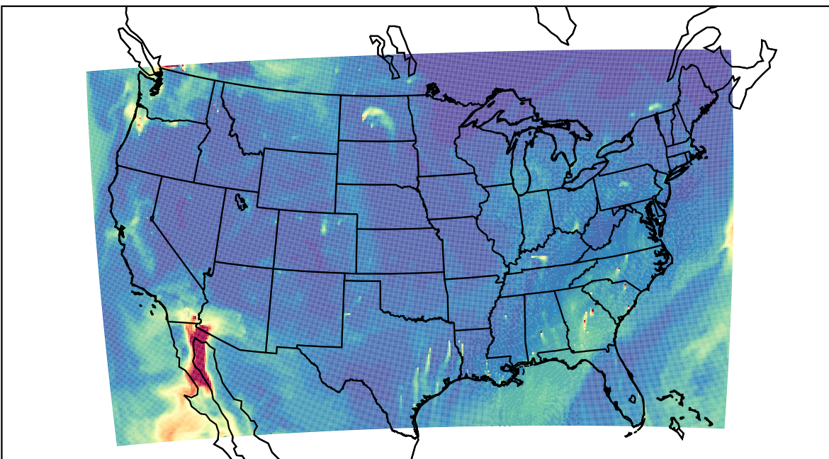
WRF 2023-10-31_19:00:00
