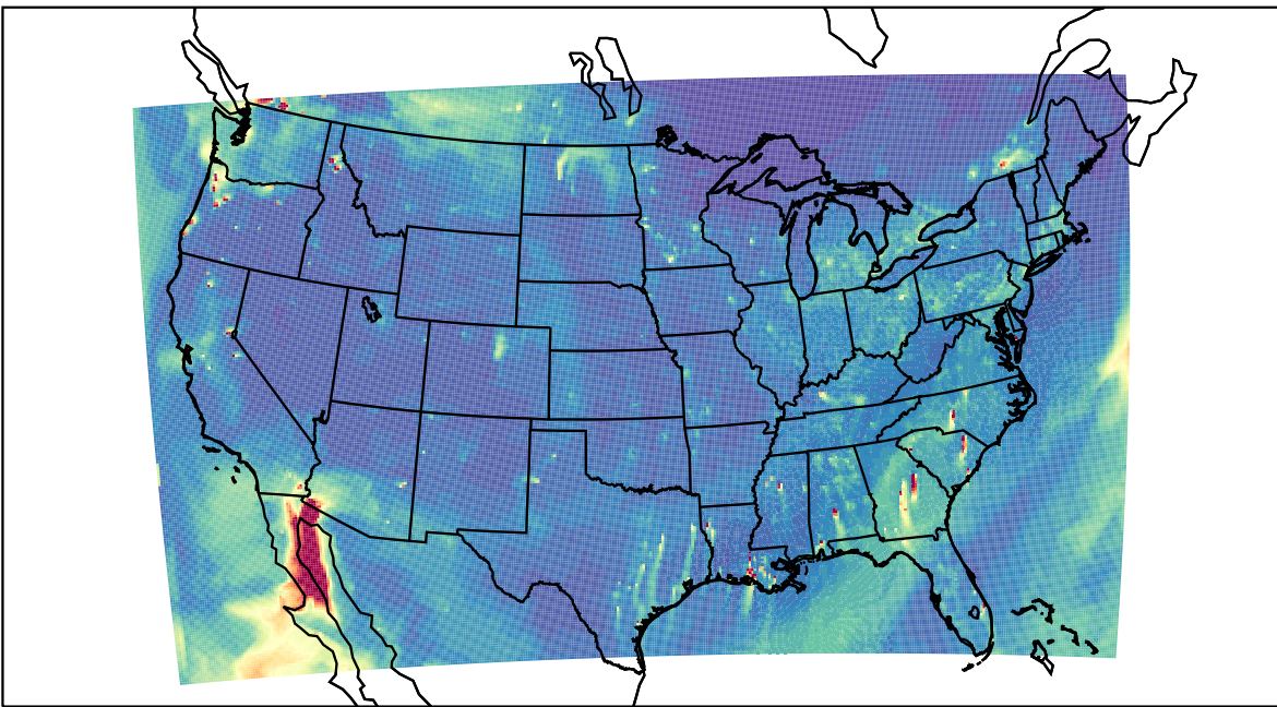
WRF 2023-10-31_23:00:00
