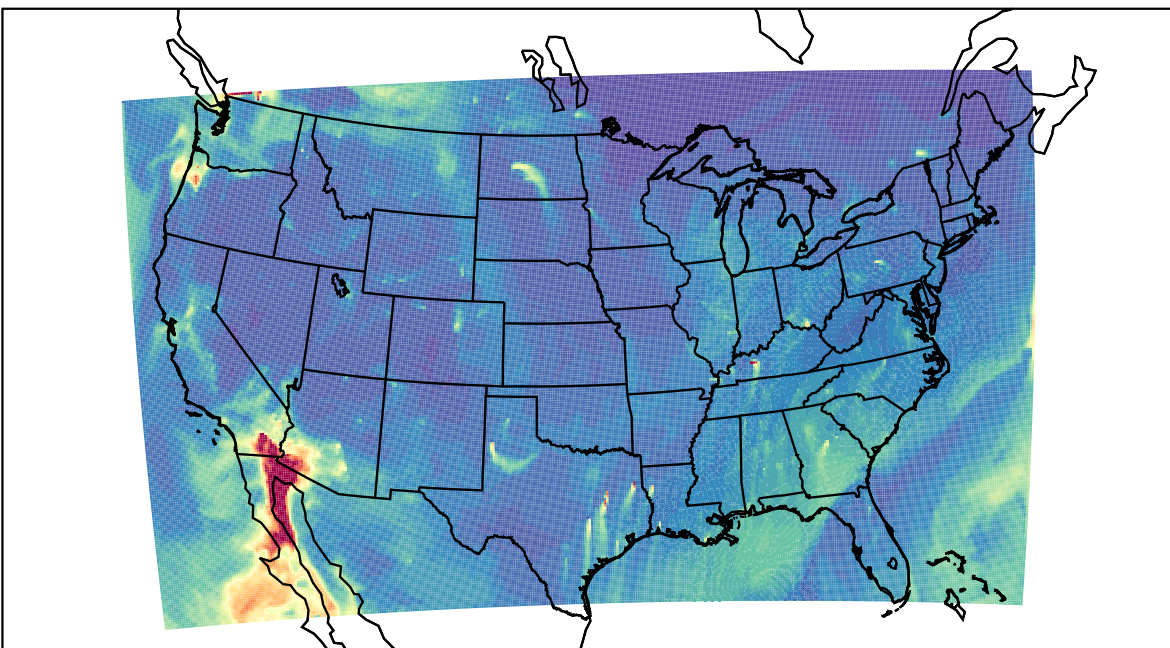
WRF 2023-10-31_16:00:00
