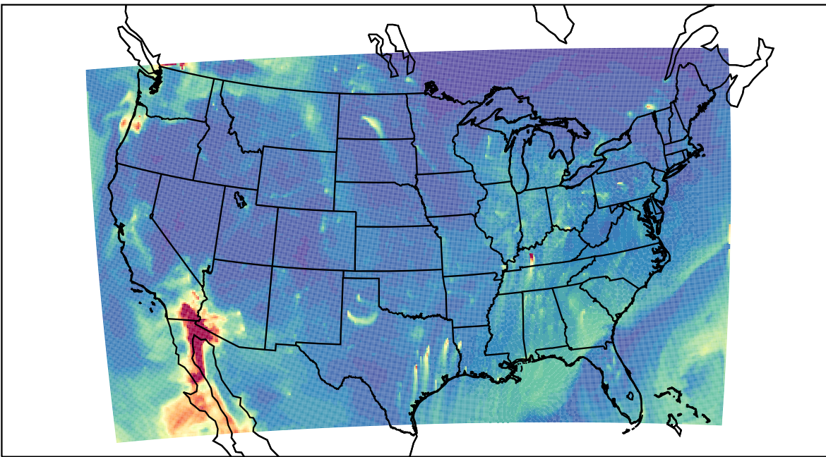
WRF 2023-10-31_14:00:00
