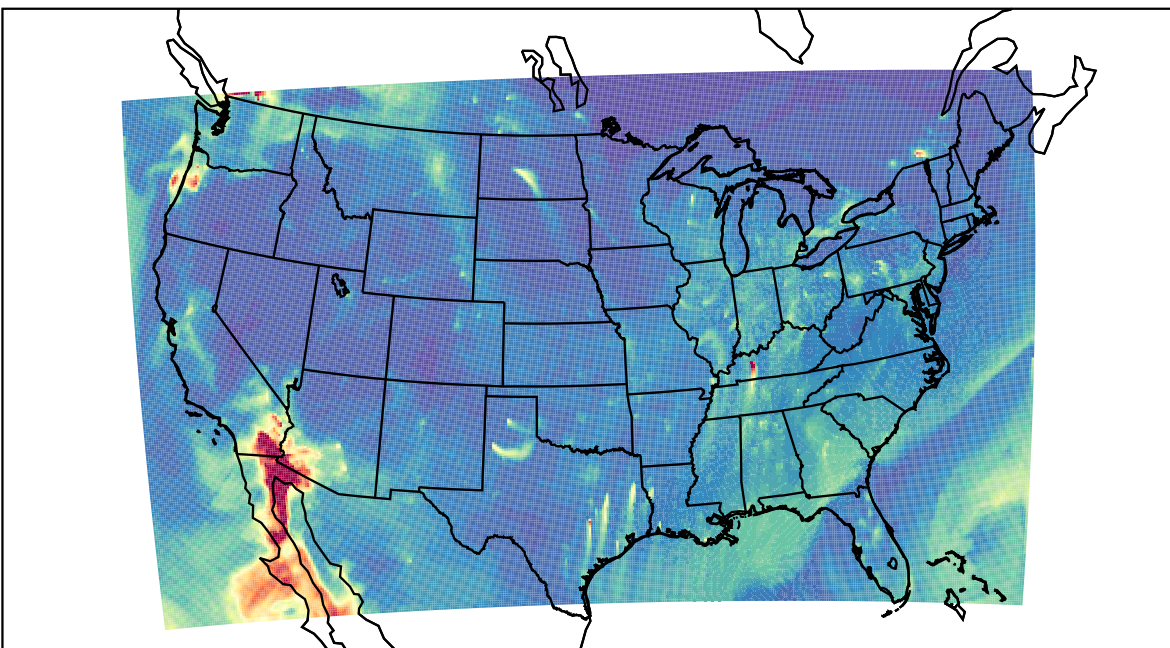
WRF 2023-10-31_13:00:00
