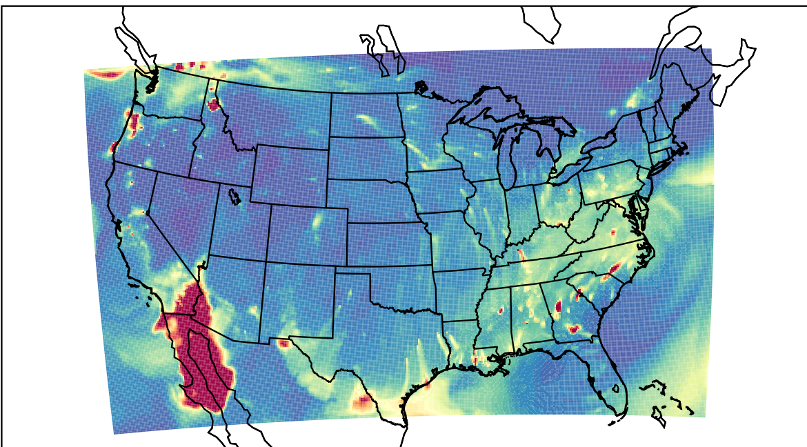
WRF 2023-10-30_03:00:00
