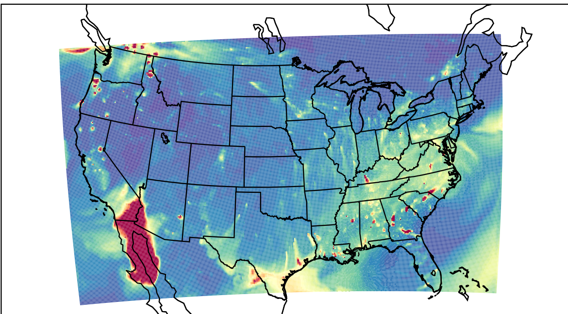
WRF 2023-10-30_01:00:00
