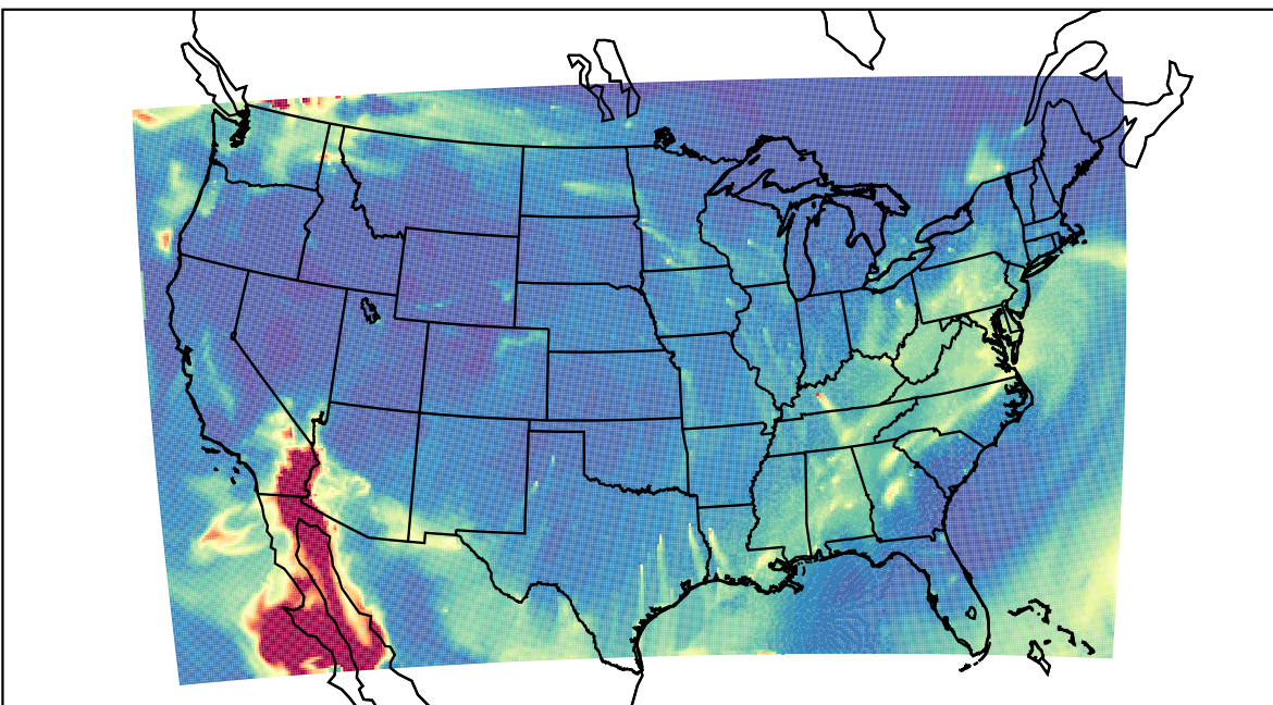
WRF 2023-10-30_10:00:00
