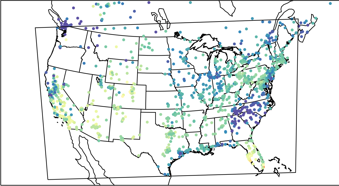
AirNOW (2023-10-31_18:00:00)
