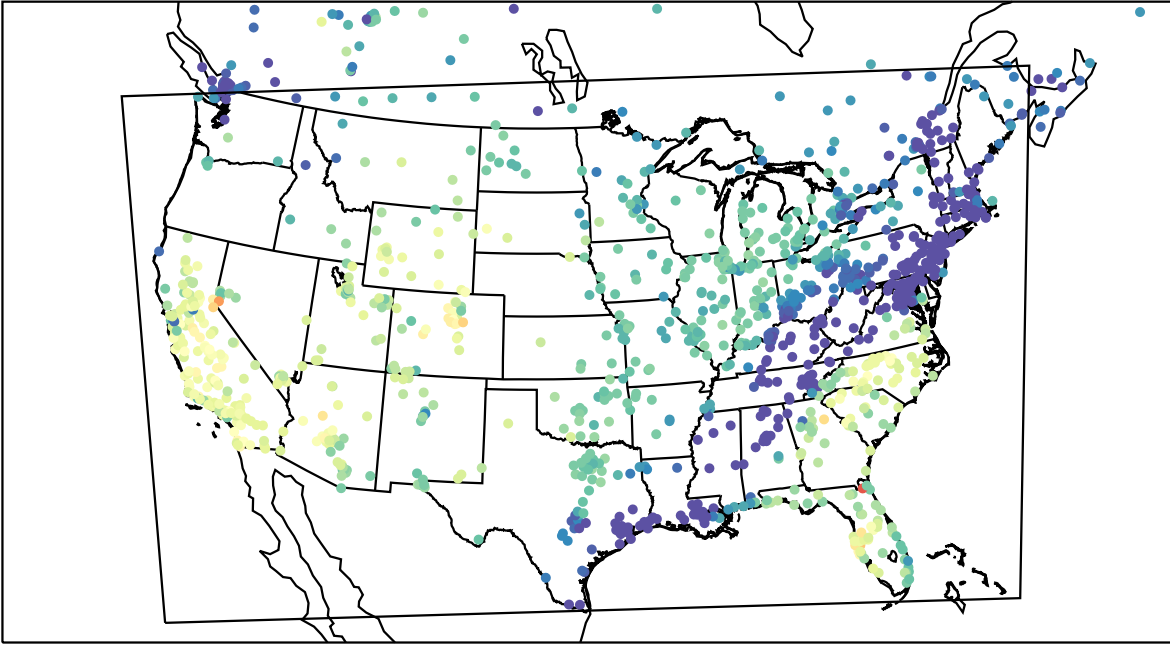
AirNOW (2023-10-30_20:00:00)
