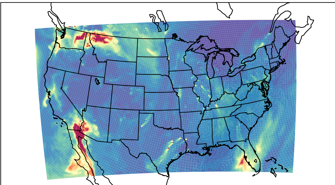
WRF 2023-11-01_15:00:00
