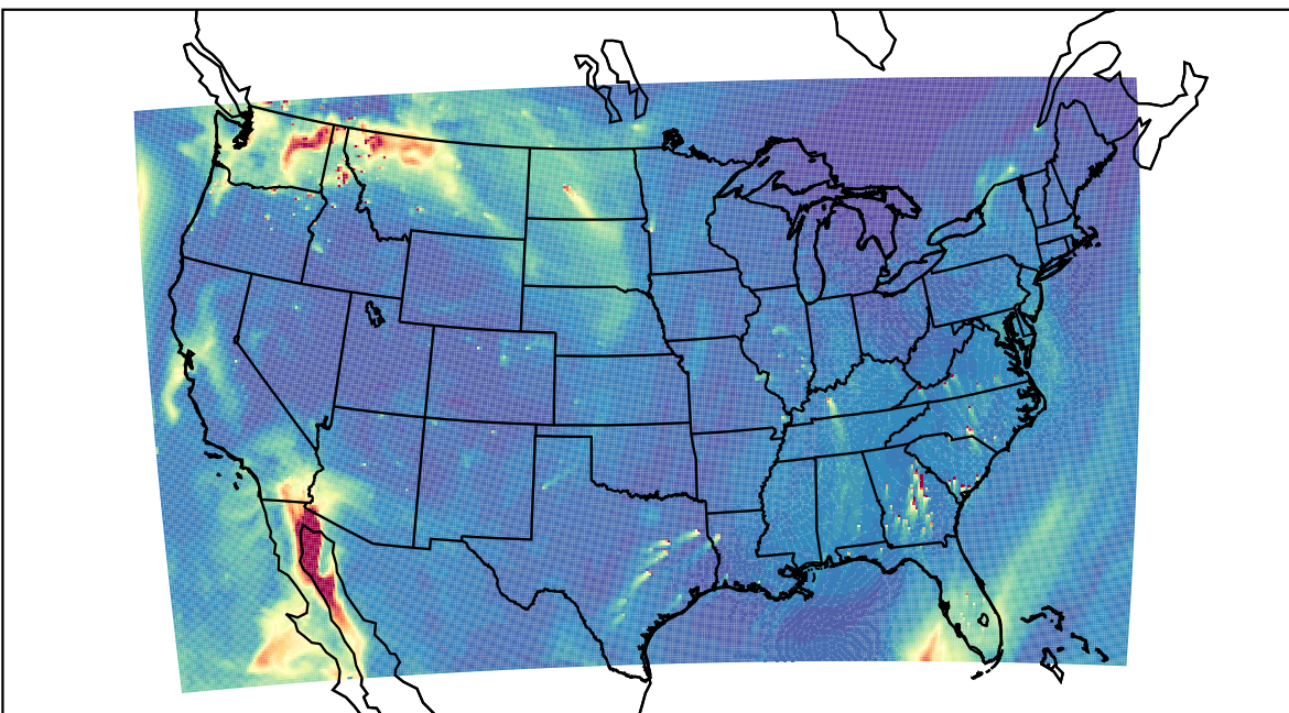
WRF 2023-11-01_19:00:00
