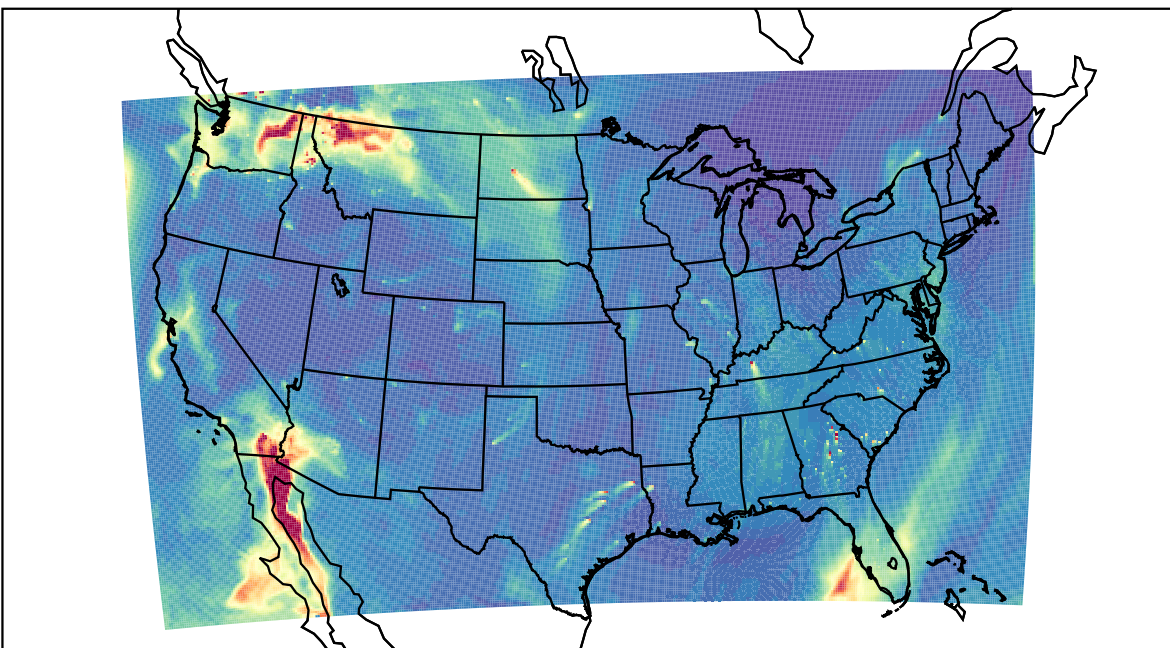
WRF 2023-11-01_17:00:00
