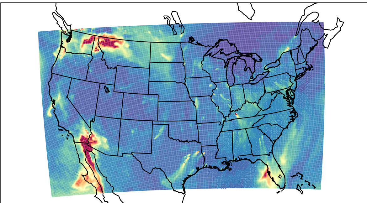
WRF 2023-11-01_14:00:00
