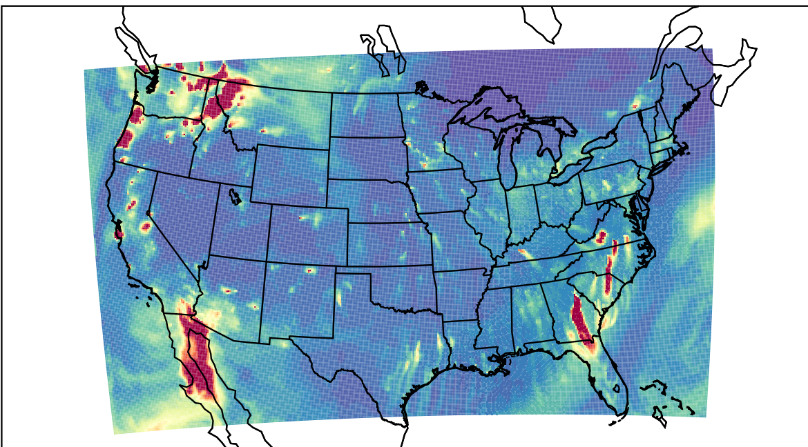
WRF 2023-11-01_03:00:00
