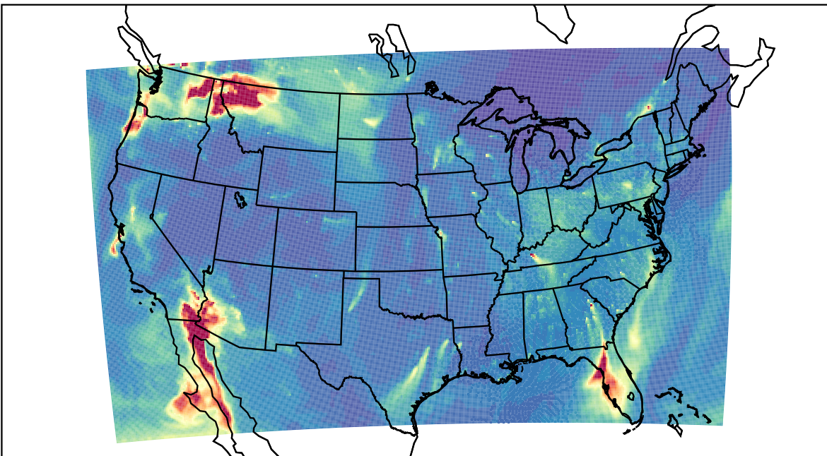
WRF 2023-11-01_11:00:00
