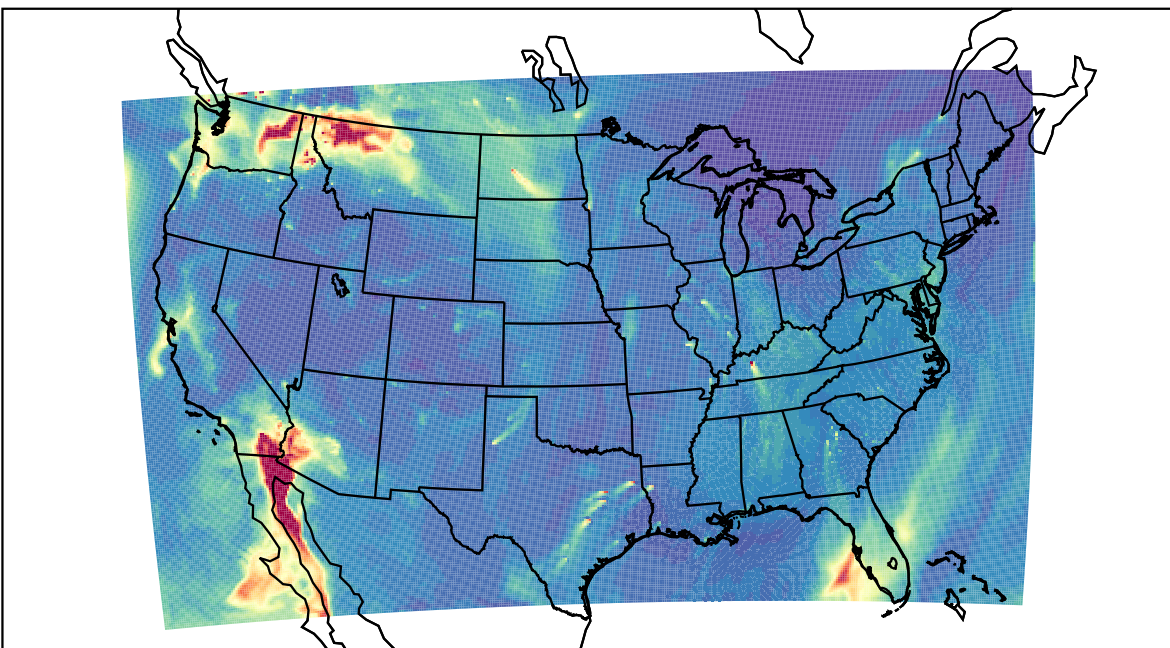
WRF 2023-11-01_16:00:00
