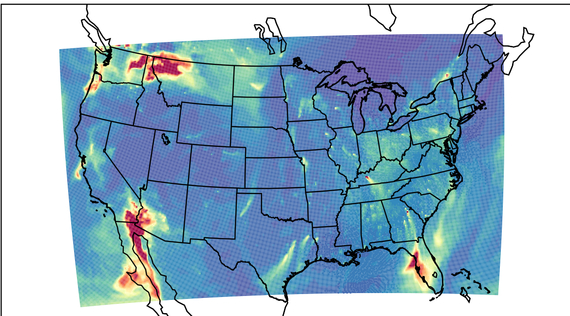
WRF 2023-11-01_12:00:00
