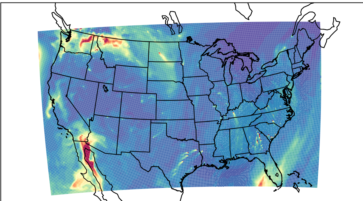
WRF 2023-11-01_18:00:00
