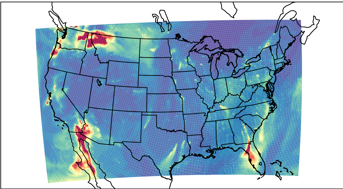
WRF 2023-11-01_10:00:00
