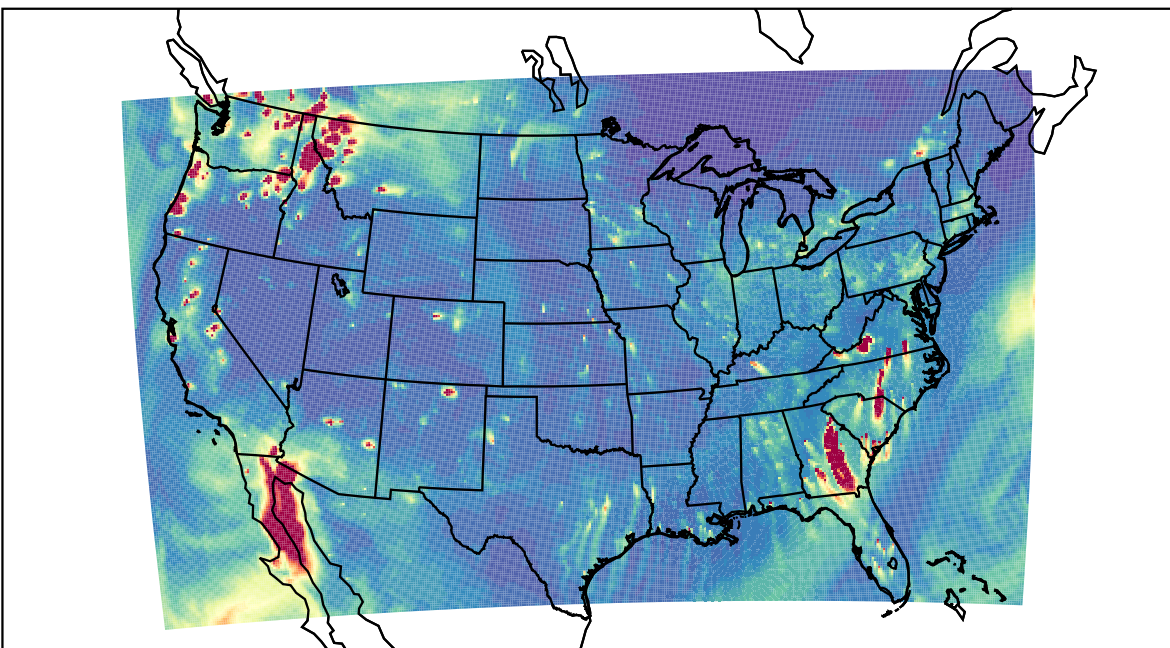
WRF 2023-11-01_01:00:00
