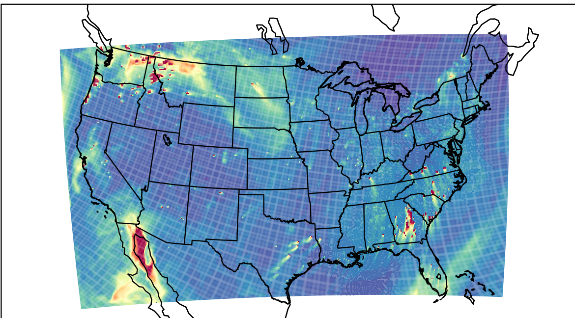
WRF 2023-11-01_22:00:00
