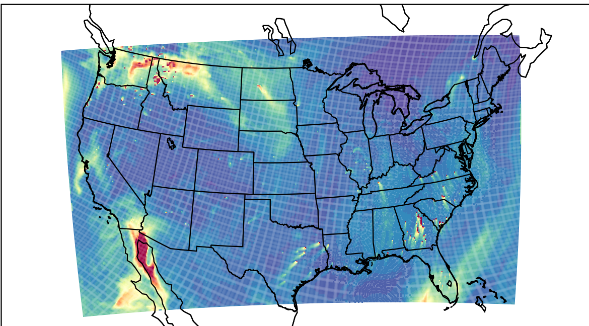
WRF 2023-11-01_20:00:00
