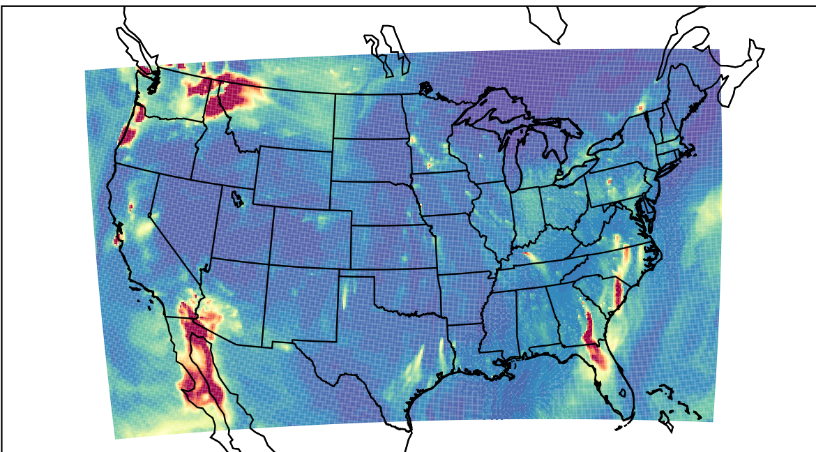
WRF 2023-11-01_06:00:00
