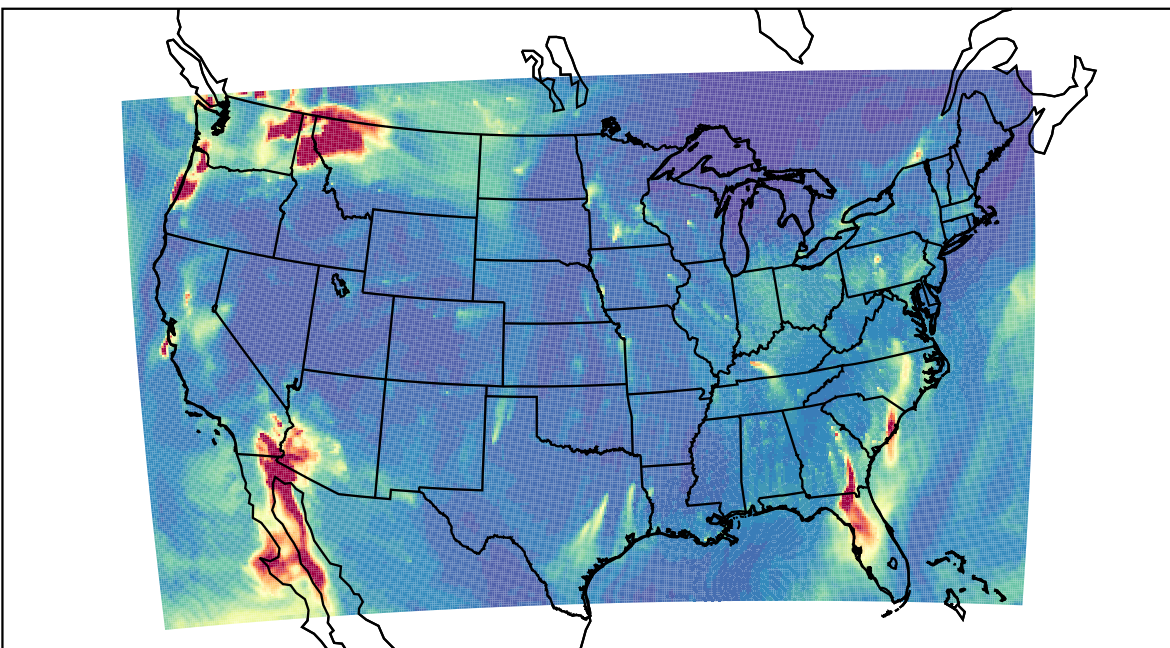
WRF 2023-11-01_08:00:00
