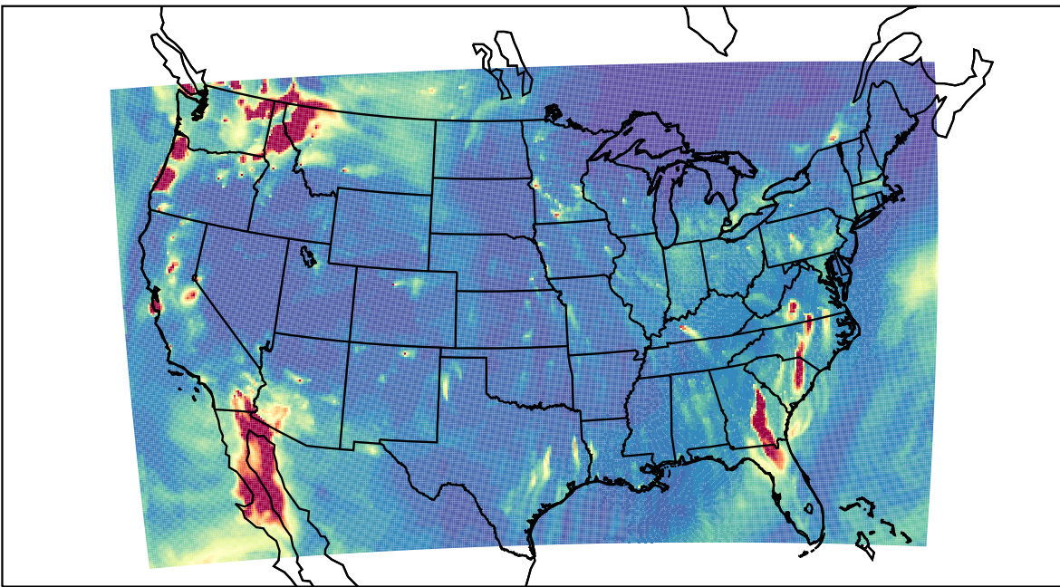
WRF 2023-11-01_04:00:00
