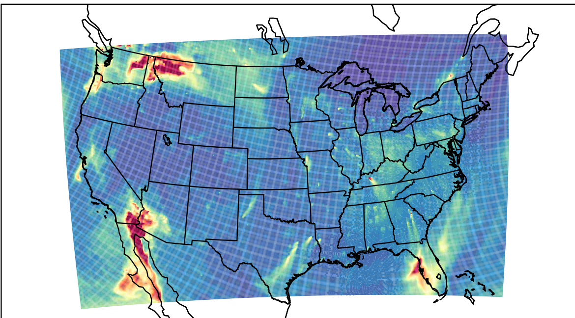
WRF 2023-11-01_13:00:00
