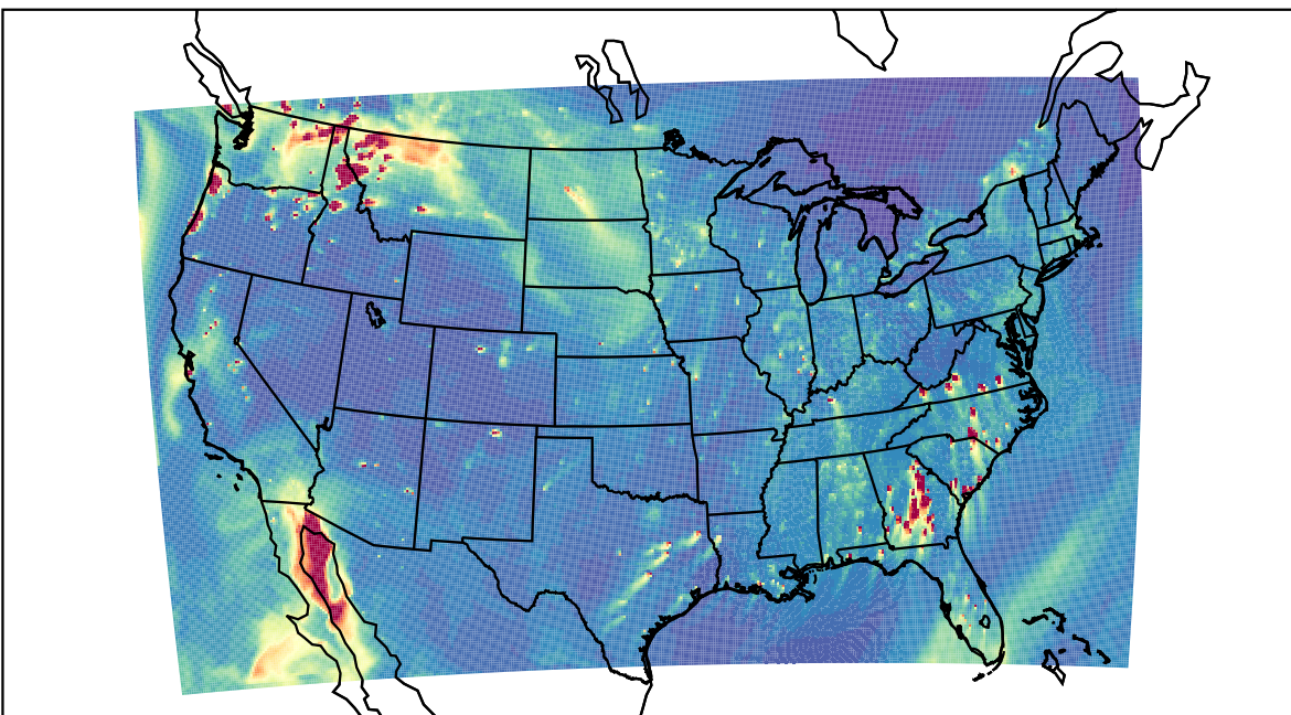
WRF 2023-11-01_23:00:00
