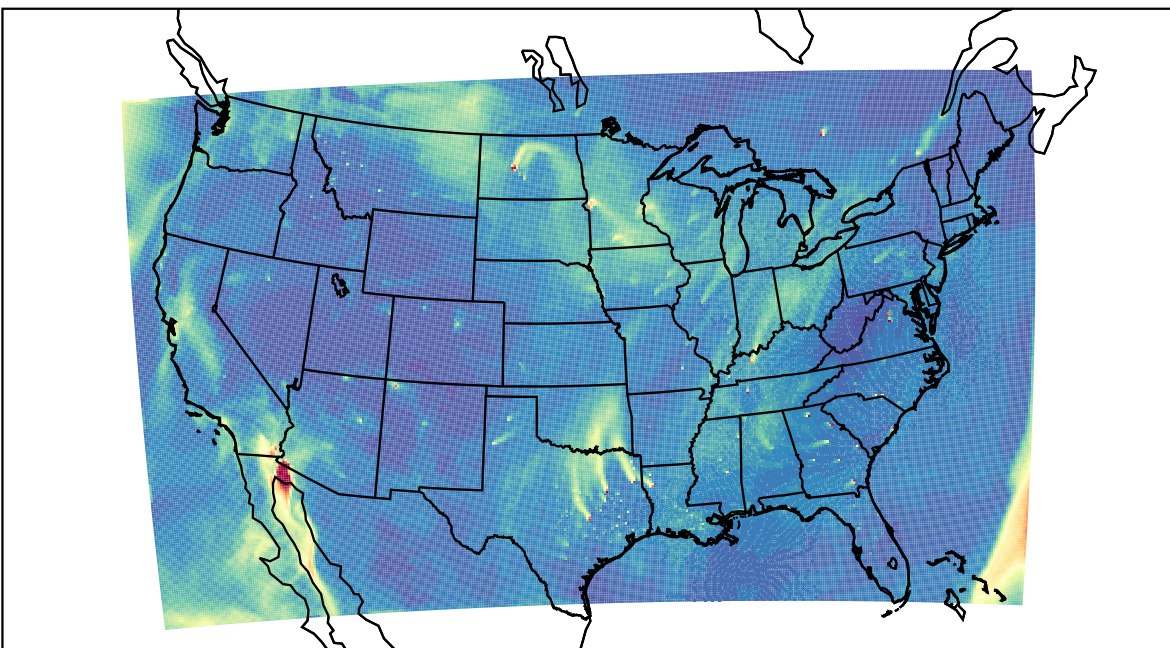
WRF 2023-11-02_18:00:00
