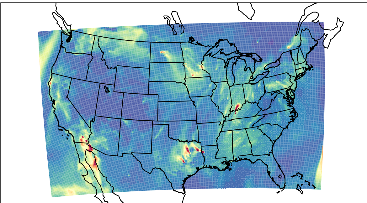
WRF 2023-11-02_10:00:00
