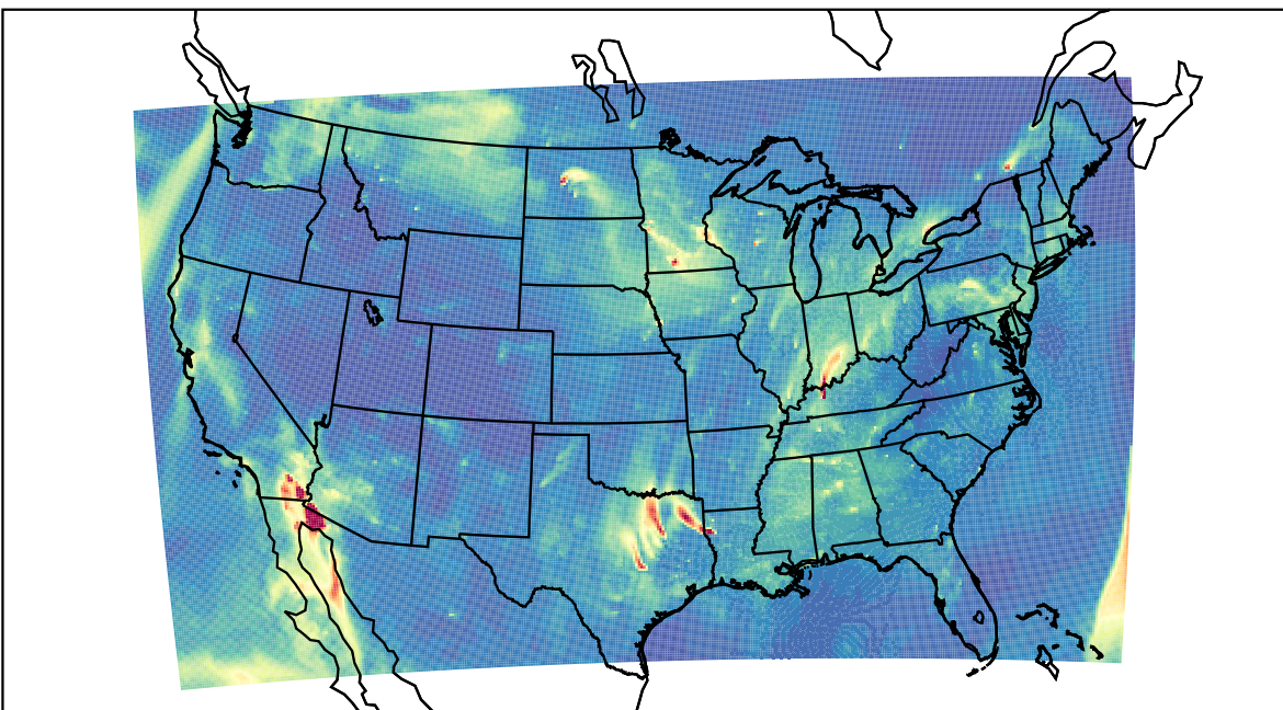
WRF 2023-11-02_13:00:00
