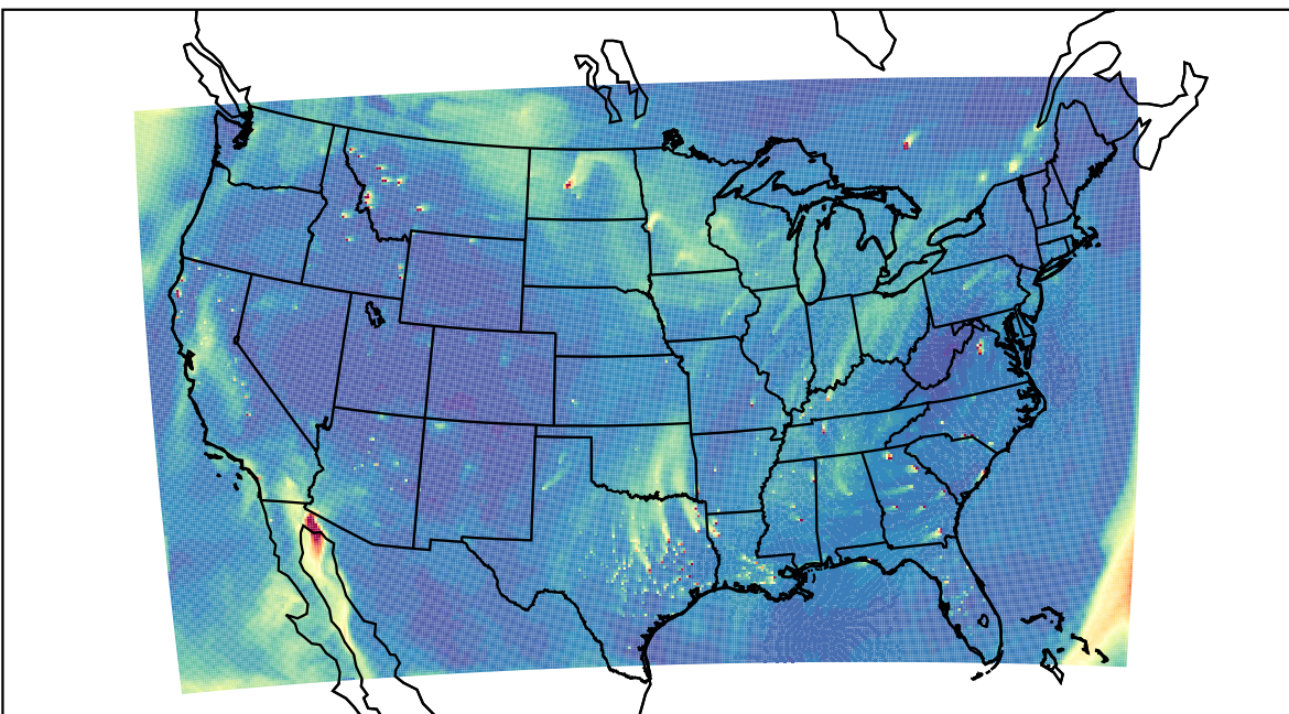
WRF 2023-11-02_20:00:00
