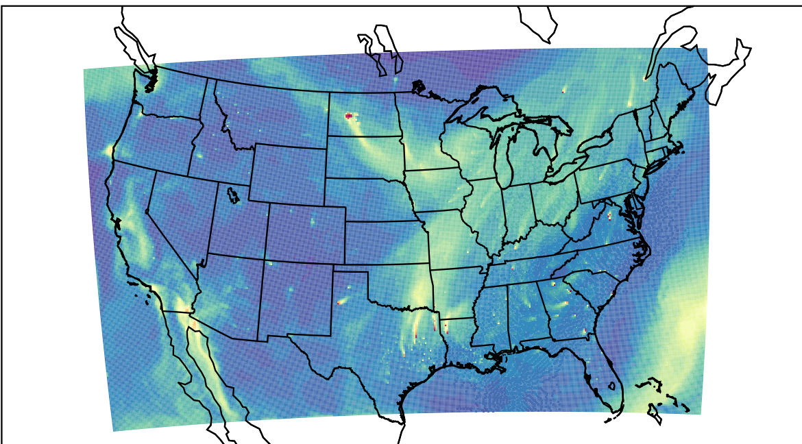
WRF 2023-11-03_18:00:00
