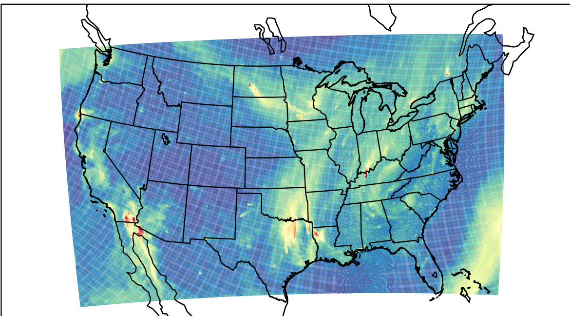
WRF 2023-11-03_13:00:00
