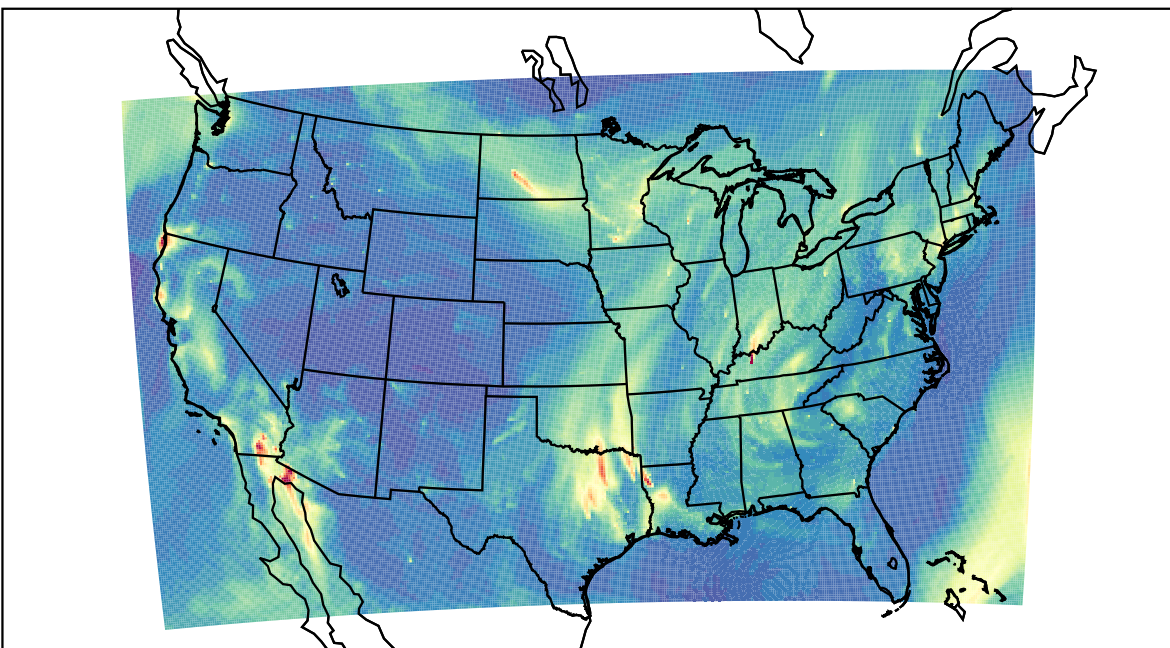
WRF 2023-11-03_10:00:00
