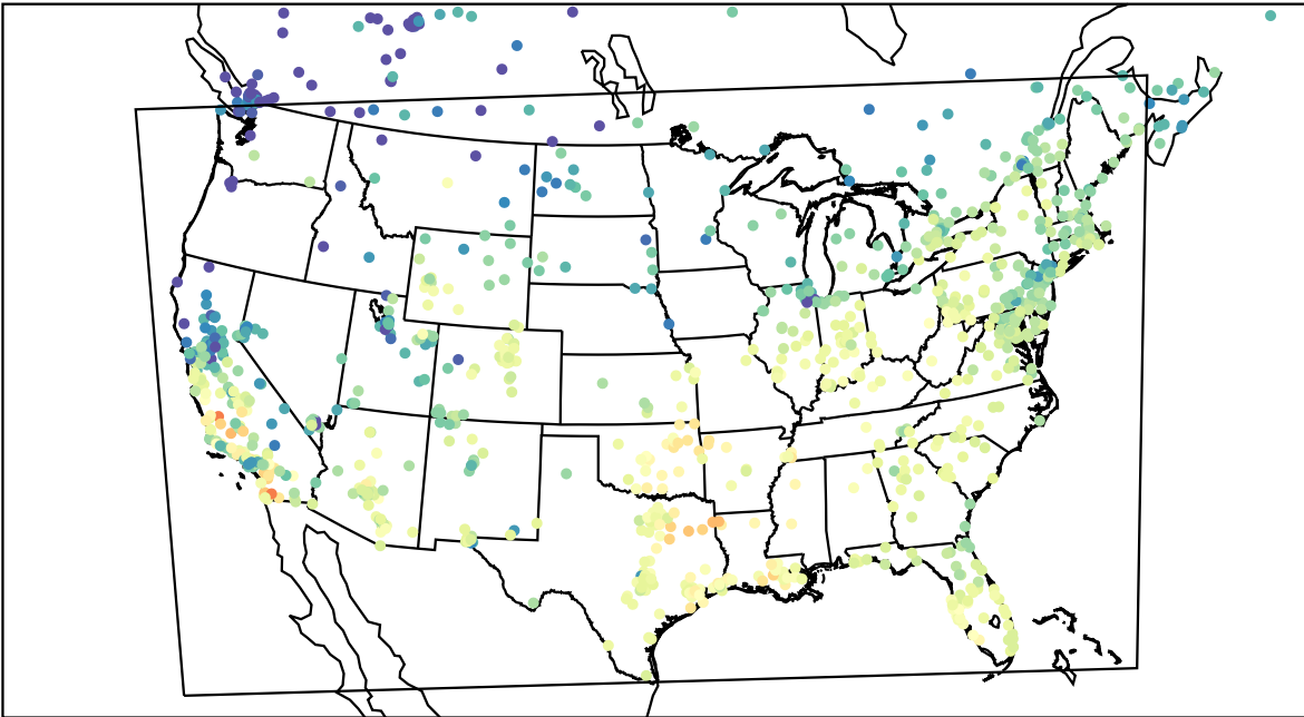
AirNOW (2023-11-03_18:00:00)
