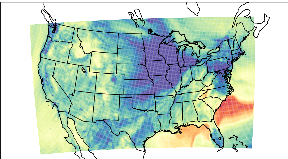
WRF (2023-11-09_04:00:00)
