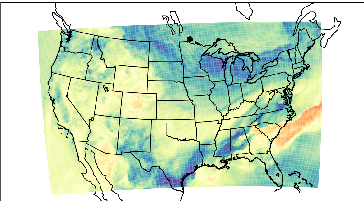
WRF (2023-11-10_20:00:00)
