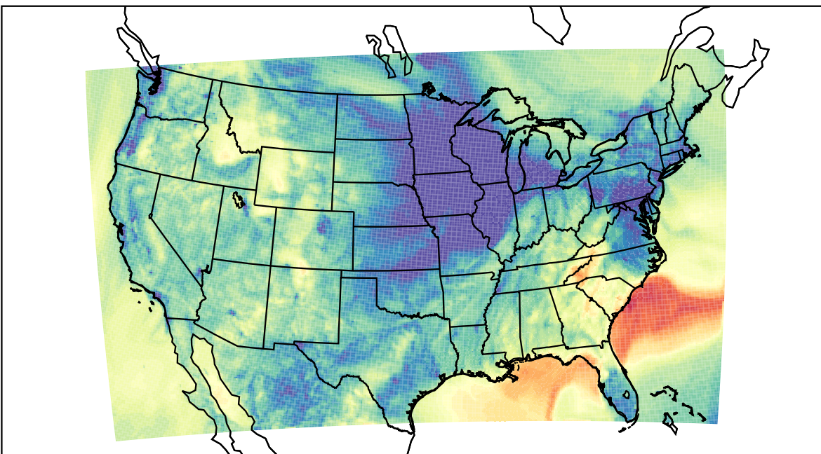
WRF (2023-11-09_03:00:00)
