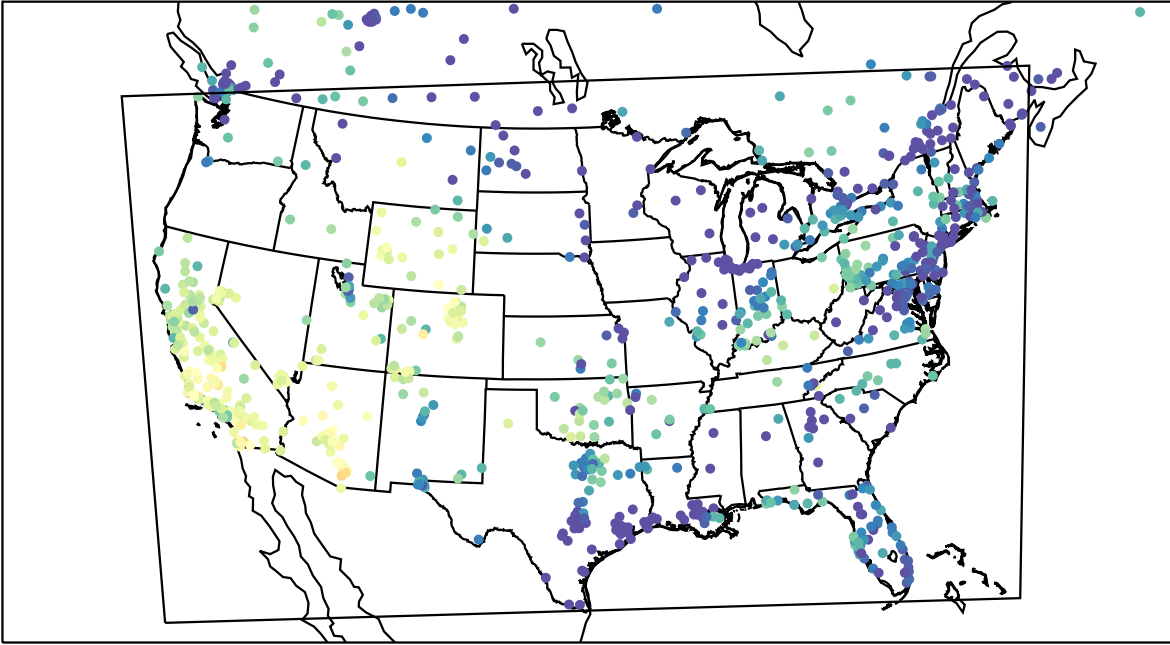
AirNOW (2023-11-10_23:00:00)
