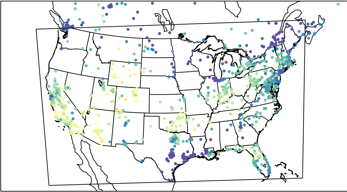
AirNOW (2023-11-10_20:00:00)
