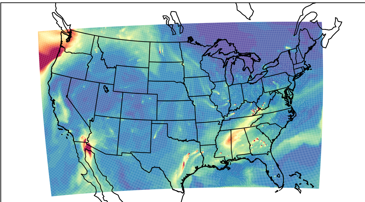
WRF 2023-11-11_18:00:00
