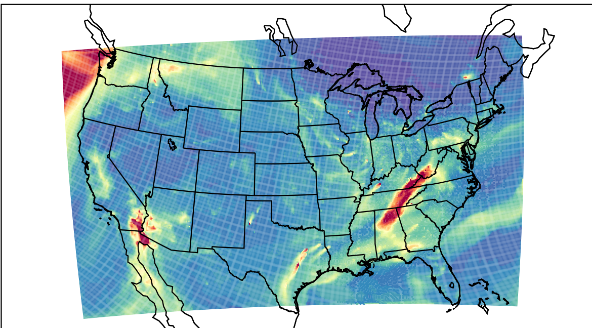
WRF 2023-11-11_13:00:00
