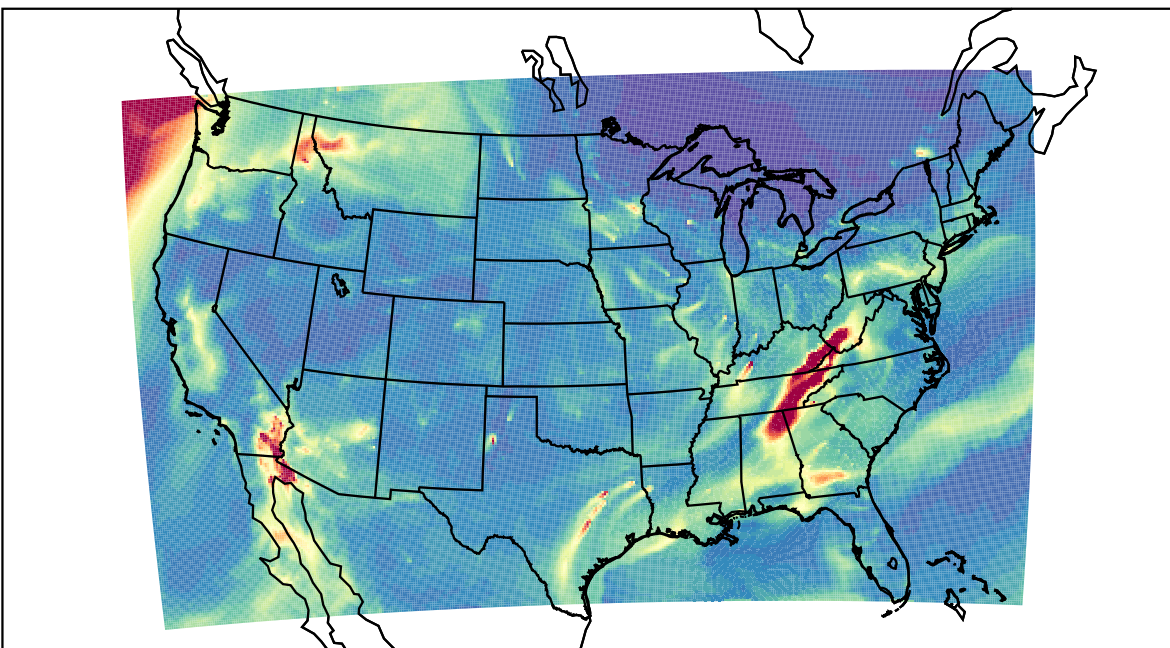
WRF 2023-11-11_10:00:00
