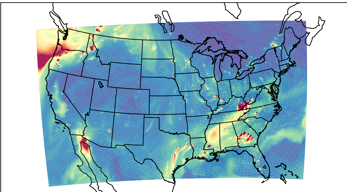
WRF 2023-11-11_22:00:00
