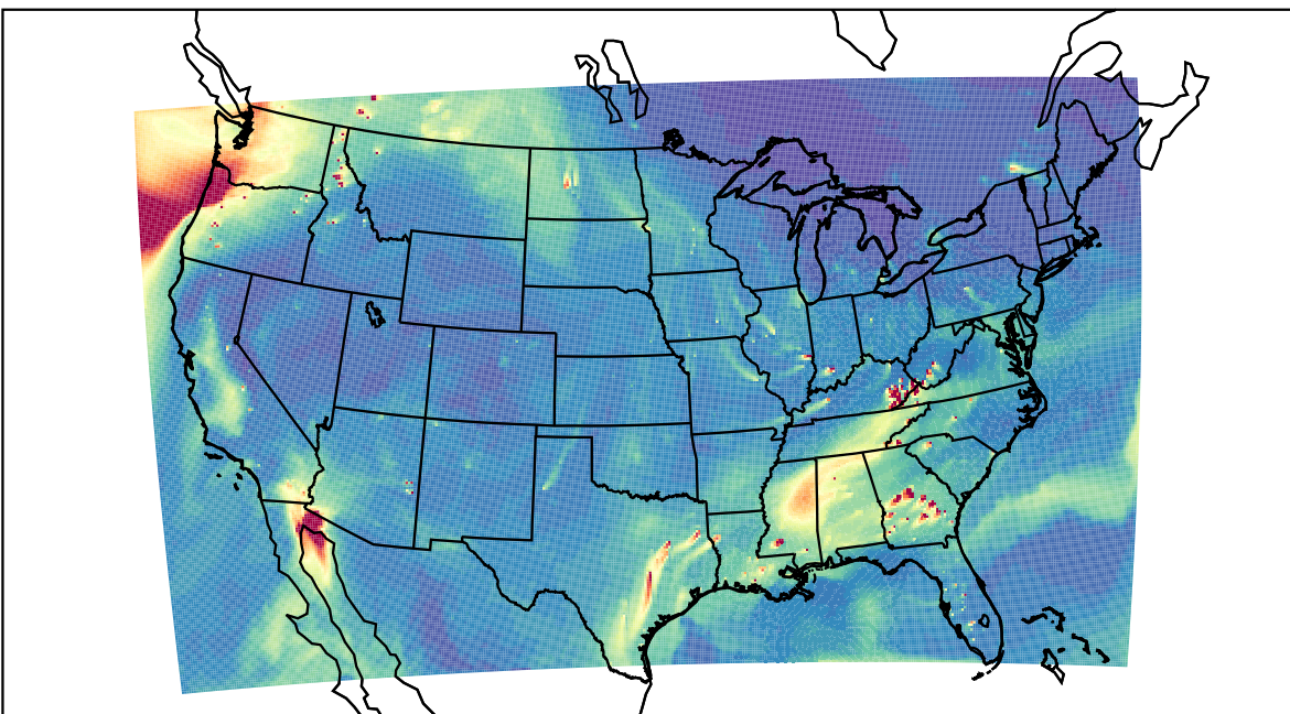
WRF 2023-11-11_20:00:00
