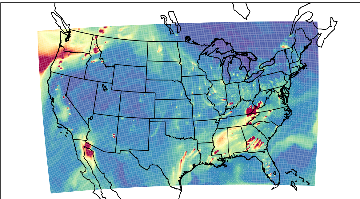
WRF 2023-11-11_23:00:00
