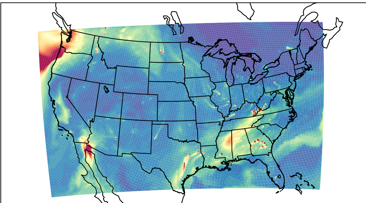
WRF 2023-11-11_19:00:00
