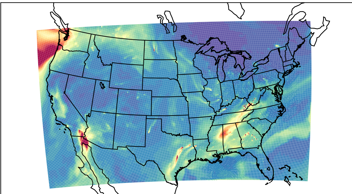
WRF 2023-11-11_17:00:00
