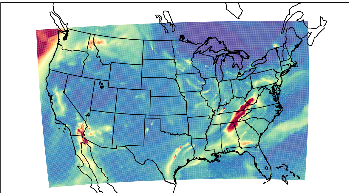
WRF 2023-11-11_11:00:00
