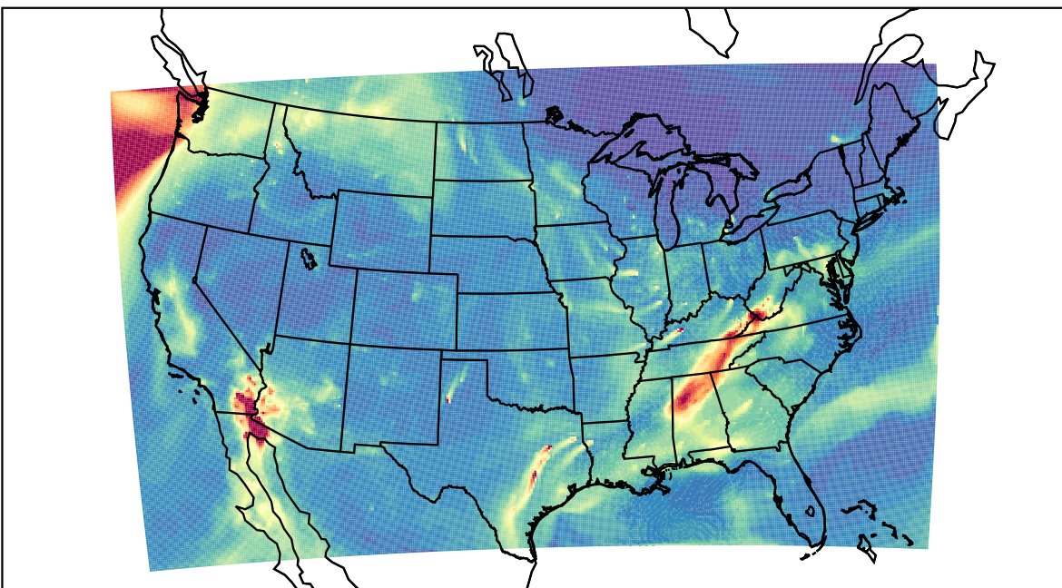
WRF 2023-11-11_15:00:00
