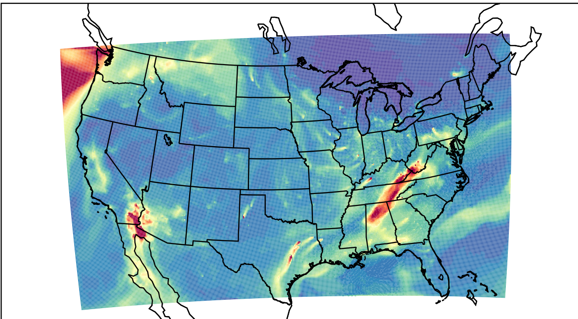
WRF 2023-11-11_14:00:00
