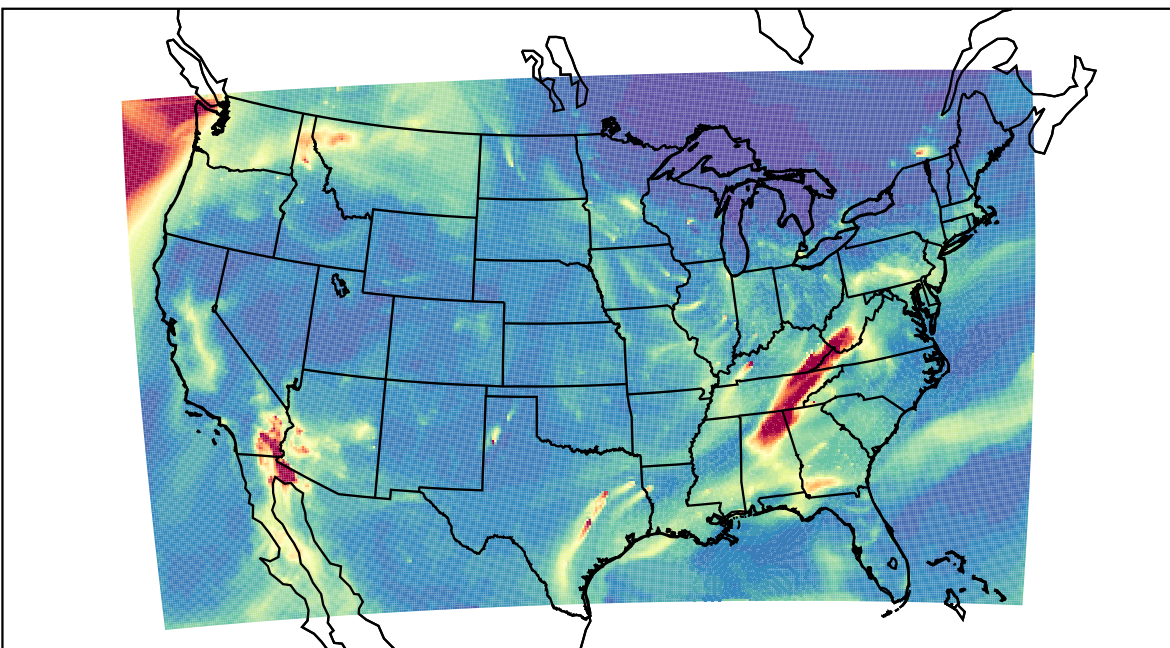
WRF 2023-11-11_12:00:00
