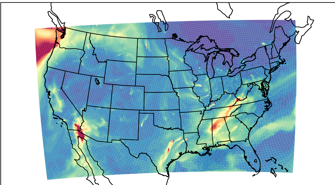
WRF 2023-11-11_16:00:00
