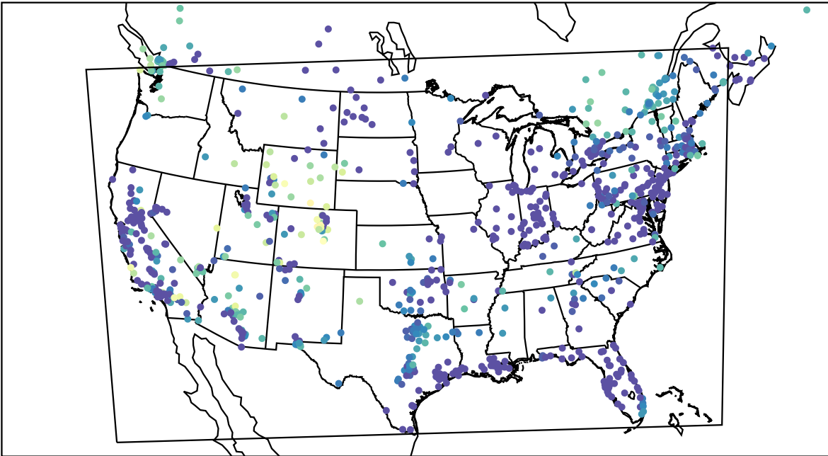
AirNOW (2023-11-11_10:00:00)
