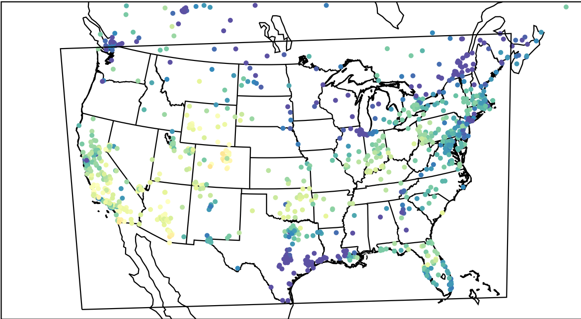
AirNOW (2023-11-10_20:00:00)
