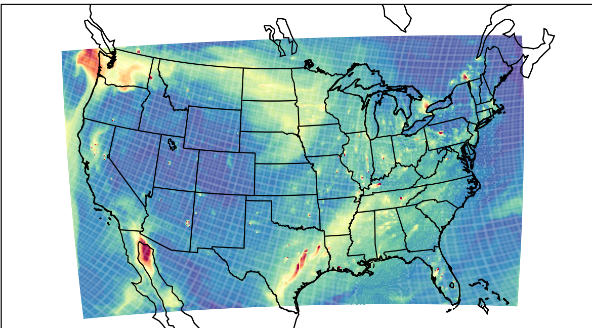
WRF 2023-11-12_23:00:00
