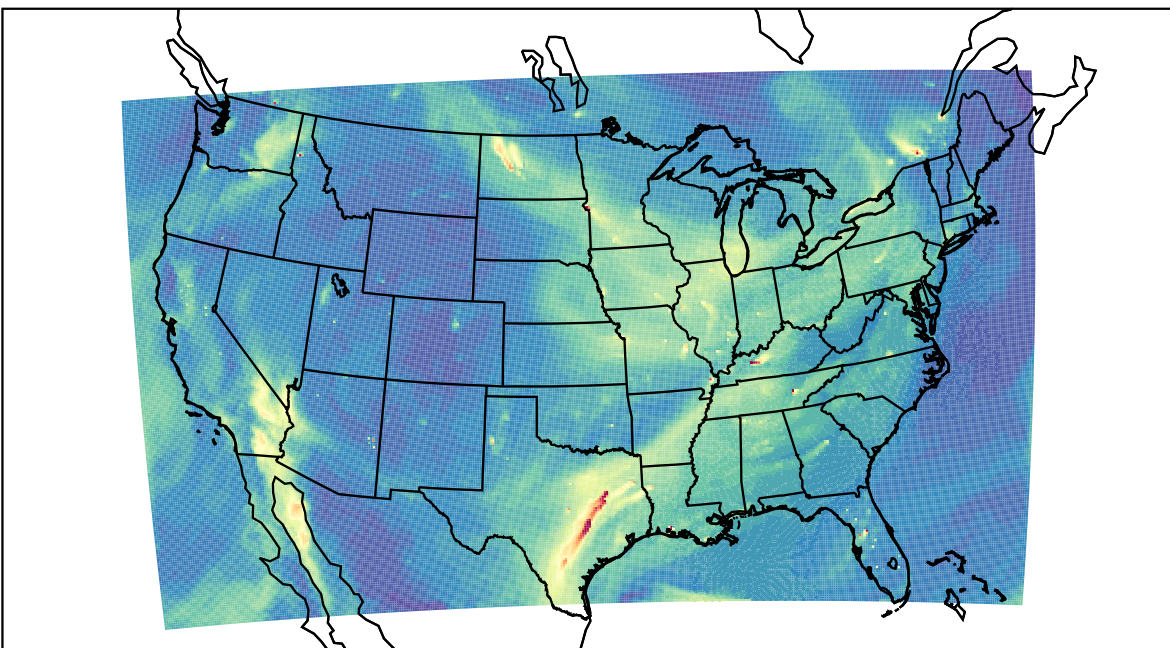
WRF 2023-11-13_20:00:00
