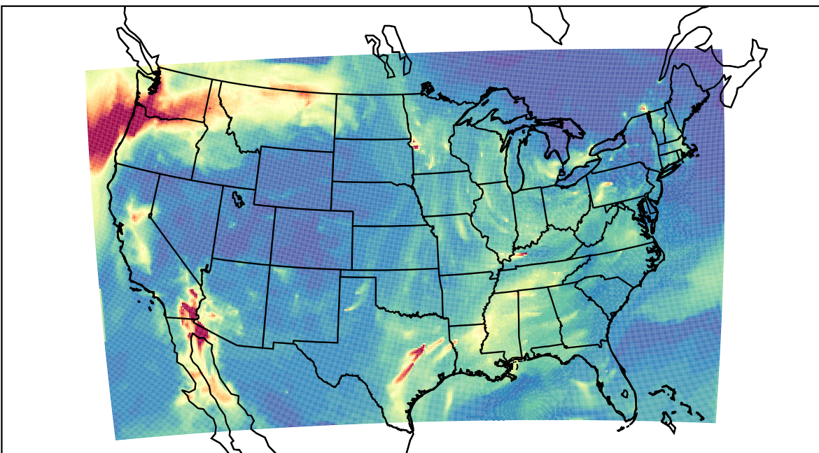
WRF 2023-11-12_10:00:00
