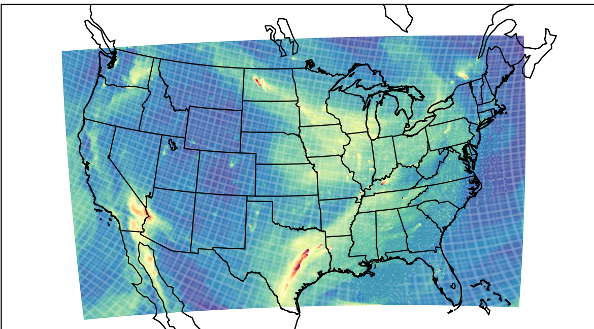
WRF 2023-11-13_18:00:00
