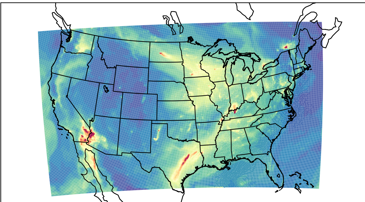
WRF 2023-11-13_13:00:00
