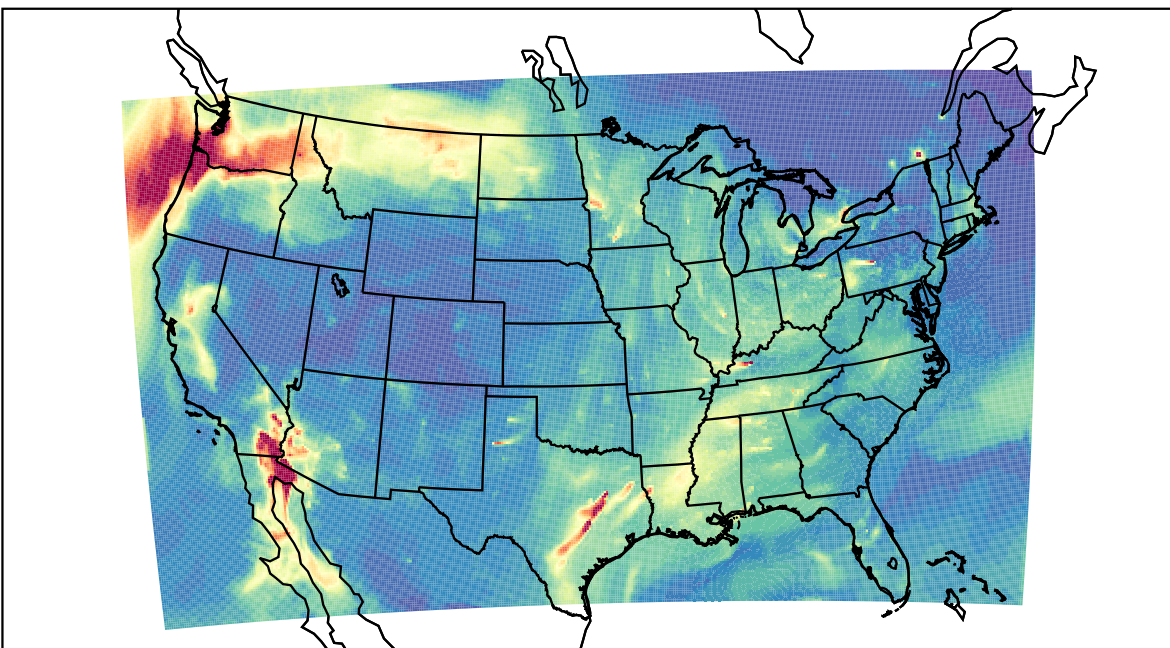
WRF 2023-11-12_13:00:00
