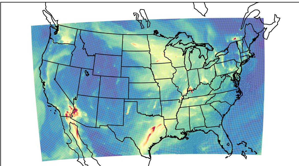
WRF 2023-11-13_10:00:00
