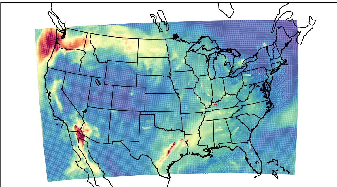
WRF 2023-11-12_16:00:00
