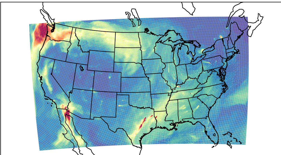
WRF 2023-11-12_18:00:00
