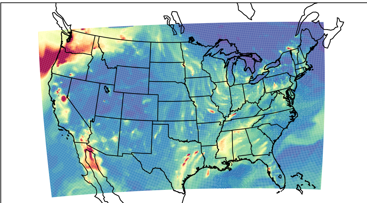
WRF 2023-11-12_04:00:00
