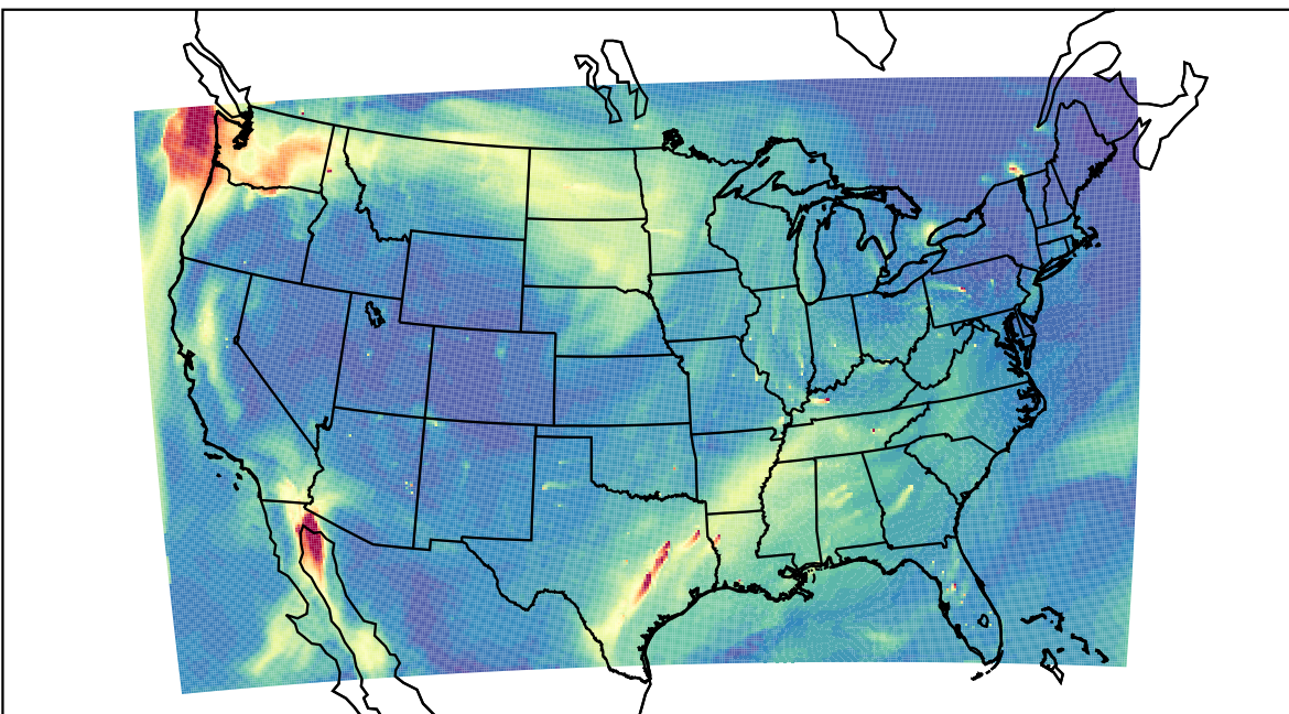
WRF 2023-11-12_20:00:00
