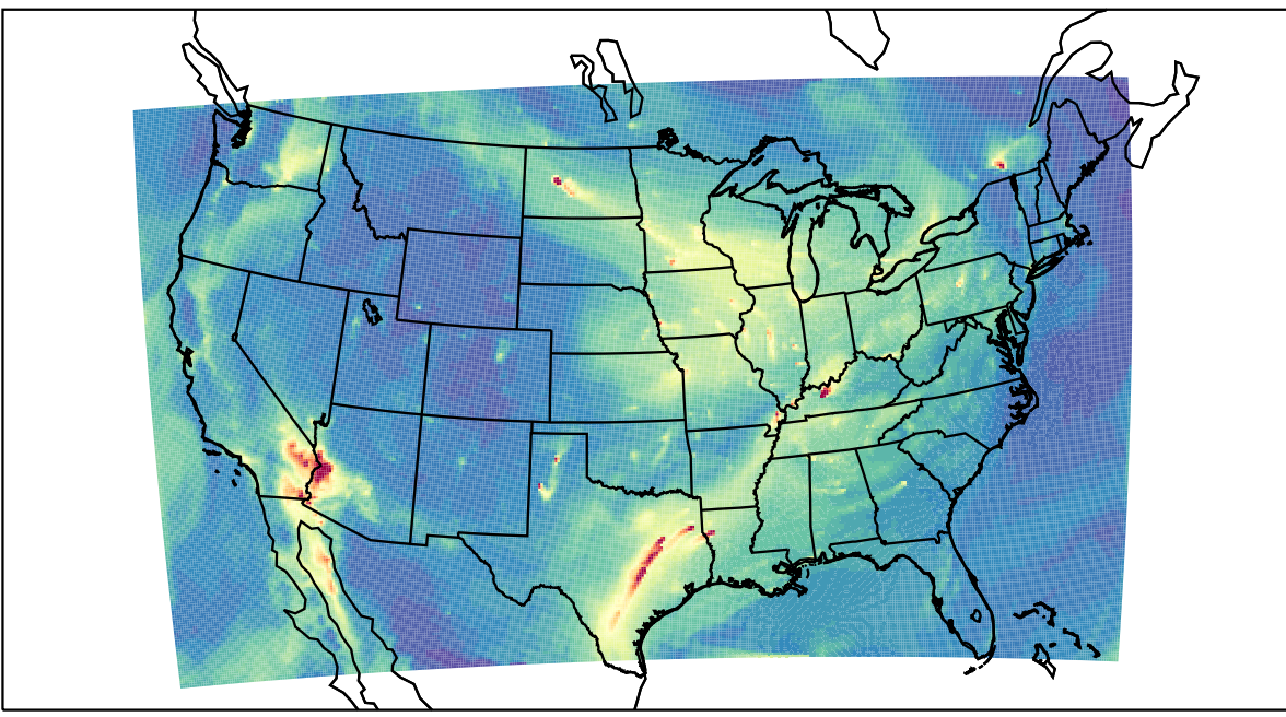
WRF 2023-11-13_16:00:00
