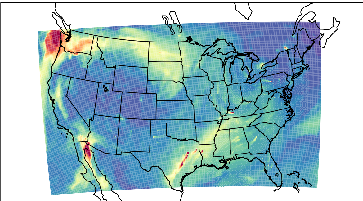
WRF 2023-11-12_19:00:00
