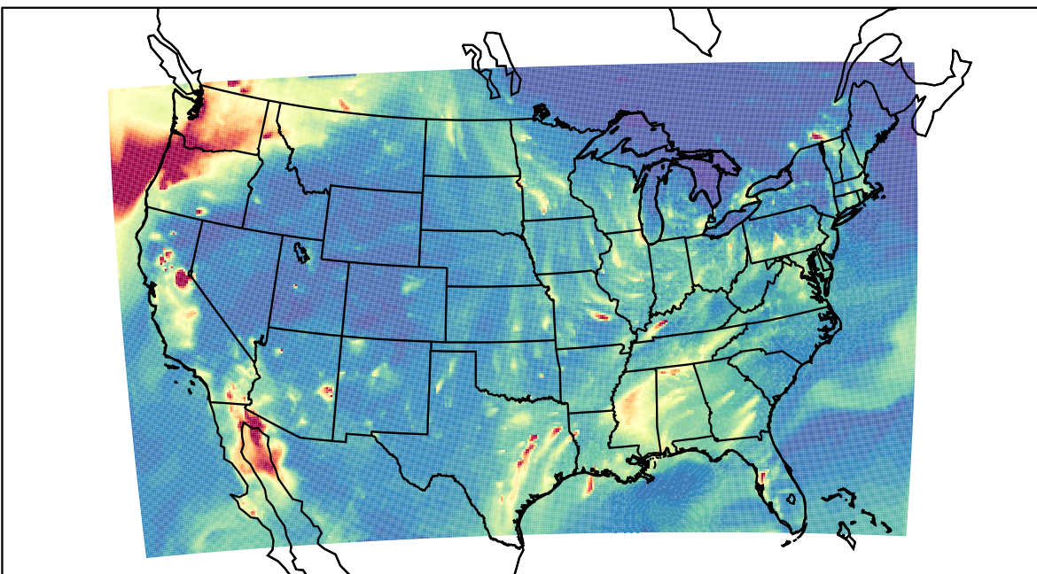
WRF 2023-11-12_03:00:00
