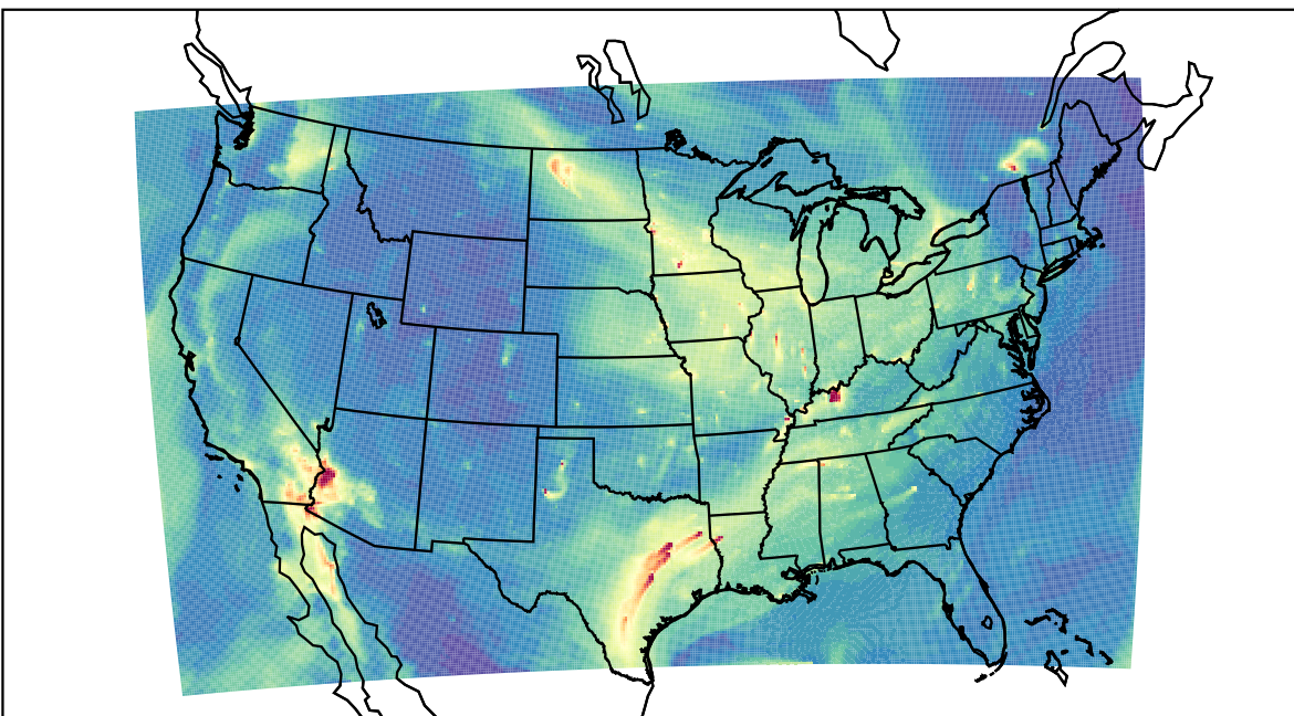
WRF 2023-11-13_16:00:00
