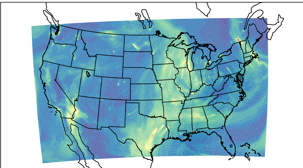
WRF 2023-11-14_18:00:00
