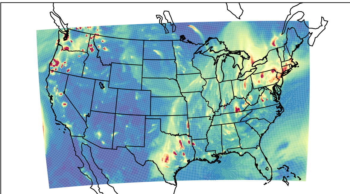
WRF 2023-11-17_03:00:00
