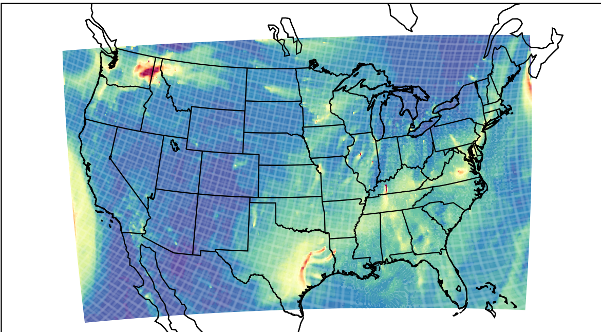
WRF 2023-11-18_11:00:00
