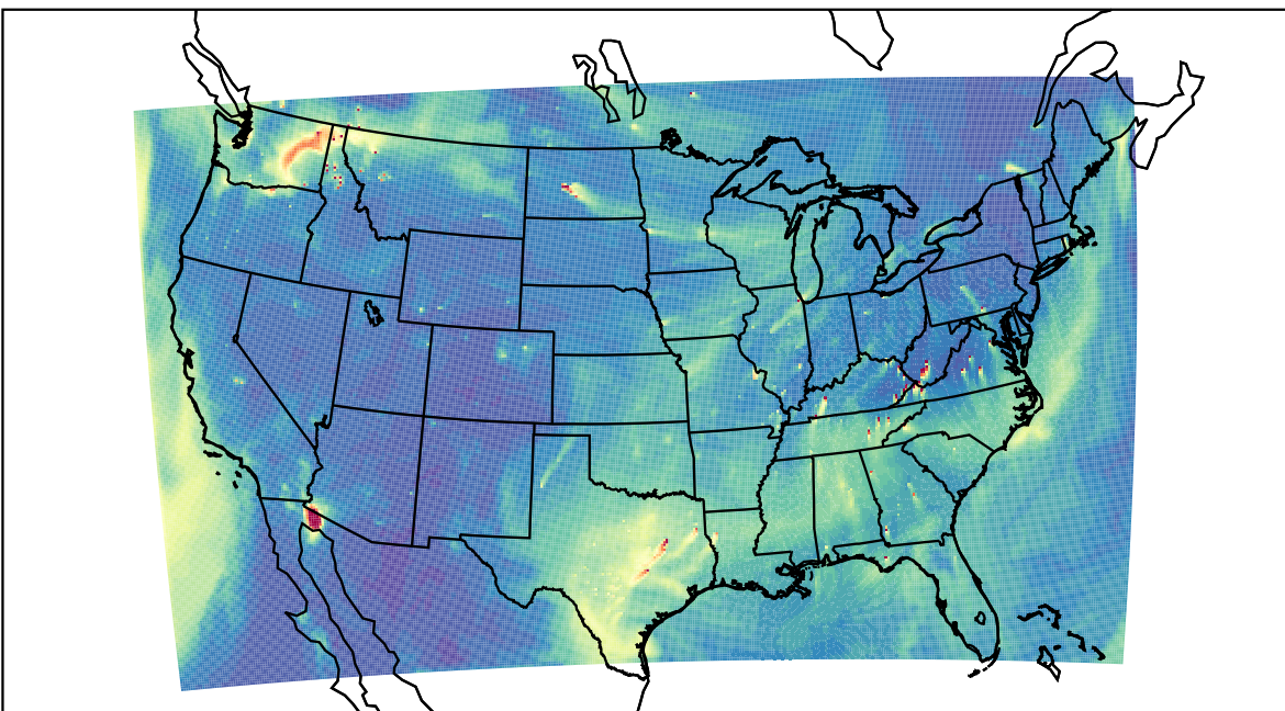
WRF 2023-11-18_19:00:00
