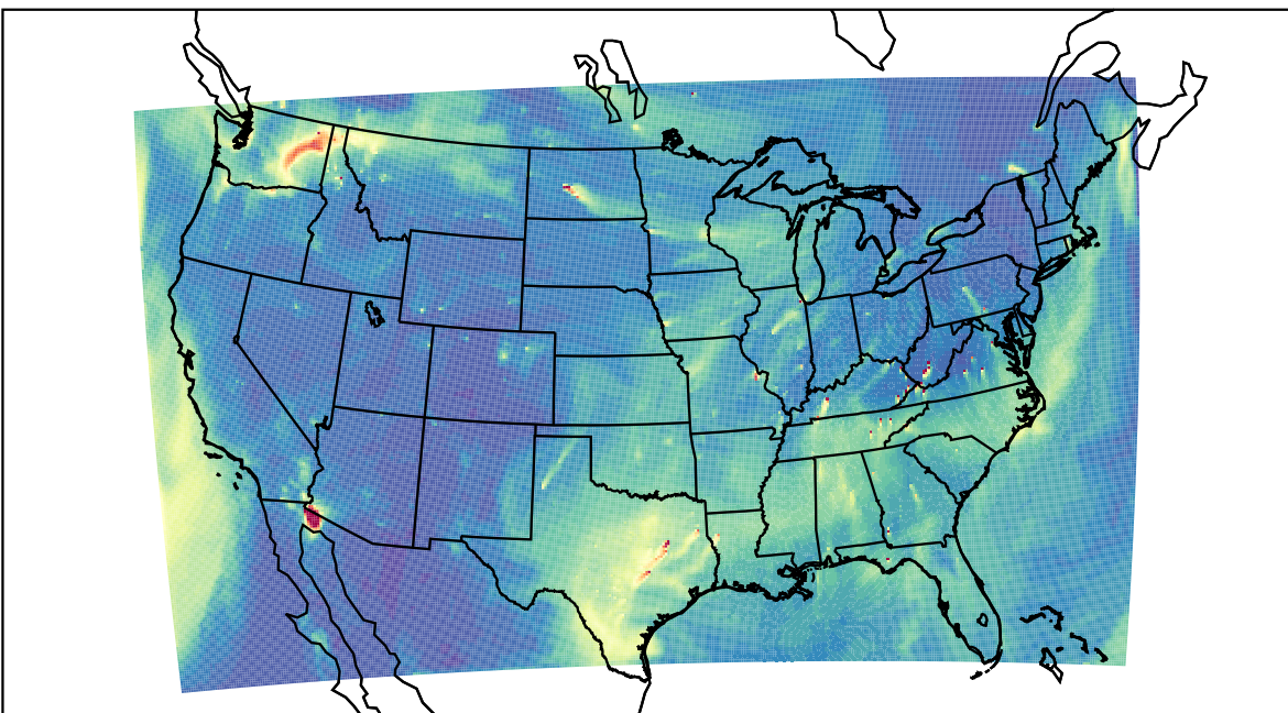
WRF 2023-11-18_18:00:00
