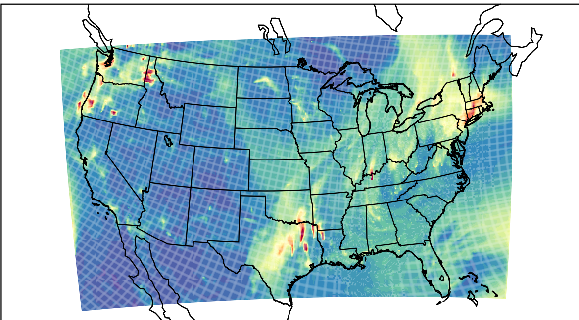
WRF 2023-11-17_08:00:00
