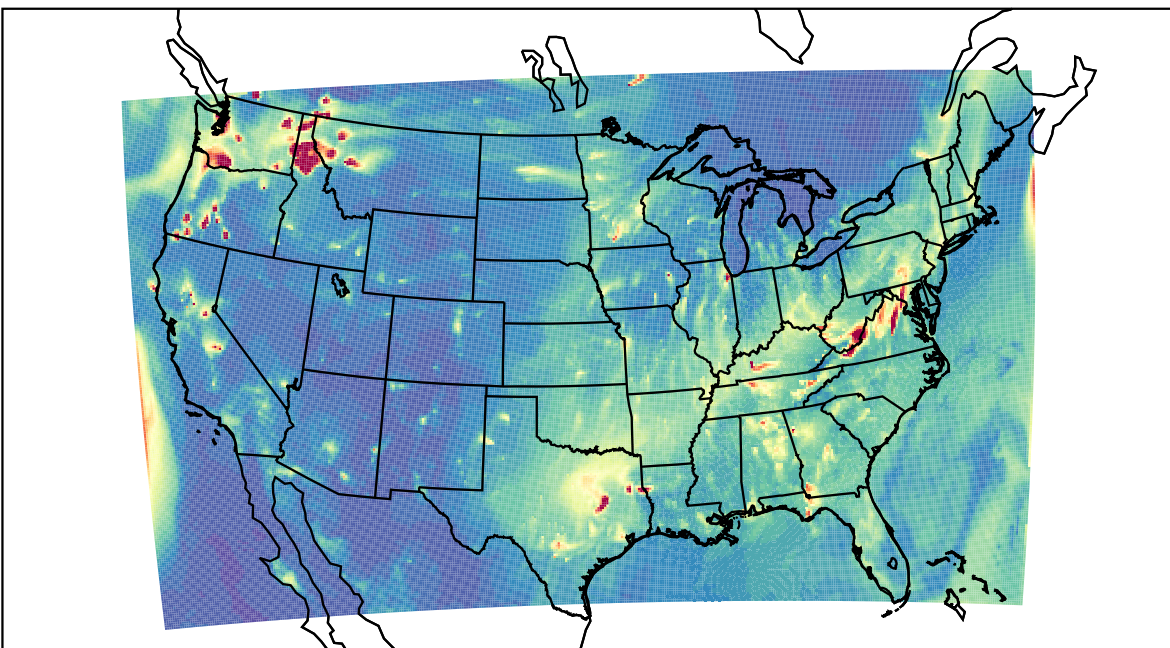
WRF 2023-11-18_03:00:00
