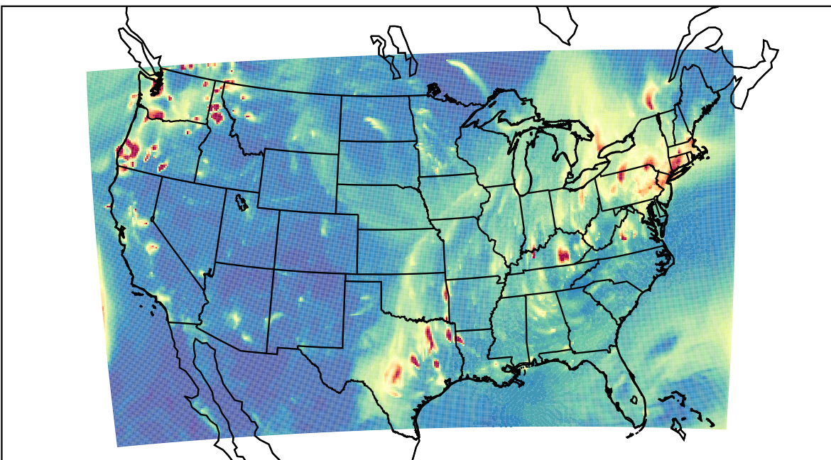
WRF 2023-11-17_04:00:00
