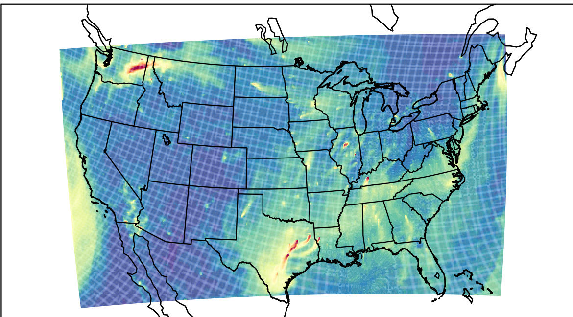
WRF 2023-11-18_15:00:00
