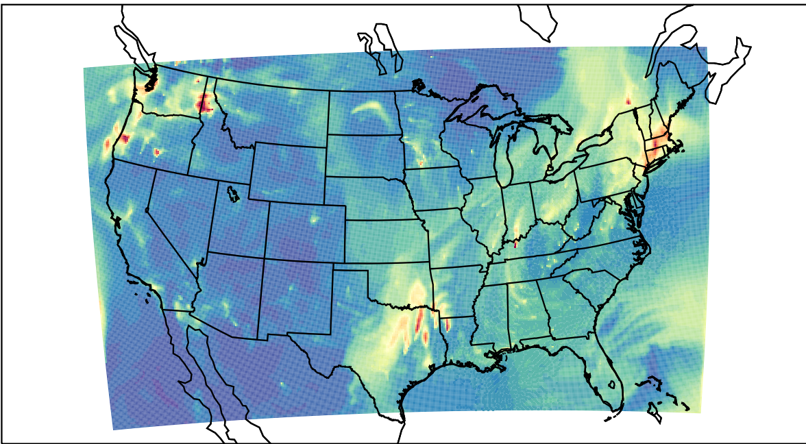
WRF 2023-11-17_10:00:00
