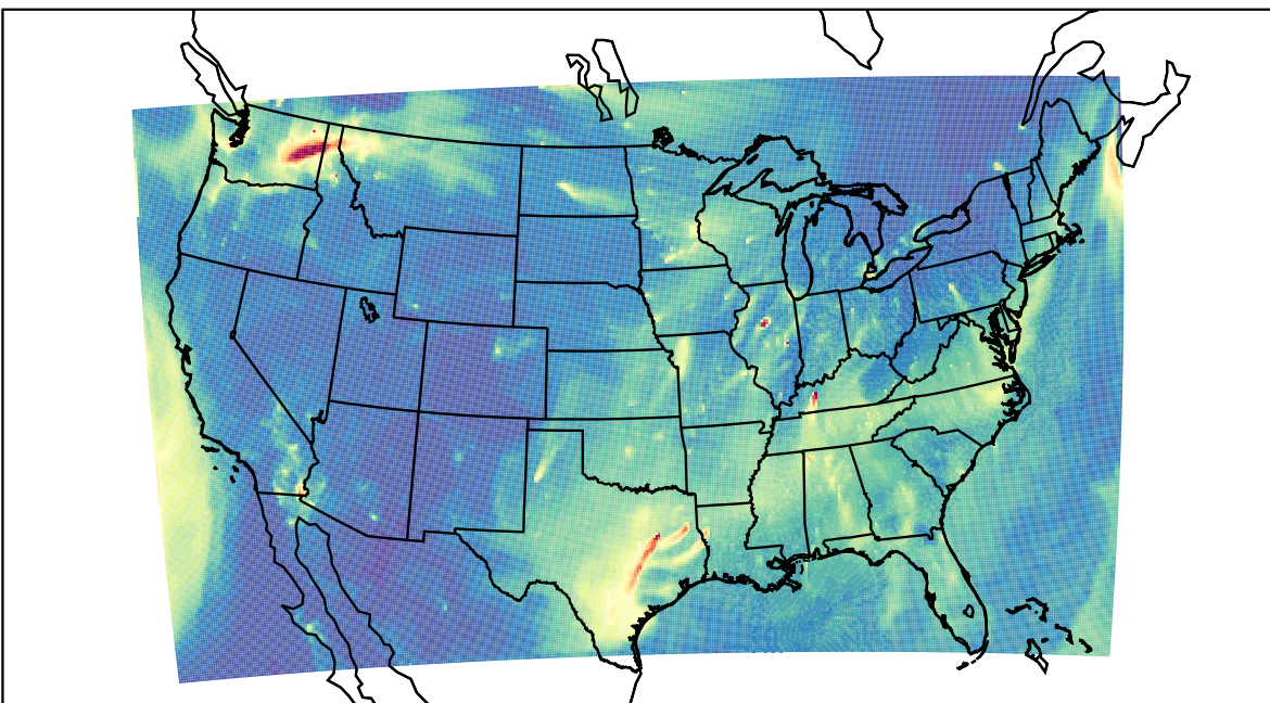
WRF 2023-11-18_14:00:00
