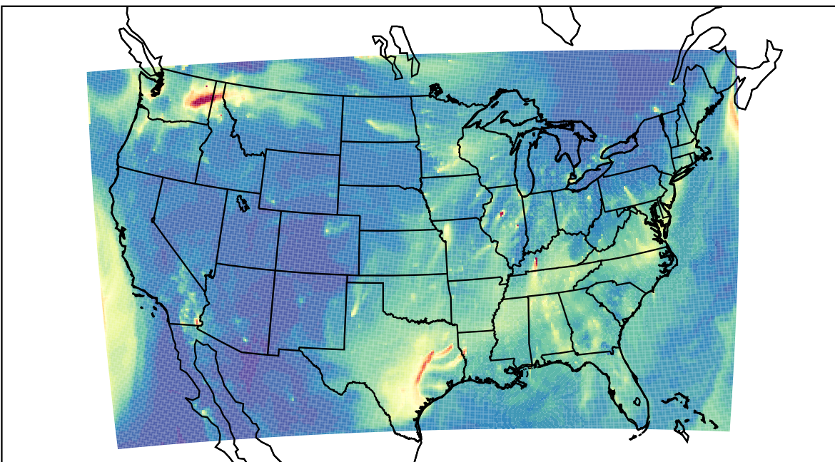
WRF 2023-11-18_13:00:00
