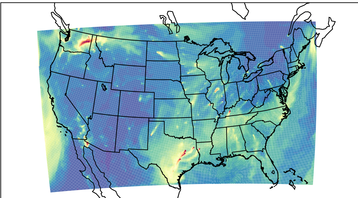
WRF 2023-11-18_16:00:00
