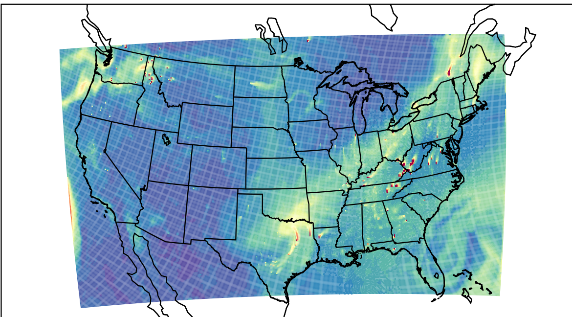
WRF 2023-11-17_20:00:00
