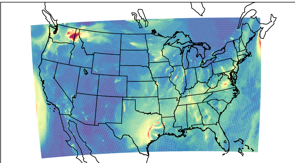
WRF 2023-11-18_10:00:00
