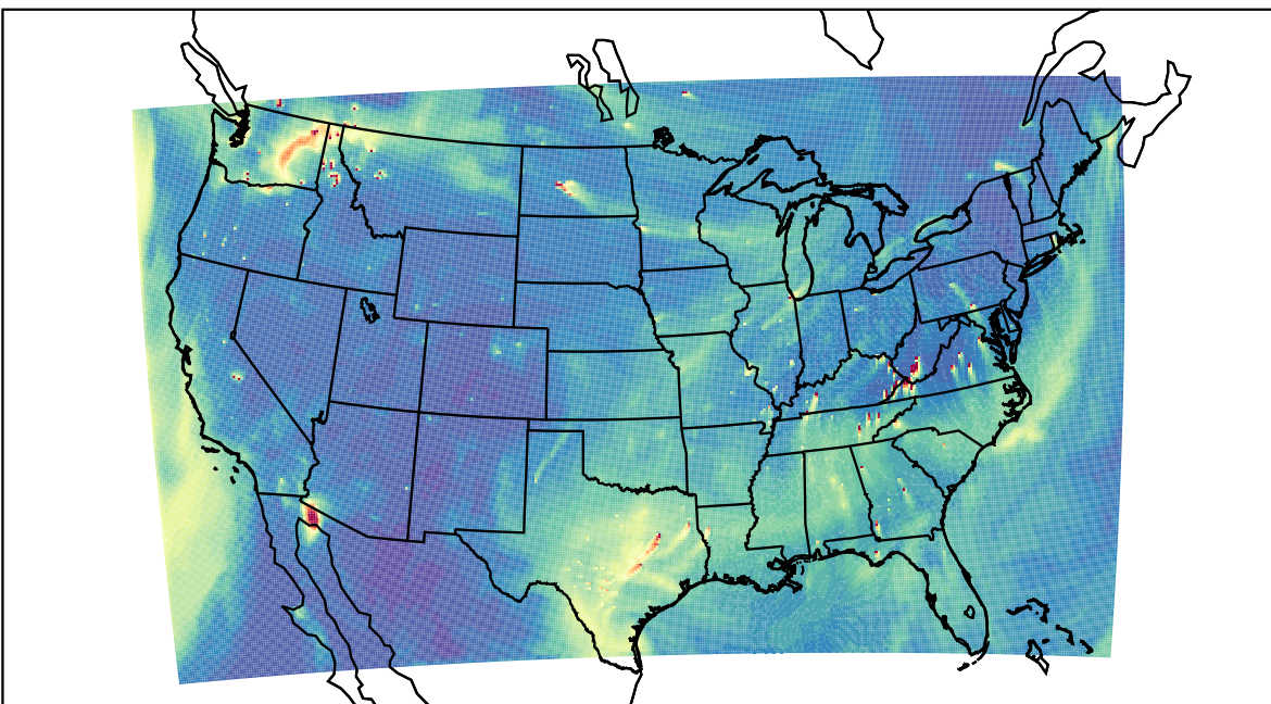
WRF 2023-11-18_20:00:00
