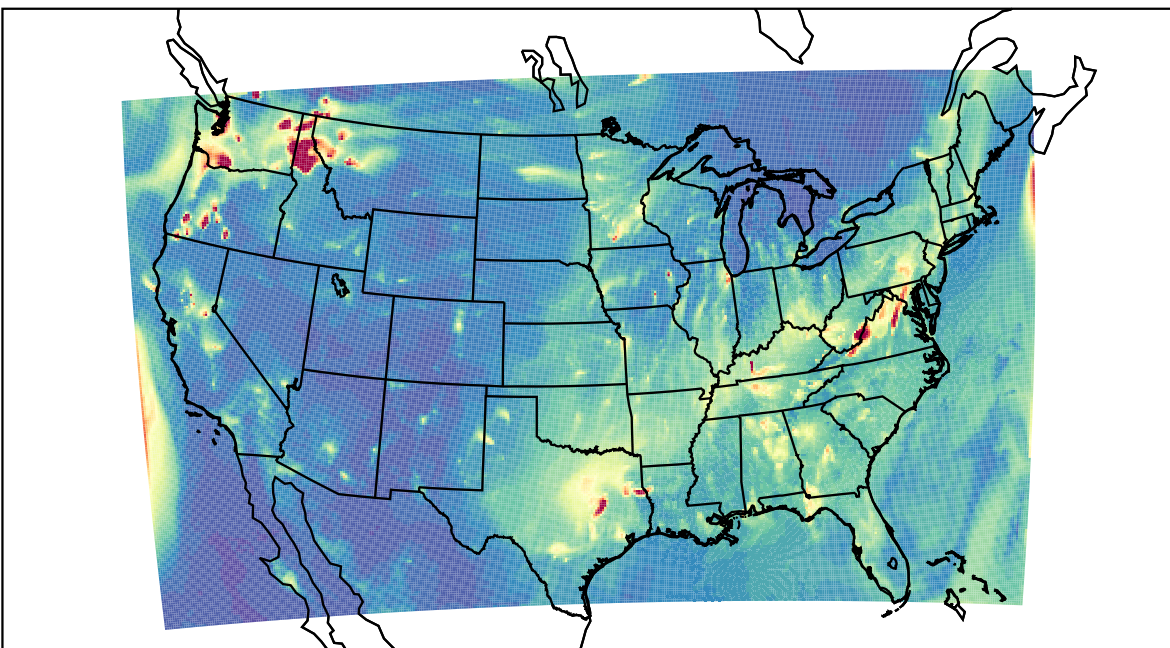
WRF 2023-11-18_04:00:00
