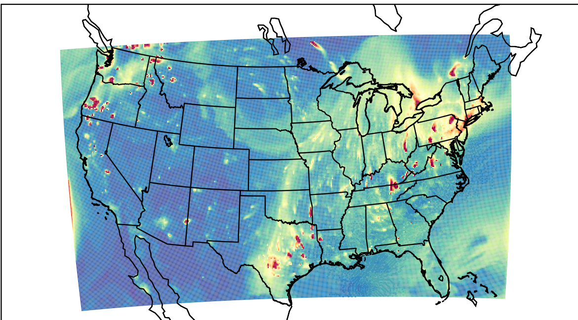
WRF 2023-11-17_01:00:00
