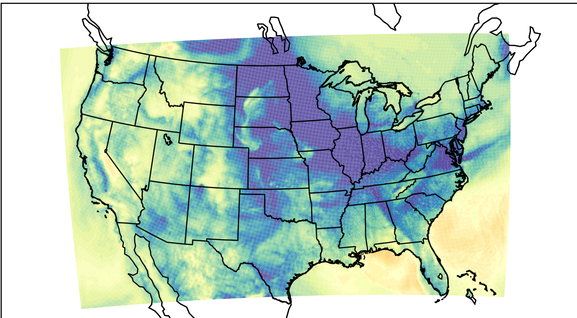
WRF (2023-11-20_10:00:00)
