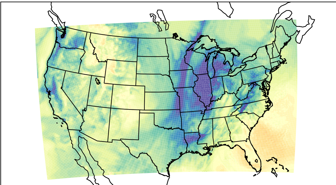
WRF (2023-11-21_18:00:00)
