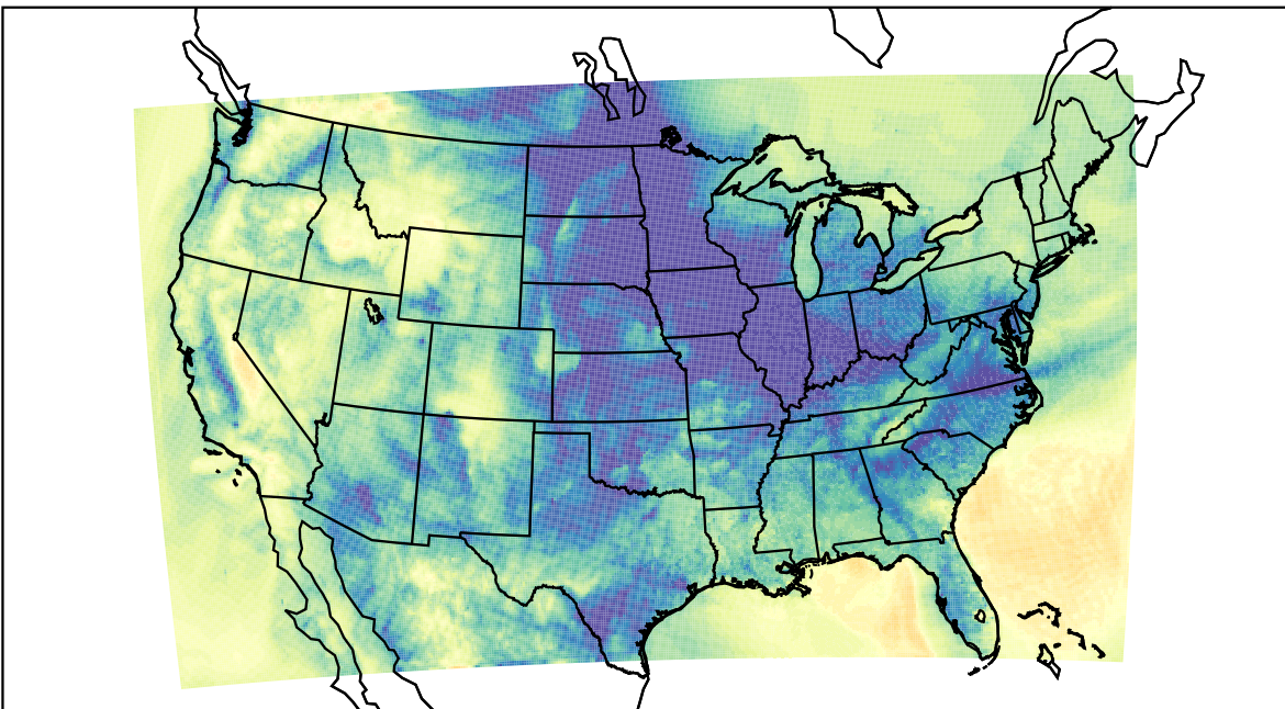
WRF (2023-11-20_14:00:00)
