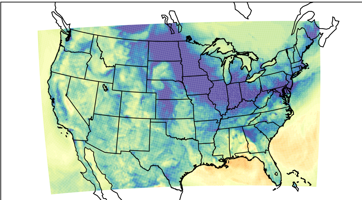
WRF (2023-11-20_04:00:00)
