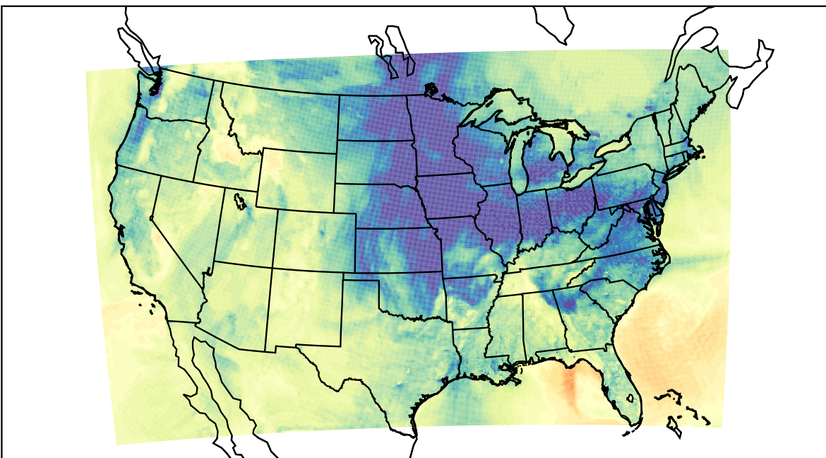
WRF (2023-11-20_23:00:00)
