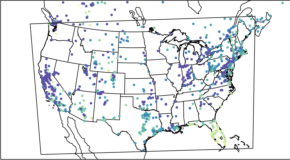
AirNOW (2023-11-21_16:00:00)
