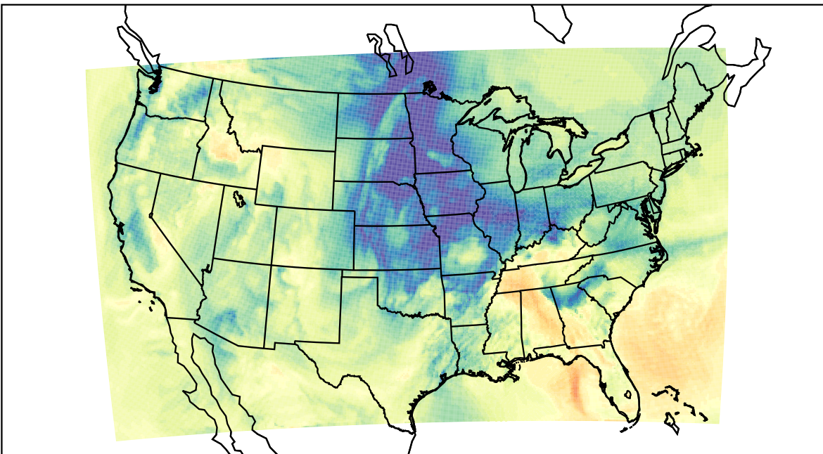
WRF (2023-11-20_19:00:00)
