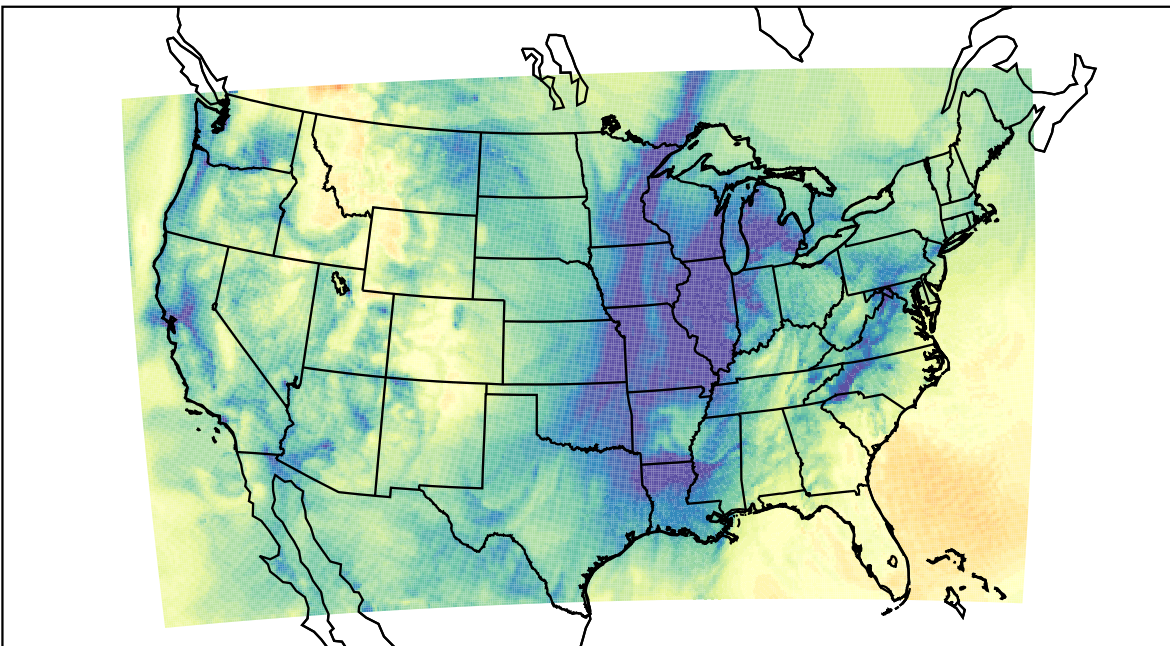
WRF (2023-11-21_16:00:00)
