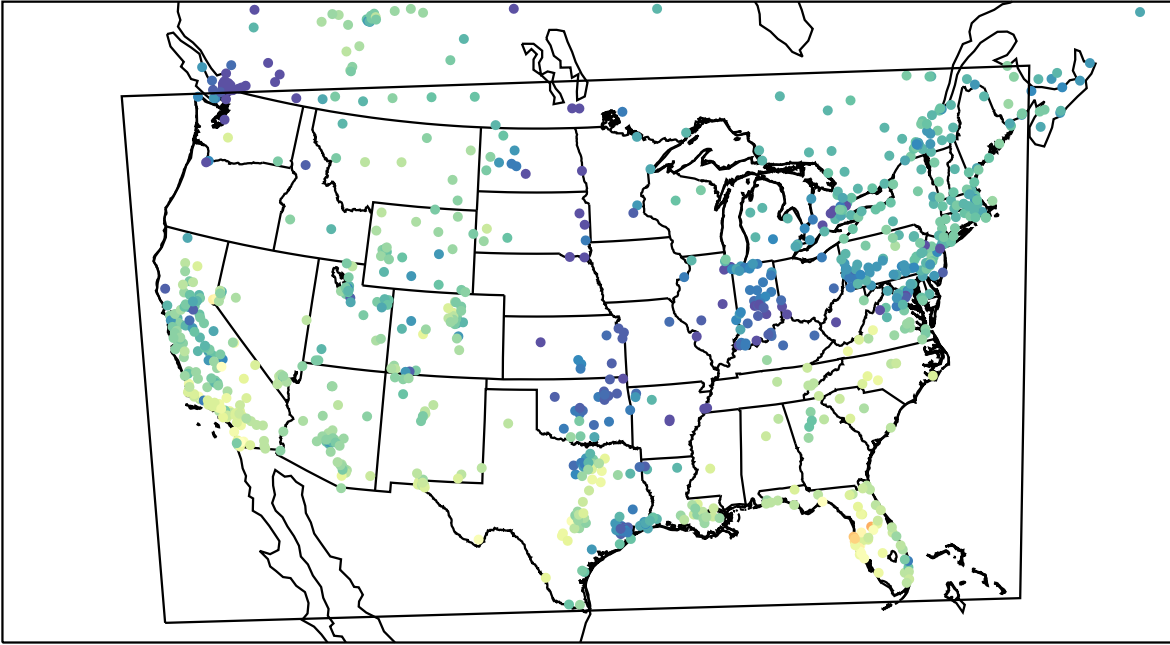
AirNOW (2023-11-20_20:00:00)
