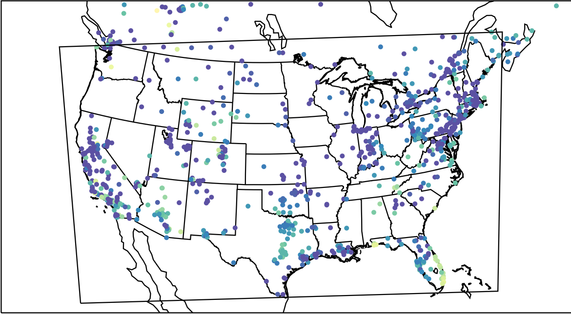
AirNOW (2023-11-21_13:00:00)
