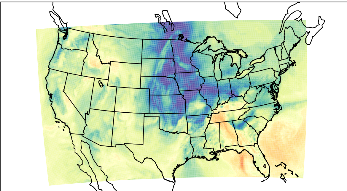
WRF (2023-11-20_20:00:00)
