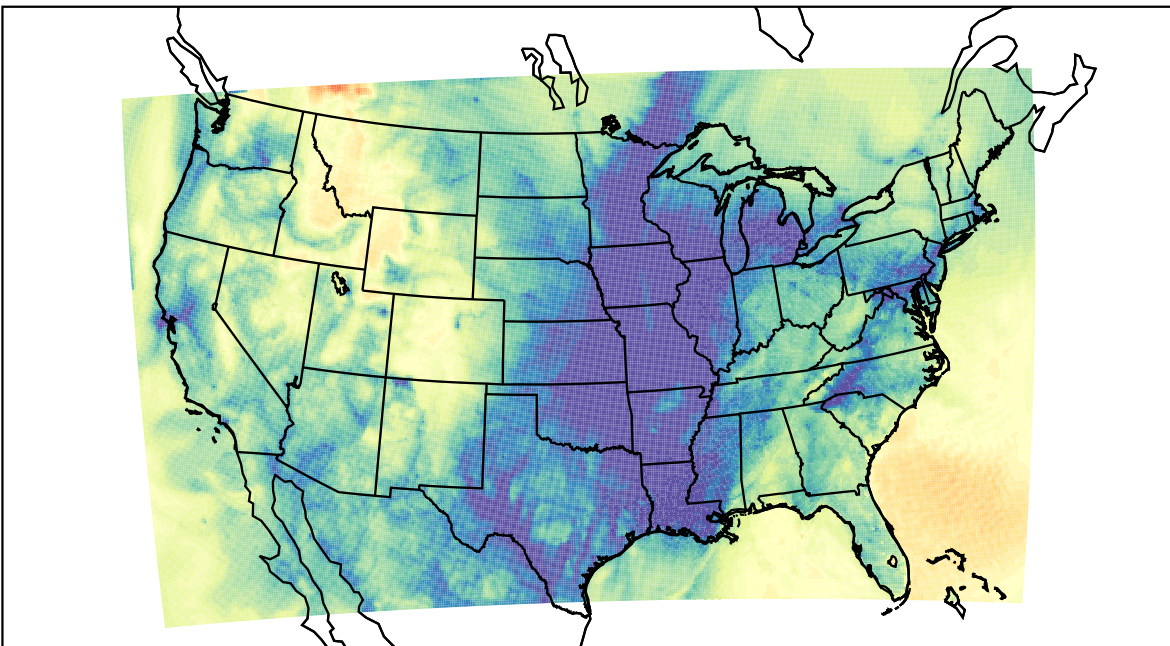
WRF (2023-11-21_13:00:00)
