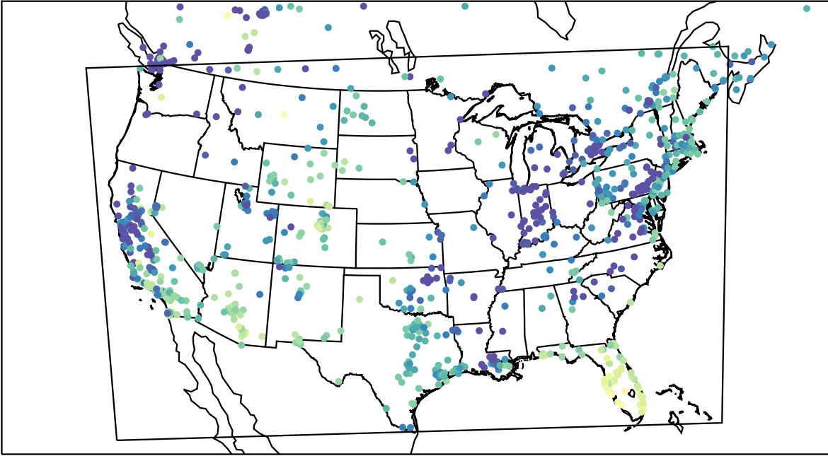
AirNOW (2023-11-21_18:00:00)
