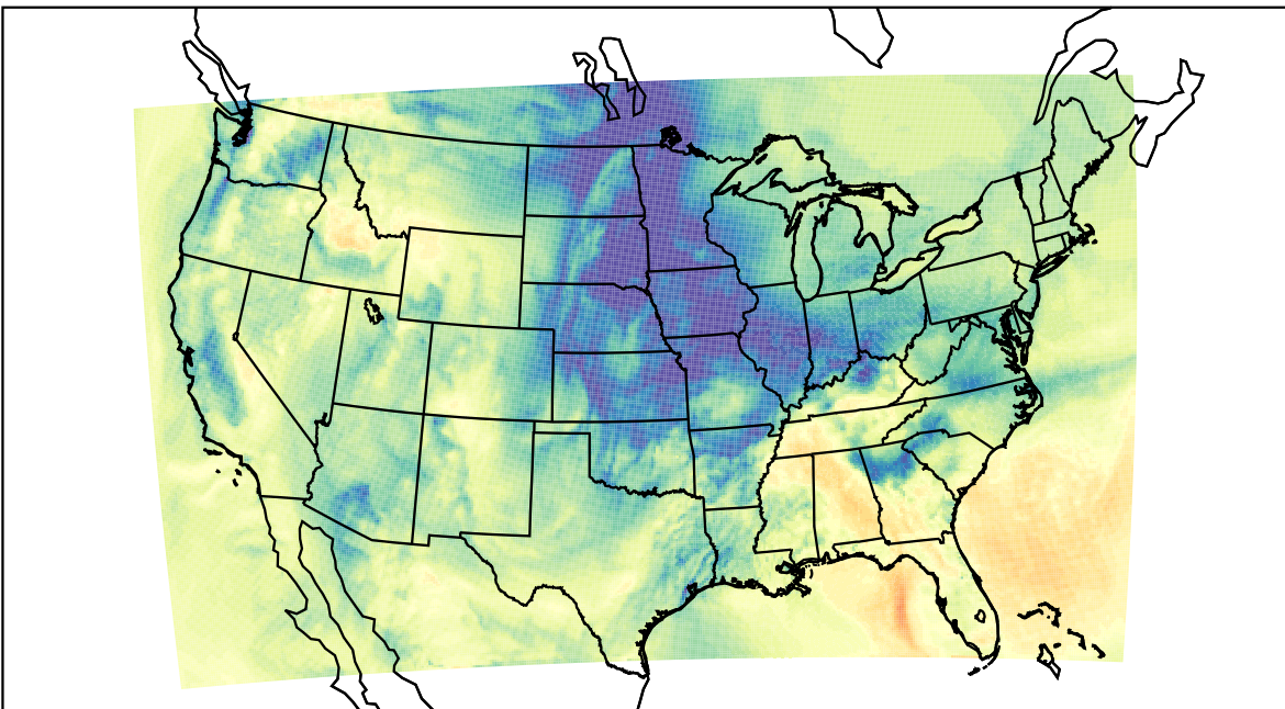
WRF (2023-11-20_18:00:00)
