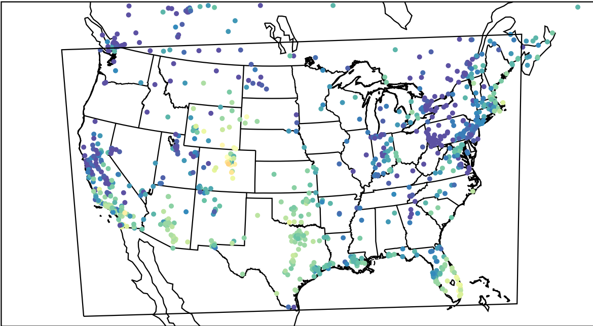
AirNOW (2023-11-22_18:00:00)
