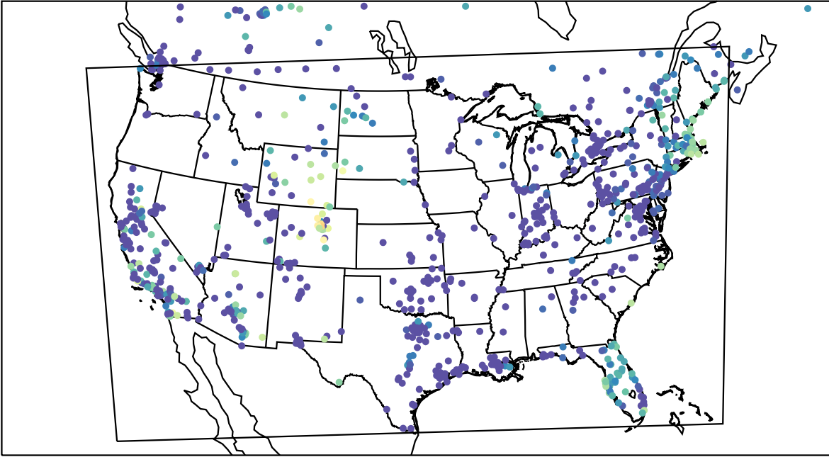
AirNOW (2023-11-22_13:00:00)
