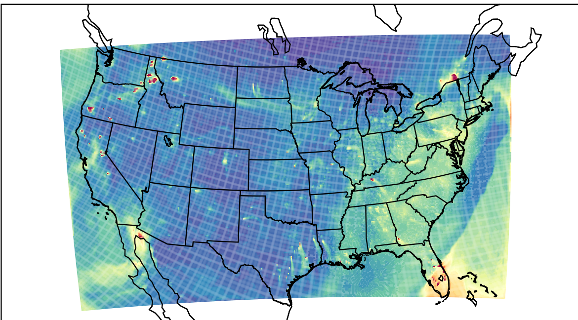
WRF 2023-11-22_23:00:00
