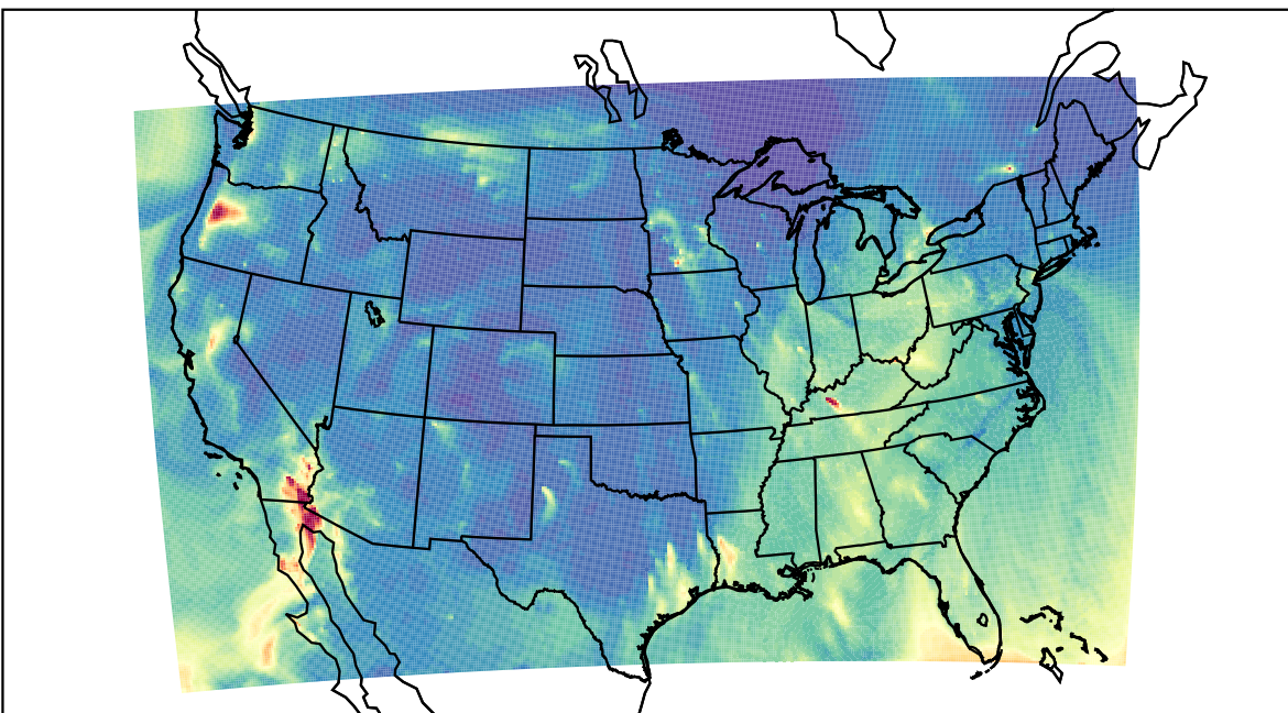
WRF 2023-11-22_10:00:00
