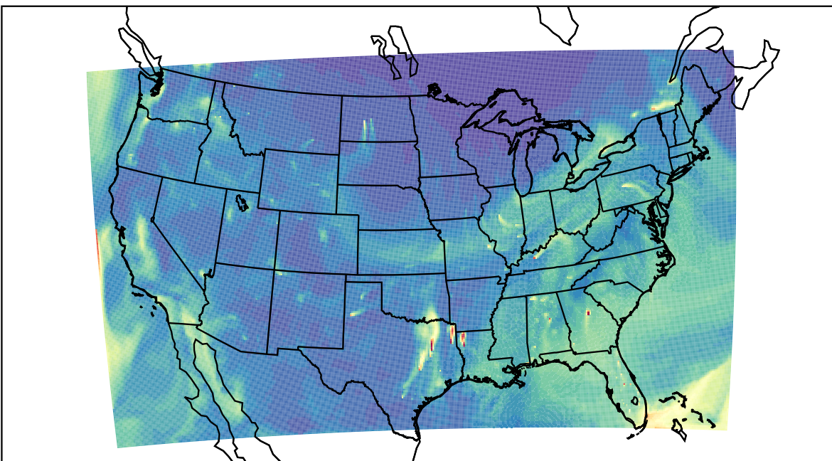
WRF 2023-11-23_18:00:00
