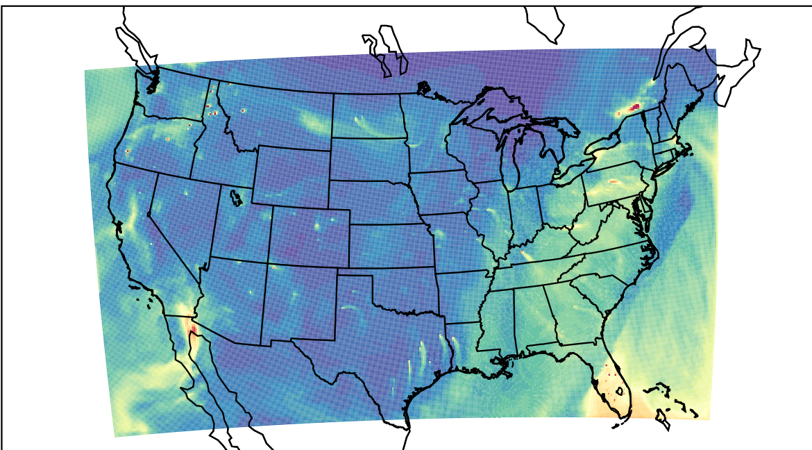
WRF 2023-11-22_19:00:00
