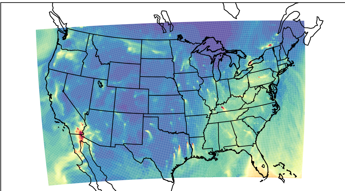
WRF 2023-11-22_15:00:00
