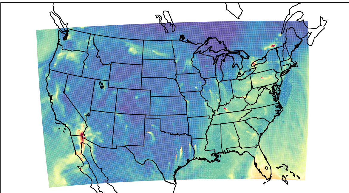
WRF 2023-11-22_16:00:00
