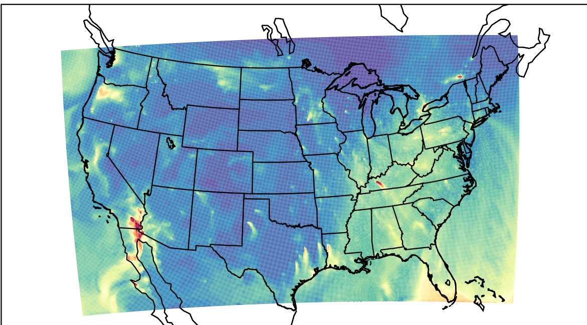
WRF 2023-11-22_13:00:00
