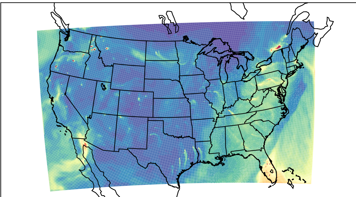
WRF 2023-11-22_20:00:00
