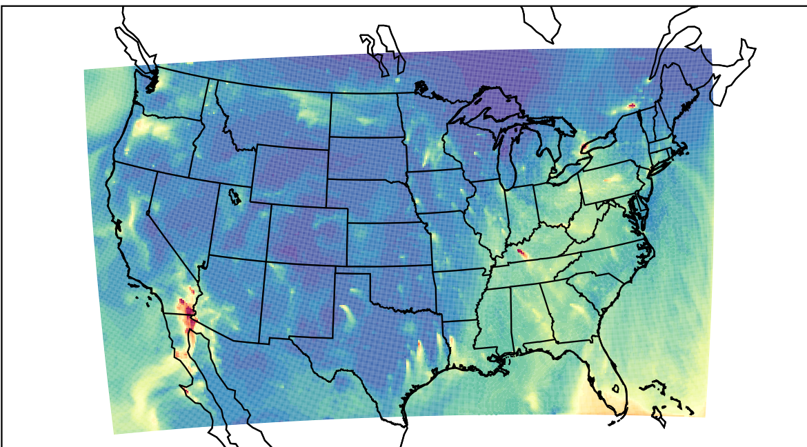
WRF 2023-11-22_14:00:00
