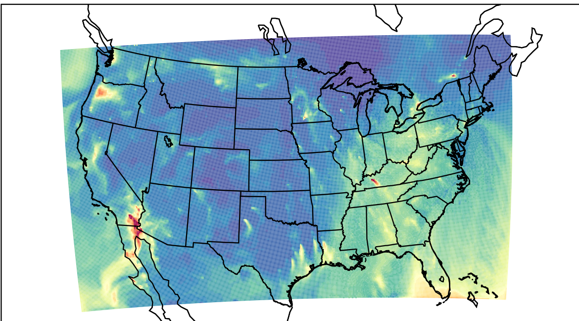
WRF 2023-11-22_12:00:00
