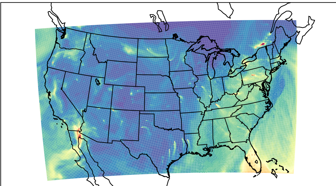
WRF 2023-11-22_18:00:00
