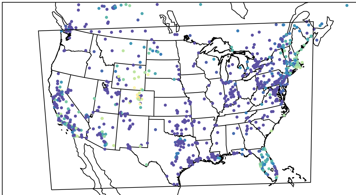
AirNOW (2023-11-22_13:00:00)
