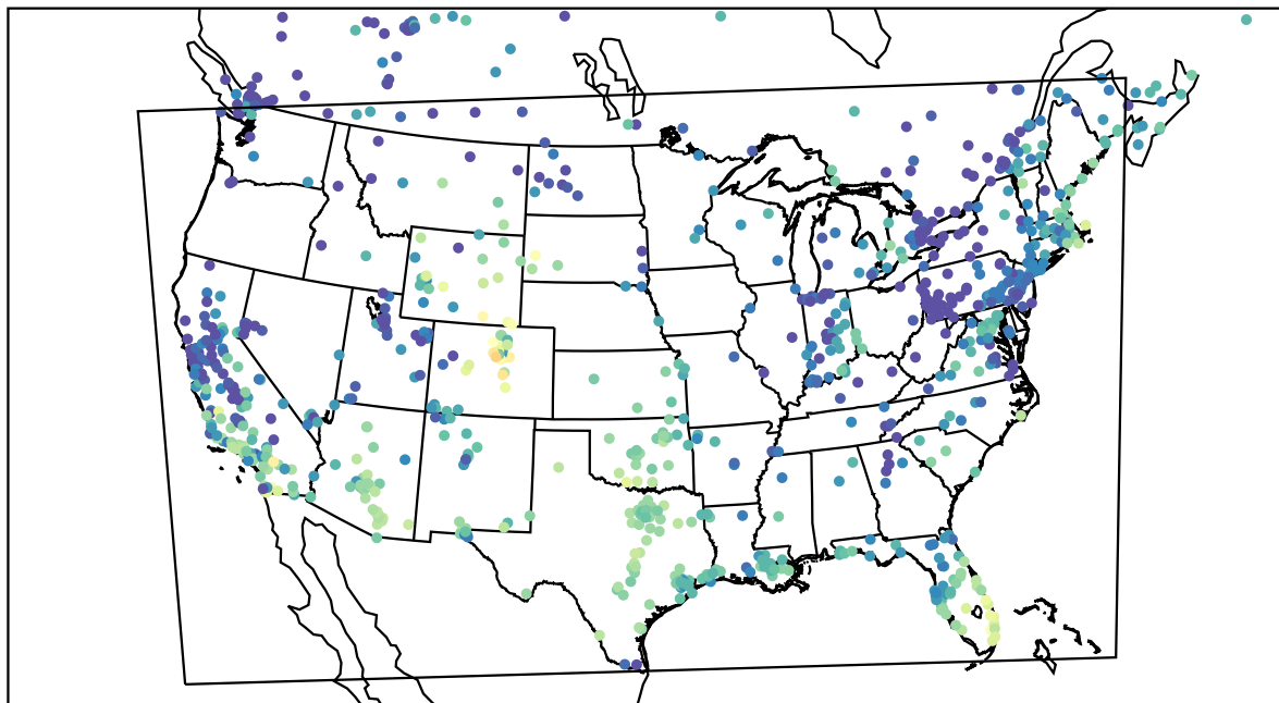
AirNOW (2023-11-22_18:00:00)
