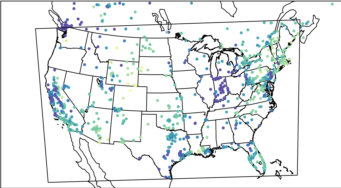
AirNOW (2023-11-26_18:00:00)
