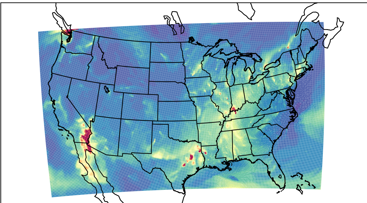
WRF 2023-11-26_10:00:00
