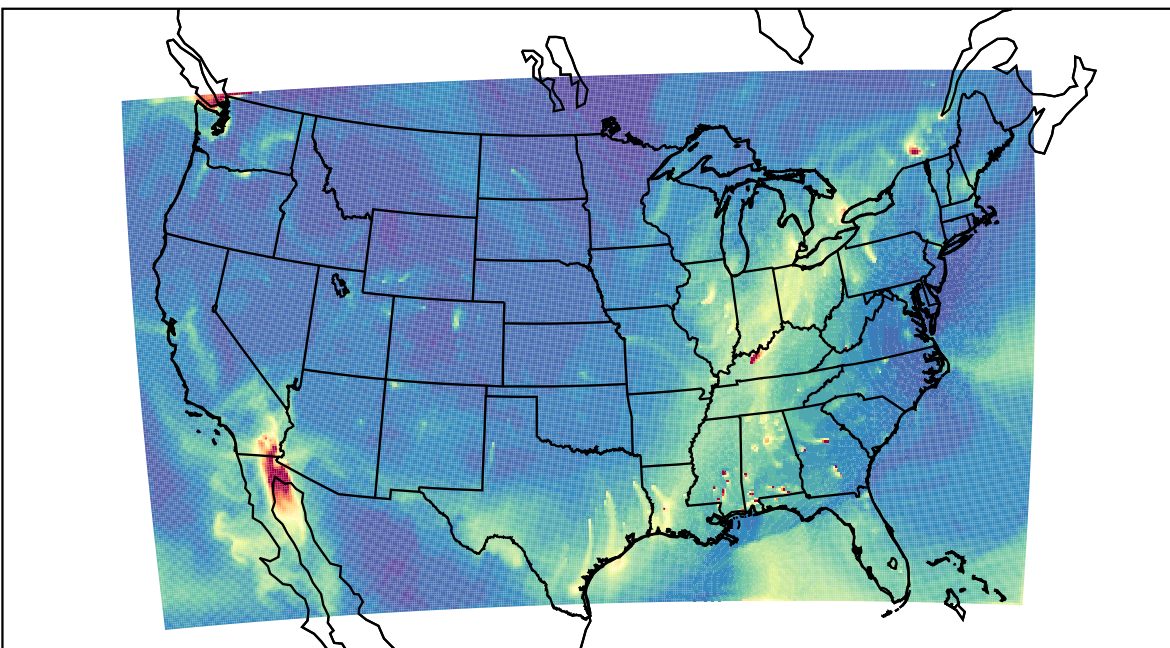
WRF 2023-11-26_19:00:00
