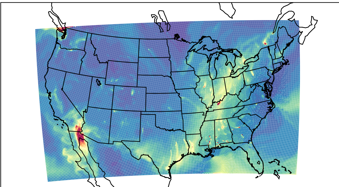
WRF 2023-11-26_18:00:00
