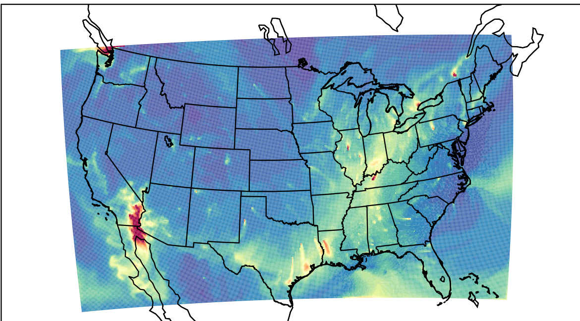
WRF 2023-11-26_16:00:00
