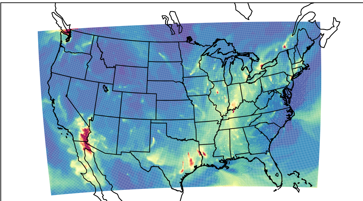
WRF 2023-11-26_14:00:00
