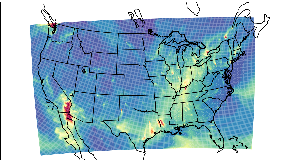
WRF 2023-11-26_15:00:00
