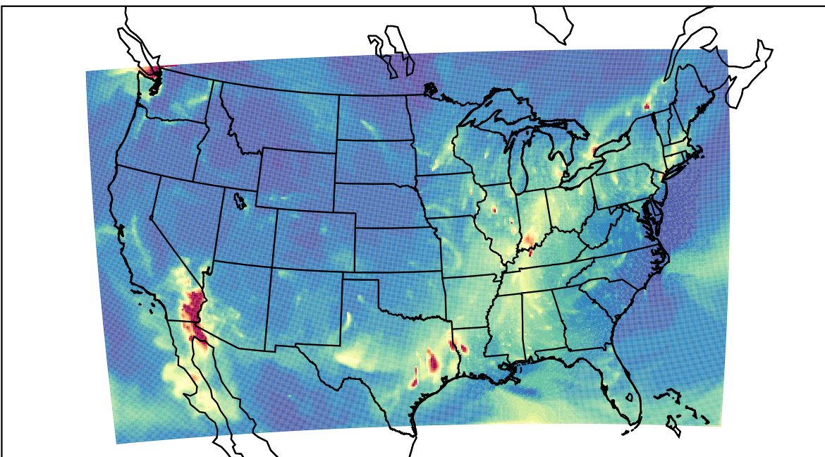
WRF 2023-11-26_13:00:00
