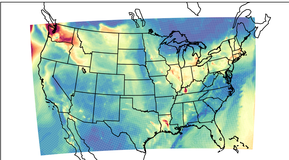
WRF 2023-12-03_10:00:00
