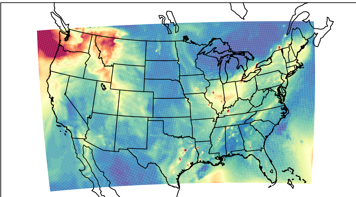
WRF 2023-12-02_18:00:00
