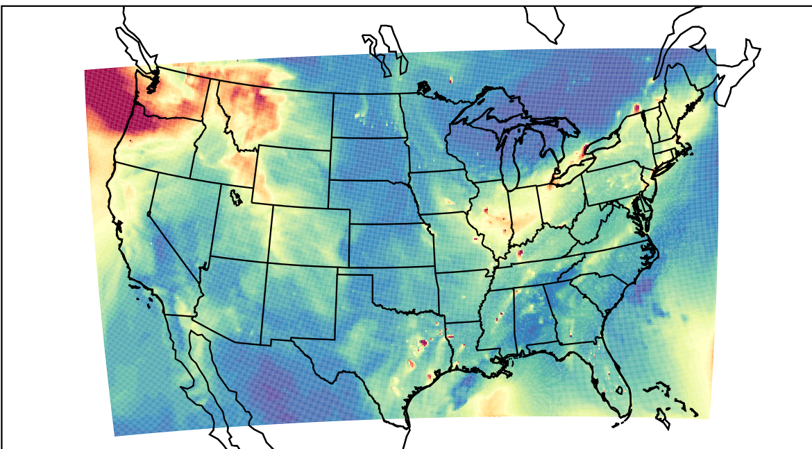
WRF 2023-12-02_19:00:00
