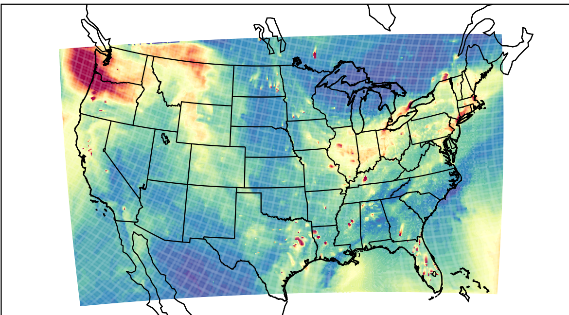
WRF 2023-12-02_23:00:00
