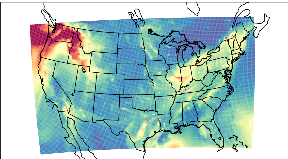
WRF 2023-12-02_14:00:00
