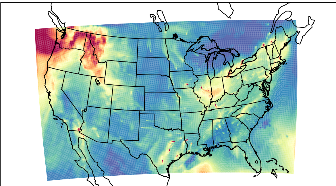
WRF 2023-12-02_16:00:00
