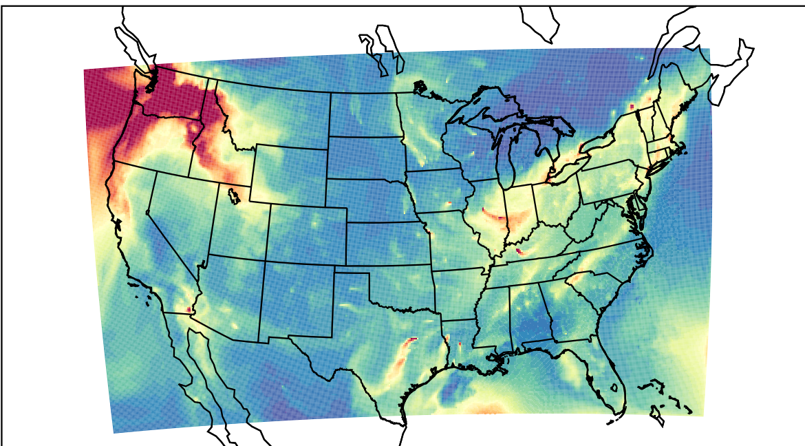
WRF 2023-12-02_13:00:00
