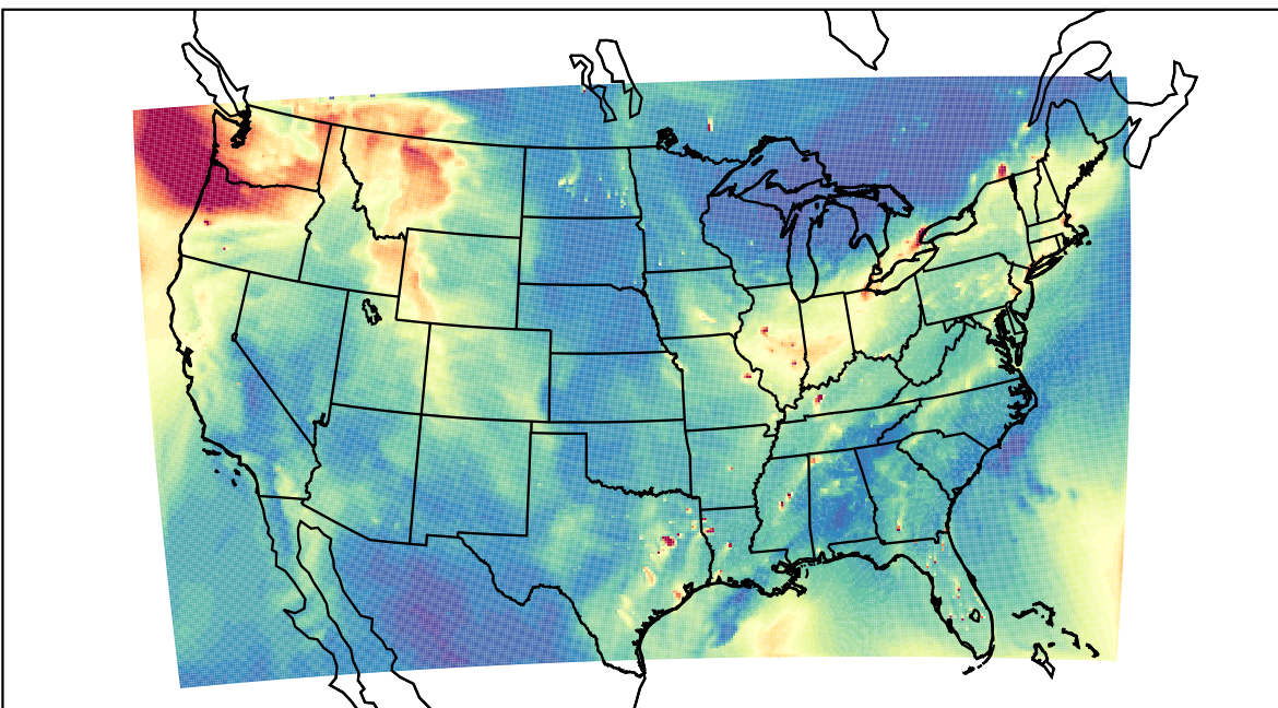
WRF 2023-12-02_20:00:00
