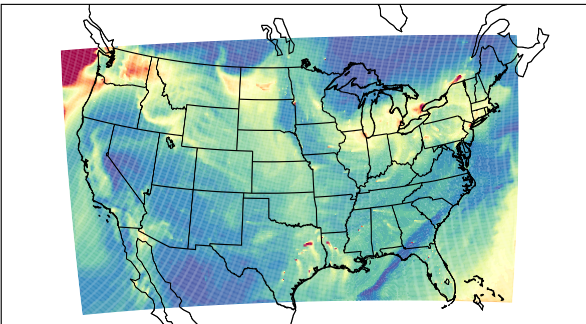
WRF 2023-12-03_18:00:00
