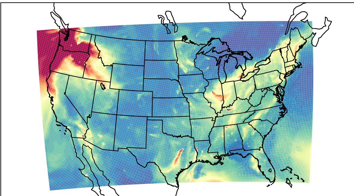
WRF 2023-12-02_10:00:00
