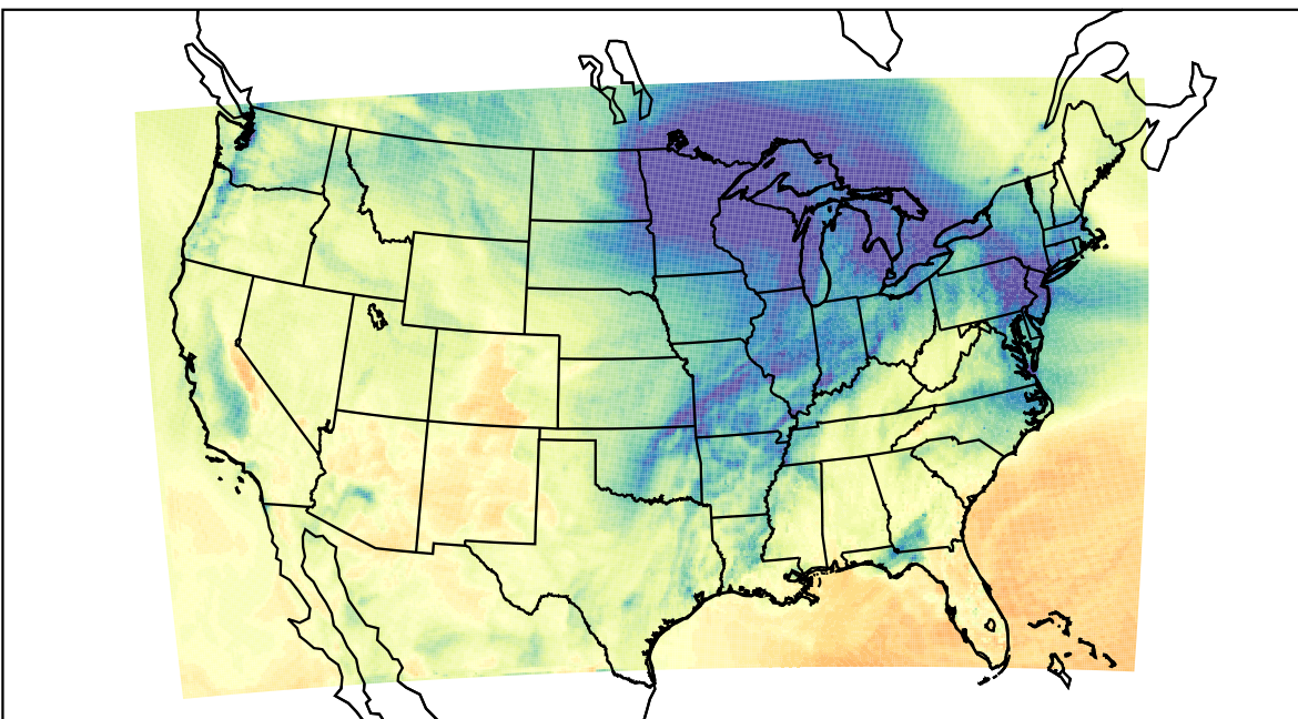
WRF (2023-12-08_20:00:00)
