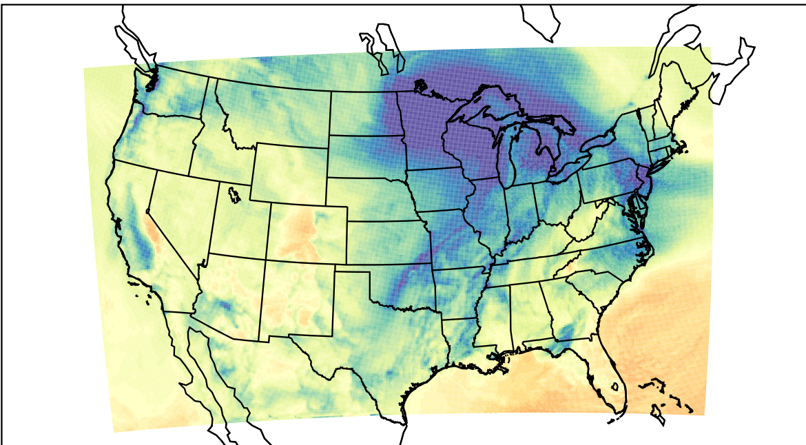
WRF (2023-12-08_18:00:00)
