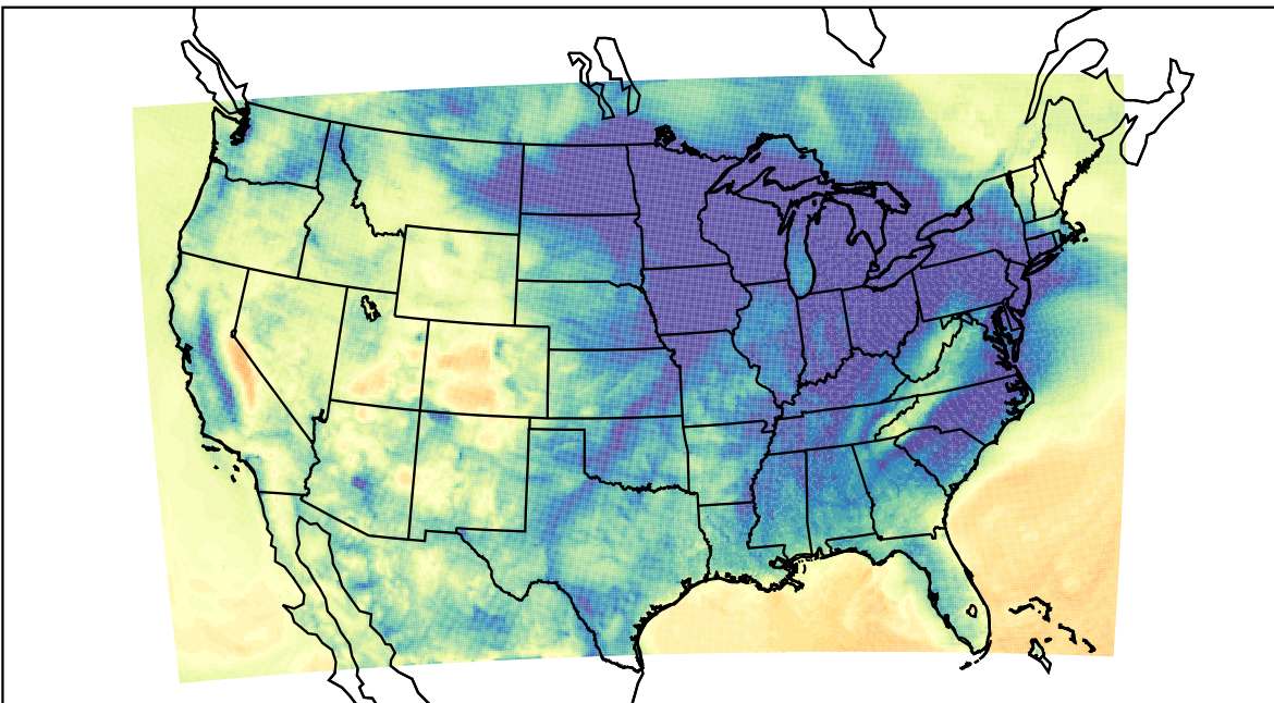
WRF (2023-12-08_10:00:00)
