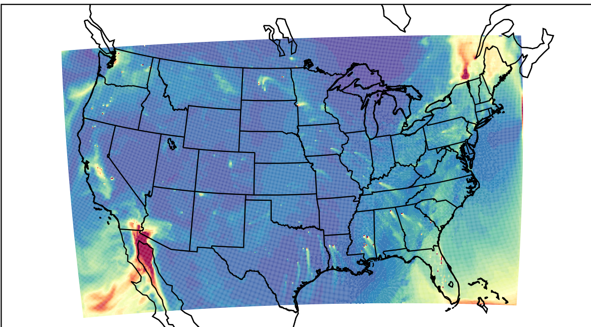
WRF 2023-12-10_20:00:00
