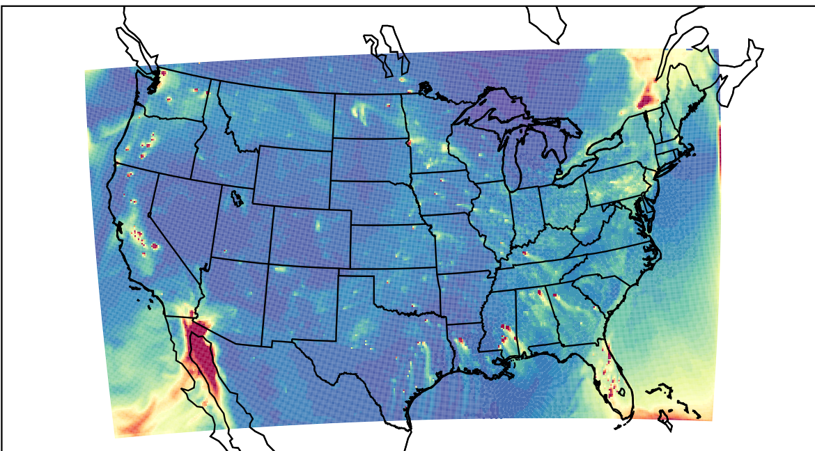
WRF 2023-12-10_23:00:00
