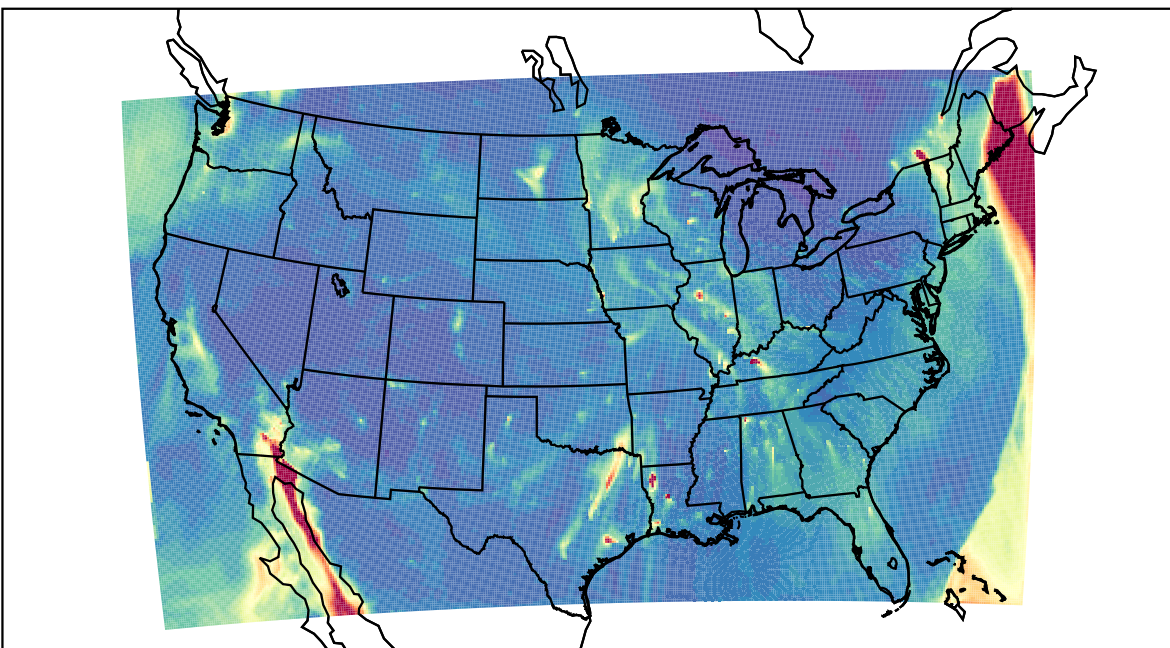
WRF 2023-12-11_15:00:00
