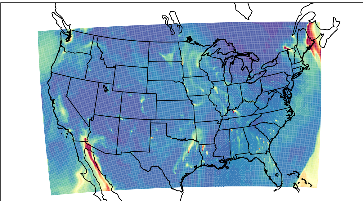
WRF 2023-12-11_18:00:00
