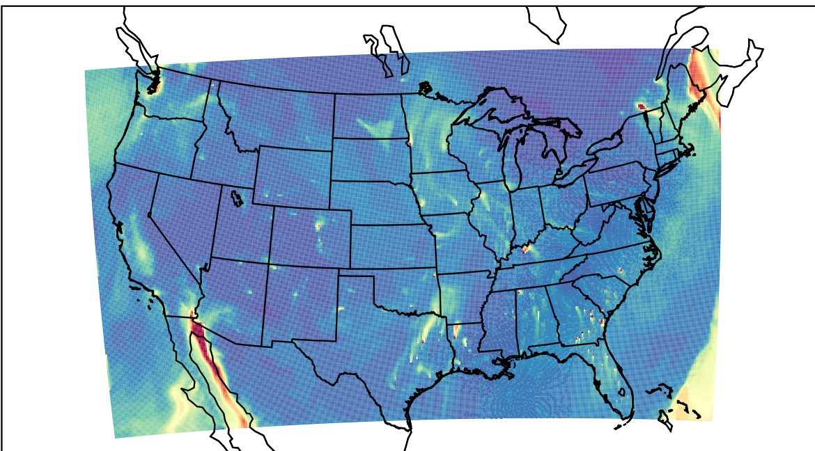
WRF 2023-12-11_19:00:00
