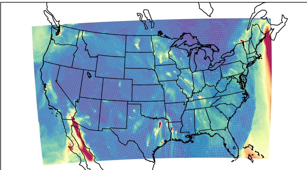
WRF 2023-12-11_10:00:00
