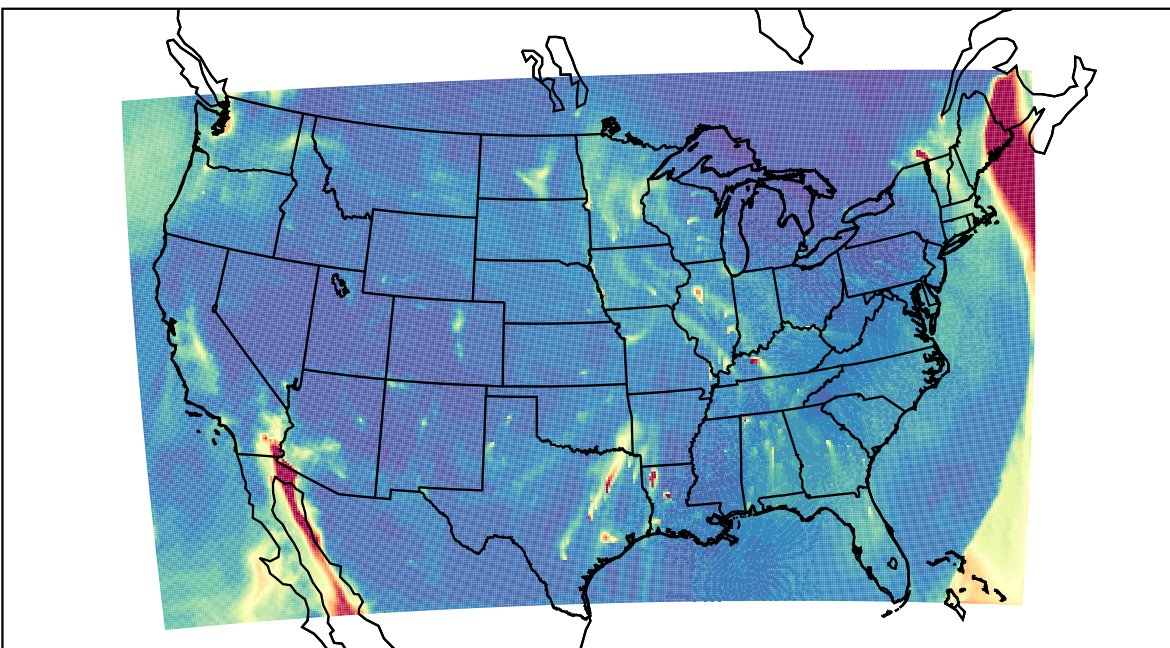
WRF 2023-12-11_16:00:00
