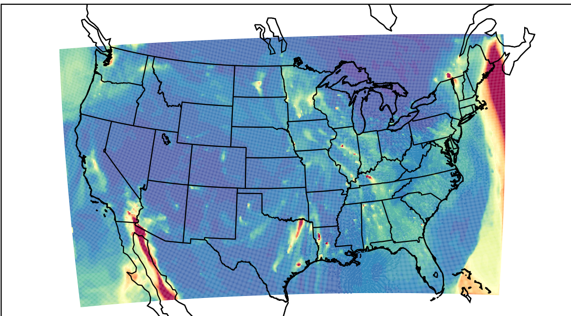
WRF 2023-12-11_13:00:00
