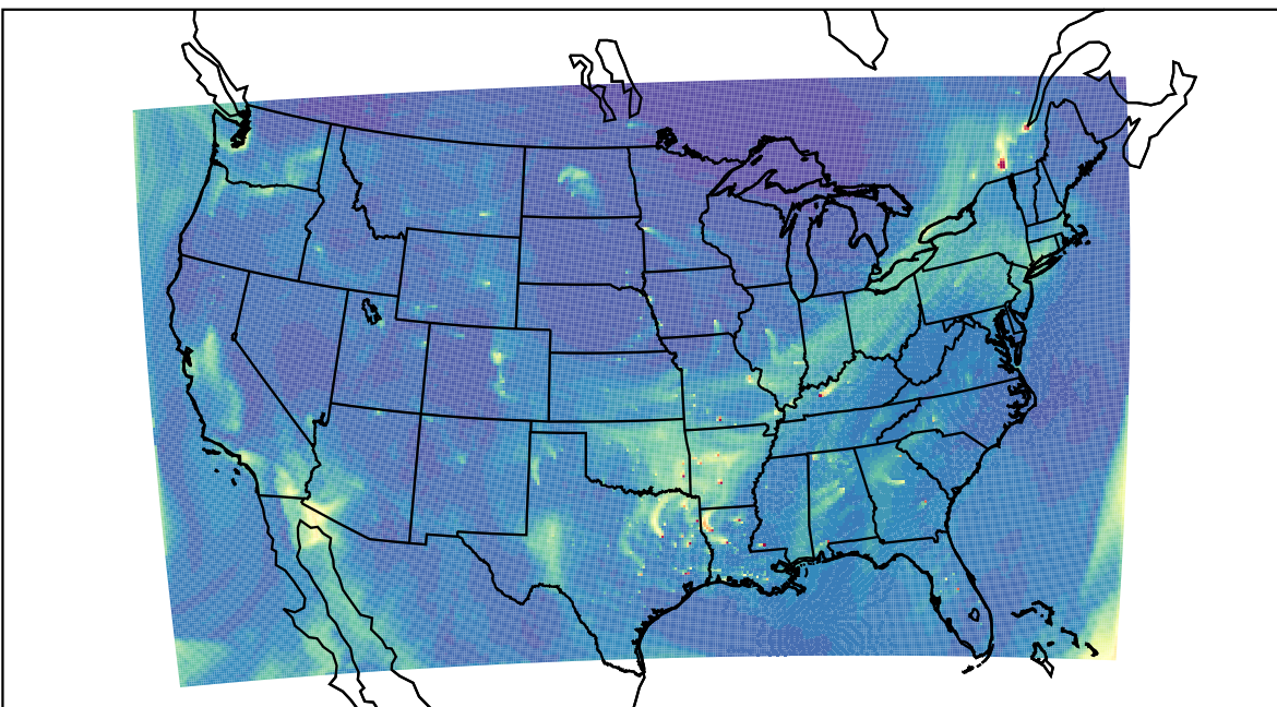
WRF 2023-12-12_19:00:00
