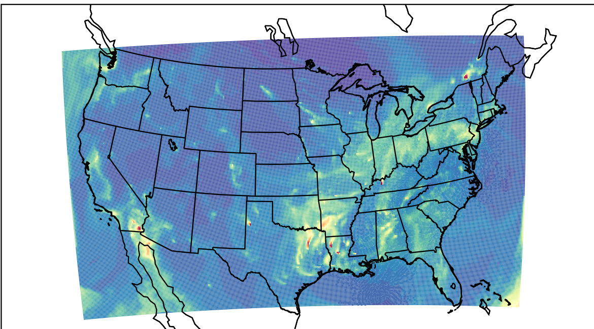
WRF 2023-12-12_13:00:00
