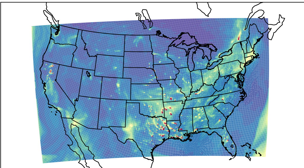
WRF 2023-12-12_23:00:00
