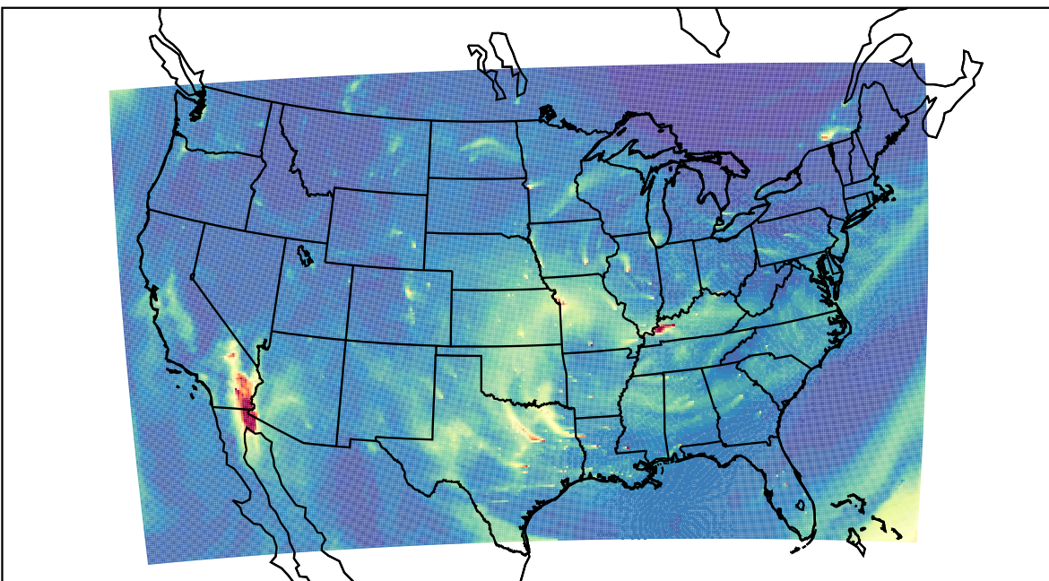
WRF 2023-12-13_18:00:00
