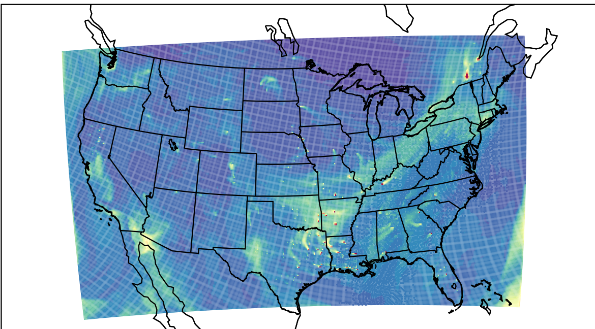
WRF 2023-12-12_20:00:00
