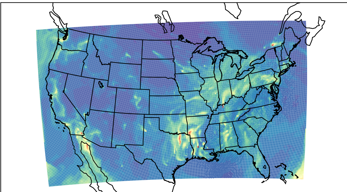
WRF 2023-12-12_10:00:00
