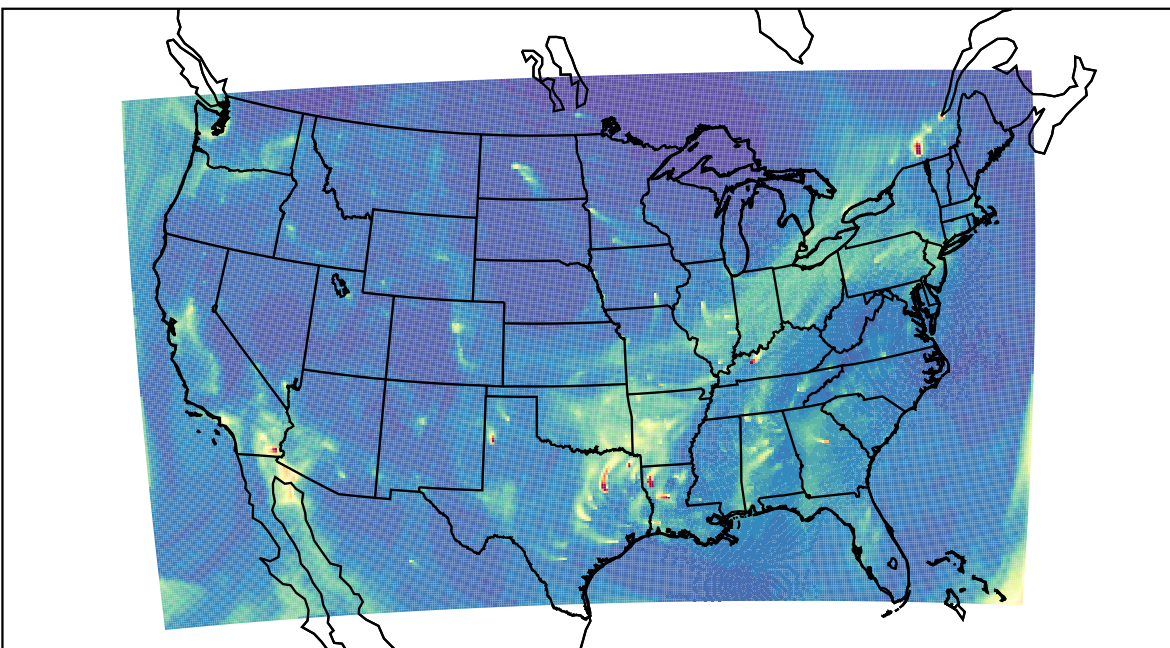
WRF 2023-12-12_16:00:00
