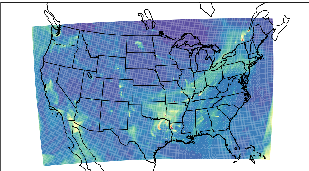
WRF 2023-12-12_18:00:00
