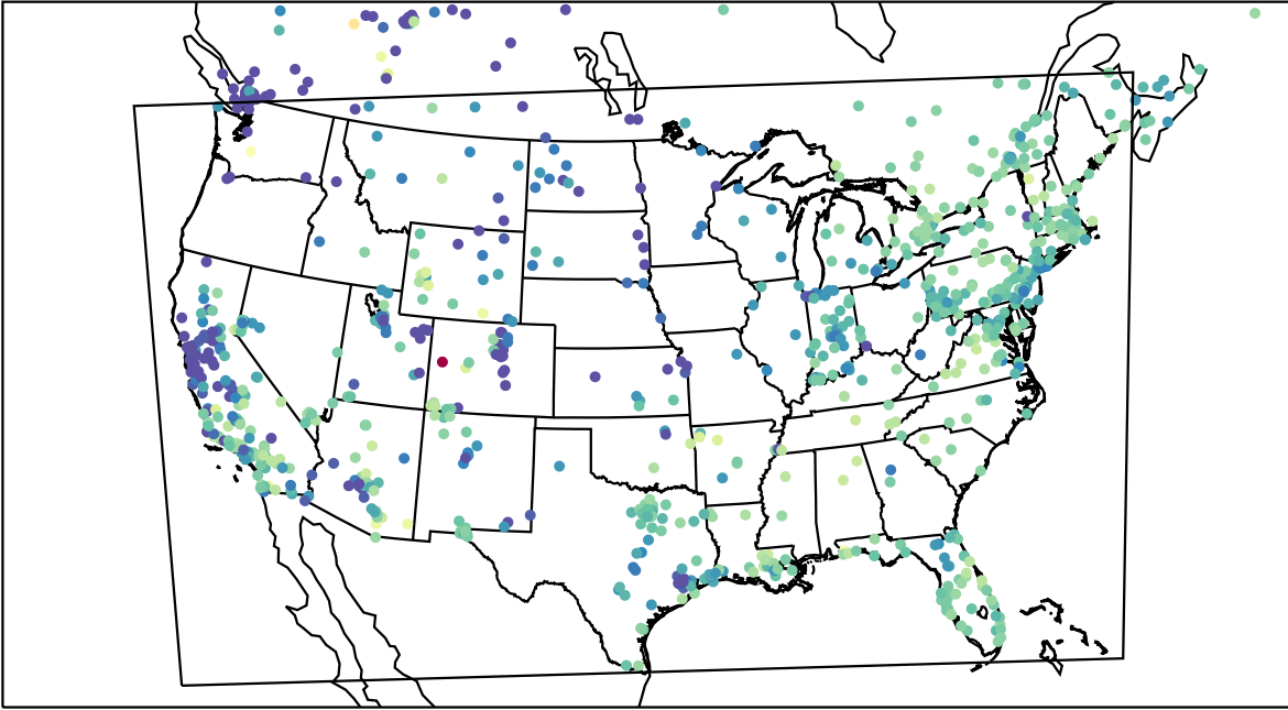
AirNOW (2023-12-13_18:00:00)
