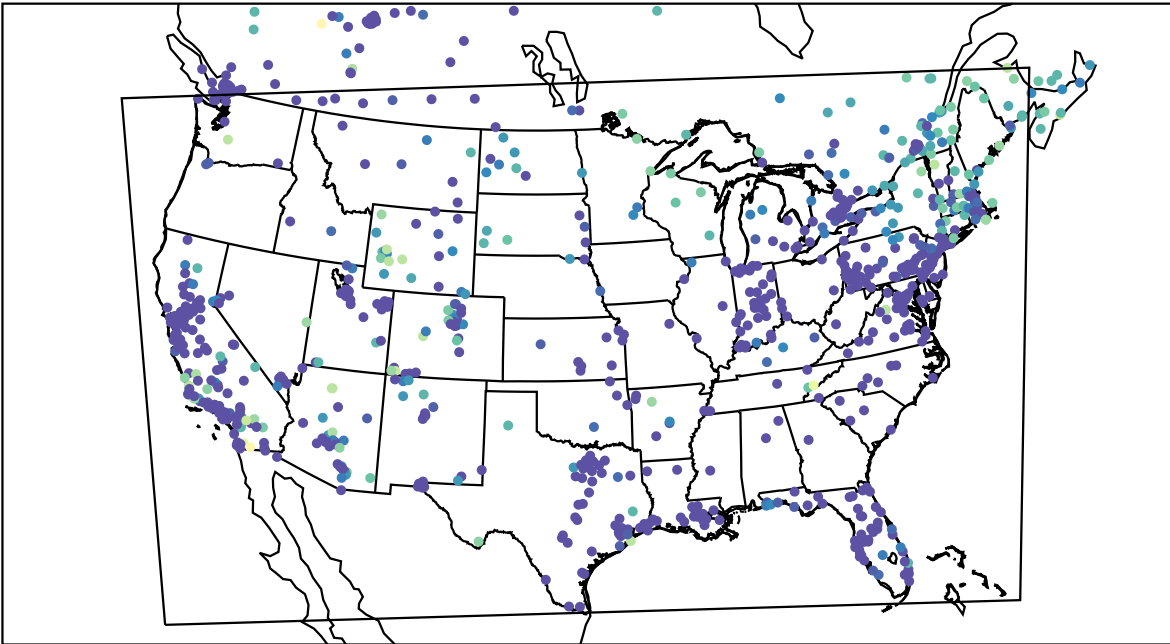
AirNOW (2023-12-12_13:00:00)
