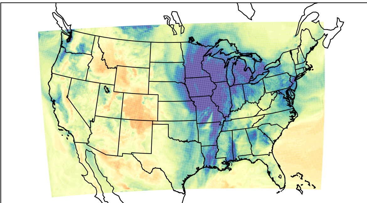
WRF (2023-12-16_20:00:00)
